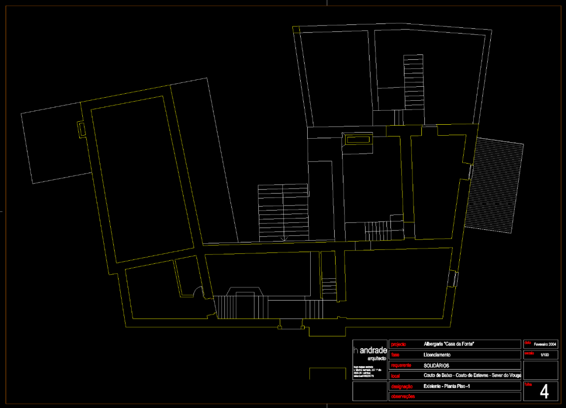
Figura 12 - Nível -1 da casa
