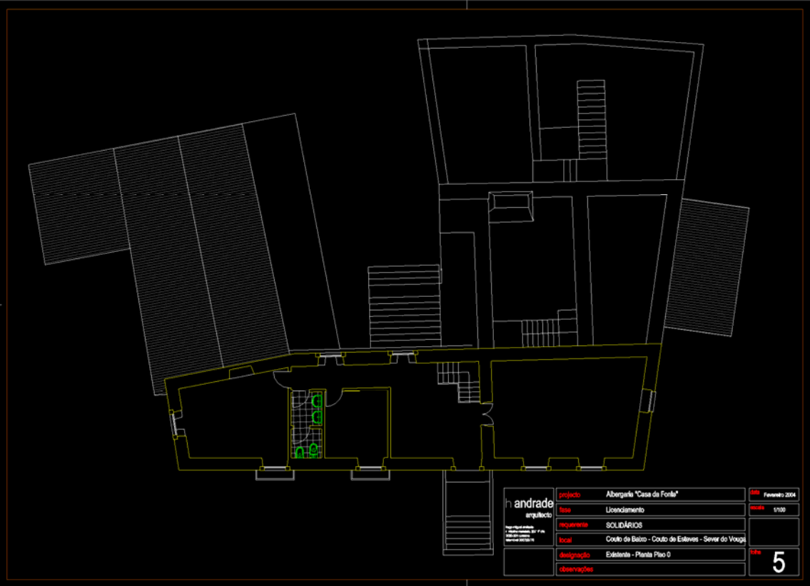
Figura 13 - Nível 0 da casa
