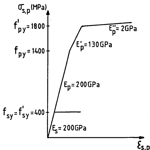
Fig. 6.2 - Diagramas tensões-extensões para o aço das armaduras ordinária e de pré-esforço.
