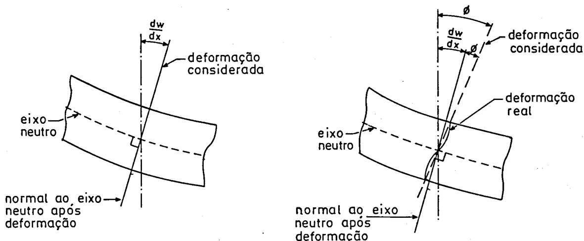
b) Elemento de viga de Timoshenko.
