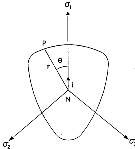
Fig. 4.2 - Projecção da intersecção da superfície de resistência com os planos de desvio.
