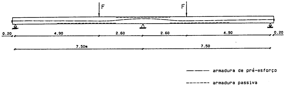
Fig. 5.11 - Geometria das vigas e cargas aplicadas.
