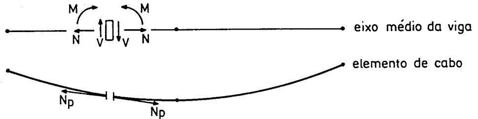
Fig. 2.12 - Convenção de sinais para os esforços.
