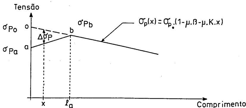
Fig. 3.6 - Perdas por escorregamento nos dispositivos de amarração.
