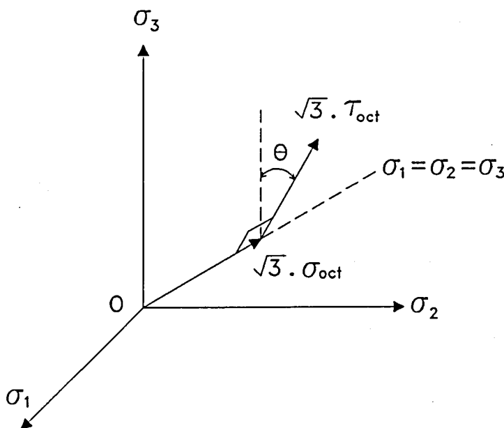
Fig. 4.3 - Interpretação física e geométrica de (\xi, r, \theta) e (\sigma_{oct}, \tau_{oct}, \theta) .
