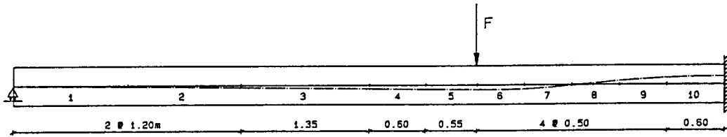
a) Discretização por elementos de viga (viga A).
