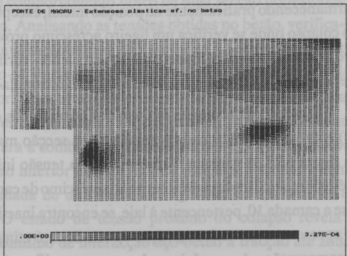
Fig. 6.23 - Distribuição das extensões plásticas equivalentes no betão (continuação).
