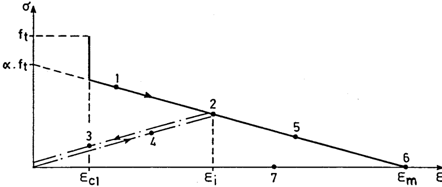
Fig. 4.18 - Diagrama de retenção de tensões de tracção para o betão fendilhado.
