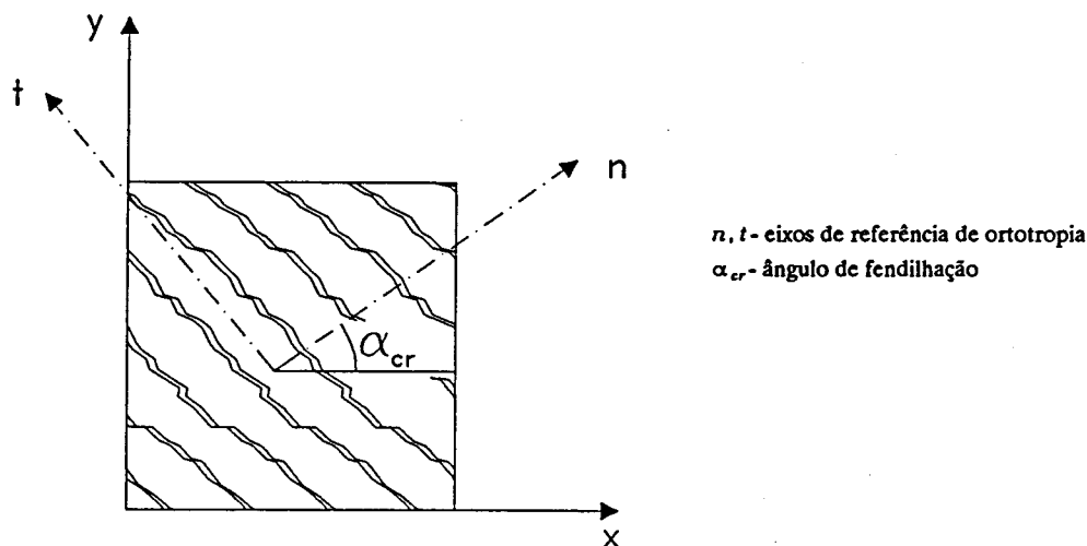
Fig. 4.11 - Direcção de fendilhação.
