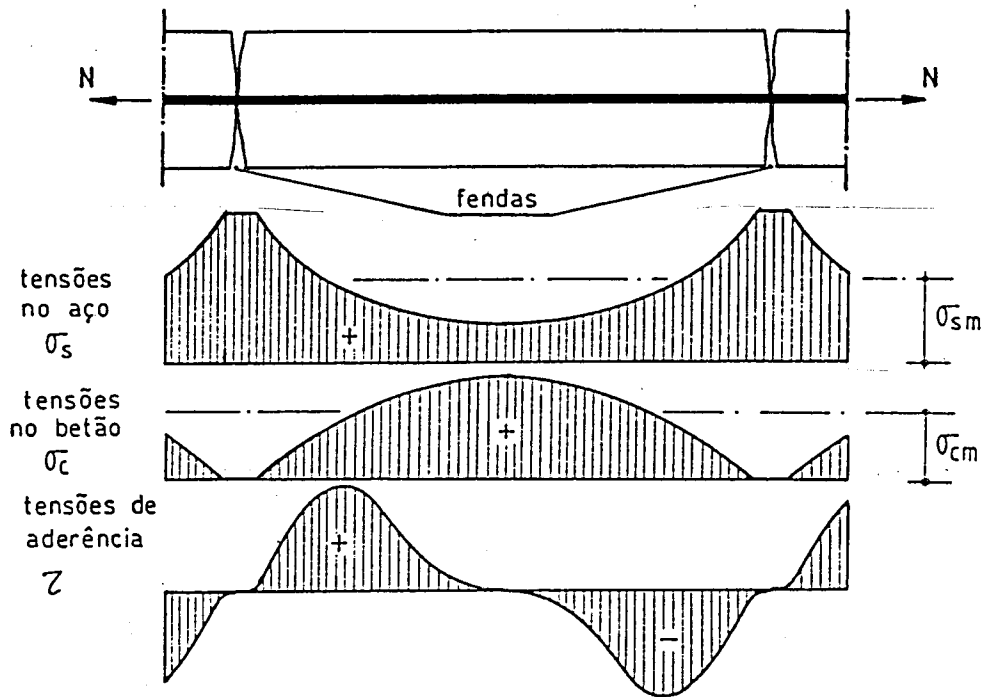
Fig. 4.14 - Representação esquemática da distribuição de tensões entre fendas.
