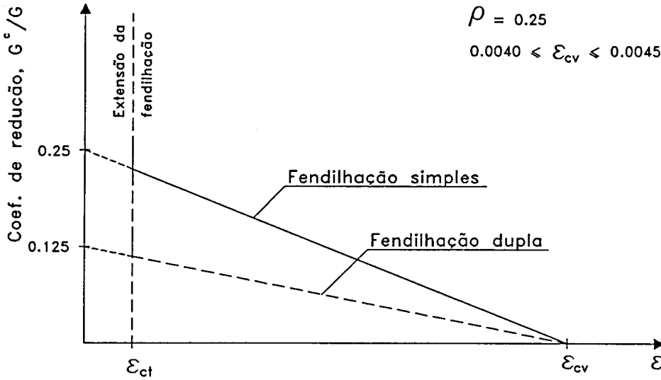
Fig. 4.20 - Coeficiente de retenção da rigidez ao corte no betão fendilhado.
