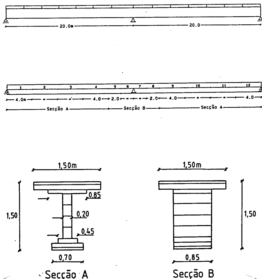
Fig. 3.12 - Viga contínua de dois vãos com secção variável. Geometria, carregamento e malha de elementos finitos.
