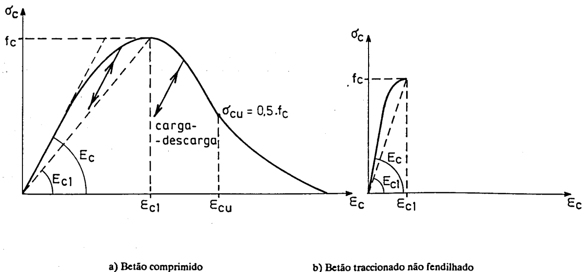
Fig. 4.8 - Representação unidimensional das relações constitutivas do betão definidas no presente modelo.
