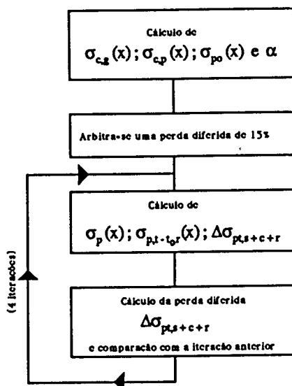
Fig. 3.7 - Cálculo das perdas diferidas.
