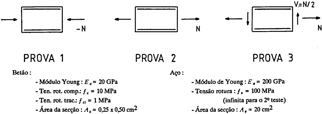
Fig. 5.7 - Testes de carga e descarga em provetes de betão armado. Condições de carga.
