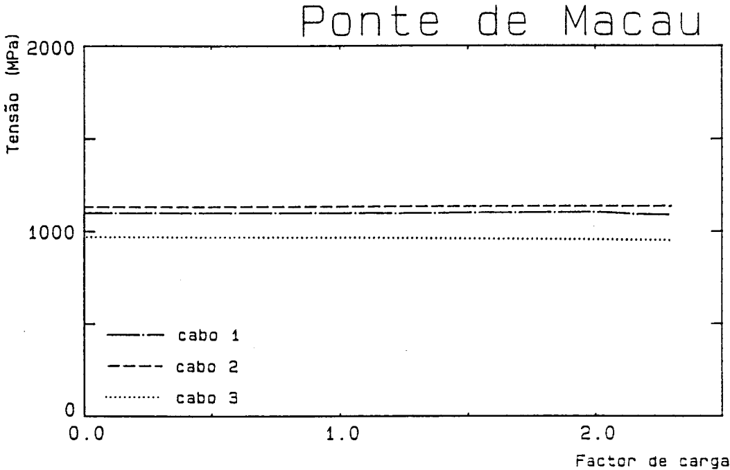
Fig. 6.26 - Curvas carga-tensões nas armaduras (continuação).
