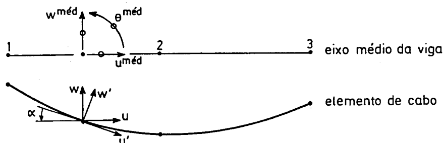
Fig. 2.11 - Campo de deslocamentos do elemento.
