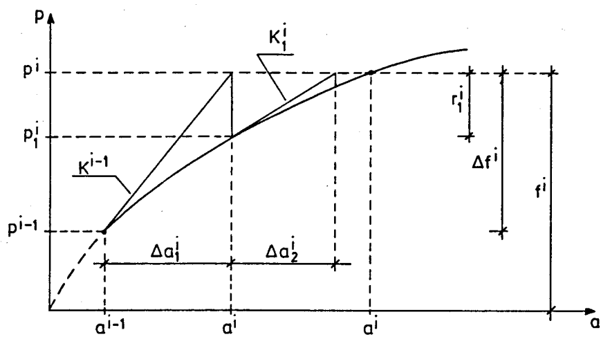
Fig. 5.2 - Processo incremental e iterativo na solução não linear de um problema unidimensional. Método de Newton-Raphson.
