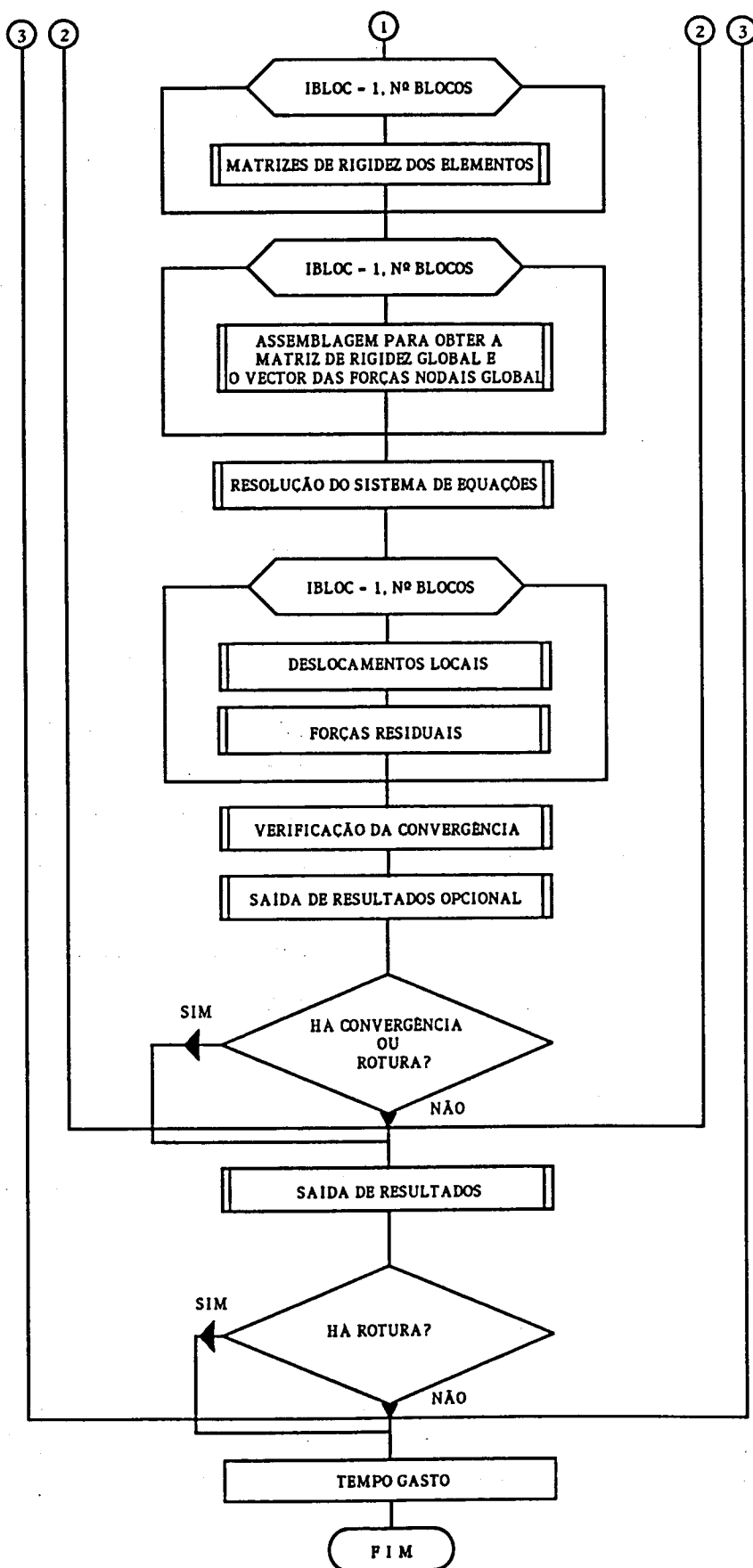
Fig. 5.1 - Fluxograma do programa PCBEAM (continuação).
