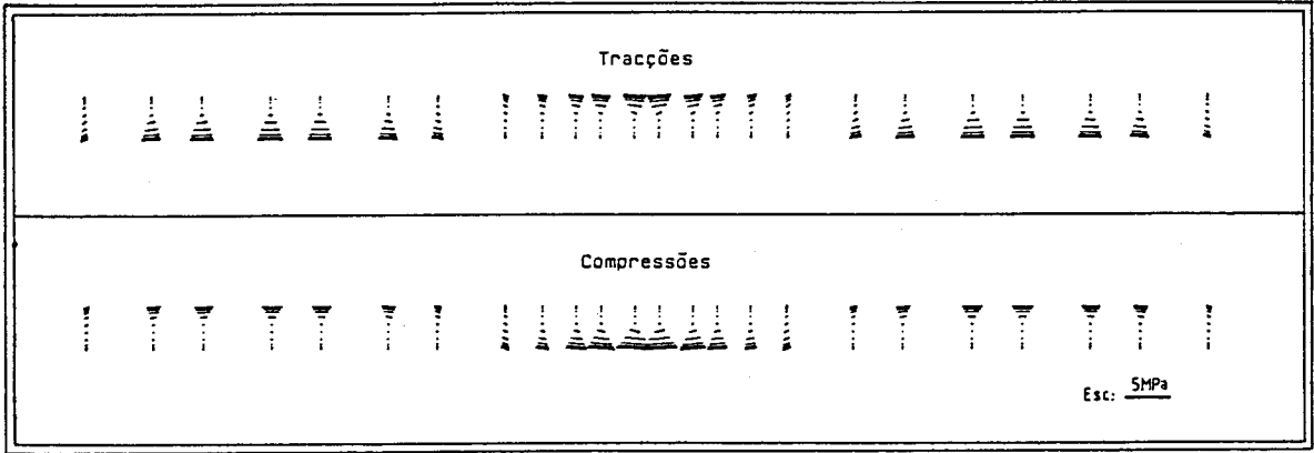
a) Tensões principais para as ações permanentes iniciais ( G_1 ).
