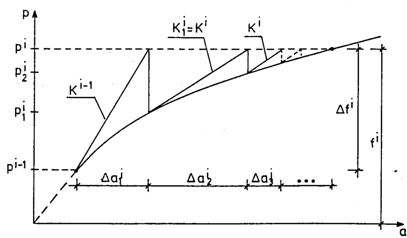
Fig. 5.4 - Método de Newton-Raphson modificado na segunda iteração.
