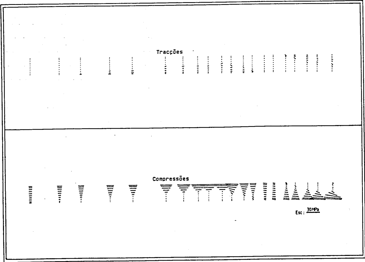
c) Tensões principais.
