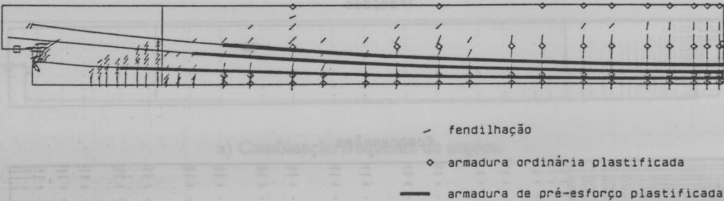
Fig. 6.22 - Configuração da fendilhação e identificação das armaduras plasticadas. Acções majoradas de \gamma = 2,30 .
