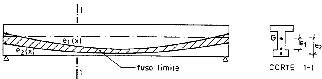
Fig. 3.4 - Fuso limite de uma viga simplesmente apoiada.
