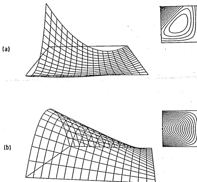
Fig. 2.17 - Funções de forma quadráticas (Serendipity): a) nó de canto; b) nó intermédio.
