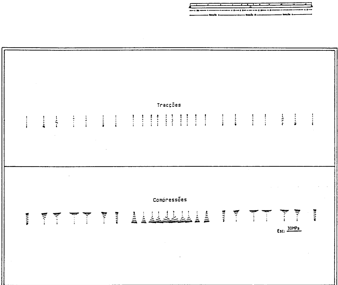
a) Tensões principais para \gamma = 2,28
