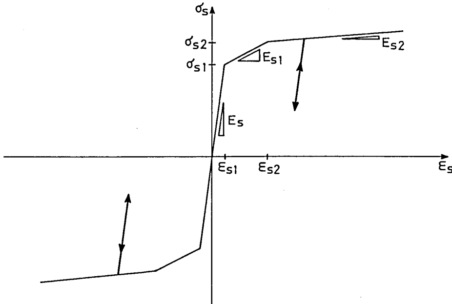
Fig. 4.27 - Diagrama tensões-deformações trilinear para o aço.
