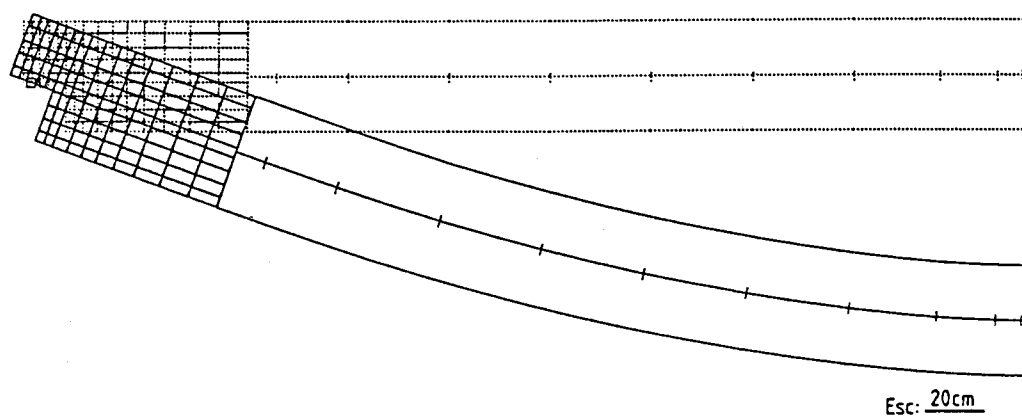
Fig. 6.19 - Deformada da viga pré-esforçada (continuação).
