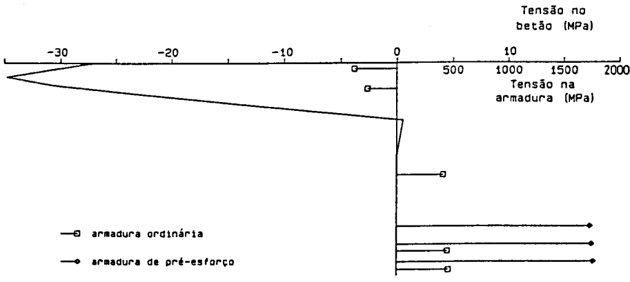
g) Acções majoradas de \gamma = 2,30 .
