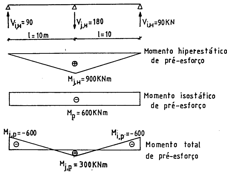
Fig. 2.15 - Viga hiperestática. Diagramas de momentos flectores devidos ao pré-esforço.
