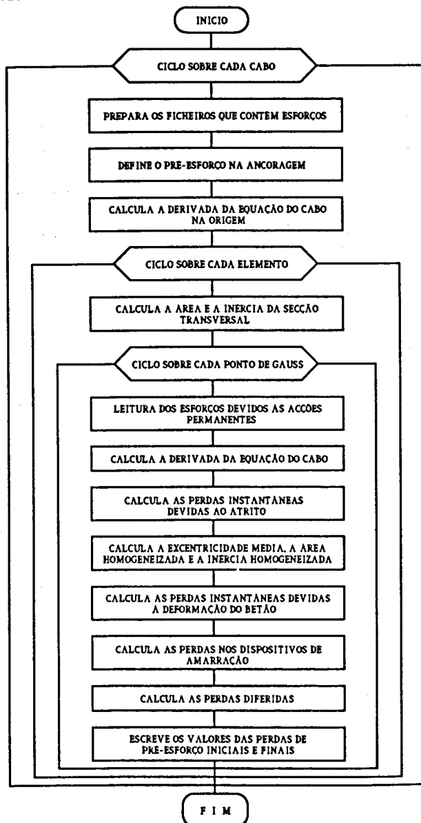
Fig. 3.8 - Subrotina de cálculo de perdas de pré-esforço.
