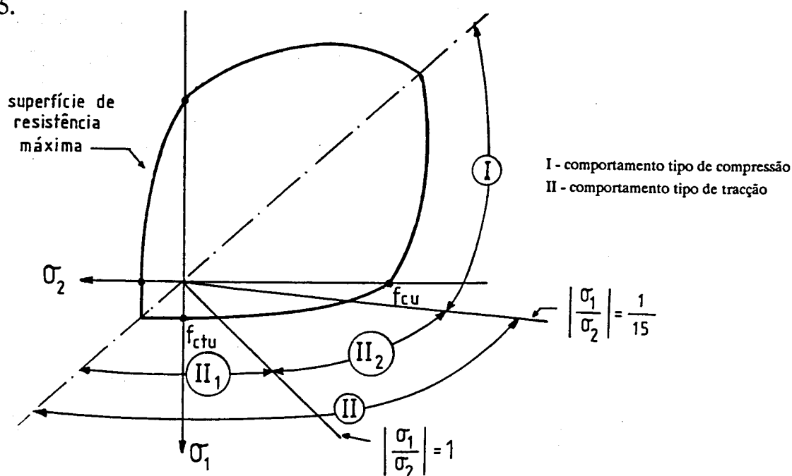
Fig. 4.24 - Regiões de comportamento do betão numa representação em estados de tensão biaxiais.
