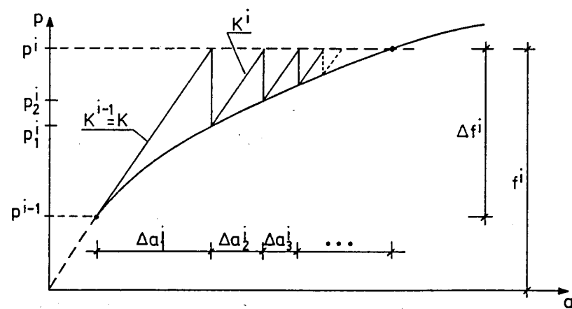
Fig. 5.3 - Método de Newton-Raphson modificado na primeira iteração.
