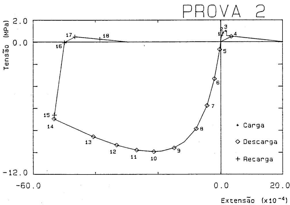
Fig. 5.9 - Diagrama tensão-extensão no betão na direcção normal ao plano da fenda. Sequência do teste: plastificação/abertura/fecho/plastificação/abertura.
