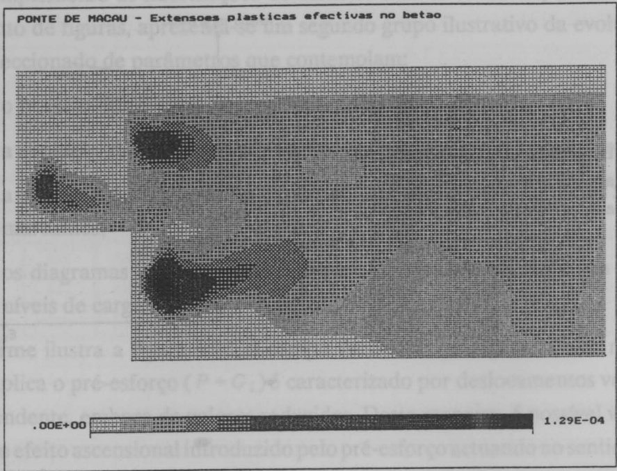
Fig.6.14 - Distribuição das extensões plásticas equivalentes no betão. Aplicação do pré-esforço.
