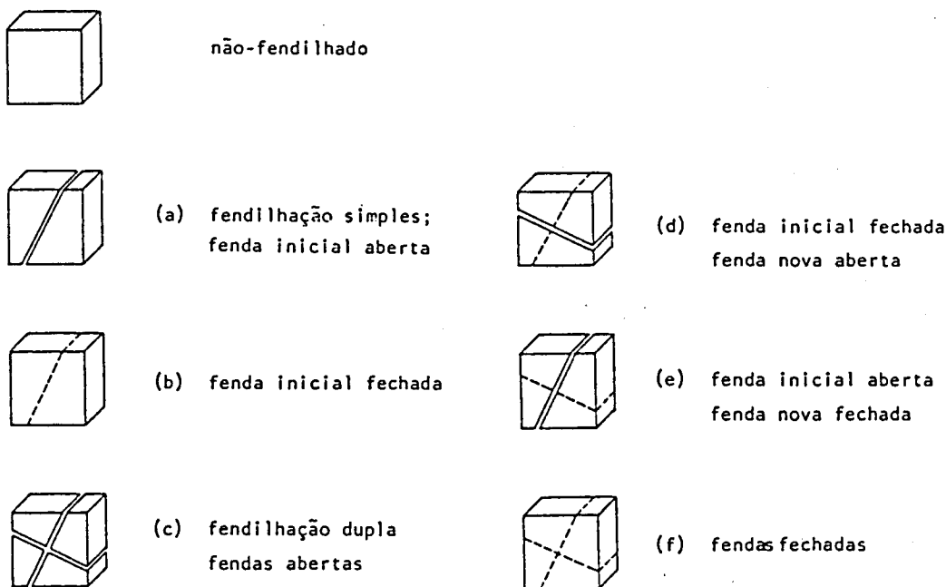
Fig. 4.21 - Configurações admitidas para a fendilhação.
