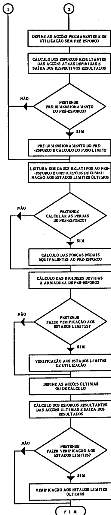
Fig. 3.1 - Segmento principal do programa de cálculo automático (continuação).
