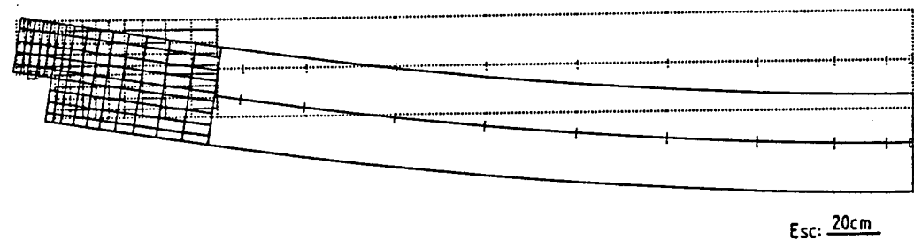
Fig. 6.19 - Deformada da viga pré-esforçada.
