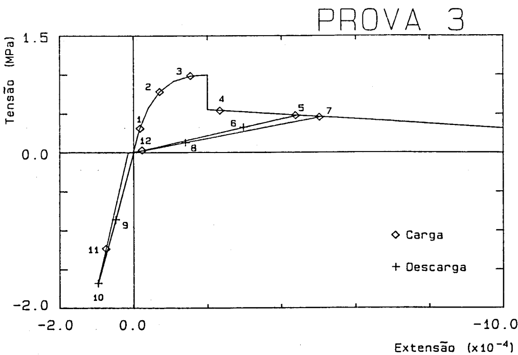
Fig. 5.10 - Diagrama tensão-extensão no betão na direcção normal ao plano da fenda. Sequência do teste: plastificação/abertura/fecho/plastificação/abertura.
