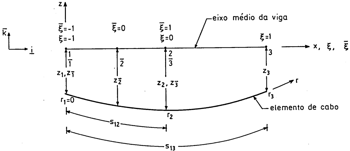
Fig. 2.10 - Definição das coordenadas curvilíneas do elemento de cabo.
