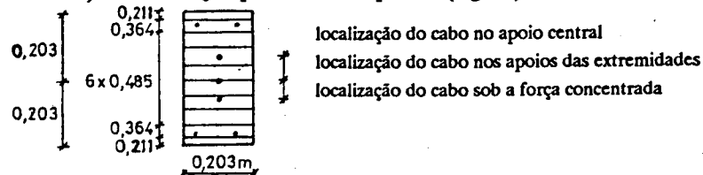
d) padrão de camadas para os elementos de viga.
