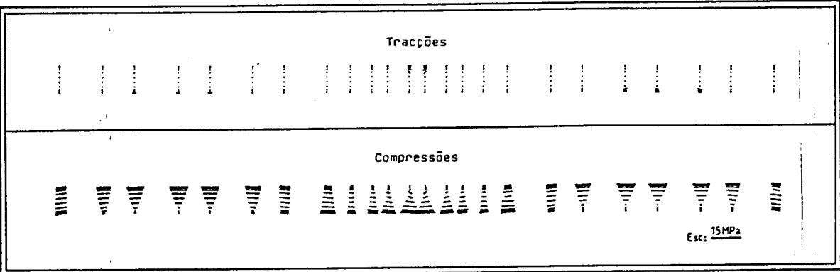
Fig. 6.4 - Distribuição das tensões principais no betão para vários níveis de carregamento (continuação).
