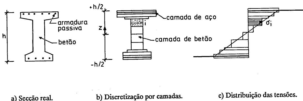
Fig. 2.5 - Secção discretizada por camadas.
