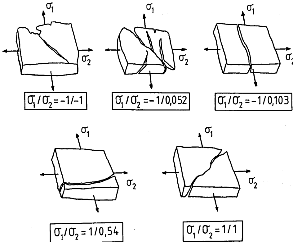
Fig. 4.23 - Modos de rotura em provetes sujeitos a tensões biaxiais.
