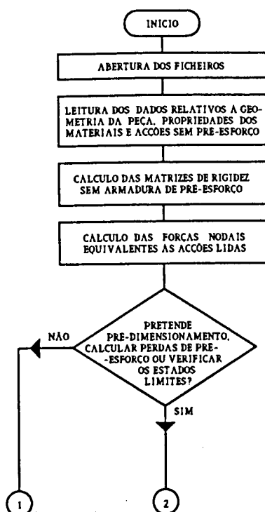
Fig. 3.1 - Segmento principal do programa de cálculo automático.
