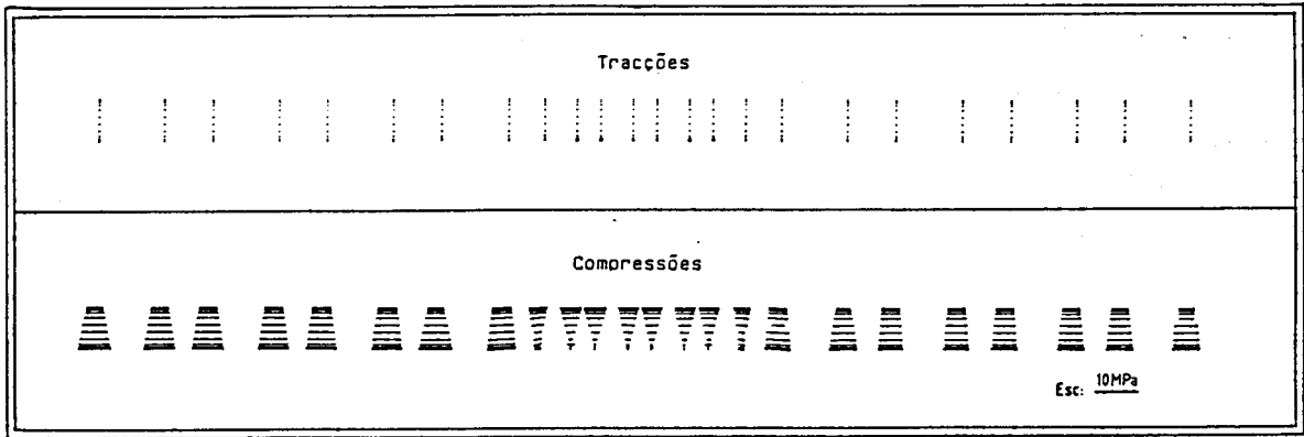
b) Tensões principais no instante de aplicação do pré-esforço ( G_1 + P ).
