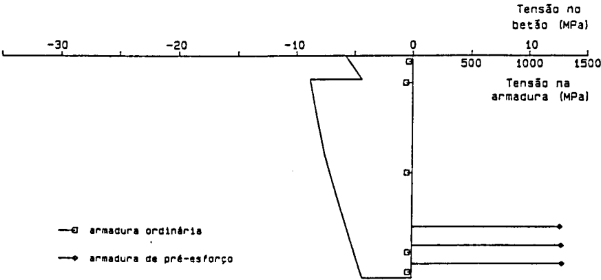
Fig. 6.27 - Diagramas de tensões na secção a meio vão.
