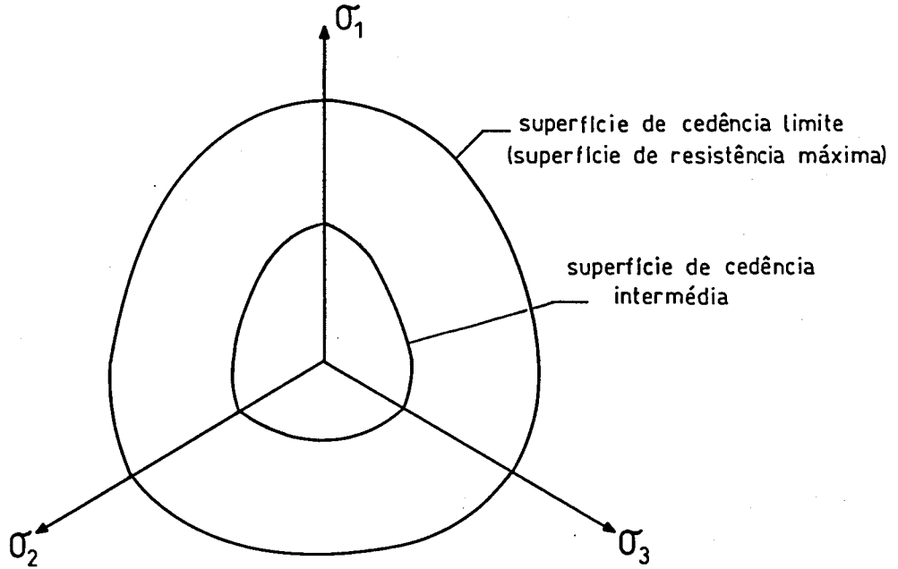
Fig. 4.7 - Representação das superfícies de cedência nos planos de desvio.
