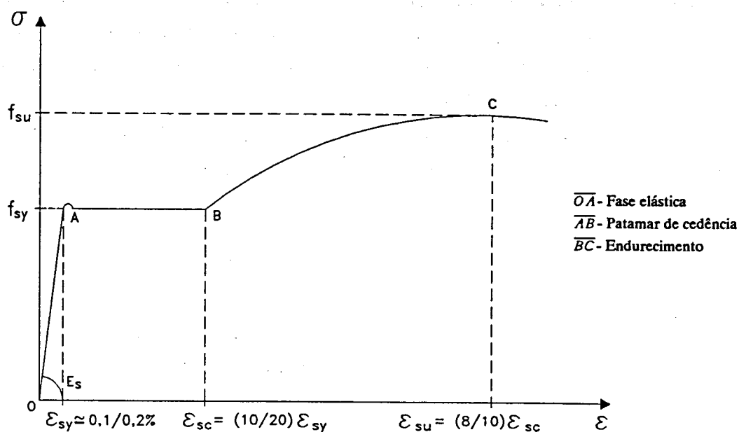
Fig. 4.25 - Diagrama tensão-deformação uniaxial do aço macio.
