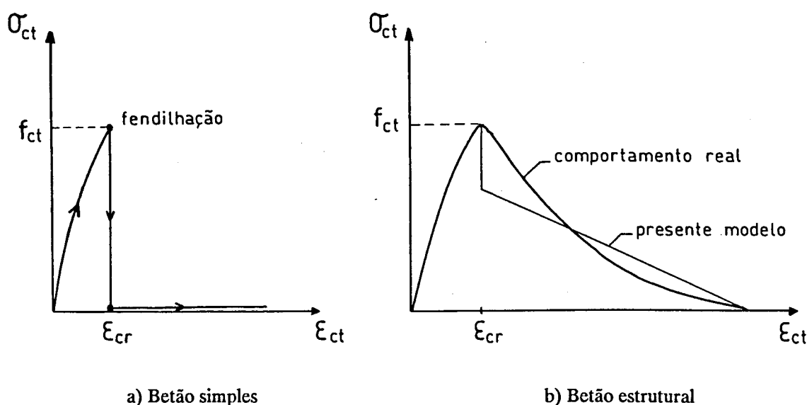
Fig. 4.10 - Resposta do betão à tracção.
