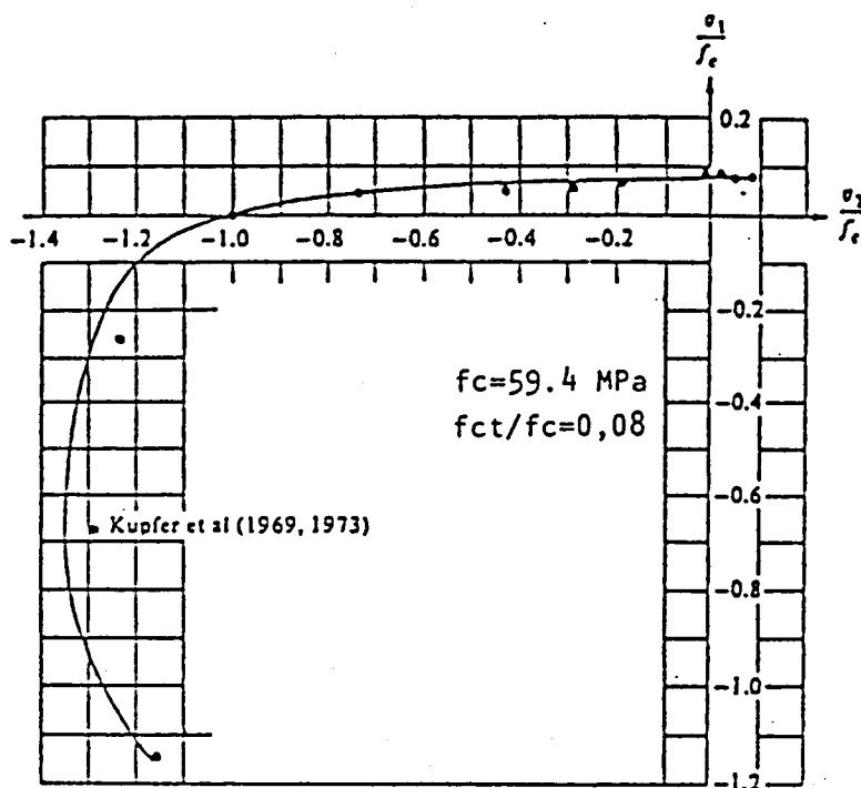
Fig. 4.6 - Comparação do critério de Ottosen com os testes biaxiais de Kupfer (1969, 1973).
