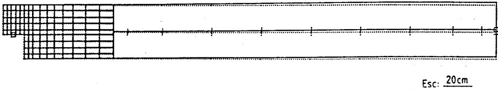
Fig. 6.12 - Deformada da viga pré-esforçada. Aplicação do pré-esforço.
