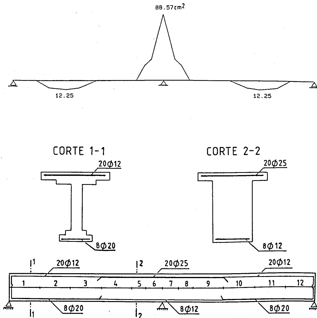
Fig. 3.16 - Dimensionamento da armadura passiva de flexão.
