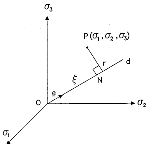
Fig. 4.1 - Espaço de tensões de Haig-Westergaard.
