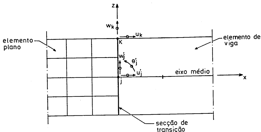
Fig. 2.21 - Associação dos graus de liberdade.
