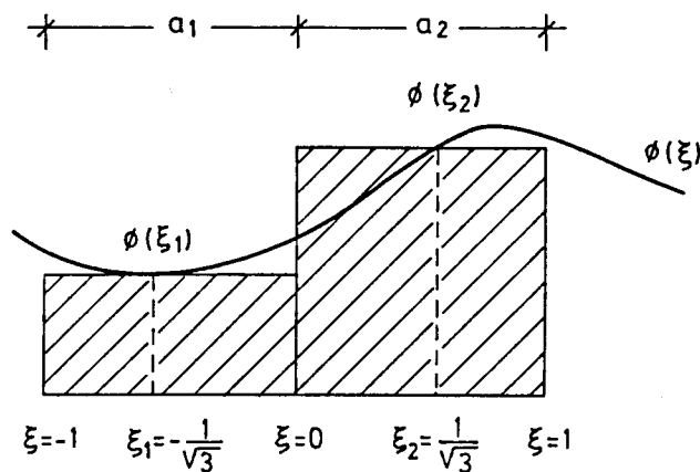
Fig. 2.8 - Integração com dois pontos de Gauss.
