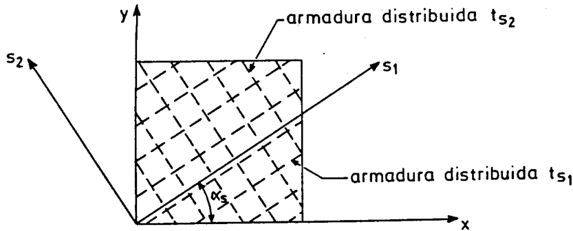
Fig. 2.18 - Representação contínua da armadura passiva.
