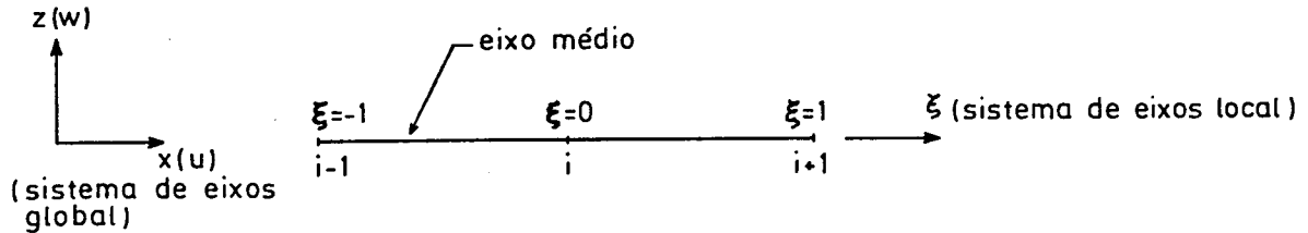
Fig. 2.2 - Elemento de viga parabólico isoparamétrico.
