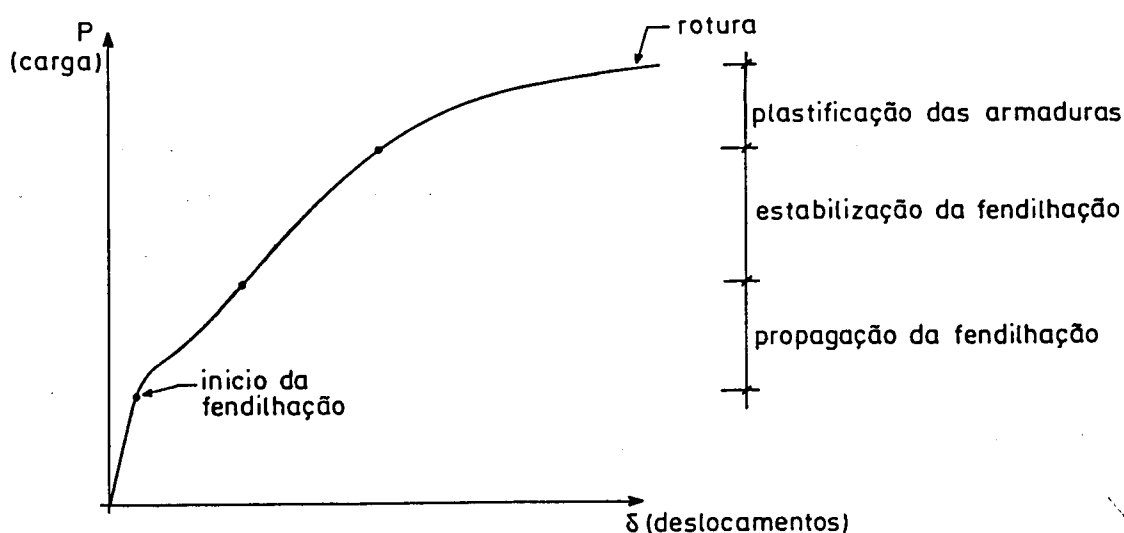
Fig. 6.1 - Traçado esquemático da resposta de uma estrutura de betão sujeita a um carregamento monotónico crescente.
