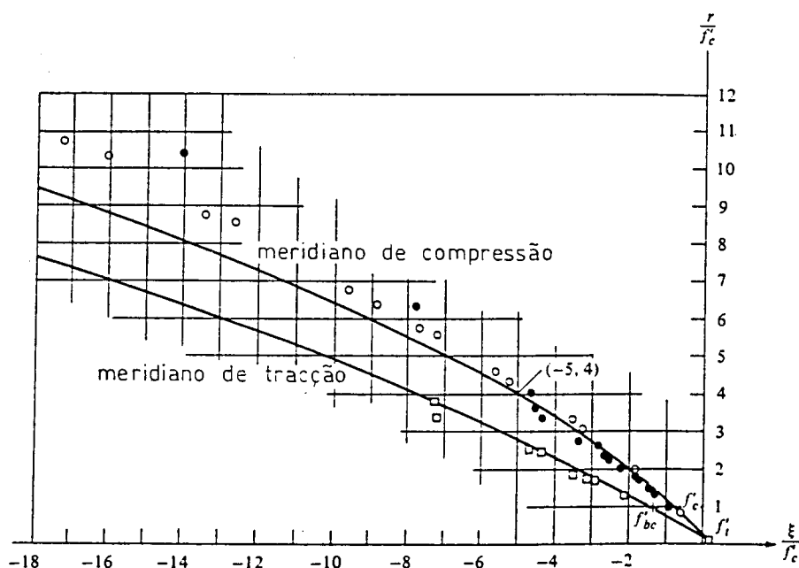
Fig. 4.5 - Comparação do critério de Ottosen com resultados experimentais nos planos meridianos: círculos abertos, Balmer (compressão); círculos a cheio, Richard (compressão); quadrados, Richard (tracção); cruzeiros, Kupfer (tracção).
