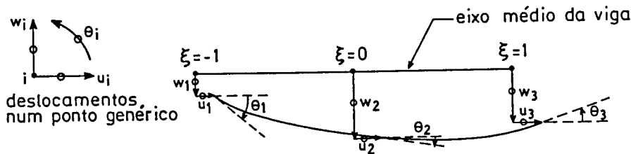
Fig. 2.4 - Deslocamentos num elemento de três nós.
