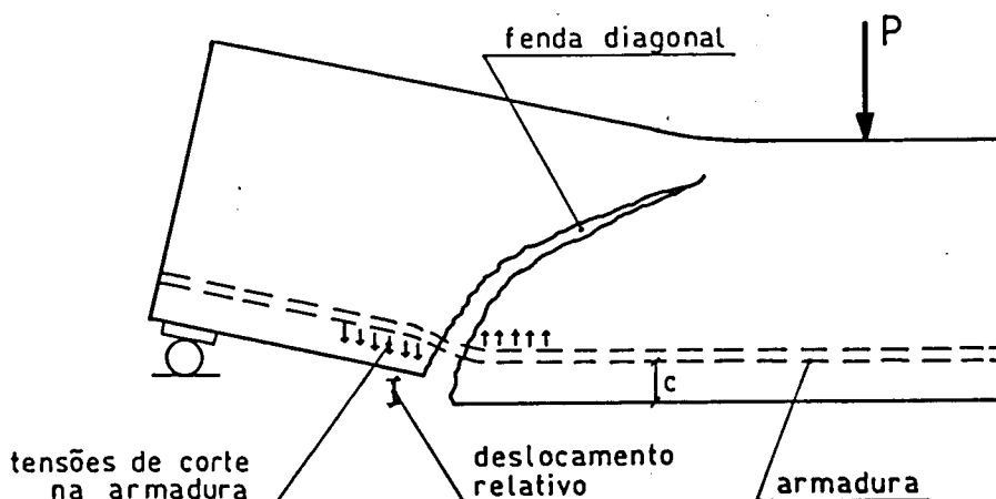
Fig. 4.15 - Contribuição da armadura na transmissão da força de corte através da fenda.
