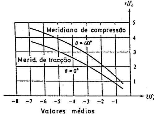
Fig. 4.4 - Forma característica dos meridianos de tração e de compressão.
