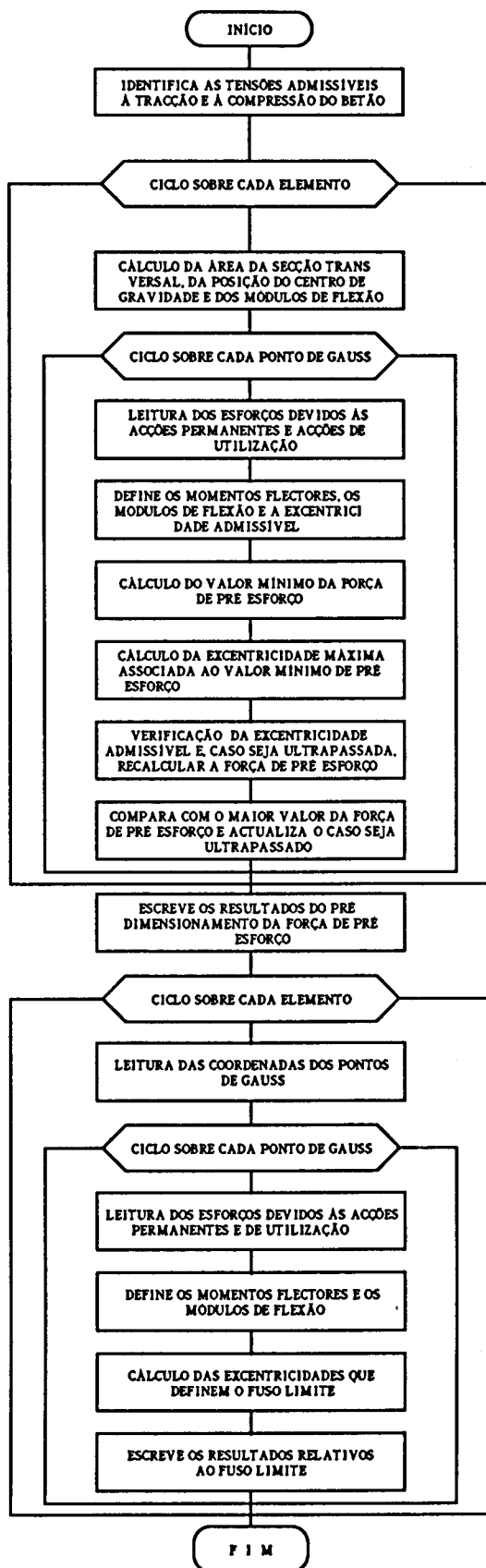
Fig. 3.5 - Subrotina de pré-dimensionamento do pré-esforço.
