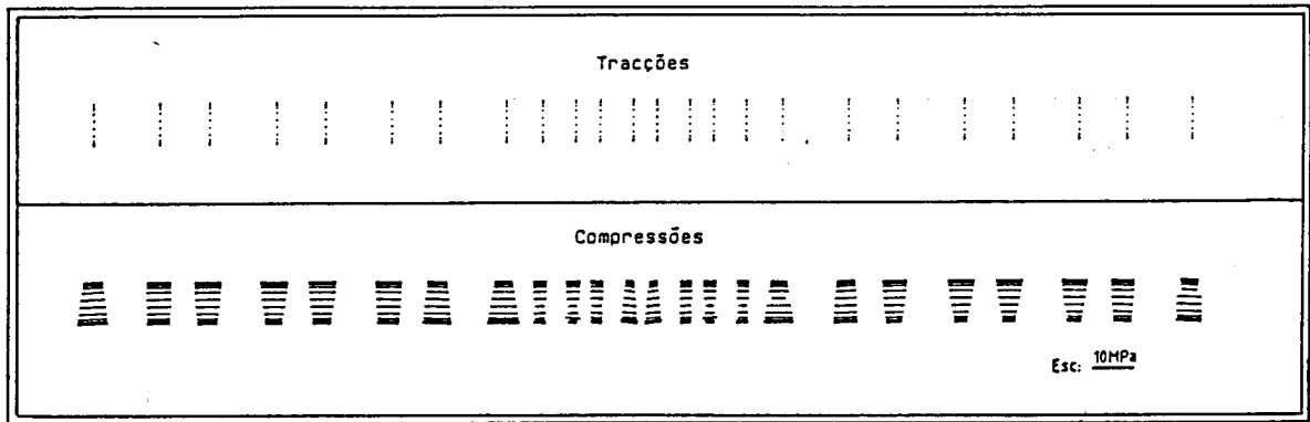
c) Tensões principais para as ações permanentes totais com pré-esforço ( G + P ).
