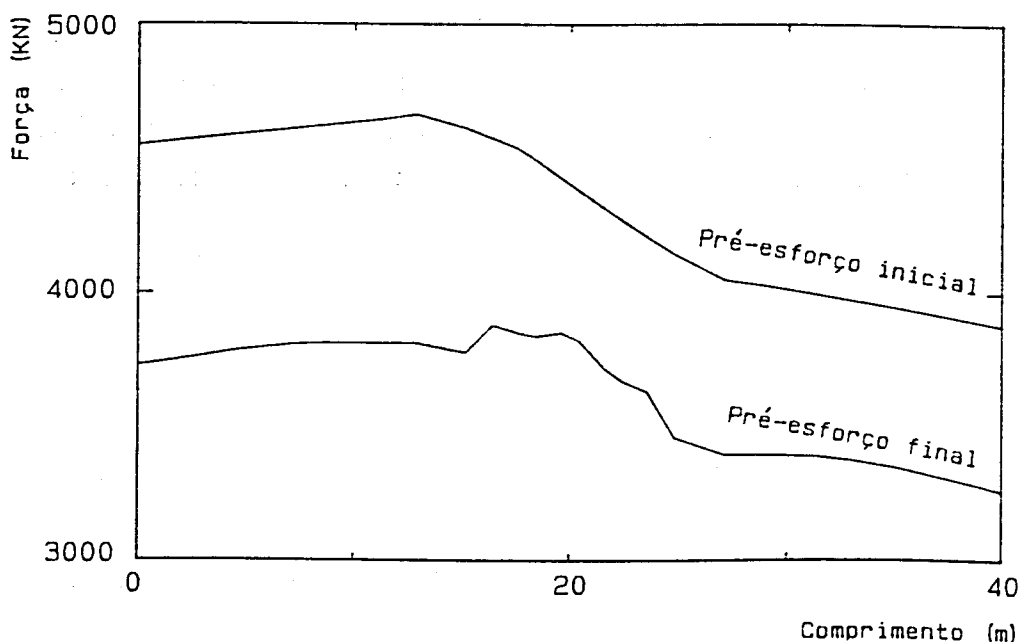
Fig. 3.14 - Variação do pré-esforço ao longo das armaduras.
