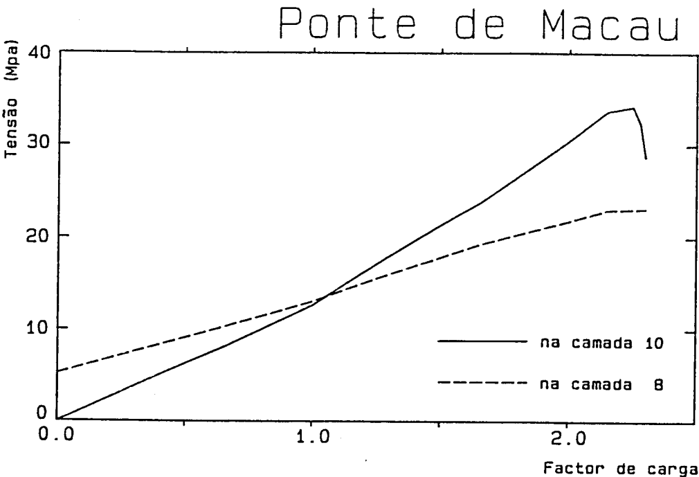
Fig. 6.25 - Curvas carga-tensões normal nas camadas a meio vão.
