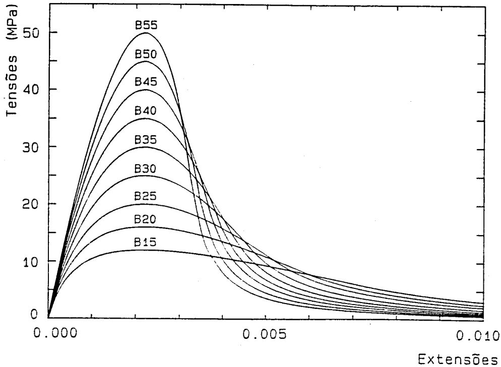
Fig. 4.9 - Relações constitutivas, para várias classes de betão, definidas pelo presente modelo.
