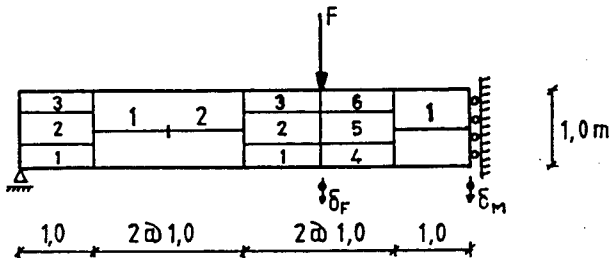
c) Malha de elementos finitos para a análise C.
