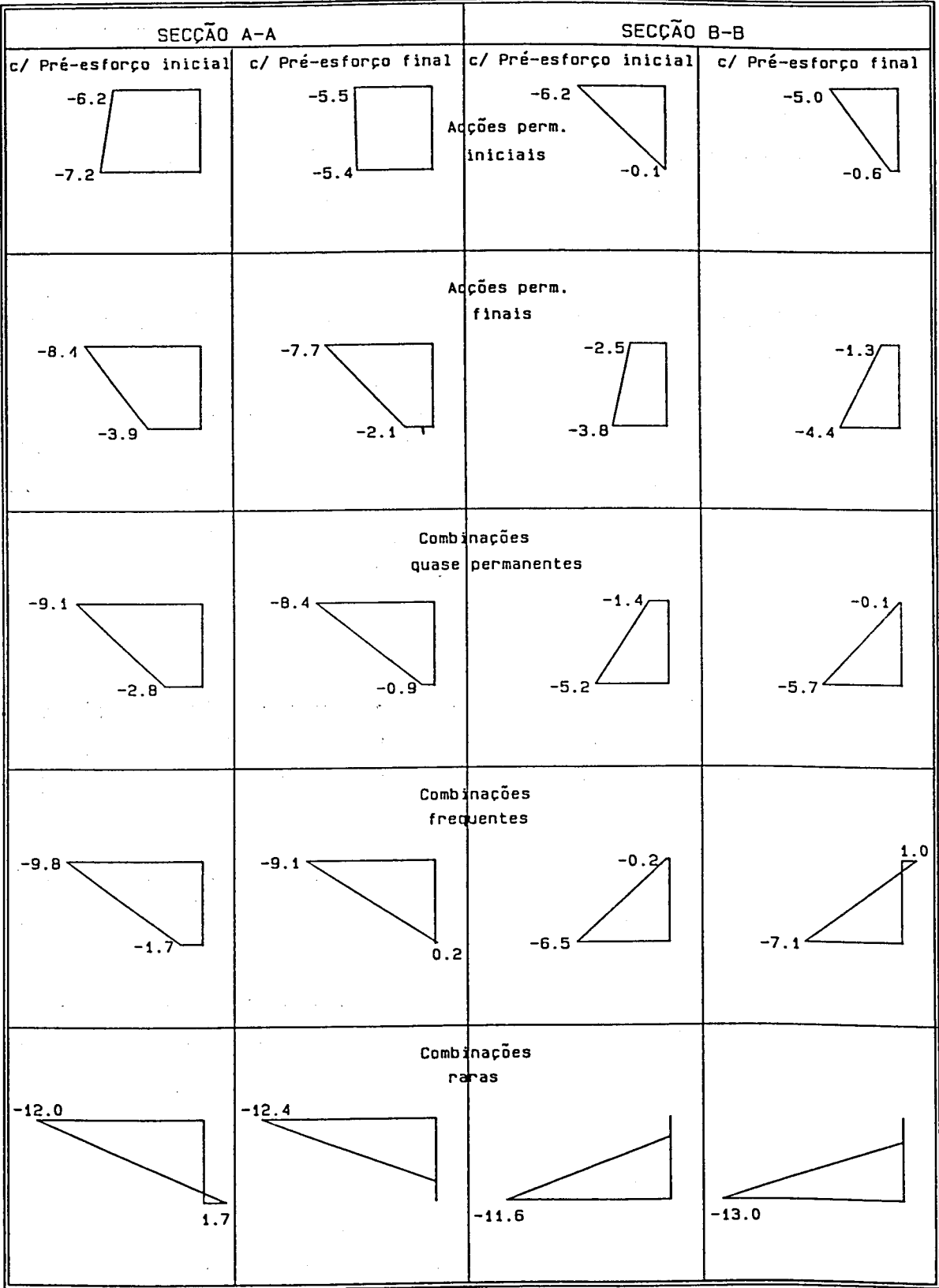
Fig. 3.17 - Diagramas de tensões para várias combinações de acções.
