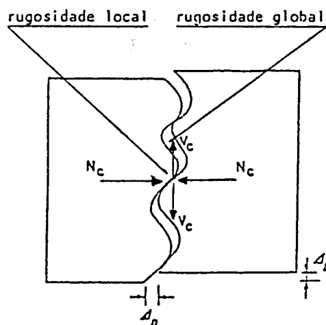
Fig. 4.16 - Transferência de esforços de corte por engrenagem entre as faces da fenda.
