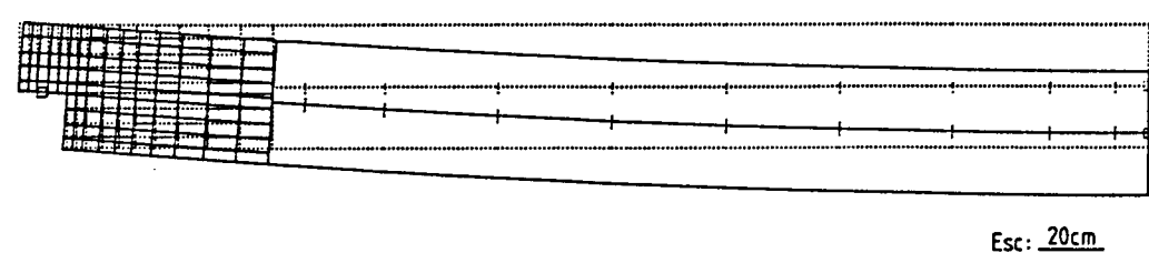
Fig. 6.18 - Configuração da fendilhação.
