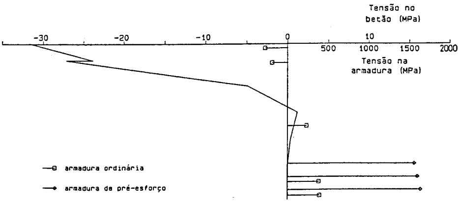
f) Acções majoradas de \gamma = 2,00 .
