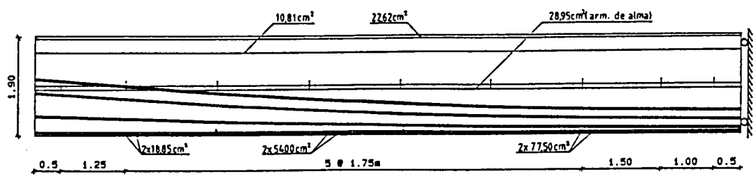
d) Disposição das armaduras nos elementos de viga.
