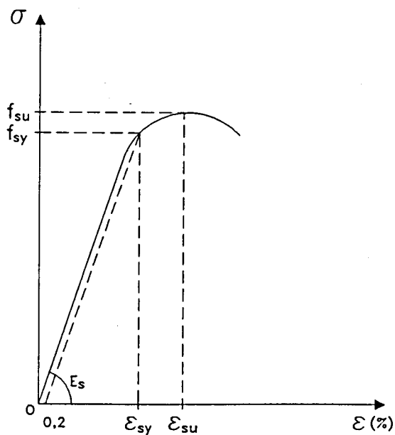
Fig. 4.26 - Diagrama tensão deformação uniaxial do aço duro.
