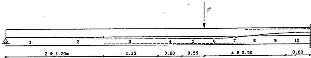
b) Discretização por elementos de viga (viga B).
