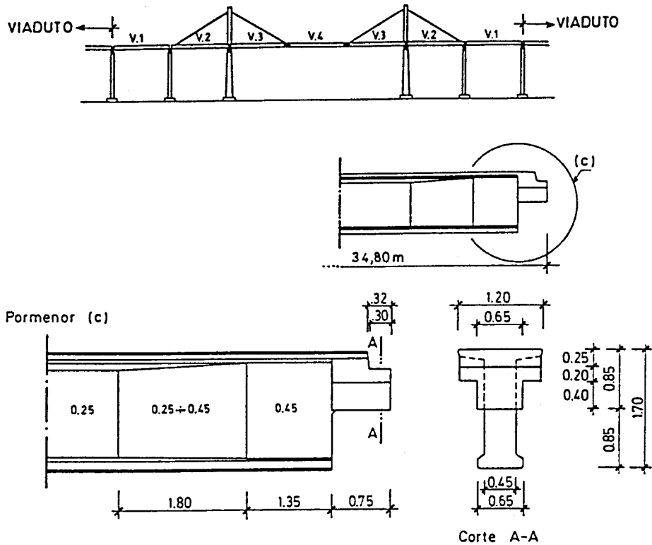
Fig. 6.8 - Geometria da viga pré-esforçada (viga V.4).
