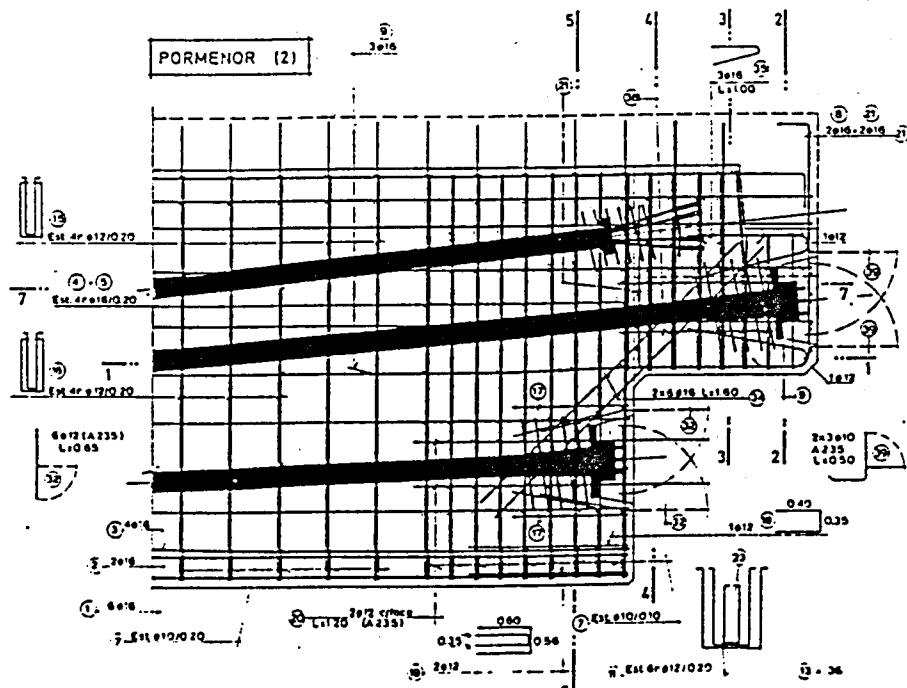
Fig. 6.9 - Pormenor da distribuição da armadura (desenho do projecto).
