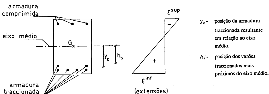
Fig. A.1 - Posicionamento da armadura traccionada.
