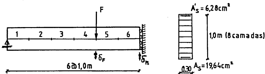
a) Malha de elementos finitos para a análise A.
