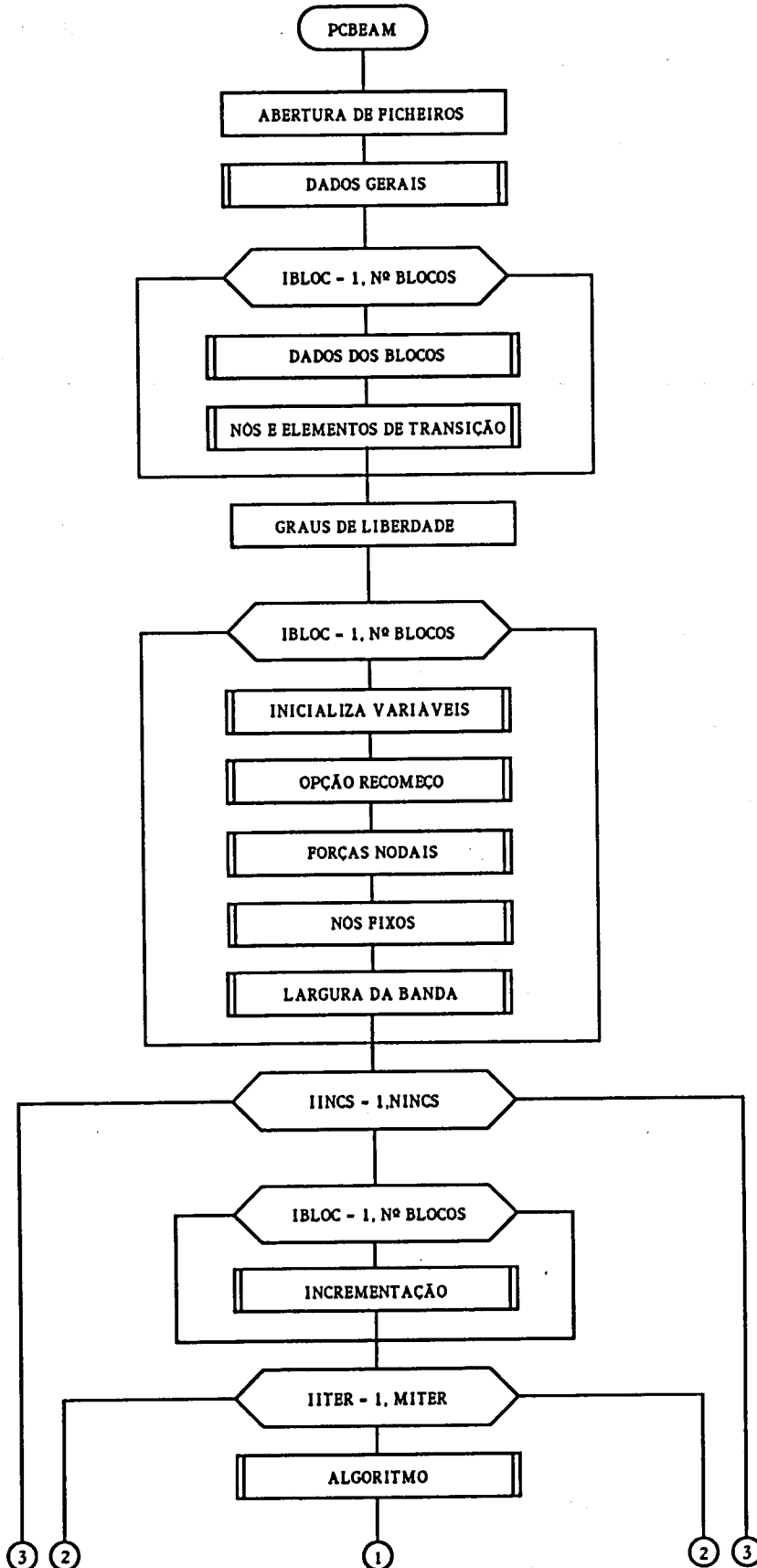
Fig. 5.1 - Fluxograma do programa PCBEAM.
