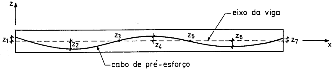
Fig. 2.9 - Definição da geometria do cabo com base em 7 pontos.
