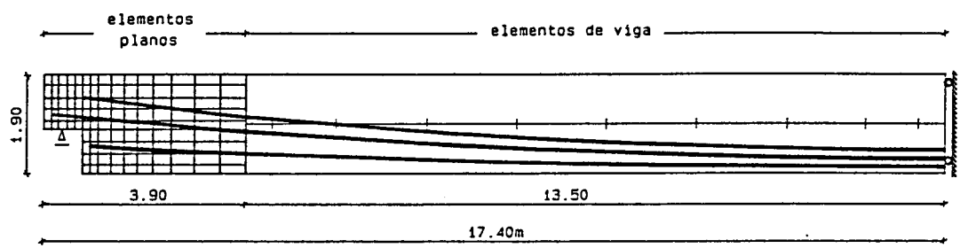
a) Malha de elementos finitos.
