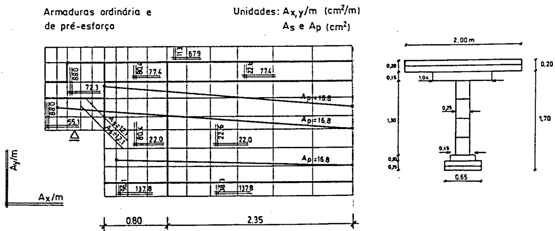
c) Disposição das armaduras nos elementos planos e padrão de camadas para os elementos de viga.
