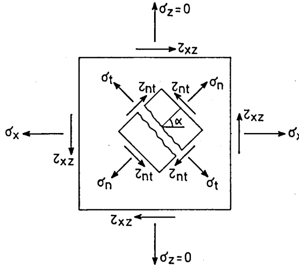
Fig. 4.17 - Direcção de fendilhação.
