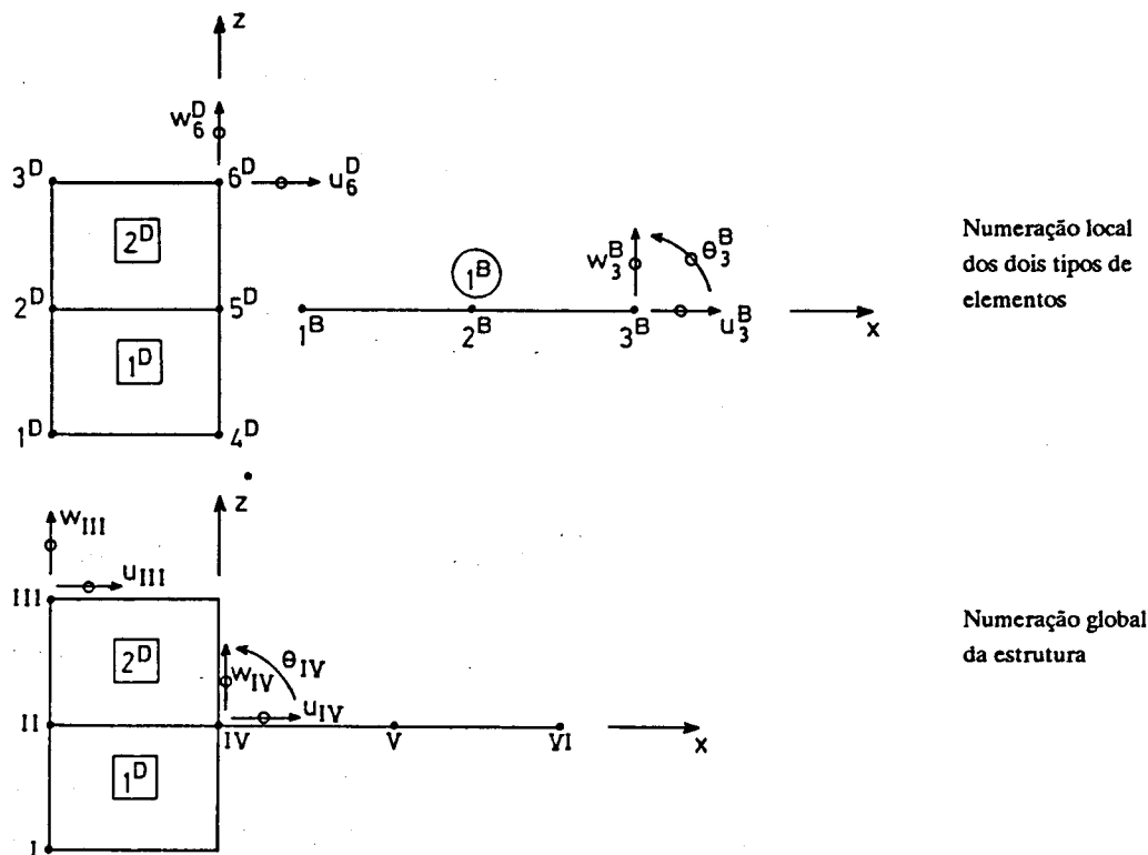
Fig 5.6 - Associação de dois elementos planos de 4 nós com um elemento de viga de 3 nós.
