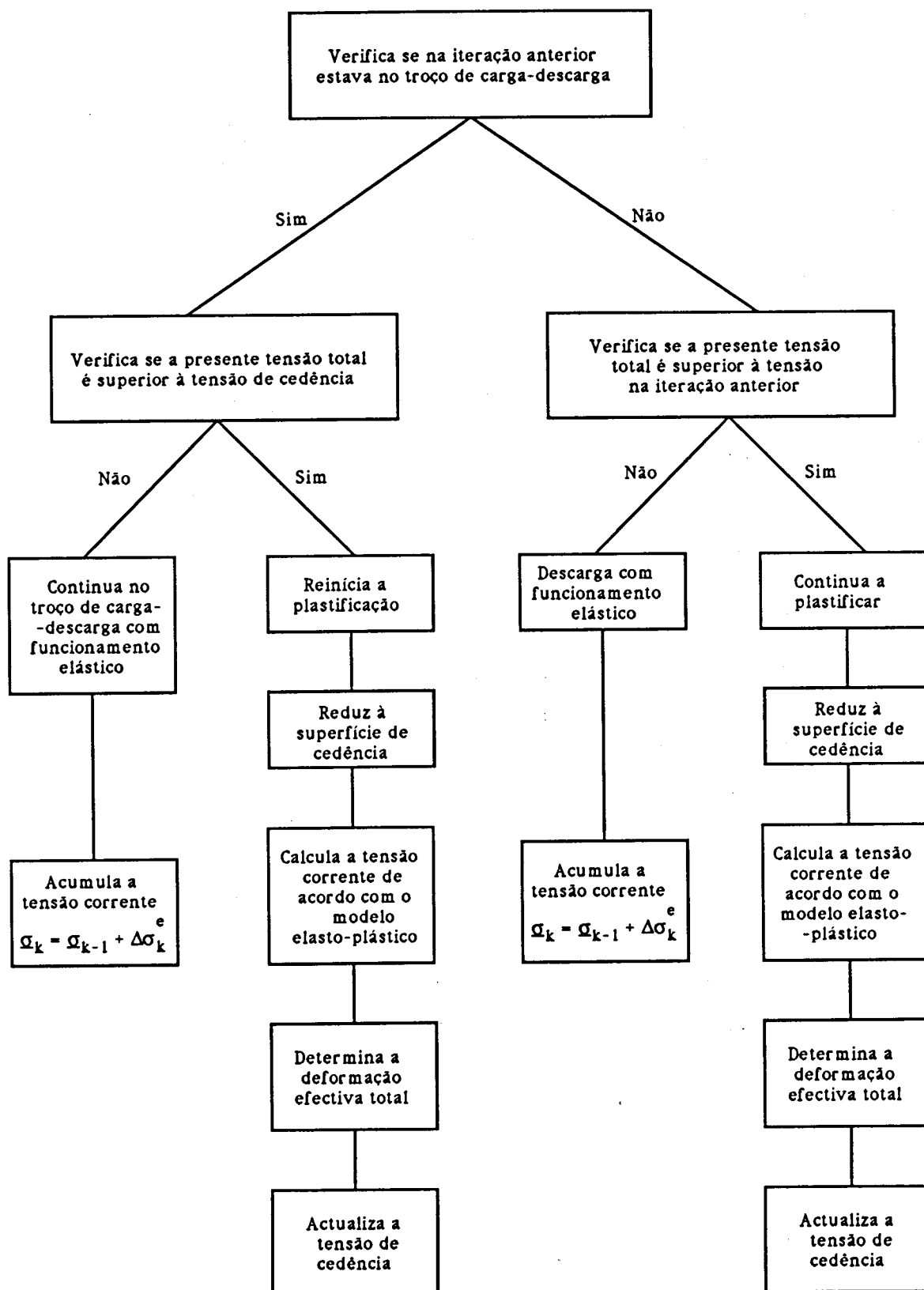
Fig. 5.5 - Determinação das tensões de acordo com as relações constitutivas dos materiais.
