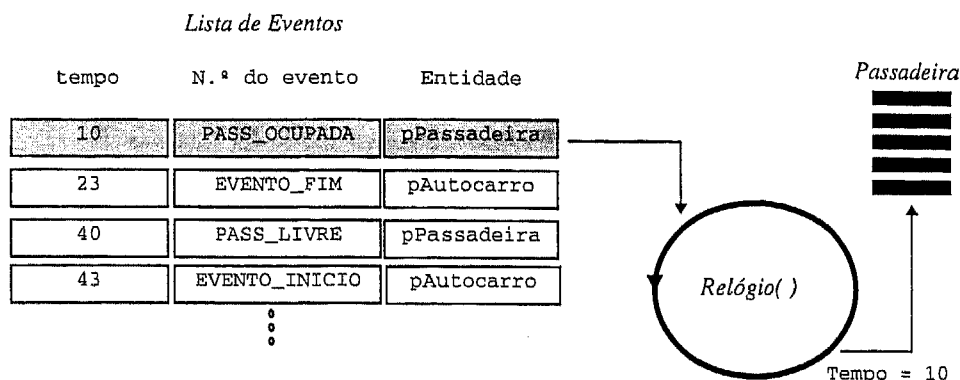
Fig. 2.5 Processo de execução de eventos na simulação.
