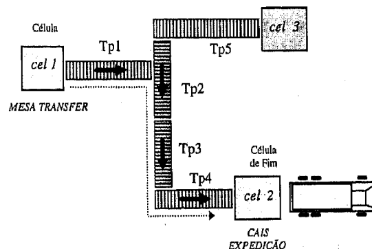
Fig. 7.11 Exemplo de um processo de transferência de material usando tapetes.
