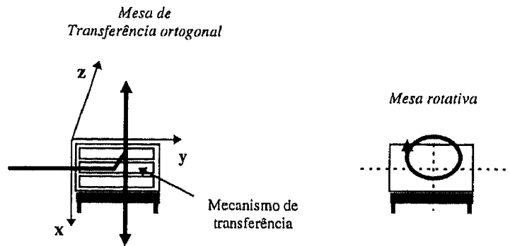
Fig. 3.10 Circulação do material. Mesa de transferência ortogonal e Mesa rotativa
