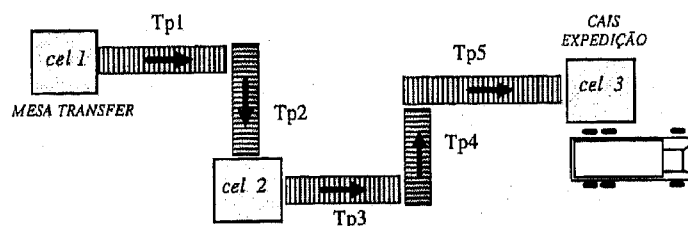
Fig. 7.12 Transferência de material entre várias células usando tapetes.
