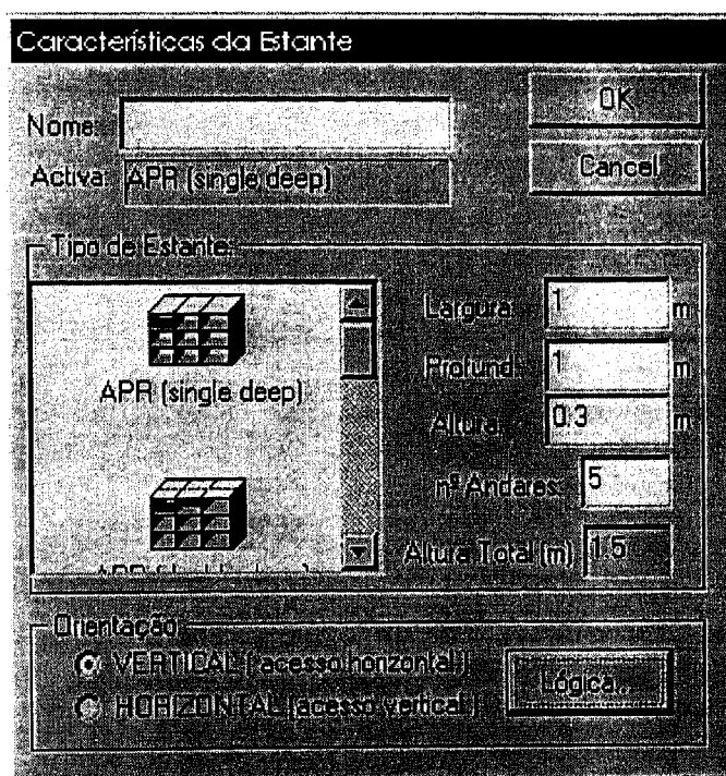
Fig. 8.3 Diálogo para caracterização da estante.
