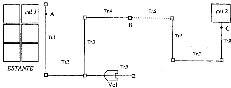
Fig. 7.9 Exemplo de uma tarefa de um Veículo.
