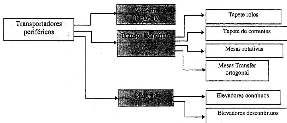
Fig. 3.7 Transportadores periféricos.
