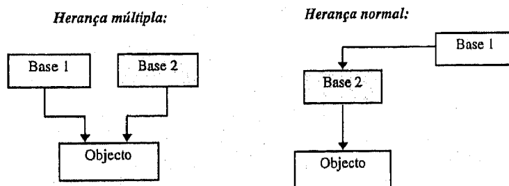
Fig. 7.3 Métodos de herança permitidos em C++.
