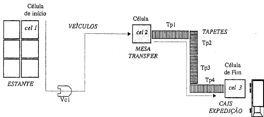
Fig.6.30 Exemplo de um percurso geral englobando veículos e tapetes.
