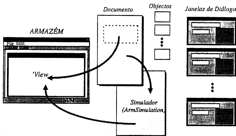
Fig. 5.1 Estrutura da aplicação ARMAZÉM em Visual C++.
