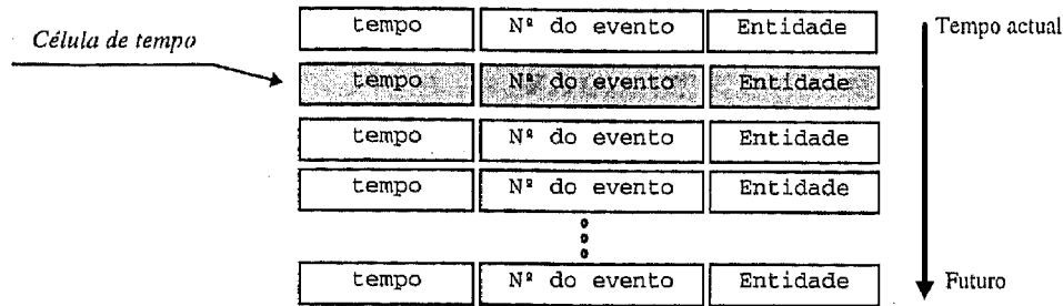
Fig. 7.1 Lista de eventos como um conjunto de células de tempo .
