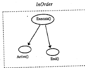
Fig. 7.14 Estrutura da entidade de simulação InOrder .
