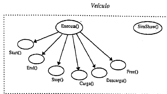
Fig. 7.8 Estrutura da entidade de simulação Veículo .
