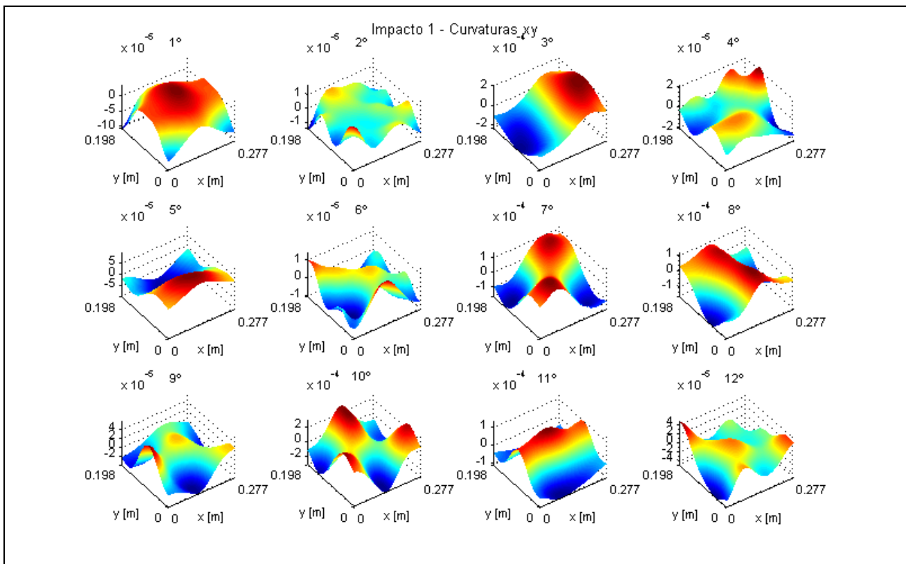
Fig. F.20 – Representação dos campos de curvaturas em xy, correspondentes aos modos naturais da placa após o impacto 1.
