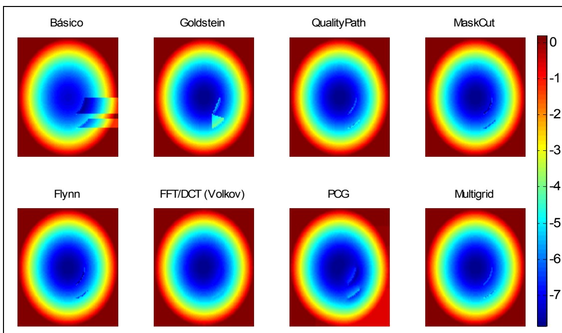
Fig. B.6 – Mapas contínuos de fase obtidos por diferentes métodos de unwrapping da fase aplicados ao mapa de fase com descontinuidades na transição da fase (Capítulo 4).
