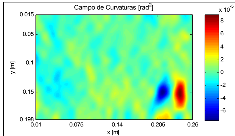
Fig. 5.35 – Campo de curvaturas segundo o eixo x para a placa laminada compósita submetida a uma variação de pressão de -500Pa.
