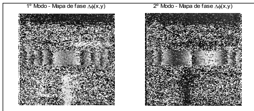
Fig. 5.14 – Os mapas de fase relativos aos dois primeiros modos naturais da viga livre-livre.
