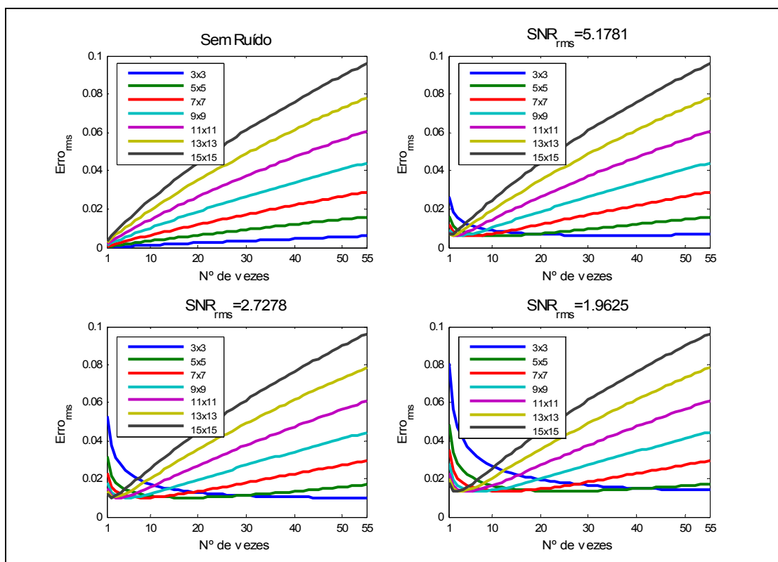
Fig. B.8 – Comportamento do filtro de Média em campos de medida com diferentes níveis de ruído.
