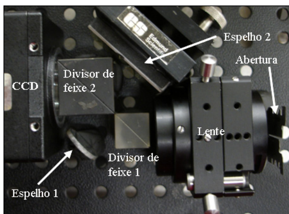
Fig. D.1 – Montagem do interferómetro óptico.
