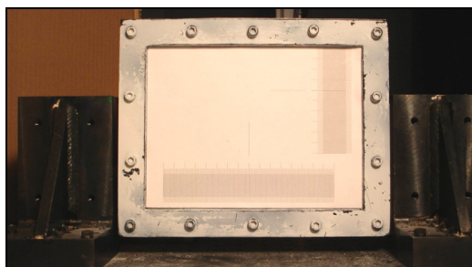
Fig. 3.35 – Ensaio da placa encastrada, submetida a uma pressão transversal uniforme de 180 \text{ N/m}^2 .
