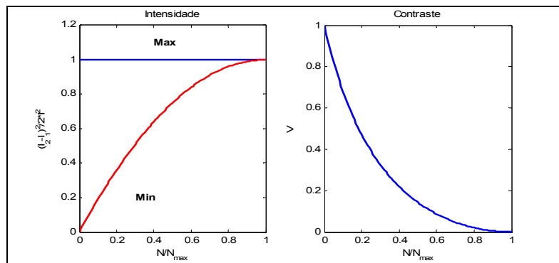
Fig. 3.21 - Intensidade e contraste das franjas para decorrelação de duas frentes de onda por rotação ( x=1 ).
