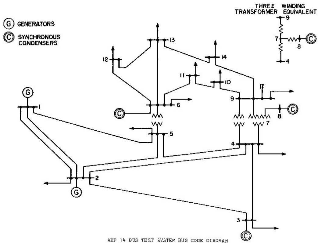
Figure A.1 - IEEE’s 14-bus test system.
