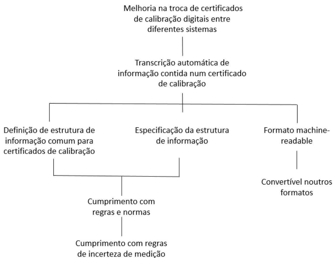
Figura 5 - Diagrama AND/OR
