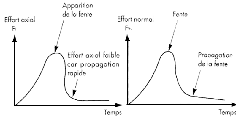
Figure II.20 -Diagramme effort de coupe/temps (d'après Koch, 1964)
