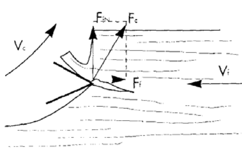
Figure II.29 -3ème phase - fendage (d'après Koch, 1964)
