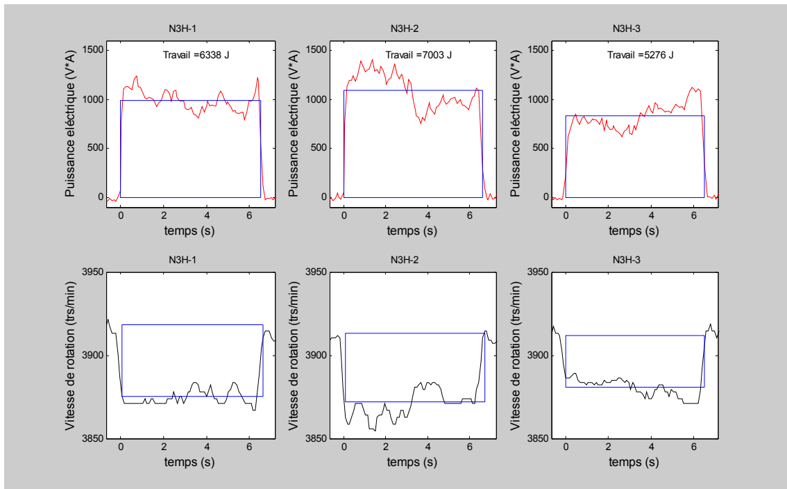
Figure IV.20 - Reproductibilité du système pour le niveau d'usinage 3, pour les trois planches de hêtre
