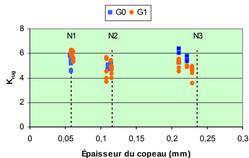
Figure IV.65 - Influence du ponçage dans le Krug (critère de rugosité)
