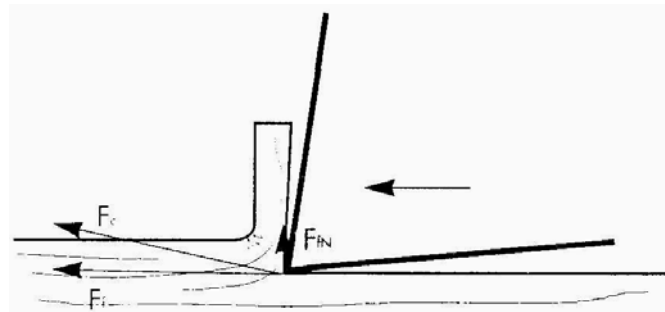
Figure II.21 -Copeau obtenu par compression (d'après Koch, 1964)
