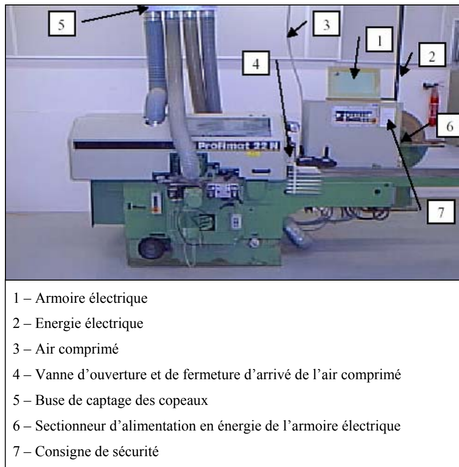
Figure II.32 -Vue d'ensemble de la corroyeuse
