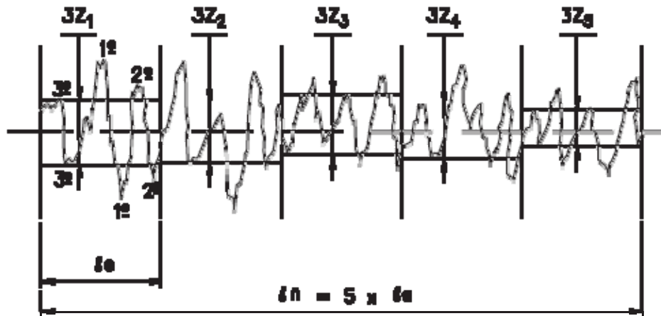
Figure II.41 -Rugosité moyenne du troisième sommet et creux (R3Z)
