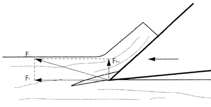
Figure II.19 -Copeau obtenu par fendage (d'après Koch, 1964)
