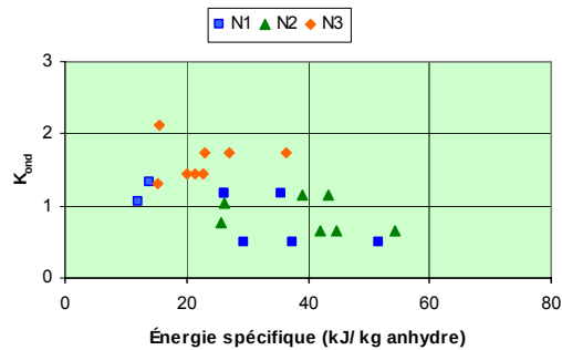
Figure IV.83 - Influence du niveau d'usinage dans le Kond (critère d'ondulation)
