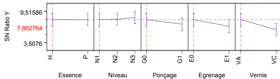
Figure IV.72 - Influence des différents facteurs dans le critère Ksub (indice signal-bruit)
