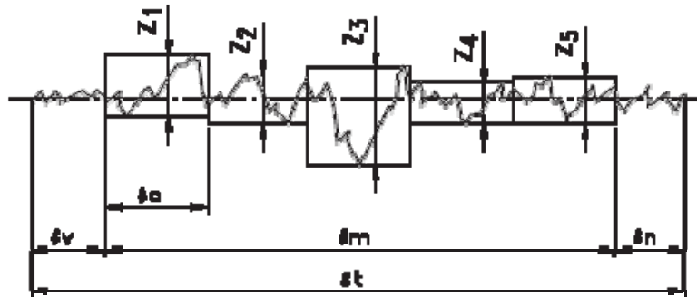
Figure II.40 -Rugosité partielle Zi pour définir Rz
