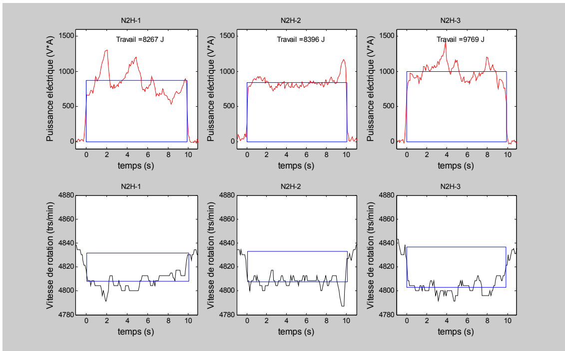
Figure IV.18 - Reproductibilité du système pour le niveau d'usinage 2, pour les trois planches de hêtre
