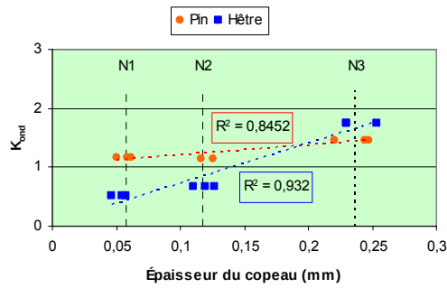
Figure IV.75 - Influence du niveau d'usinage dans le Kond (critère d'ondulation)
