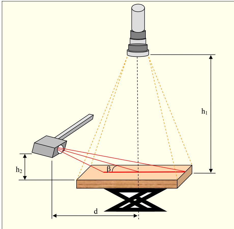
Figure III.13 - Schéma du système de vision laser
