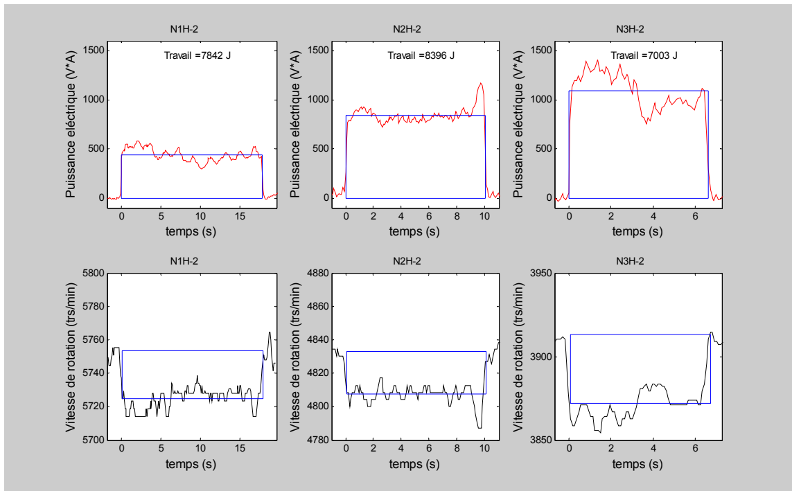
Figure IV.22 - Monitorisation d'usinage – Hêtre
