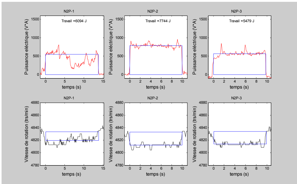
Figure IV.17 - Reproductibilité du système pour le niveau d'usinage 2, pour les trois planches de pin
