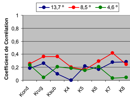
Figure IV.27 - Corrélation avec le grain de ponçage
