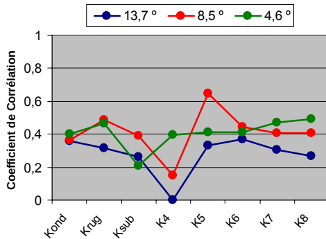
Figure IV.26 - Corrélation avec le niveau d'usinage
