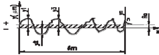
Figure II.36 -Rugosité moyenne (Ra)
