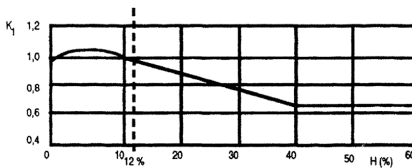
Figure A1.1 - Détermination du coefficient d'humidité K_h :
