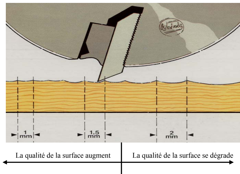
Figure III.9 - Rapport entre l'avance par dent et la qualité de la surface usinée du bois (Adapté du manuel de l'équipement industriel réf. WEINIG)
