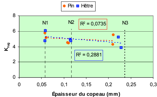
Figure IV.60 - Influence du niveau d'usinage dans le Krug (critère de rugosité)
