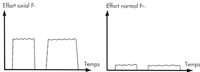
Figure II.24 -Diagramme effort de coupe/temps (d'après Koch, 1964)
