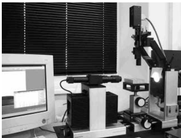
Figure III.15 - Goniomètre
