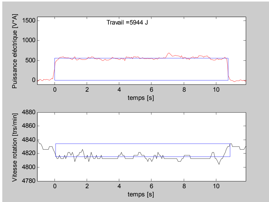
Figure III.8 - Puissance électrique totale absorbée et vitesse de rotation instantanée
