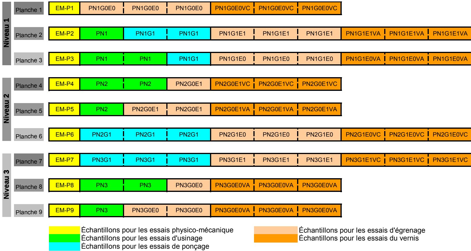
Figure IV.13 - Plan de coupe des éprouvettes de pin
