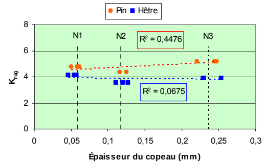
Figure IV.76 - Influence du niveau d'usinage dans le Krug (critère de rugosité)
