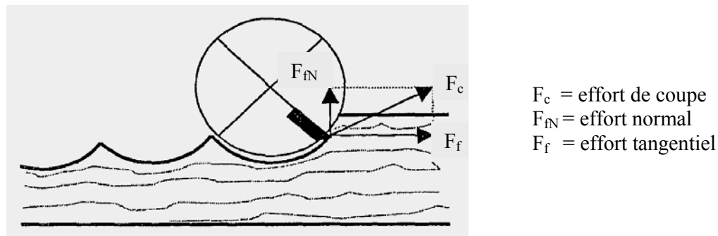
Figure II.11 -Décomposition de l'effort de coupe (Koch, 1964)
