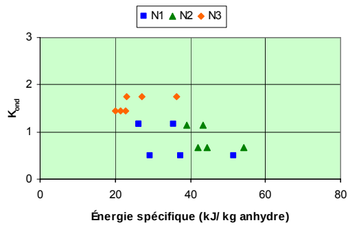
Figure IV.78 - Influence du niveau d'usinage dans le Kond (critère d'ondulation)
