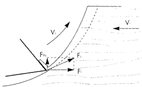
Figure II.28 -2ème phase - compression (d'après Koch, 1964)
