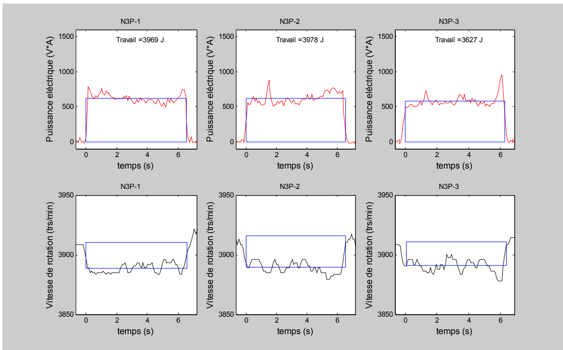
Figure IV.19 - Reproductibilité du système pour le niveau d'usinage 3, pour les trois planches de pin
