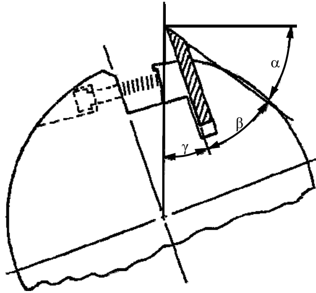
Figure II.16 -Les angles de l'outil de coupe
