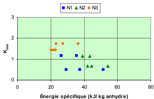
Figure IV.31 - Influence du niveau d'usinage dans le Kond (critère d'ondulation)
