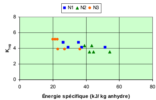
Figure IV.79 - Influence du niveau d'usinage dans le Krug (critère de rugosité)
