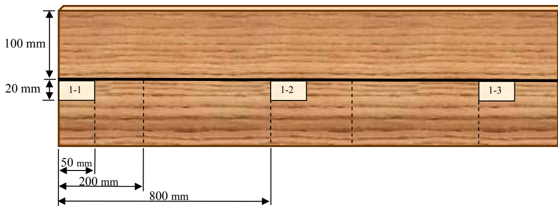
Figure III.3 - Débit des éprouvettes pour les essais physico-mécaniques
