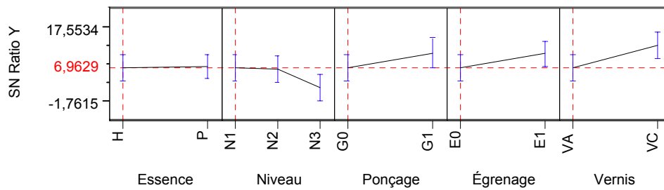
Figure IV.35 - Influence des différents facteurs dans le critère Kond (indice signal-bruit)
