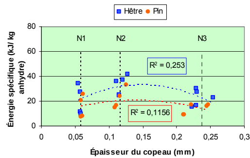
Figure IV.82 - Influence du niveau d'usinage dans l'énergie spécifique
