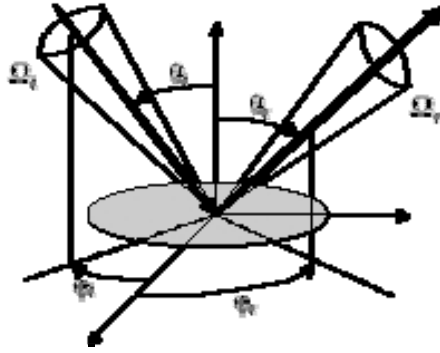
Figure II.56 -Goniospectrophotométrie - Notation des angles
