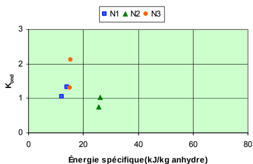
Figure IV.62 - Influence du niveau d'usinage dans le Kond (critère d'ondulation)
