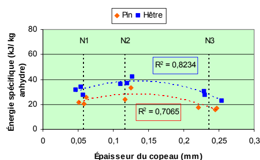
Figure IV.30 - Influence du niveau d'usinage dans l'énergie spécifique
