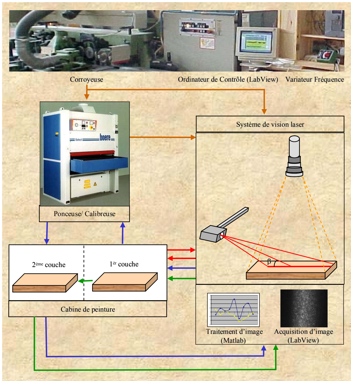
Figure III.1 - Séquences des protocoles expérimentaux
