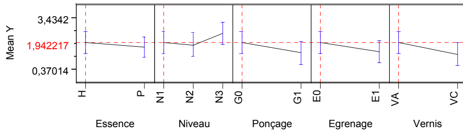
Figure IV.67 - Influence des différents facteurs dans le critère Kond (moyenne)
