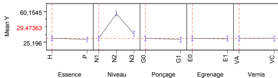
Figure IV.73 - Influence des différents facteurs dans l'énergie spécifique consommée (moyenne)
