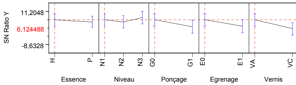
Figure IV.68 - Influence des différents facteurs dans le critère Kond (indice signal-bruit)
