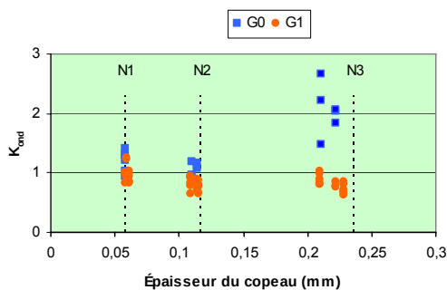
Figure IV.64 - Influence du ponçage dans le Kond (critère d'ondulation)
