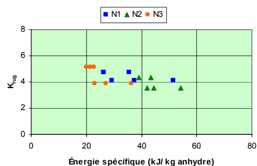
Figure IV.32 - Influence du niveau d'usinage dans le Krug (critère de rugosité)
