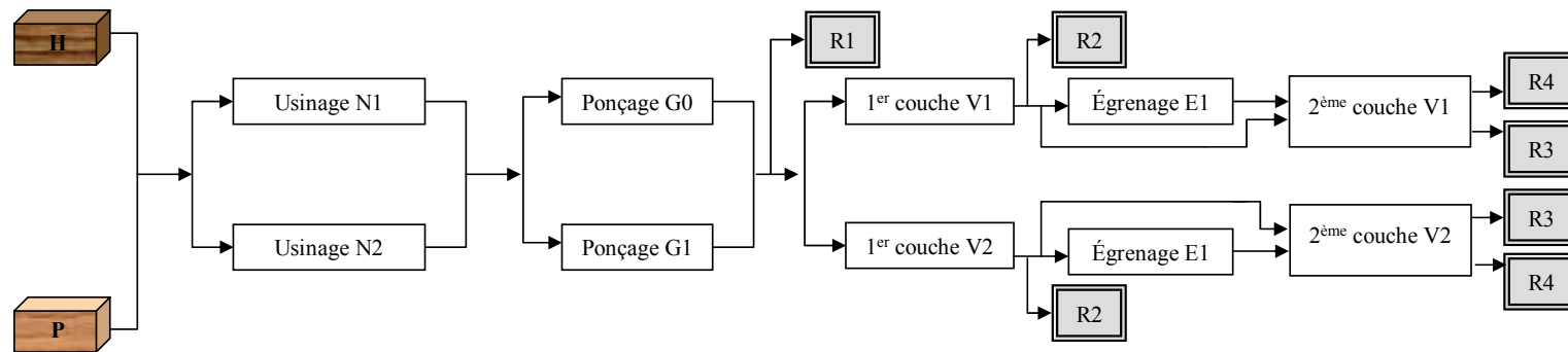
Figure IV.4 - Séquence opératoire pour l'obtention des éprouvettes
