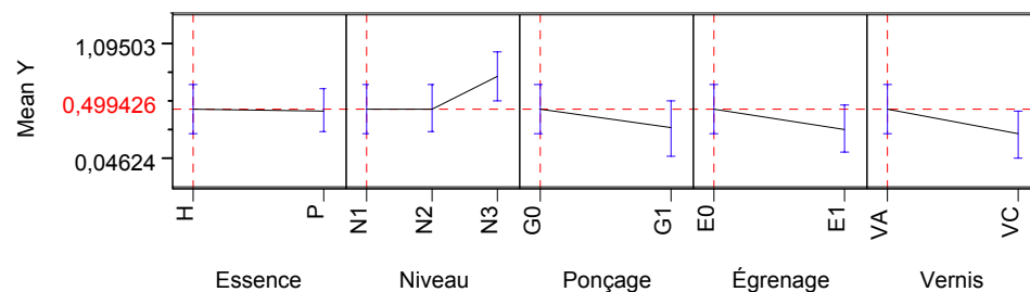
Figure IV.34 - Influence des différents facteurs dans le critère Kond (moyenne)
