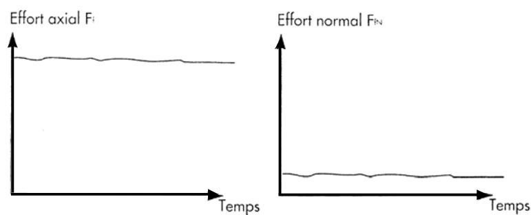
Figure II.22 -Diagramme effort de coupe/temps (d'après Koch, 1964)
