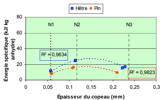
Figure IV.61 - Influence du niveau d'usinage dans l'énergie spécifique
