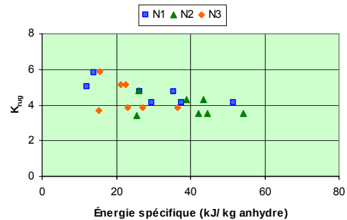
Figure IV.84 - Influence du niveau d'usinage dans le Krug (critère de rugosité)
