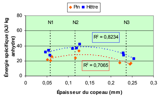
Figure IV.77 - Influence du niveau d'usinage dans l'énergie spécifique
