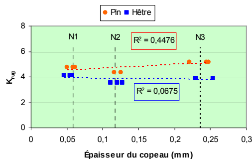
Figure IV.29 - Influence du niveau d'usinage dans le Krug (critère de rugosité)
