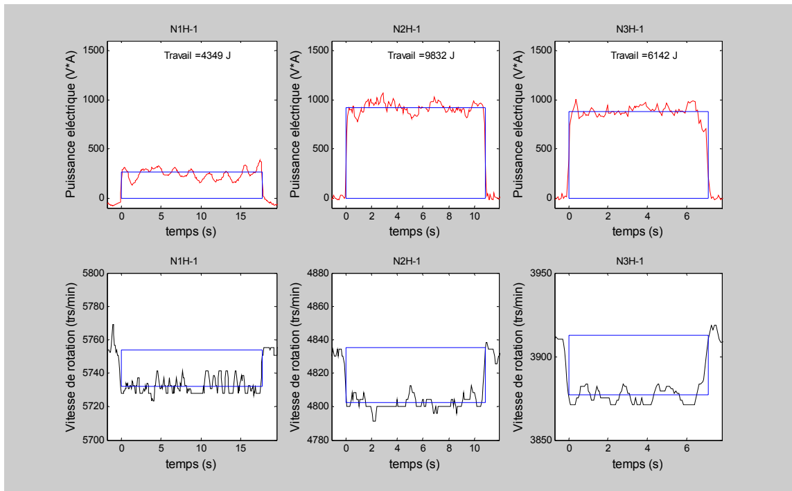
Figure IV.55 - Monitorisation d'usinage – Hêtre
