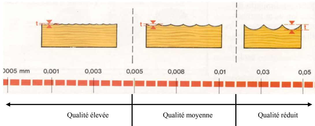
Figure III.10 - Rapport entre la profondeur des marques de coupe et la qualité de la surface du bois (Adapté du manuel de l'équipement industriel réf. WEINIG)
