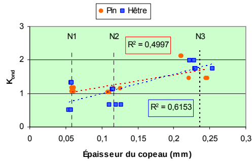
Figure IV.80 - Influence du niveau d'usinage dans le Kond (critère d'ondulation)
