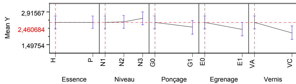
Figure IV.71 - Influence des différents facteurs dans le critère Ksub (moyenne)
