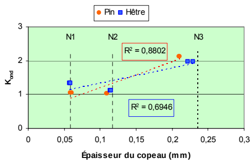
Figure IV.59 - Influence du niveau d'usinage dans le Kond (critère d'ondulation)
