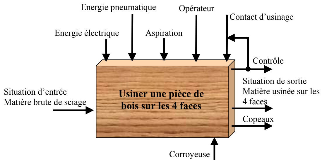
Figure II.34 -L'étude fonctionnelle du système de la corroyeuse
