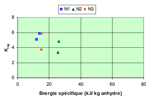
Figure IV.63 - Influence du niveau d'usinage dans le Krug (critère de rugosité)
