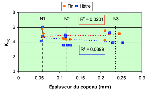
Figure IV.81 - Influence du niveau d'usinage dans le Krug (critère de rugosité)
