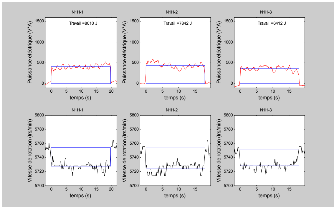
Figure IV.16 - Reproductibilité du système pour le niveau d'usinage 1, pour les trois planches de hêtre
