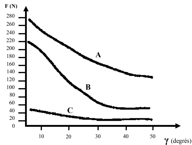
Figure II.17 -Influence de l'angle d'attaque sur les efforts de coupe suivant les directions de coupe A, B, C (voir figure II.1) pour le cas du hêtre (à 12% d'humidité, copeau de 0,2 mm d'épaisseur, outil usé à 50%) (d'après la thèse de Eyma, 2002)
