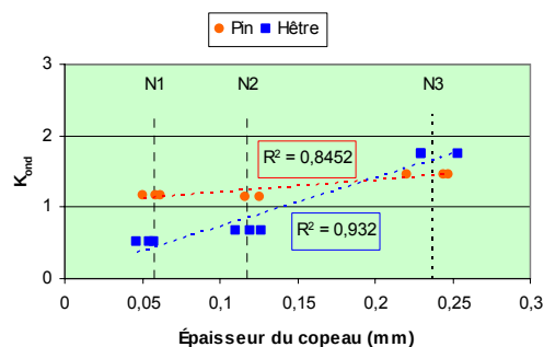
Figure IV.28 - Influence du niveau d'usinage dans le Kond (critère d'ondulation)
