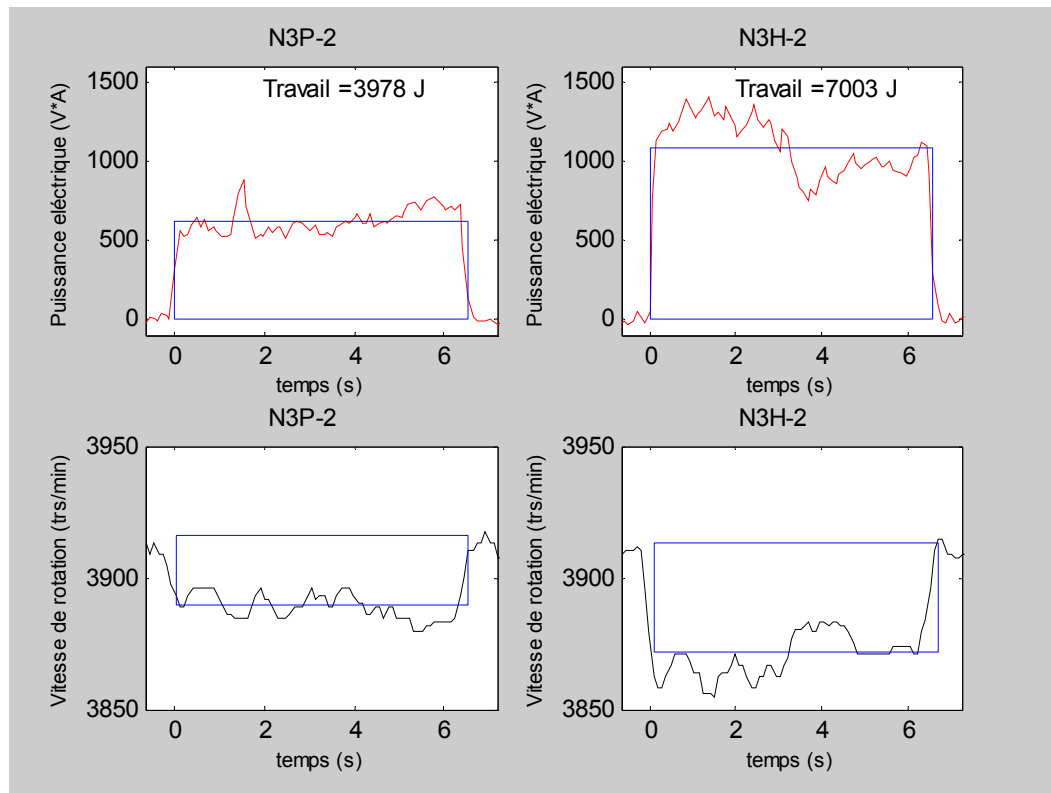
Figure IV.25 - Monitorisation d'usure du pin et de hêtre pour le niveau 3
