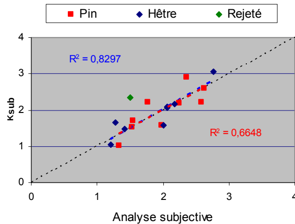
Figure IV.90 - Corrélation entre le critère objectif ( K_{sub} ) et subjectif d'évaluation de la surface
