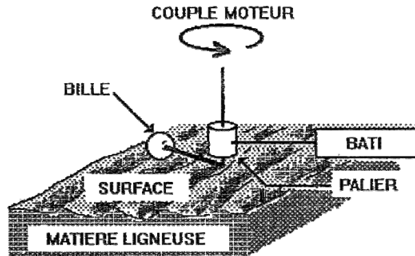
Figure II.45 -Principe de la mesure du frottement
