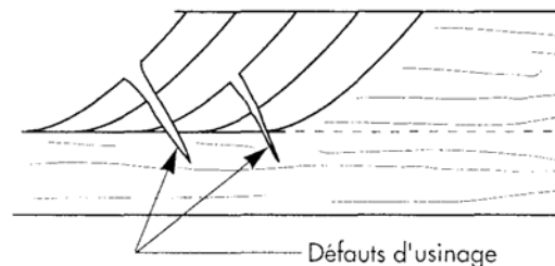
Figure II.30 -Défauts d'usinage dus à la coupe par fendage (d'après Koch, 1964)
