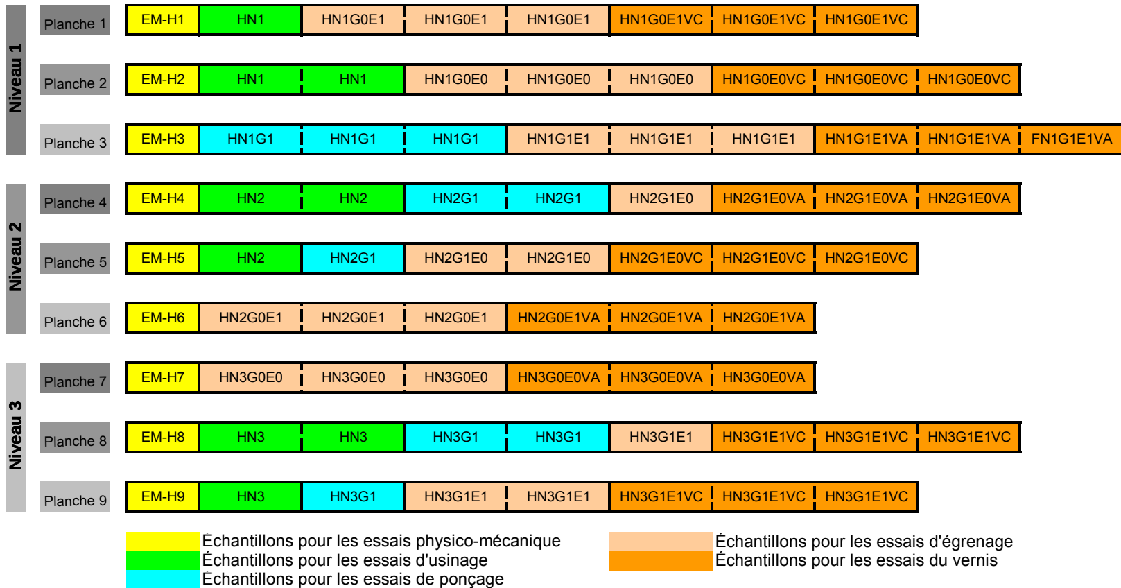
Figure IV.14 - Plan de coupe des éprouvettes de hêtre
