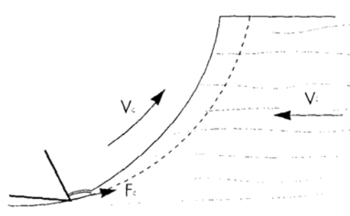
Figure II.27 -1ère phase - flambage (d'après Koch, 1964)
