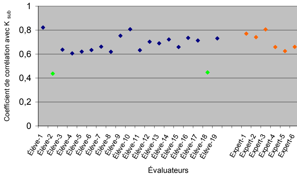
Figure IV.91 - Coefficient de corrélation entre le critère objectif ( K_{sub} ) et l'évaluation subjective de la surface pour chaque observateur
