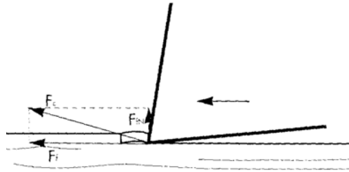
Figure II.23 -Copeau obtenu par flambage (d'après Koch, 1964)
