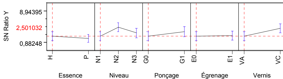
Figure IV.37 - Influence des différents facteurs dans le critère Krug (indice signal-bruit)
