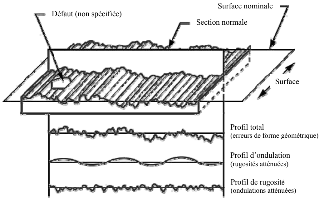
Figure II.35 -Diagramme schématique des caractéristiques de la surface (ASME B46.1, 1995)
