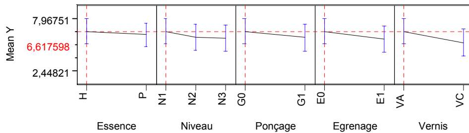
Figure IV.69 - Influence des différents facteurs dans le critère Krug (moyenne)
