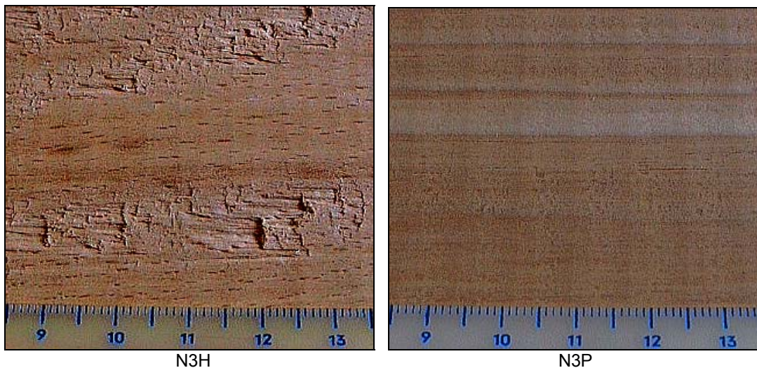
Figure IV.1 - Surface de hêtre (H) et du pin (P), avec l'usinage au niveau 3 (N3)
