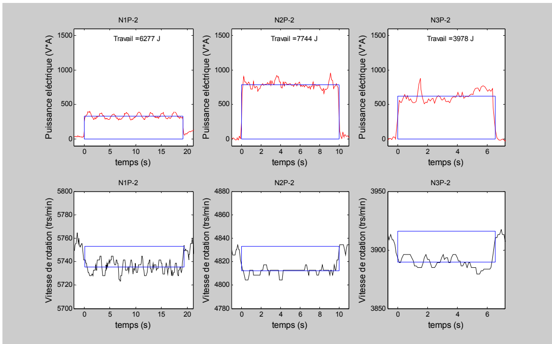
Figure IV.21 - Monitorisation d'usinage – Pin
