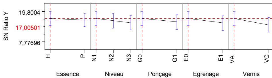
Figure IV.70 - Influence des différents facteurs dans le critère Krug (indice signal-bruit)
