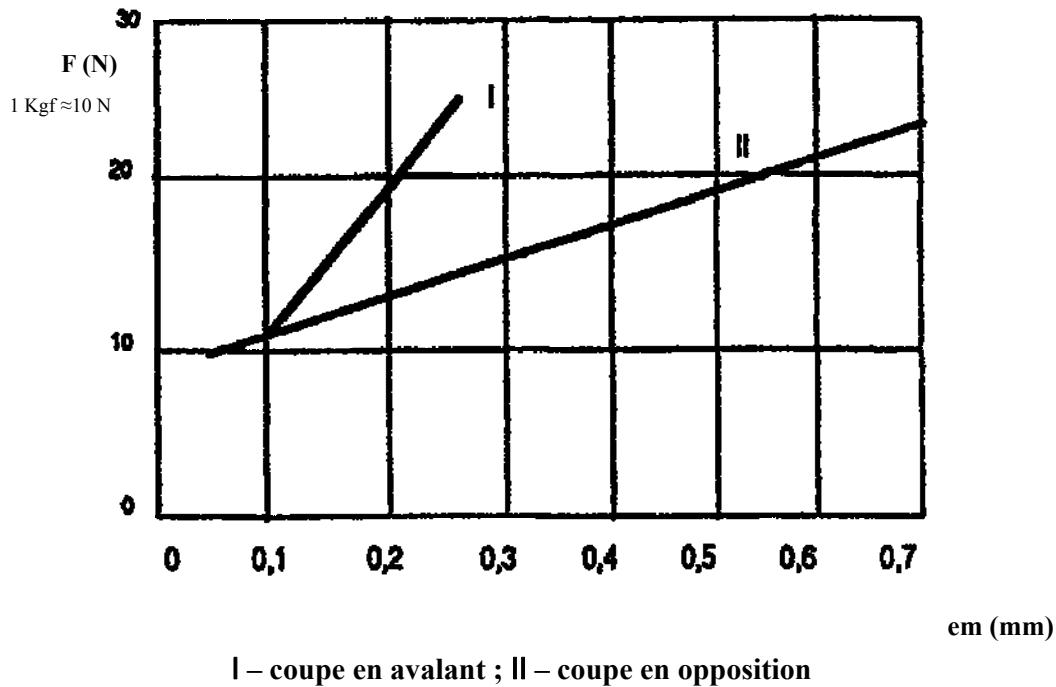
Figure II.15 -Influence du sens de travail de l'outil sur l'effort de coupe (d'après la thèse de Eyma, 2002)
