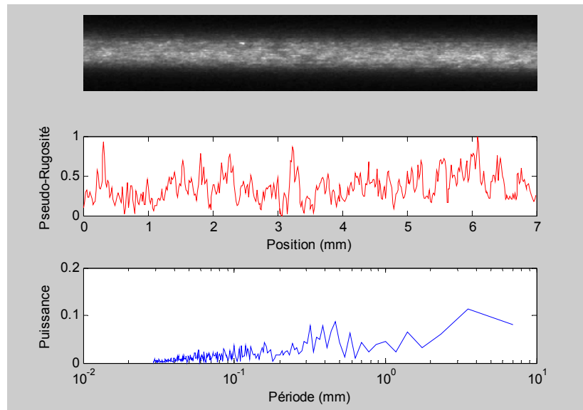
Figure III.7 - Image de la surface d'une éprouvette, profil de pseudo-rugosité et courbe de puissance (FFT)
