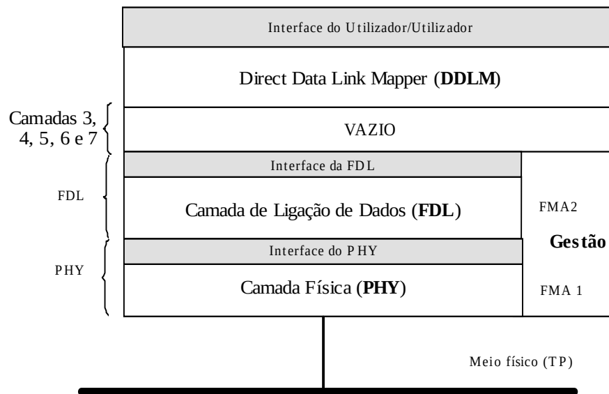
Figura 18 - Arquitetura Protocolar PROFIBUS-DP
