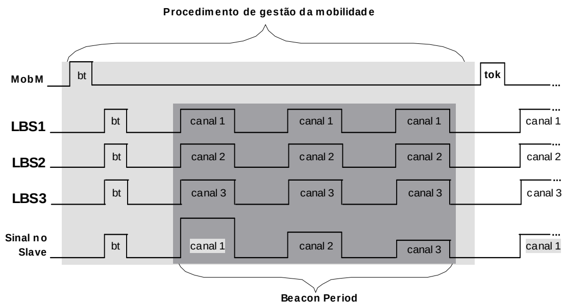
Figura 34 - Diagrama temporal do procedimento de gestão da mobilidade
