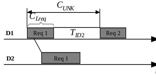
Figura 82 - Duração de um ciclo de mensagem sem resposta/ack
