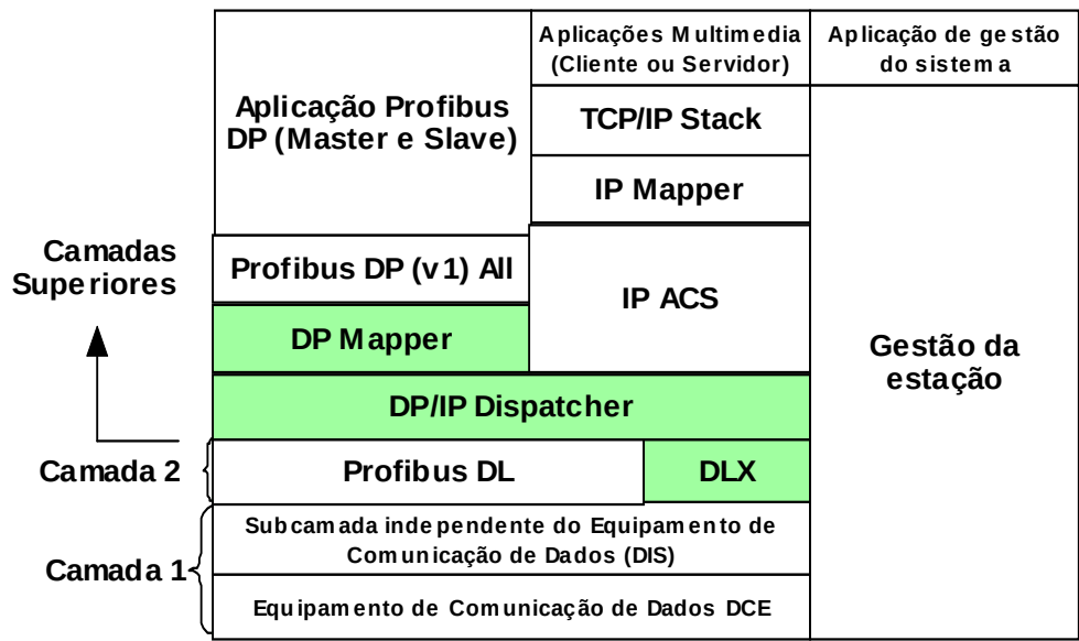
Figura 37 - Arquitectura do protocolo de comunicações para estações RFiellbus (ES)
