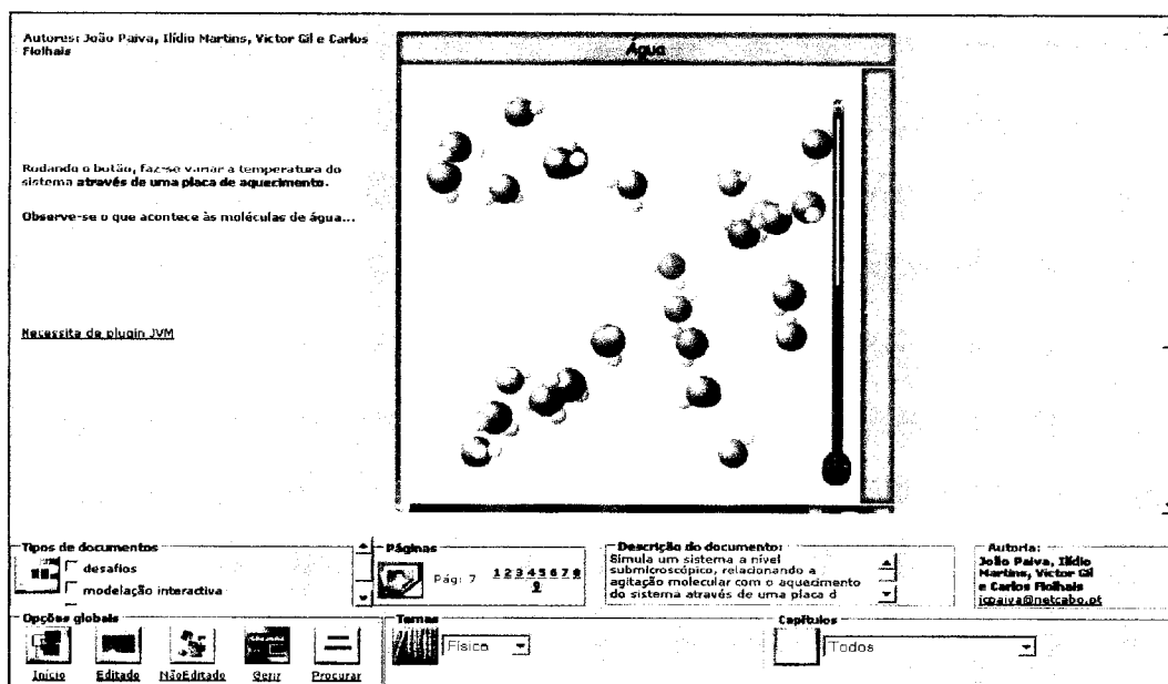
Imagem A. 7 - Simula um sistema a nível submicroscópico, relacionando a agitação molecular com o aquecimento do sistema através de uma placa de aquecimento (João Paiva, Ilídio Martins, Victor Gil e Carlos Fiolhais)
