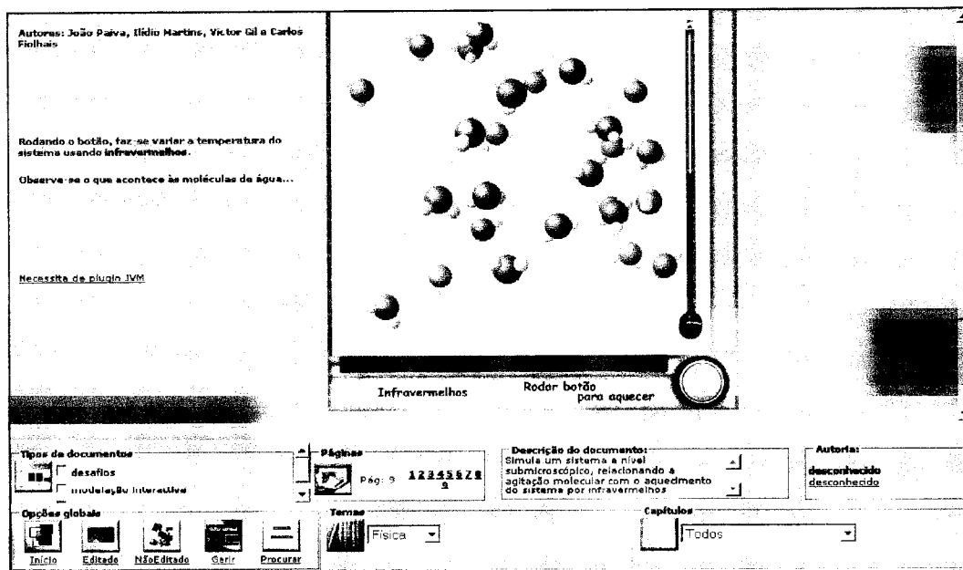
Imagem A. 9 - Simula um sistema a nível submicroscópico, relacionando a agitação molecular com o aquecimento do sistema por infravermelhos (João Paiva, Ilídio Martins, Victor Gil e Carlos Fiolhais)
