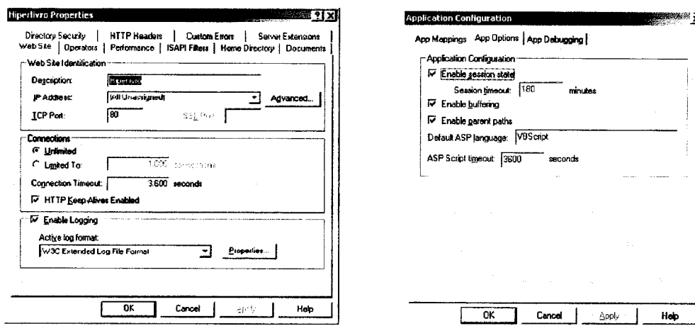
Imagem 45 – Janelas de configuração do servidor Web (IIS) especificando a permissão de uma ligação até 1 hora (3600 segundos)
