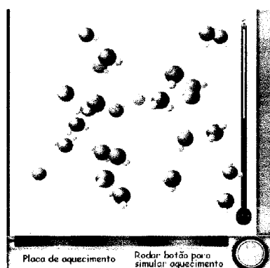
Imagem 40 – Modelação de uma simulação submicroscópica ilustrando a variação da agitação de moléculas de água por aquecimento
