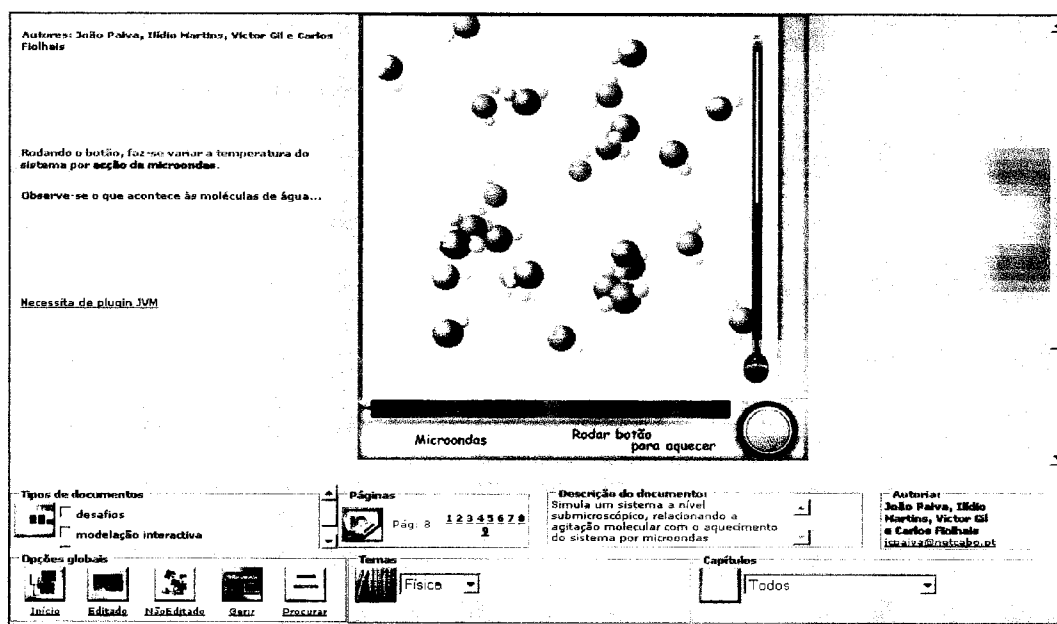
Imagem A. 8 - Simula um sistema a nível submicroscópico, relacionando a agitação molecular com o aquecimento do sistema por microondas (João Paiva, Ilídio Martins, Victor Gil e Carlos Fiolhais)
