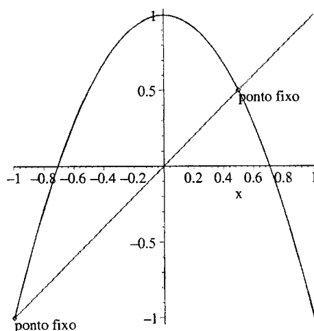
Figura 2.4: Pontos fixos de f(x) = 1 - 2x^2 no intervalo [-1, 1]
