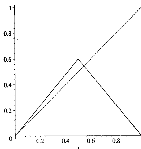
Figura 3.6: pontosfixosplot de T_{1.2}
