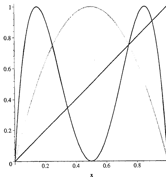
Figura 2.7: Pontos periódicos de período dois de f(x) = 4x(1 - x)
