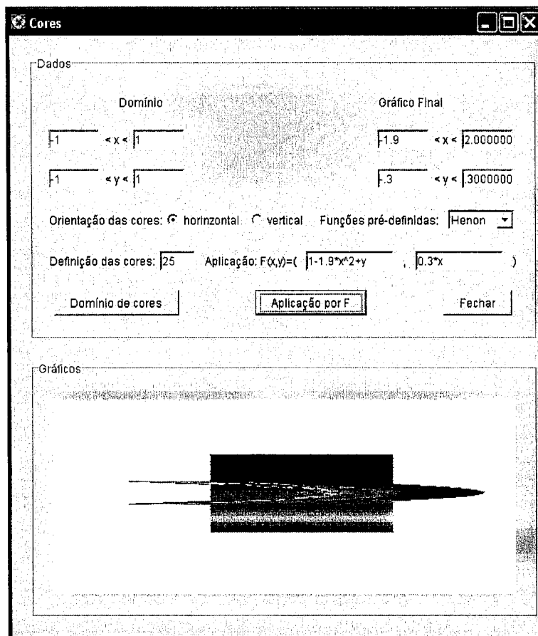
Figura 5.10: Região [-1, 1] \times [-1, 1] invariante por F(x, y)
