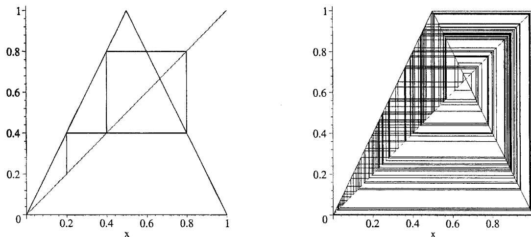
Figura 3.4: Representação gráfica da órbita para x_0 = 0.2 e para x_0 = 0.2001
