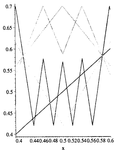
Figura 3.16: Pontos periódicos de período seis de T_{1.4}(x) no intervalo [0.4; 0.6]
