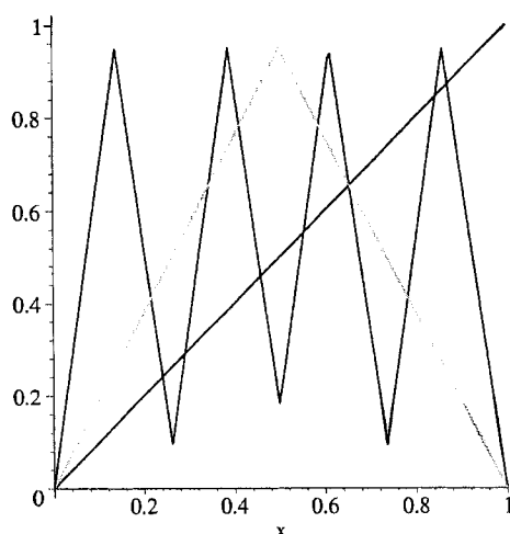
Figura 3.14: Pontos periódicos de período três de T_{1,9}(x)
