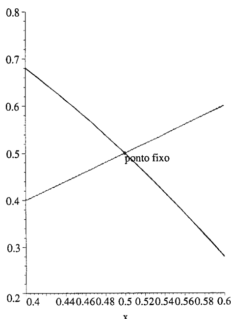
Figura 2.6: Pontos fixos de f(x) = 1 - 2x^2 no intervalo [0.4, 0.6]
