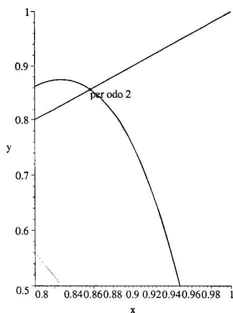
Figura 4.9: perdoisplot f_{3.5} com xmin = 0.8 e xmax = 1
