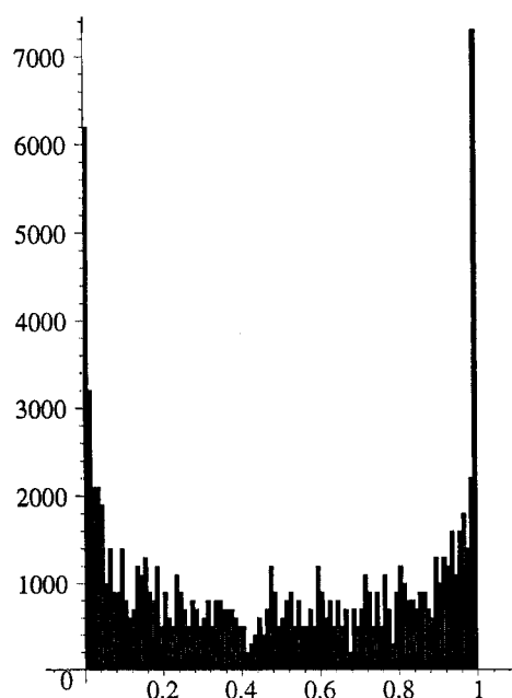
Figura 2.13: Diagrama de frequências de x_0 = 0.2 pela função f(x) = 4x(1 - x)
