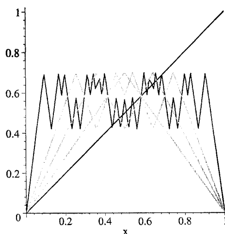
Figura 3.15: Pontos periódicos de período seis de T_{1.4}(x)
