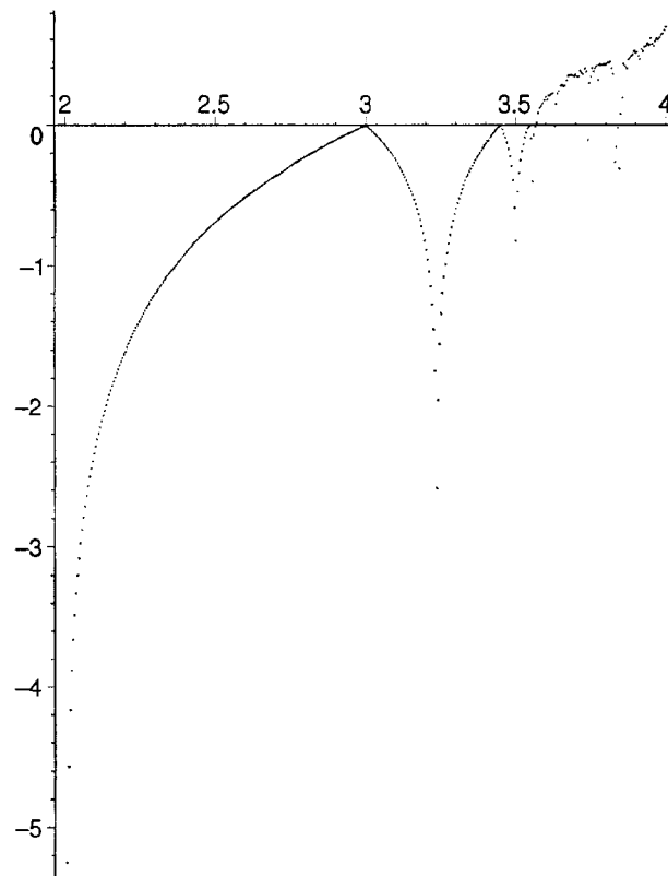
Figura 4.22: Diagrama dos expoentes de Lyapunov
