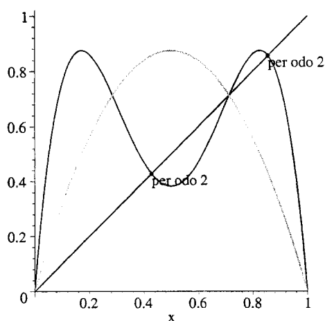
Figura 4.8: perdoisplot f_{3.5} com xmin = 0 e xmax = 1
