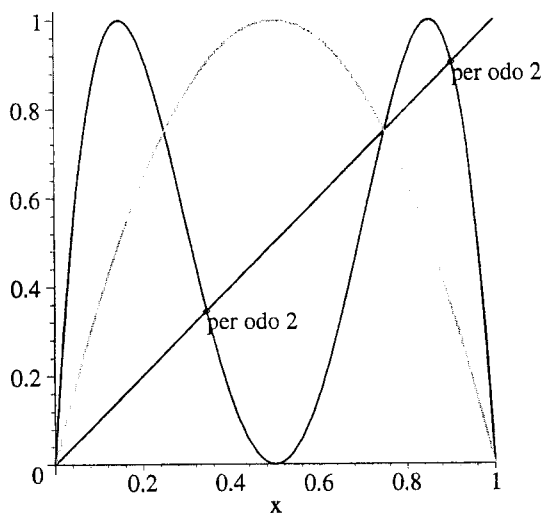
Figura 2.8: Indicação dos pontos periódicos de período dois de f(x) = 4x(1 - x)
