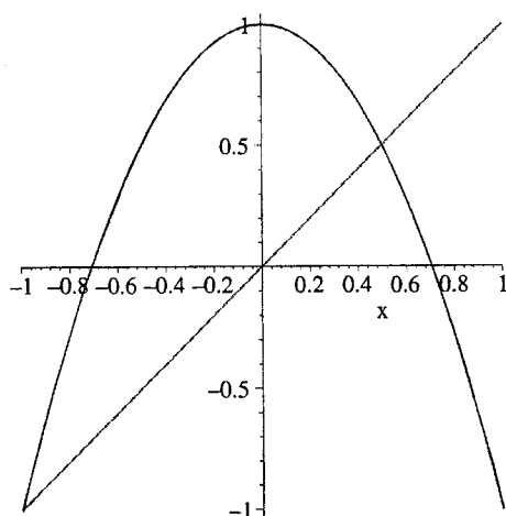
Figura 2.3: Pontos fixos de f(x) = 1 - 2x^2 no intervalo [-1, 1]
