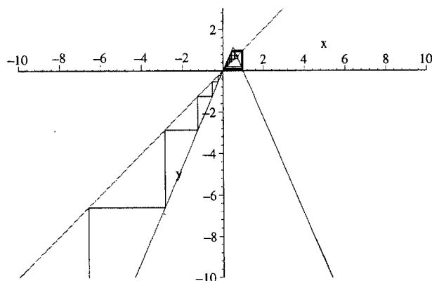
Figura 3.5: Órbita de T_{2.3}(0.4)
