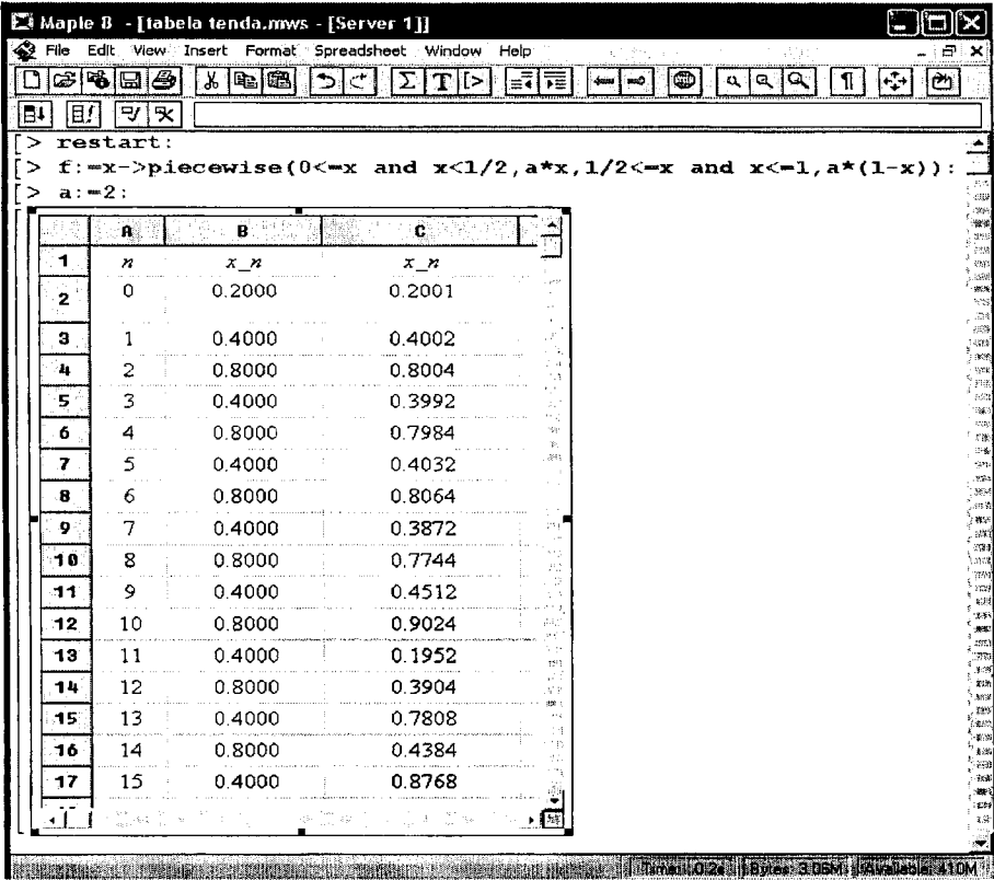
Figura 3.3: Primeiros quinze elementos da órbita de T_2(0.2) e de T_2(0.2001)
