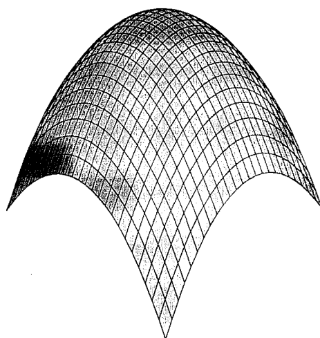
Figura 1.9: Gráfico do parabolóide z = -x^2 - y^2
