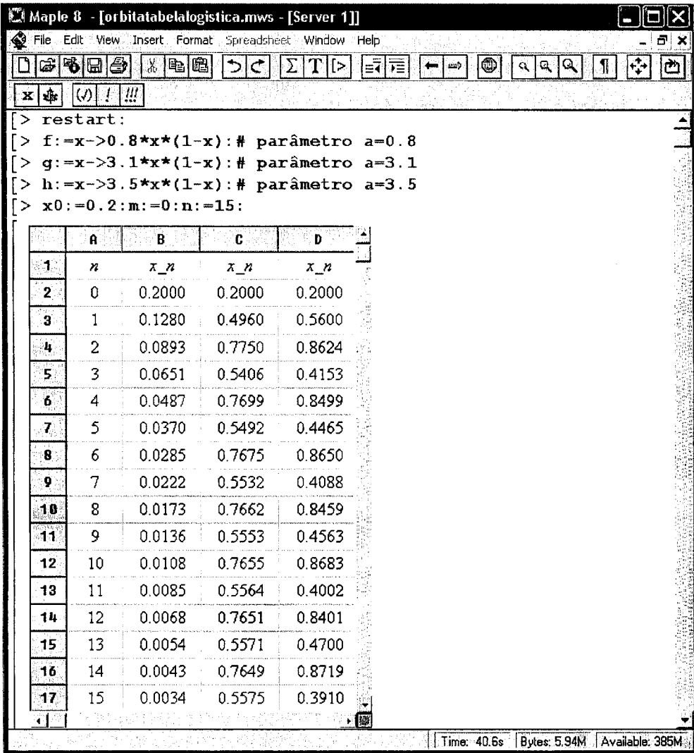
Figura 4.3: Primeiros quinze elementos da órbita de f_{0.8}(0.2) , f_{3.1}(0.2) e de f_{3.5}(0.2)
