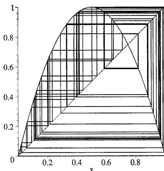
Figura 2.12: Órbita de x_0 = 0.2 pela função f(x) = 4x(1 - x)
