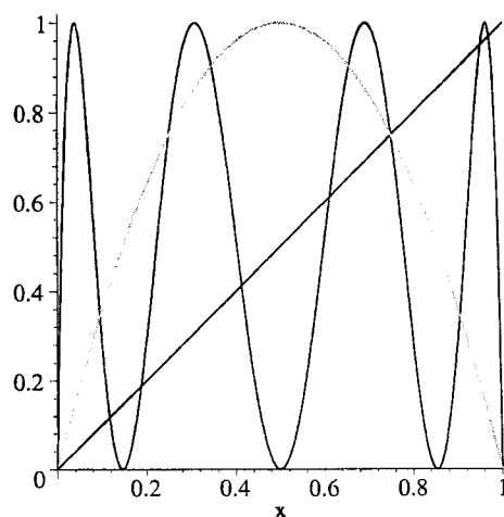
Figura 2.9: Pontos periódicos de período três de f(x) = 4x(1-x)
