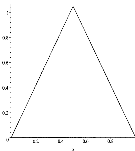
Figura 3.2: Gráfico da aplicação tenda para a = 2.1
