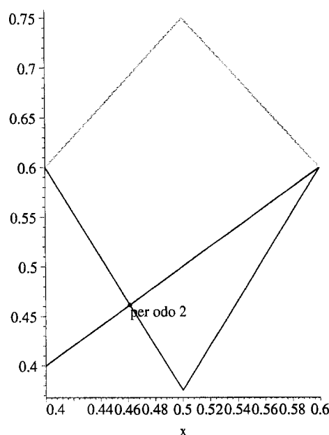
Figura 3.12: perdoisplot de T_{1,2}(x) com xmin = 0.4 e xmax = 0.6
