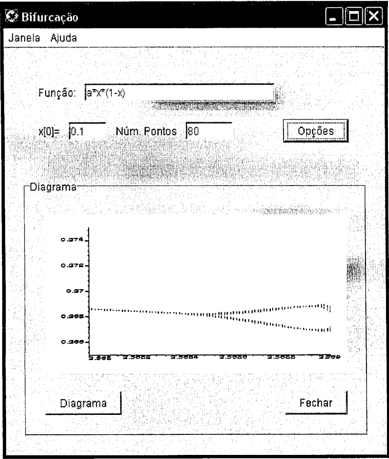
Figura 5.8: Bifurcação em a = 3.5687594 obtida com a Maplet bifurcação
