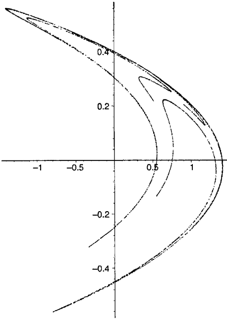
Figura 5.11: Atrator de Hénon
