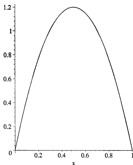
Figura 4.2: Gráfico da aplicação logística para a = 4.8
