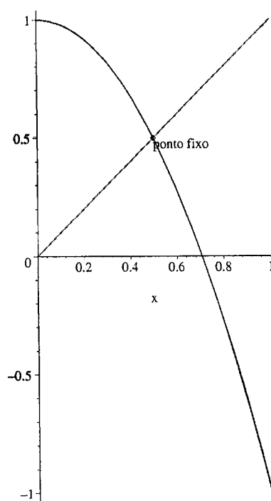
Figura 2.5: Pontos fixos de f(x) = 1 - 2x^2 no intervalo [0, 1]
