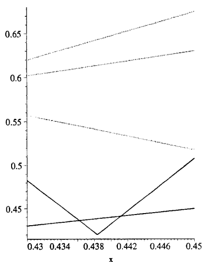
Figura 3.17: Pontos periódicos de período seis de T_{1,4}(x) no intervalo [0.43; 0.45]
