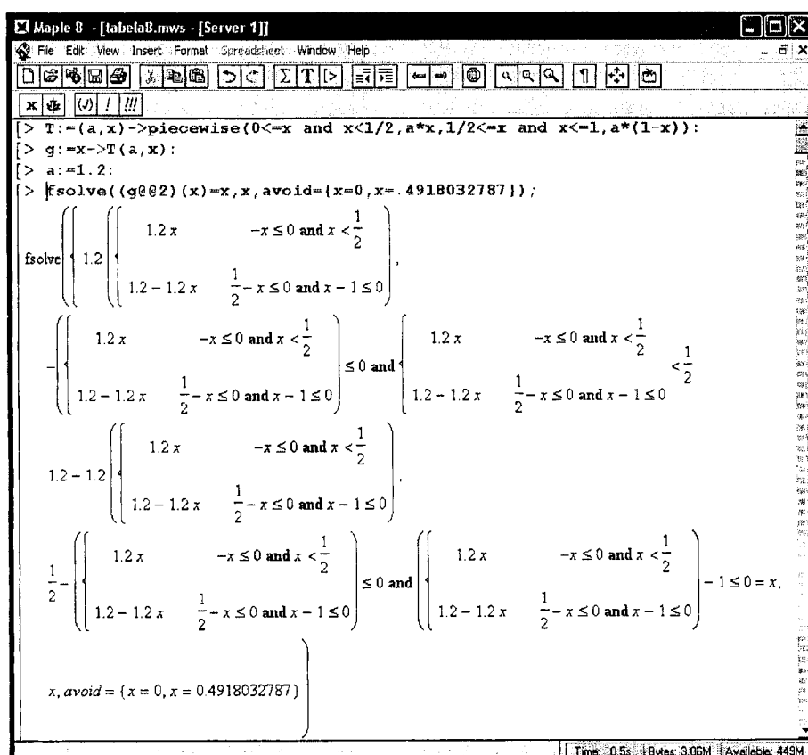
Figura 3.9: Resposta dada ao tentar determinar a terceira raiz da equação T_{1.2}^2(x) = x
