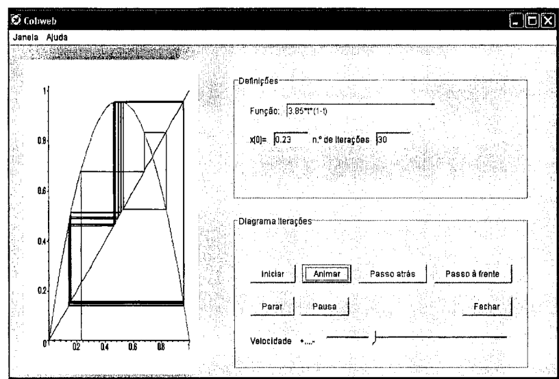
Figura 5.5: Maplet da representação gráfica da órbita de um ponto pela aplicação logística
