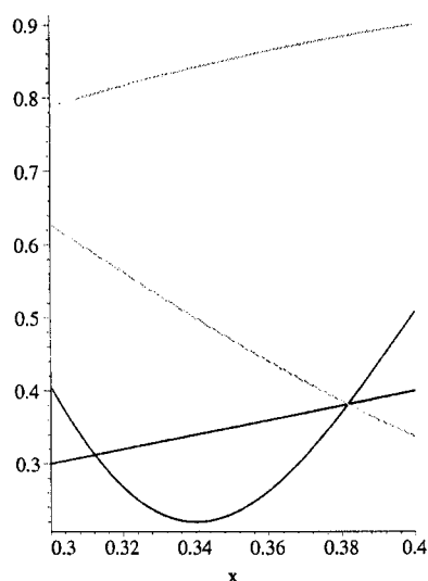
Figura 4.12: ponto periódico de período 4 de f_{3.75} em [0.3, 0.4]
