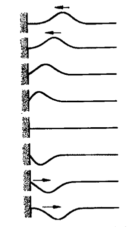
Figura 3.3 – A fase do impulso reflectido é invertida, sendo de 180^\circ a diferença de fase entre o impulso incidente e o reflectido.
