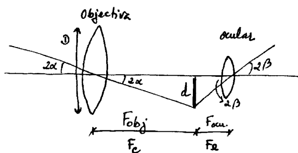
Figura 4.2 – Representação esquemática de um refractor.
