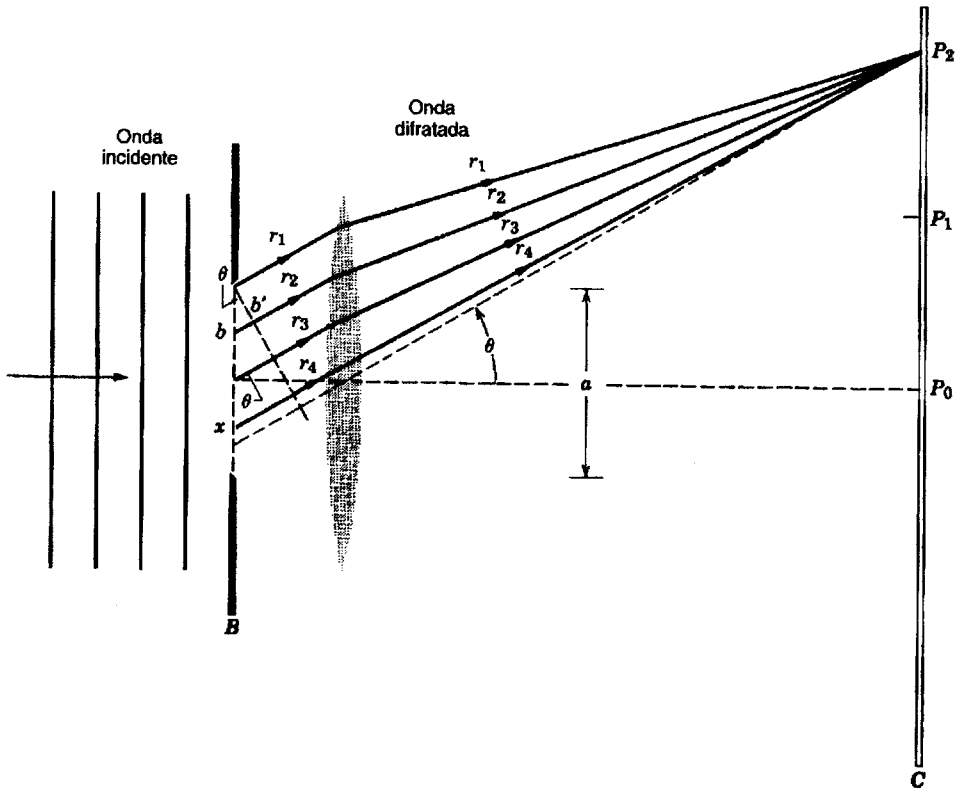
Figura 3.8 – As condições para o segundo mínimo do padrão de difracção. O ângulo \theta é tal que a distância bb' é igual a meio comprimento de onda.
