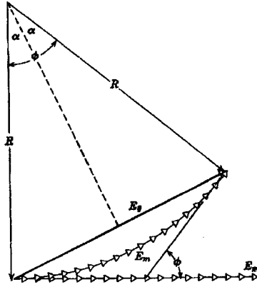
Figura 3.11 – Uma construção usada para calcular a intensidade na difração de fenda única.
