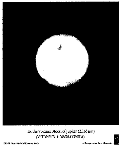
Figura 7.14 - Imagem da lua Io, foi obtida com um filtro de 2.166 \mu\text{m} , obtida a 5 de Dezembro de 2001.
