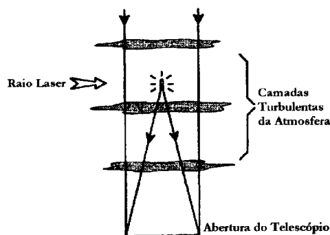
Figura 6.3 – Anisoplanetismo focal ou efeito de cone dado por uma amostra incompleta da turbulência atmosférica com um raio laser.
