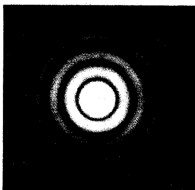
Figura 3.12 – Padrão de difracção de uma abertura circular.
