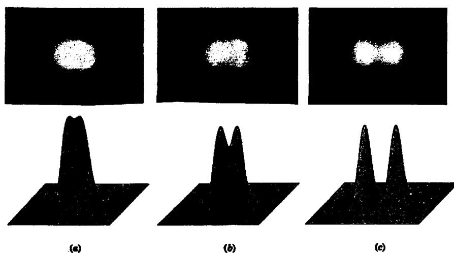
Figura 3.13 – Imagens de duas fontes pontuais (estrelas) distantes formadas por uma lente convergente. Por baixo das imagens estão representados perfis das intensidades gerados por computador.
