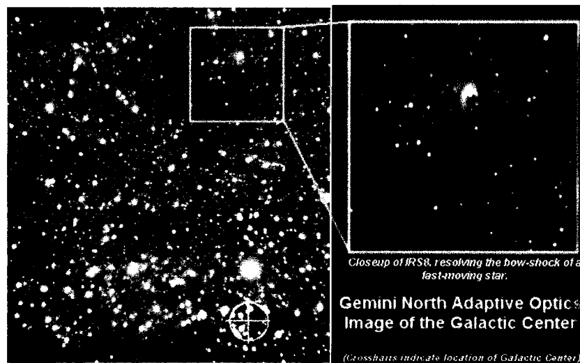
Figura 7.1 - A poucos anos de luz do Centro da Galáxia (cruz amarela) encontra-se o IRS8. Distingue-se a onda de choque que a estrela produz no gás circundante.
