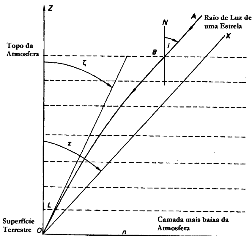
Figura 5.5 – Refracção da luz de uma estrela pela atmosfera terrestre.
