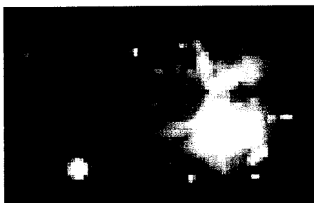
Figura 7.8 – Imagem infravermelha de uma estrela que dá forma à região G45.45+0.06 da nossa Galáxia, obtida com o telescópio Gemini (Norte).
