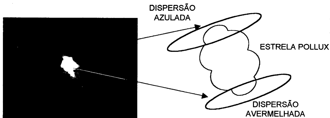
Figura 4 – Dispersão da luz da Pollux
