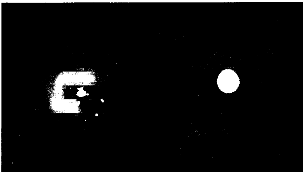
Figura 7.3 - Imagens da região nuclear da galáxia próxima NGC 7469, a da direita é sem óptica adaptativa e a imagem da esquerda obtida com óptica adaptativa (CFHT).
