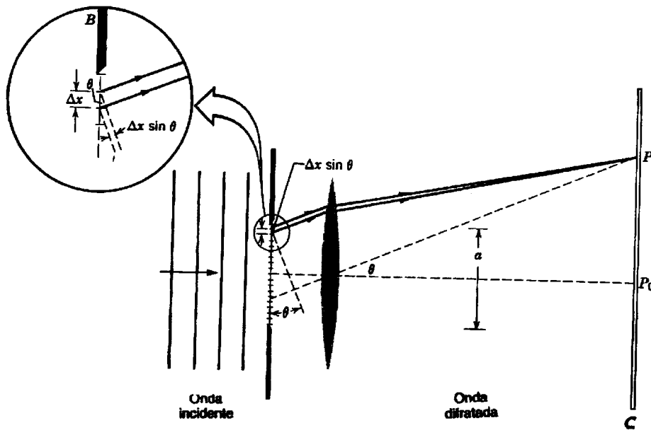
Figura 3.9 – Uma fenda de largura a é dividida em N faixas de largura \Delta x .
