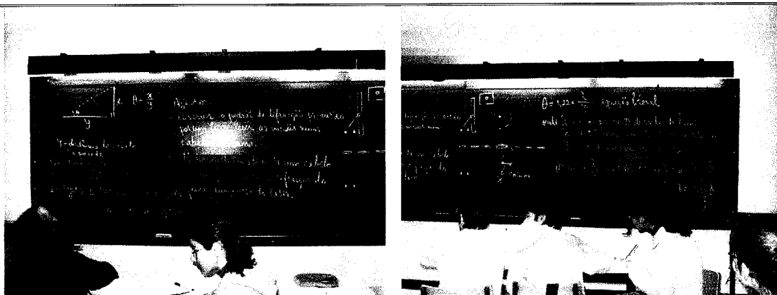
Figura 4 – Explicação teórica e cálculos do diâmetro do cabelo.
