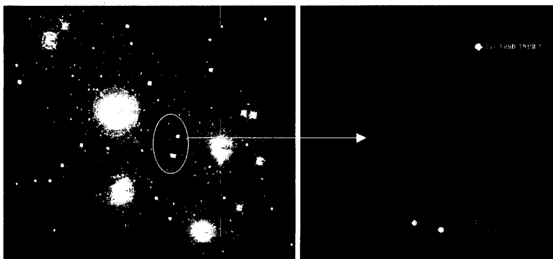
Figura 1 – A imagem da esquerda foi obtida com o programa starry night e mostra as estrelas Pleiades. A imagem da direita foi obtida pelo telescópio Celestron CG-11 usando um CCD.
