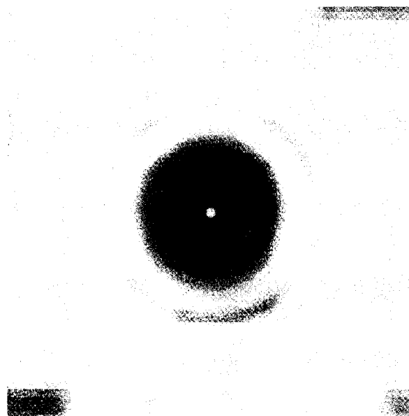
Figura 3.5 – Difracção num disco circular.
