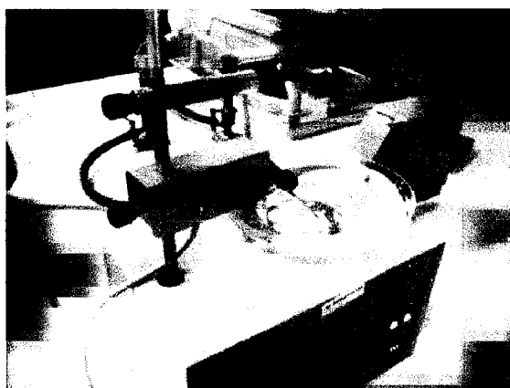
Figura 1 – Observação da refração utilizando a ponta linear.
