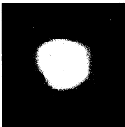
Figura 7.9 – Imagem da nebulosa planetária BD+303639 obtida no observatório Gemini.
