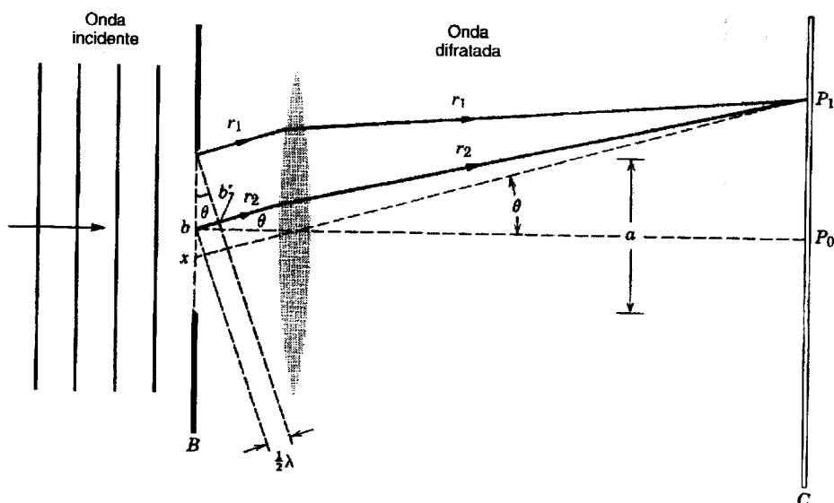
Figura 3.7 – As condições para o primeiro mínimo do padrão de difracção.
