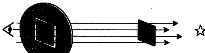
Figura 6.1 – Sistema de mira, anterior à invenção do telescópio, usado por Tycho Brahe, no século XVI, para eliminar a paralaxe. A estrela foi alinhada por cima simultaneamente pelas quatro fendas dos quatro lados da pínula quadrada.
