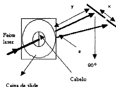
Figura 1 – Representação do ângulo \theta . Figura 2 – Esquema do raio laser ao incidir no cabelo.
