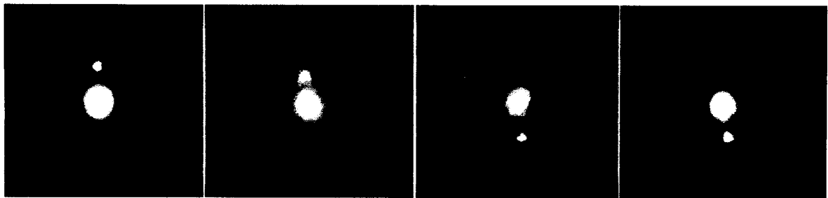
Figura 7.7 – Sequência de quatro imagens infravermelhas de Plutão e da sua lua Caronte.
