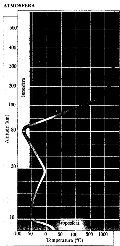
Figura 5.1 – Camadas da atmosfera terrestre.
