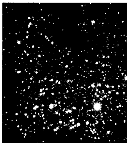
Figura 7.10 – Observação do centro galáctico com o telescópio Gemini do Norte.
