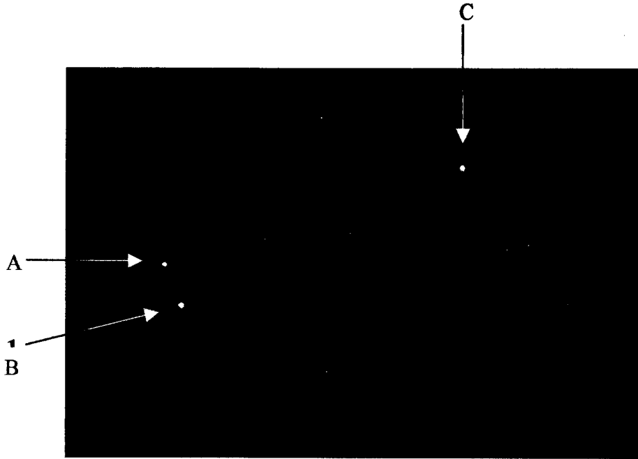
Figura 2 – Imagem de três Pleiades: A – TYC 1800-1961-1; B – TYC 1800-1974-1 e C - TYC 1800-1908-1.
