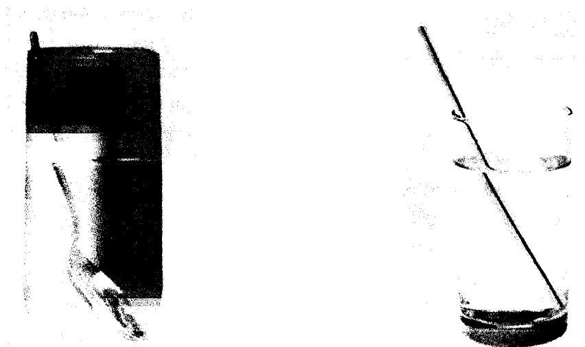
Figura 5.3 – Uma colher e uma palhinha mergulhadas na água parecem quebradas à superfície.
