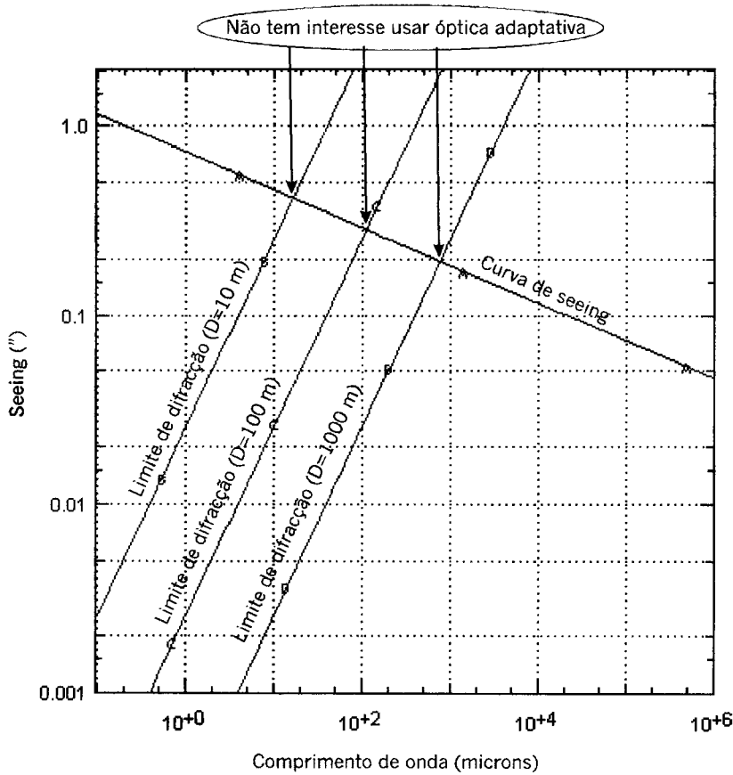
Figura 5.8 – Gráfico que relaciona o limite de difracção com o seeing.
