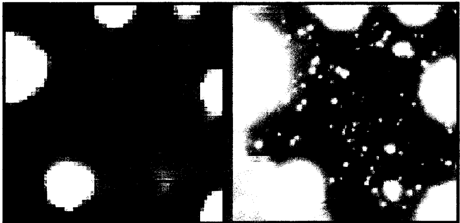
Figura 7.6 – A imagem da direita mostra uma pequena região do núcleo do aglomerado globular M13 usando o Hokupa'a com 2,2\ \mu m . A imagem da esquerda mostra o campo correspondente a uma imagem de curta exposição nos comprimentos de onda do visível ( 0,55\ \mu m ) usando a câmara de aquisição.
