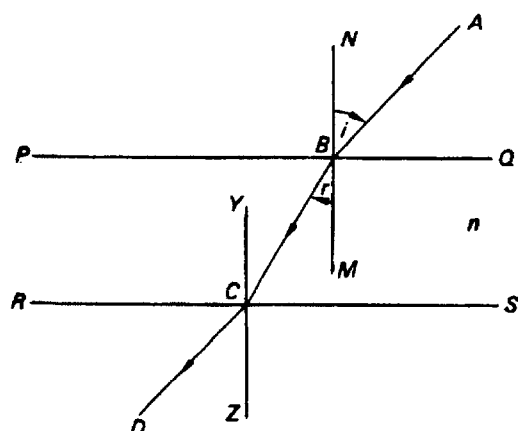
Figura 5.4 – Representação do trajecto de um raio através da lâmina de faces paralelas.
