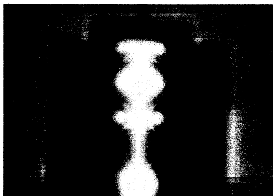
Figura 3.6 – Padrão de difracção gerado por uma lâmina de barbear iluminada com luz monocromática.
