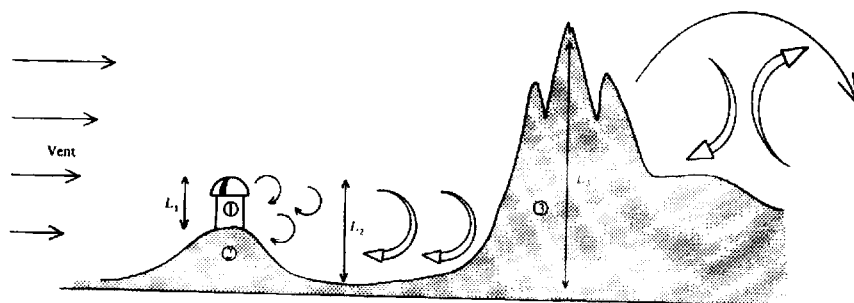
Figura 5.7 – Representação esquemática da geração da turbulência atmosférica por diferentes obstáculos. As escalas L_1 , L_2 e L_3 são características das escalas externas.
