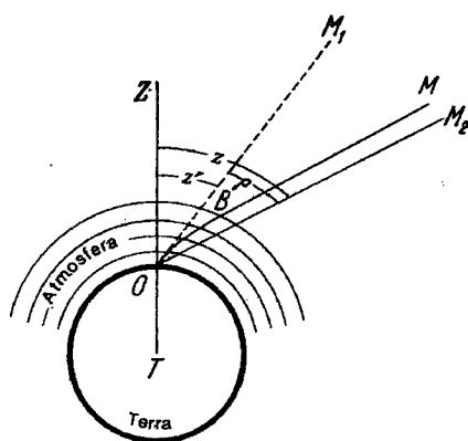
Figura 5.6 – Refracção atmosférica.
