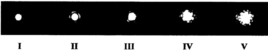
Figura 4.3 – Imagens das categorias do seeing segundo a escala de Antoniadi.
