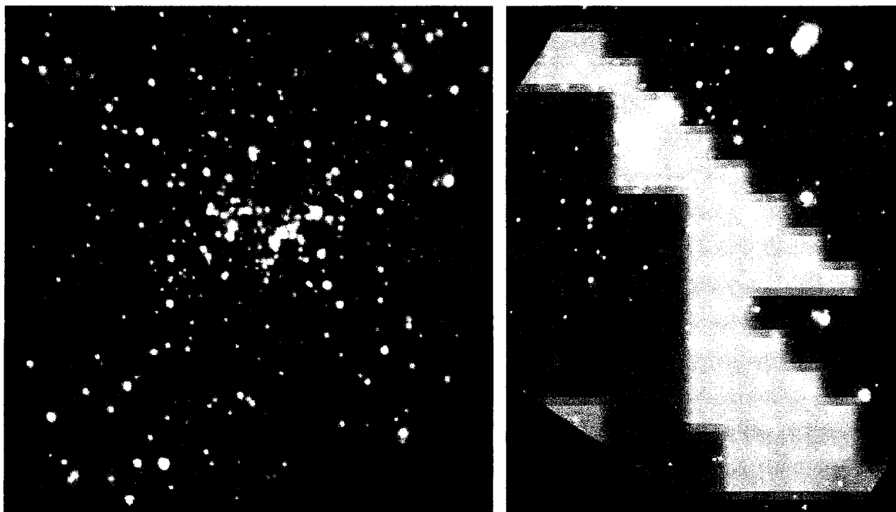
Figura 7.11 – Imagens do aglomerado globular NGC 6934. A imagem da esquerda é uma imagem óptica e a da direita é uma imagem infravermelha do mesmo aglomerado e foram ambas obtidas com o telescópio Gemini recorrendo ao sistema de óptica adaptativa Hokupa’a.
