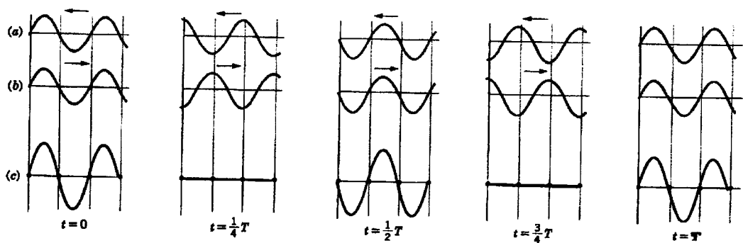
Figura 3.2 – a) e b) Duas ondas progressivas com o mesmo comprimento de onda e a mesma amplitude e movendo-se em sentidos contrários. c) A sobreposição das duas ondas em instantes de tempo diferentes.
