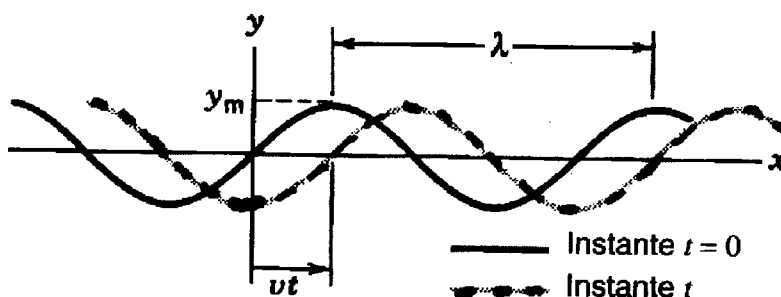
Figura 2.4 – No instante t , a onda percorre a distância x = vt , para a direita. As duas ondas têm forma sinusoidal.
