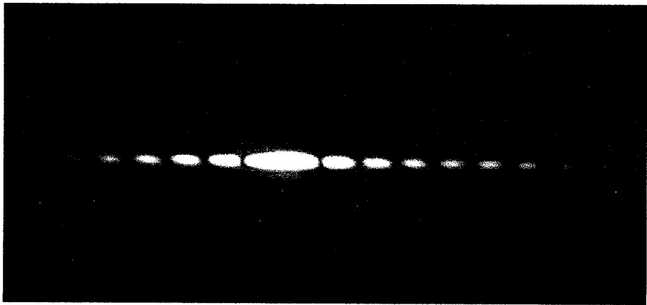
Figura 3 – Teste padrão de difracção criado por um cabelo humano.
