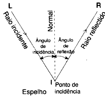
Figura 2.6 – O raio que incide segundo LI reflecte-se segundo IR. Do mesmo modo, um raio que incida segundo RI reflectir-se-á segundo IL.
