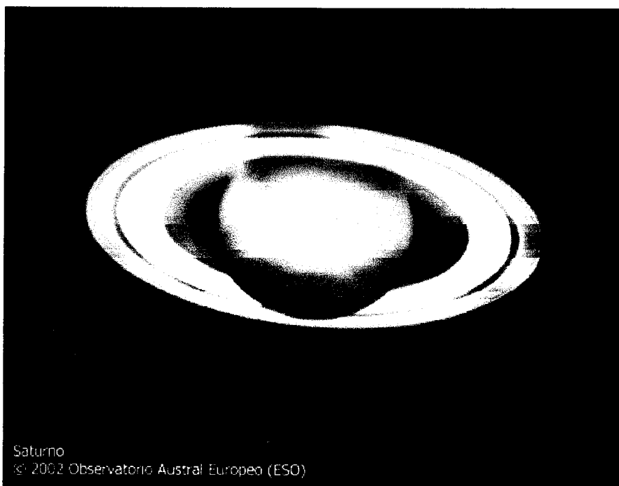
Figura 7.13 - Esta fotografia de Saturno foi obtida a 8 de Dezembro de 2001 através do sistema NAOS-CONICA. São visíveis várias estruturas na atmosfera de Saturno bem como um grande pormenor na região dos anéis. A lua Thetys é visível na região abaixo do planeta.
