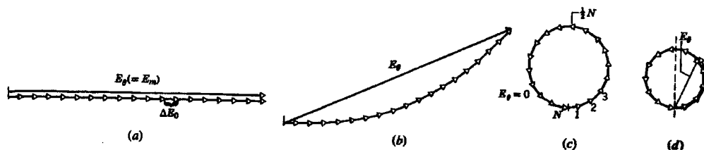
Figura 3.10 – Fasores na difracção de fenda única. Mostra as condições:
