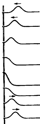
Figura 3.4 – A fase da onda reflectida não muda em relação à fase da onda incidente.
