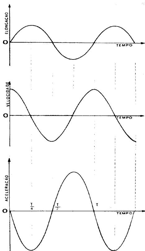
Figura 2.1 - Representações gráficas das funções de elongação, velocidade e aceleração relativas a um mesmo oscilador harmónico.
