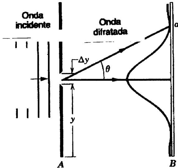
Figura 3.14 — Um feixe de electrões incidente é difractado na fenda da tela A. Se estreitarmos a fenda, o padrão torna-se mais largo.
