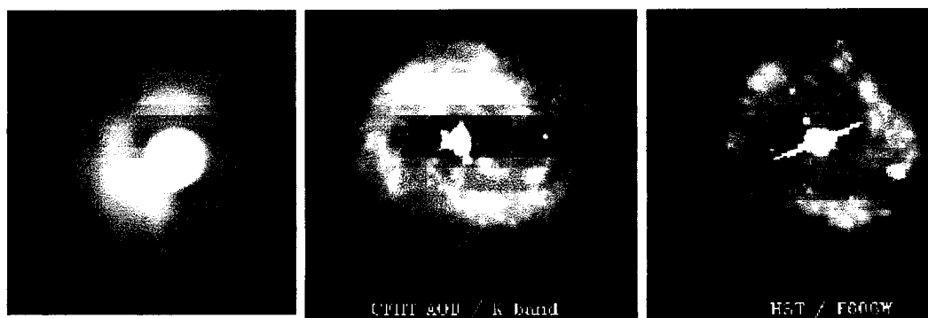
Figura 7.5 - A imagem da esquerda é típica de um grande telescópio sem óptica adaptativa. A largura a meia altura (FWHM) é de 0,7 arcsec. Nas imagens do centro e da direita faz-se a comparação de uma imagem da galáxia NGC7469 De Seyfert obtida na banda K usando óptica adaptativa PUEO do CFHT (FWHM=0,13 arcsec) com uma imagem obtida pelo HST da mesma galáxia.
