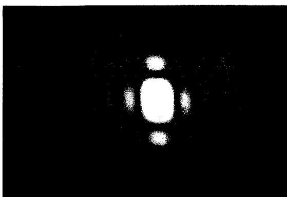
Figura 1 – Teste padrão de difracção criado por um orifício circular.
