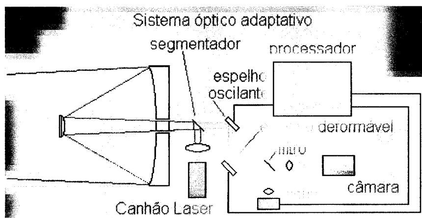
Figura 6.2 – Imagem esquemática do funcionamento de um sistema de óptica adaptativa.
