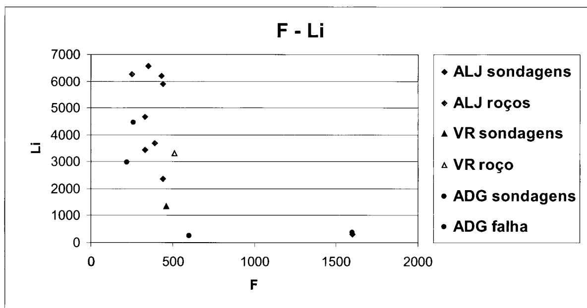
Figura VI.19 - Diagrama de relação Li-F nas amostras dos filões estudados, onde se verifica uma certa correlação negativa. As amostras alteradas destacam-se pelo seu enriquecimento em F.
