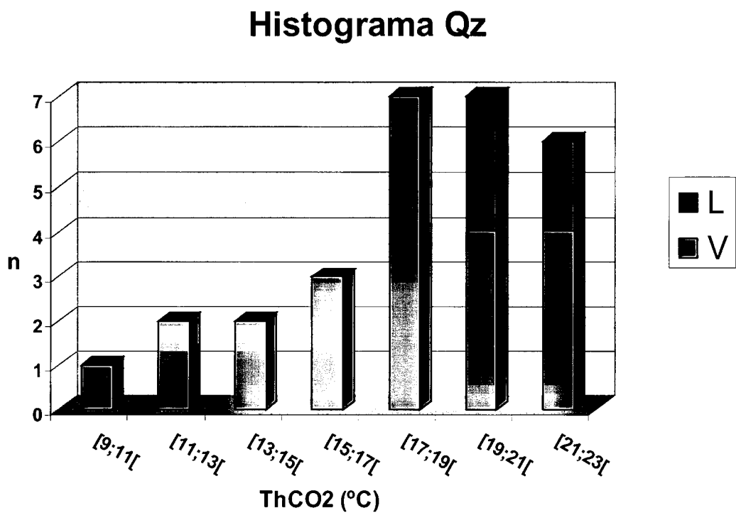
Fig. V.3e – Histograma do n.º de medidas em IF contido em cada classe de temperatura de homogeneização do CO 2 .
