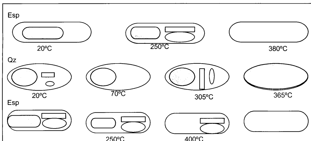
Figura V.19 – Esquema representando os diferentes comportamentos das IF, face ao aquecimento tanto no quartzo como na espodumena.
