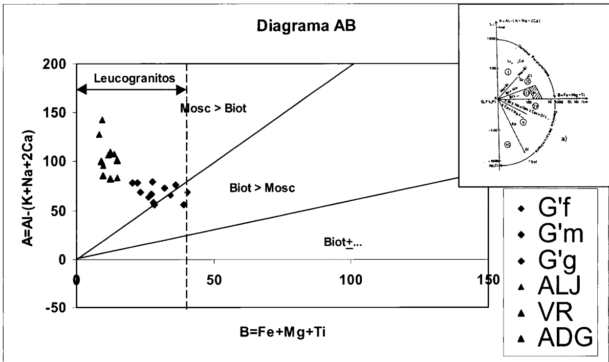
Figura VI.13 - Diagrama A-B de minerais característicos (Debon & Le Fort, 1982). Os filões projectam-se no campo dos leucogranitos e com uma maior percentagem de moscovite do que biotite. Os granitos formam um alinhamento típico da alumina. (Parâmetros expressos em milicátions de cada elemento em 100g de rocha).
