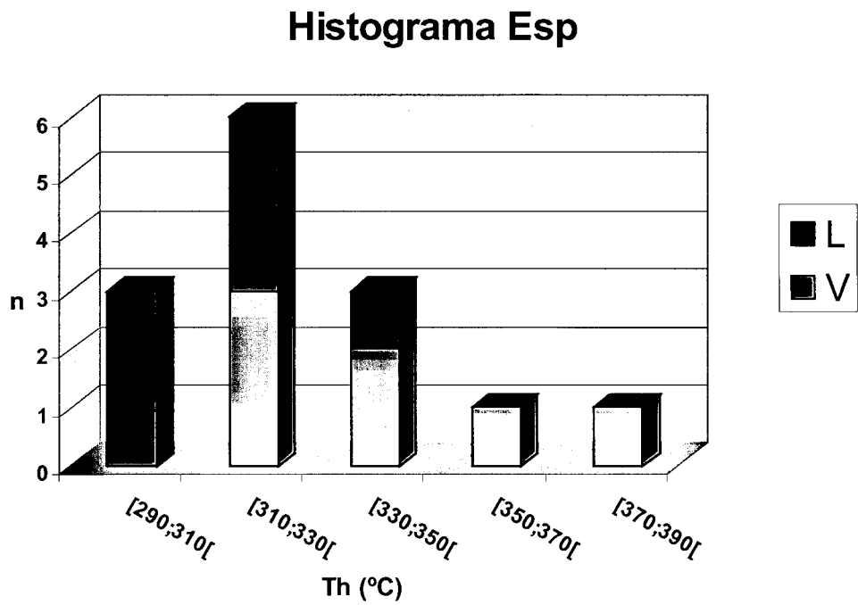
Fig. V.2f – Histograma do n.º de medidas em IF contido em cada classe de homogeneização global.
