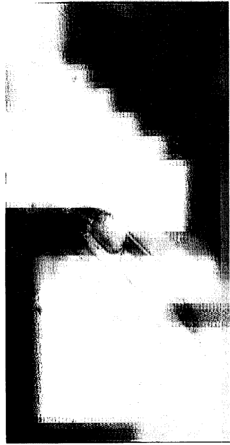
Est. V.2a – IF tipo Vw-(m)-s na espodumena de Alijó, com sólido (carbonato) de grandes dimensões.
