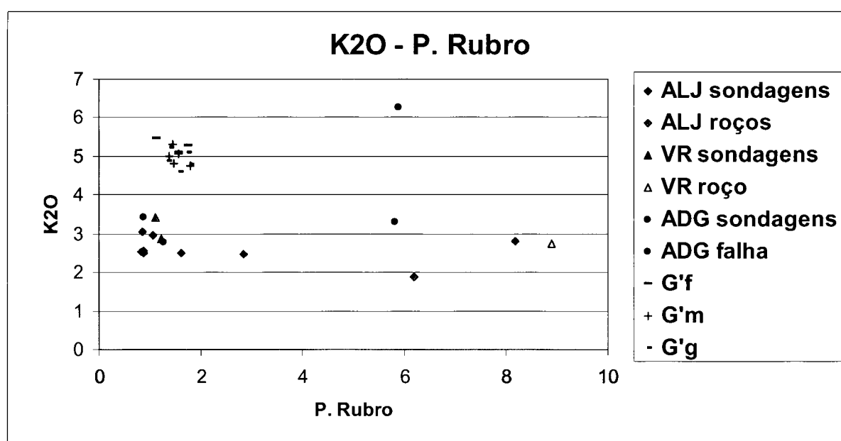
Figura VI.16 - Diagrama de \text{K}_2\text{O} -P. Rubro dos granitos de Cabeceiras de Basto e dos filões estudados, onde não se verifica nenhuma correlação franca pelas razões apontadas no texto.
