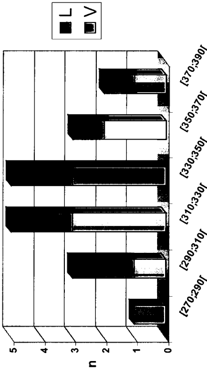
Fig. V.9d – Histograma do n.º de medidas em IF contido em cada classe de temperatura homogeneização global.
