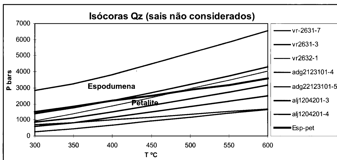
Figura V.22 – Diagrama P-T no qual estão representadas algumas isócoras das IF do quartzo, mas calculadas sem ter em consideração os sais presentes. A linha a negro representa a separação dos campos de estabilidade da espodumena e petalite definidos por London (1984).
