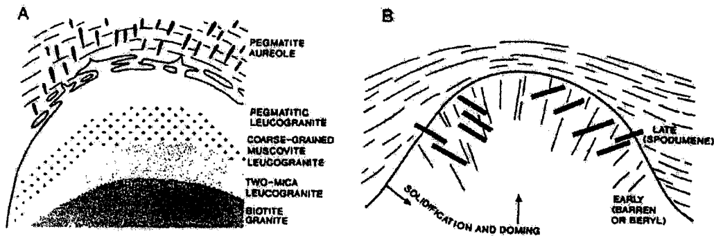
Fig. VII.2 - Ilustração esquemática de dois estilos de consolidação de granitos, acumulação de magmas residuais, e instalação de pegmatitos de elementos raros. A – granitos férteis com uma auréola de pegmatitos exteriores; B – Pegmatitos interiores mas marginais num granito parental fraccionado (retirado de Černý, 1998).
