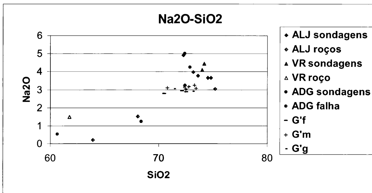
Figura VI.14 - Diagrama de \text{SiO}_2\text{-Na}_2\text{O} com projecção dos granitos de Cabeceiras de Basto e filões estudados, onde se verifica uma certa correlação positiva.
