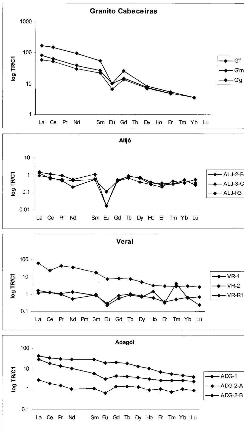
Figura VI.24 – Espectros de terras raras, normalizadas ao condrito C1 (Evensen et al. (1978), das amostras mais frescas dos granitos de Cabeceiras de Basto (dados de Almeida, 1994) e de cada um dos três filões estudados: ALJ – Alijó; VR – Veral; ADG – Adagói;
