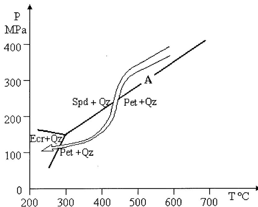
Fig. IV.31 b) - O caminho P-T inferido para a cristalização magmático-hidrotermal dos filões de Veral e Adagói, e consequentemente do sector E. (Spd-espodumena; Pet-petalite; Ecr-eucryptite; Qz-quartzo); A - O campo de estabilidade das fases dos aluminossilicatos de Li (London, 1984);
