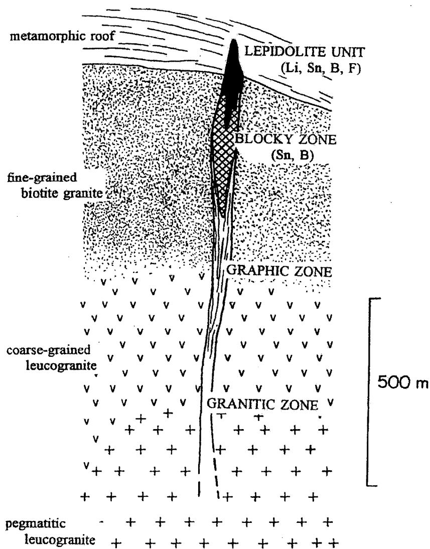
Fig. VII.1 - Ilustração esquemática de um pegmatito com elementos raros com uma zonation vertical, gerada por diferenciação de uma zona interna de um leucogranito. O filão penetra ainda numa camada superior de granitos primitivos metamorfizados (retirado de Černý 1998).
