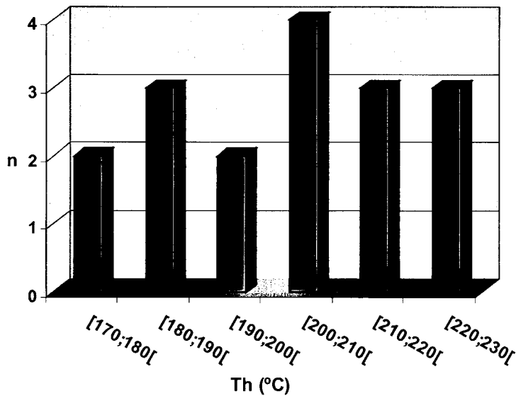
Fig. V.10b – Histograma do n.º de medidas em IF contido em cada classe de homogeneização global.
