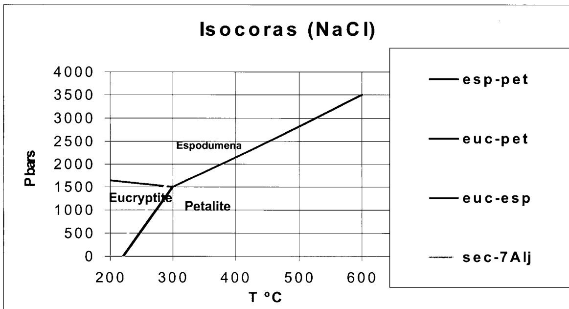
Figura V.25 – Diagrama P-T no qual está representada uma isócora representativadas IF secundárias do quartzo, calculadas tendo em consideração os sais presentes. As outras linhas representam a separação dos campos de estabilidade da espodumena, petalite e eucryptite definidos por London (1984).
