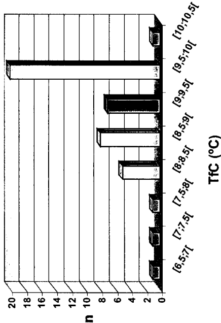
Fig. V.4b – Histograma do n.º de medidas em IF contido em cada classe de temperatura de fusão dos clatratos.
