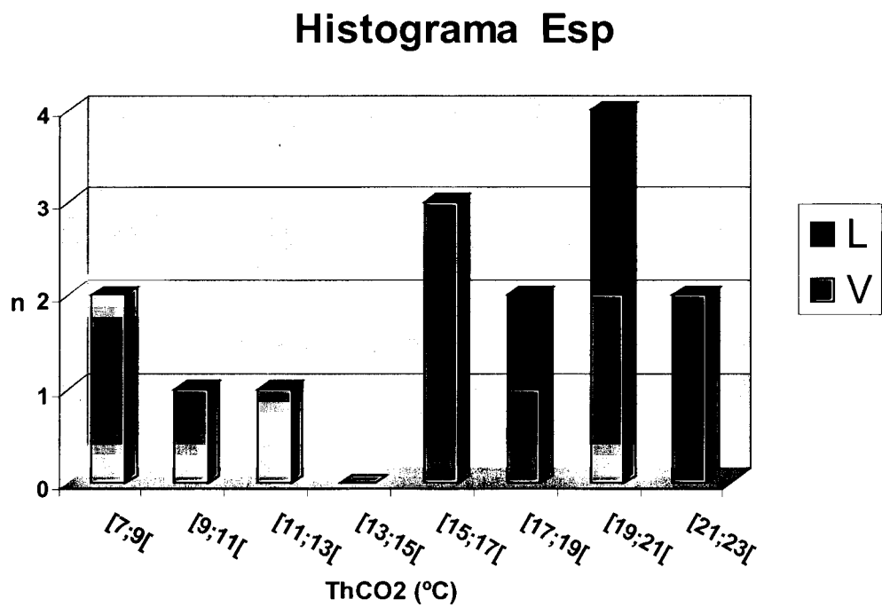
Fig. V.2e – Histograma do n.º de medidas em IF contido em cada classe de temperatura de homogeneização do CO 2 .
