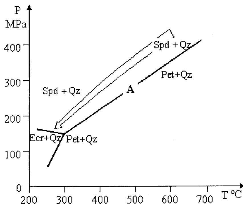
Fig. IV.31 a) – O caminho P-T inferido para a cristalização magmático-hidrotermal do filão de Alijó, e consequentemente do sector W. (Spd-espodumena; Pet-petalite; Ecr-eucryptite; Qz-quartzo); A - O campo de estabilidade das fases dos aluminossilicatos de Li (London, 1984);
