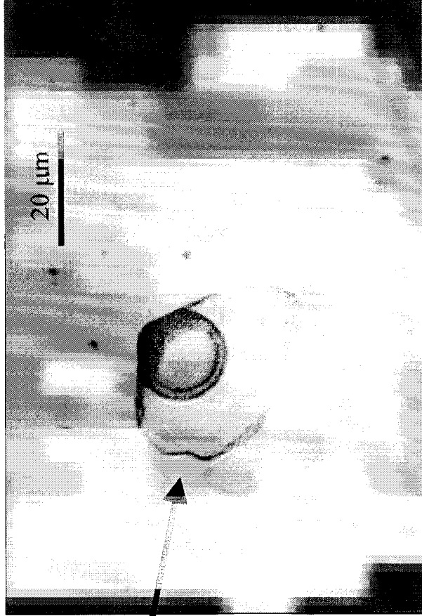
Fig. V.2b – IF onde é visível um sólido (carbonato) formado aquando da incidência do Laser (nicóis paralelos).
