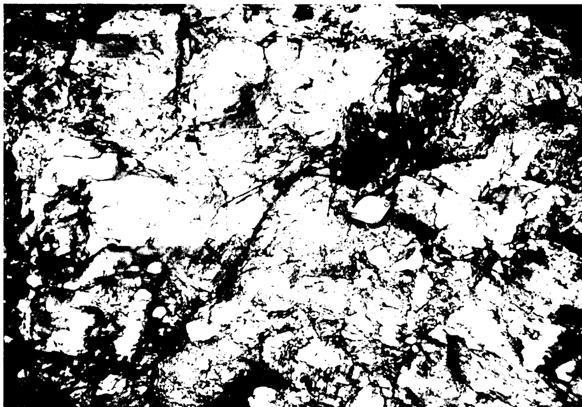
Figura IV.6 – Inclusões de quartzo a preencher fracturas nos cristais de espodumena.
