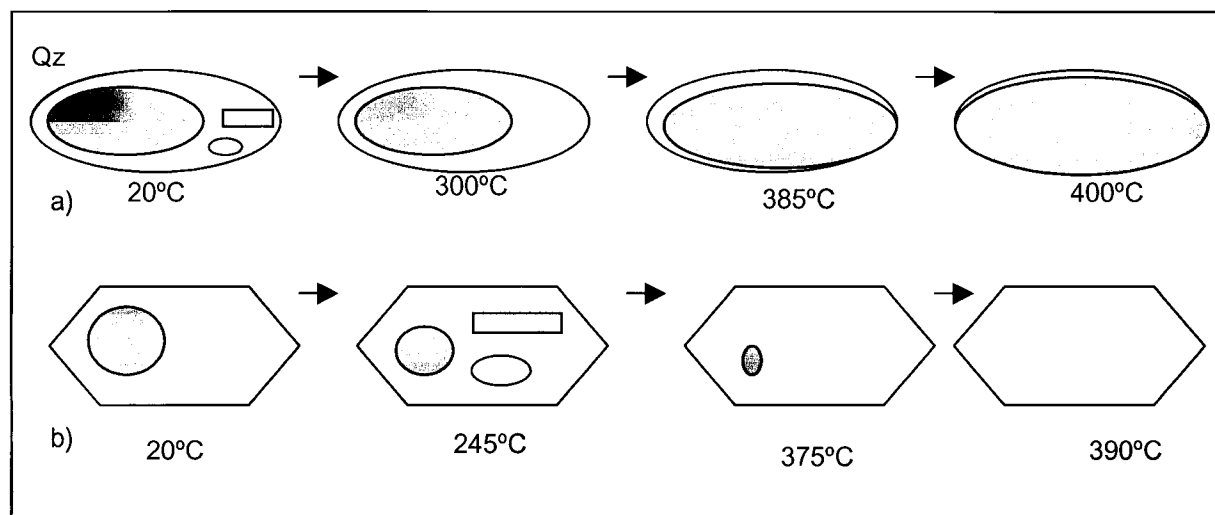
Figura V.5 – Esquema mostrando os diferentes comportamentos das IF no quartzo em relação ao aquecimento, com desaparecimento (caso a) ou a formação e seu desaparecimento antes da homogeneização total (caso b).
