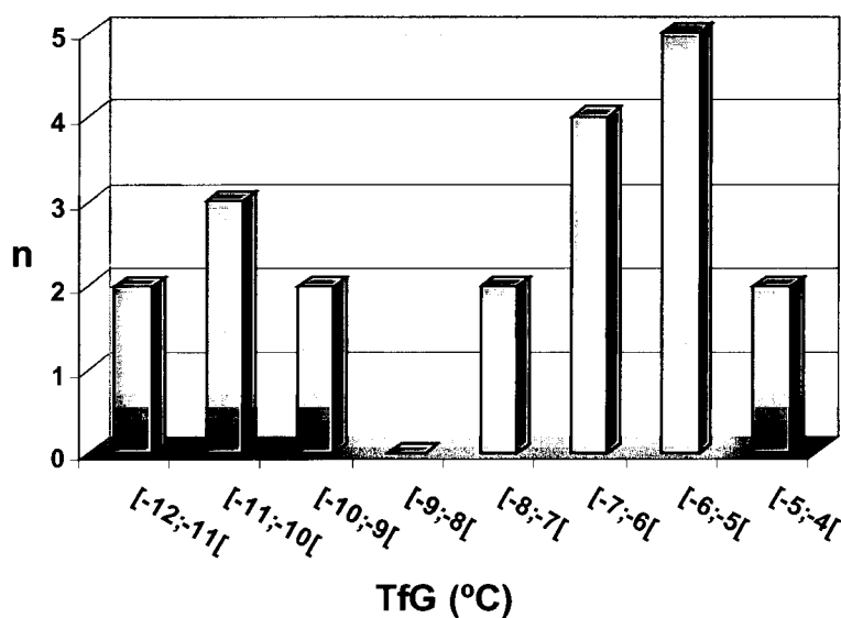
Fig. V.8a – Histograma do n.º de medidas em IF contido em cada classe de temperatura de fusão do gelo.
