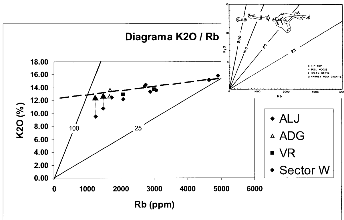
Figura VI.8 – Relação do Rb “versus” K 2 O de Fk de diferentes zonas do campo aplitopegmatítico estudado e, no canto superior direito, gráfico equivalente retirado de Shearer et al., (1985), com os vários dados de cada tipo de filão do campo pegmatítico de Black Hills (South Dakota) .
