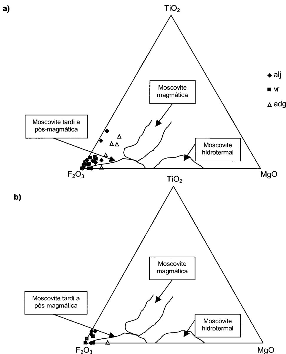
Figura VI.2 – Distribuição das micas brancas primárias (a) e secundárias (b) no diagrama \text{TiO}_2\text{-Fe}_2\text{O}_3\text{-MgO} de Monier et al., (1984). (alj-alijó; vr-veral; adg-adagói)
