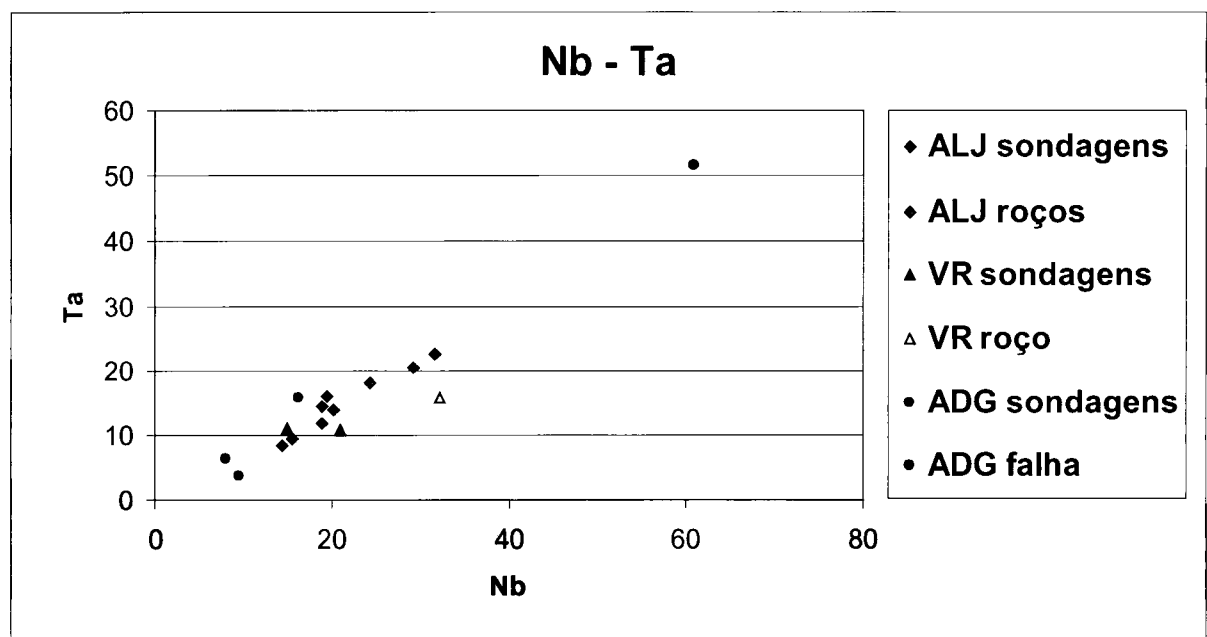
Figura VI.20 - Diagrama de relação Nb-Ta nas amostras dos filões estudados, onde se verifica uma certa correlação positiva.
