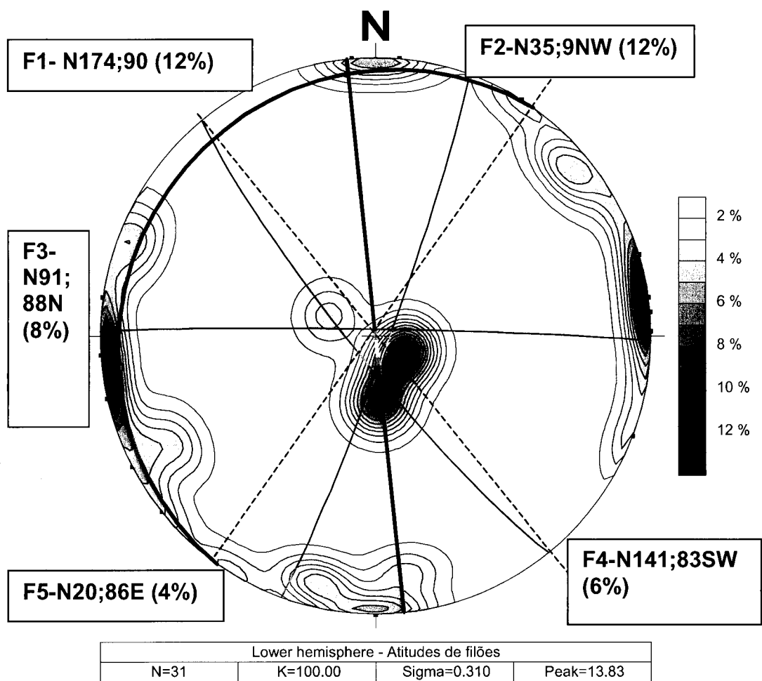
Figura III.6 – Projecção das medições feitas filões espoduménicos do campo estudado, no qual foram definidas 5 famílias principais (n.º de medições = 31)
