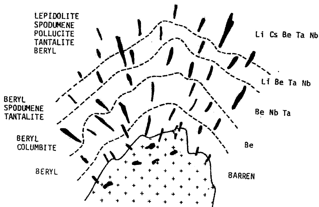
Fig. VII.3 - Representação esquemática de uma zonação regional de um grupo de pegmatitos à volta de um granito parental: fraccionação, enriquecimento de componentes voláteis, complexidade na zonação interna e extensão dos processos em “subsolidus”, que aumentam todos de dentro para fora do granito parental. (retirado de Černý 1998)
