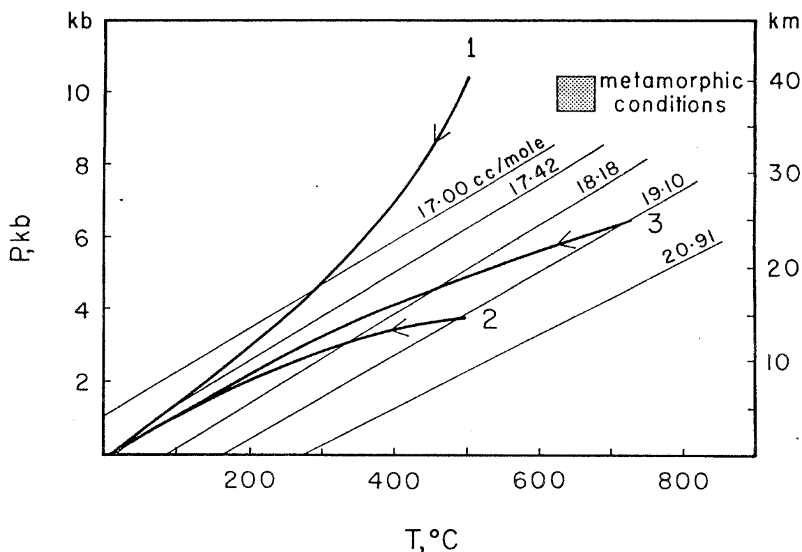
Figura V.26 – Trajectos de "up lift" calculados para os Alpes (Clark & Jager, 1969, curvas 1,2) e para o sul dos Apalaches (Dallmeyer, 1978, curva 3). Razões de "up lift": curva 1=0,74 mm/ano; curva 2=0,47 mm/ano; curva 3=0,1 mm/ano. As isócoras são de fluidos de 25 wt. NaCl. (retirado de Crawford et al., 1979).
