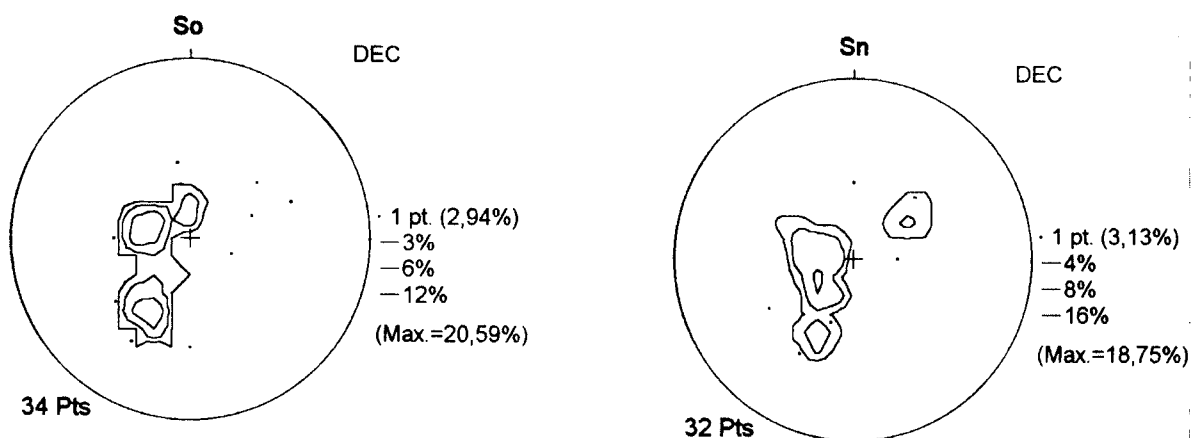
Fig. II.3 – Projecção estereográfica relativa à estratificação S_0 e a estratificação S_2 ( S_n ), nas unidades do DEC (projecção polar, rede de Schmidt) (retirado de Ribeiro, 1998).
