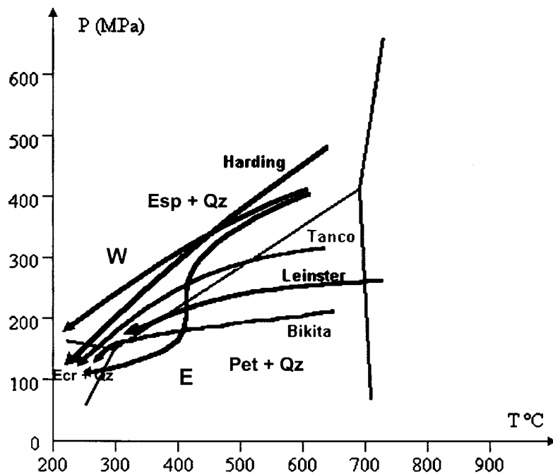
Fig. VII.5 - O caminho P-T inferido para a cristalização magmático-hidrotermal dos sectores E e W, comparados com pegmatitos estudados em todo o mundo. (Esp-espodumena; Pet-petalite; Ecr-eucryptite; Qz-quartzo); A - O campo de estabilidade das fases dos aluminossilicatos de Li (London, 1984);
