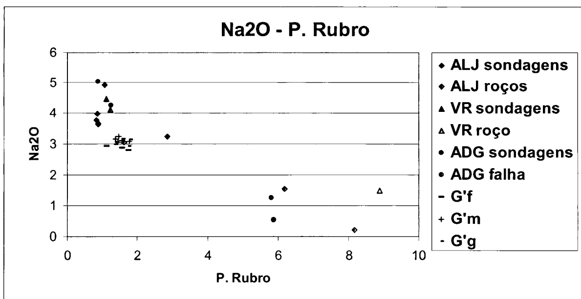
Figura VI.15 - Diagrama de \text{Na}_2\text{O-P} . Rubro dos granitos de Cabeceiras de Basto e dos filões estudados, onde se verifica uma certa correlação negativa.
