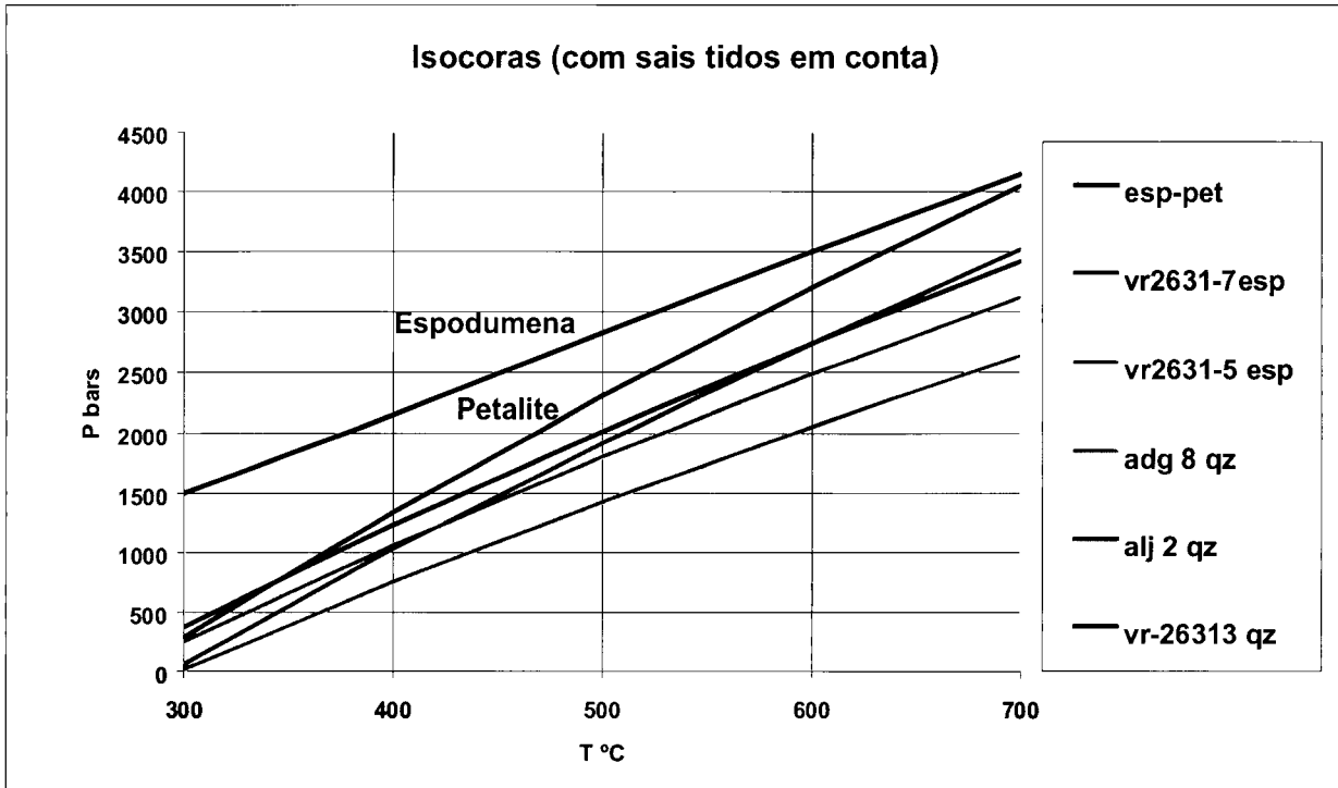
Figura V.24 – Diagrama P-T no qual estão representadas algumas isócoras das IF do quartzo, mas calculadas tendo em consideração os sais presentes. A linha a negro representa a separação dos campos de estabilidade da espodumena e petalite definidos por London (1984).
