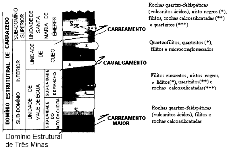
Fig. II.2 – Coluna litoestratigráfica das unidades individualizadas no DEC (retirado de Ribeiro 1998)
