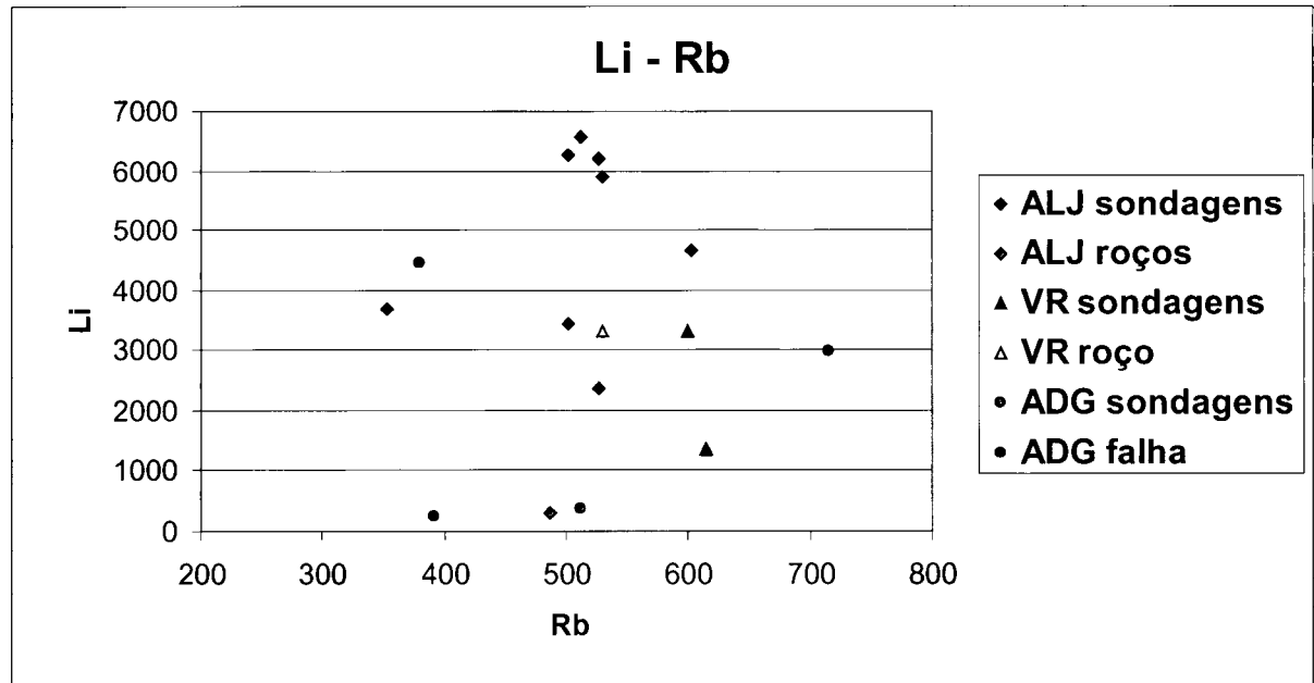
Figura VI.21 - Diagrama de relação Li-Rb nas amostras dos filões estudados, onde não se verifica qualquer tipo de correlação, ao contrário do que acontece nos filões de outros campos, onde a fase litinífera é a lepidolite.
