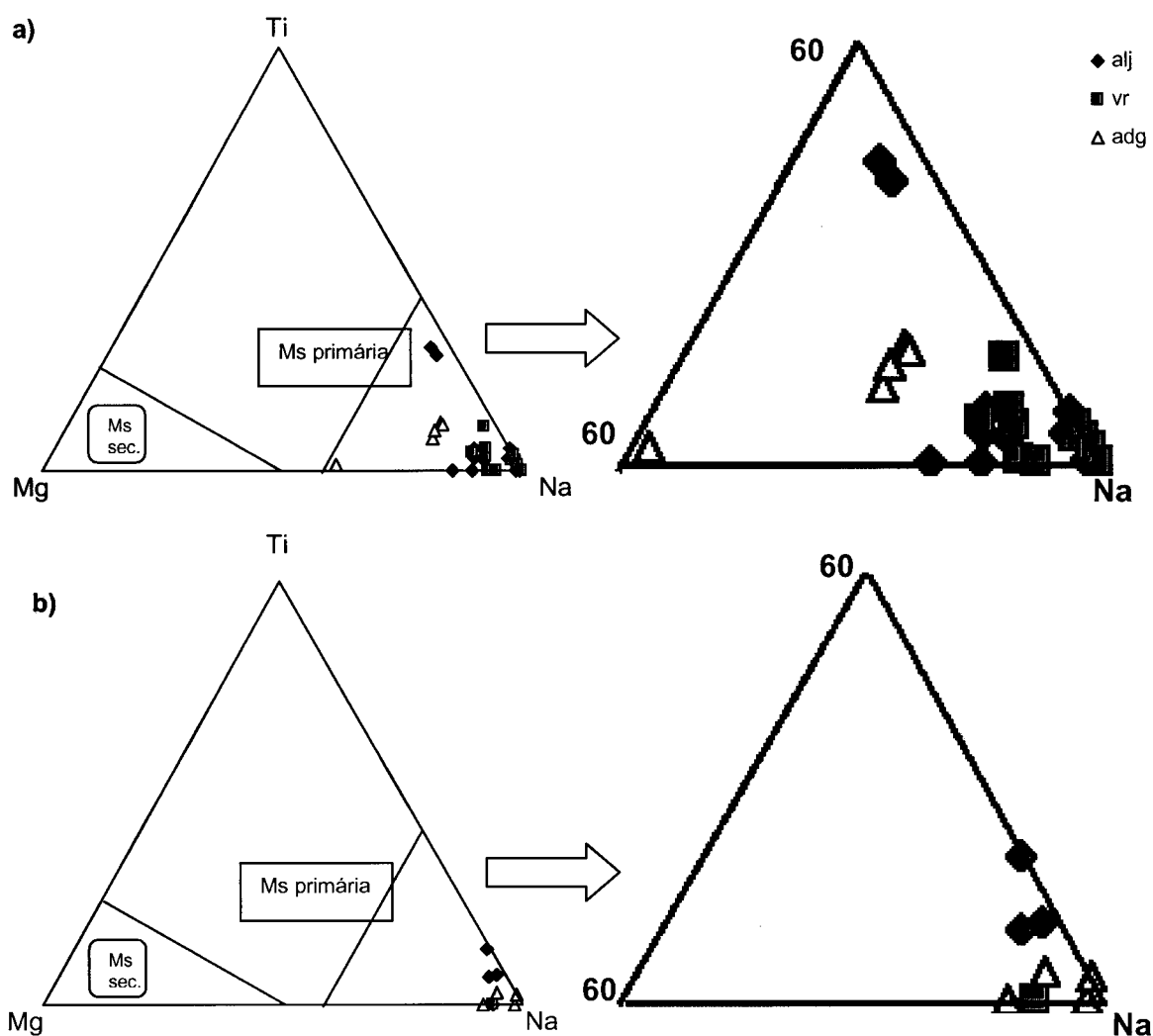
Figura VI.1 – Distribuição das micas brancas primárias (a) e secundárias (b) no diagrama Ti-Mg-Na de Miller et al., (1981). (alj-alijó; vr-veral; adg-adagói)
