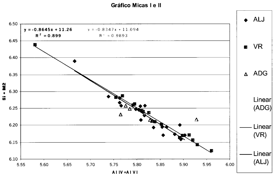
Figura VI.5 – Substituição fengítica das micas brancas dos três filões estudados.
