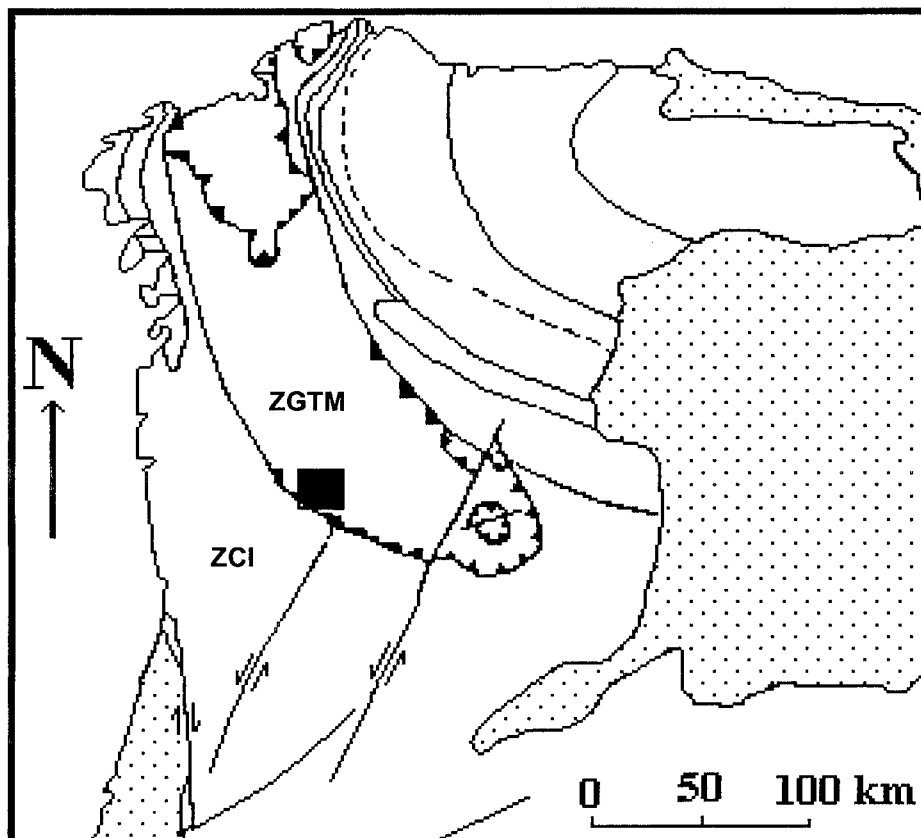
Fig. II.1 – Localização geotectónica da região do Barroso-Alvão (ZGTM - Zona Galiza Trás-os-Montes; ZCI - Zona Centro-Ibérica, Julivert et al., 1974).
