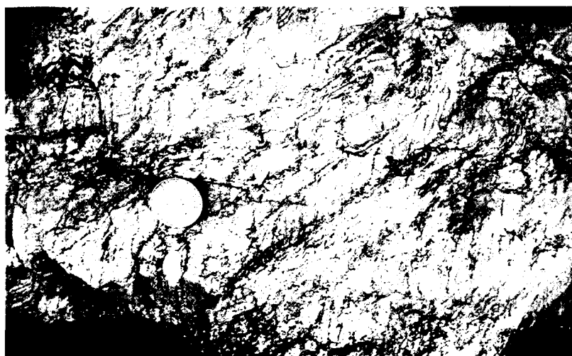
Fig. II.4 – a) Rochas quartzofeldspáticas onde facilmente se identifica “microlithons” e em que é observada a preservação da foliação S_1 no interior de estruturas S_2 .
