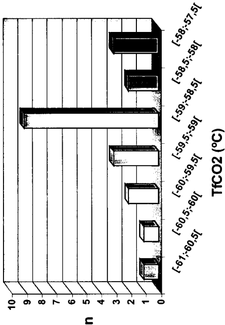
Fig. V.7a – Histograma do n.º de medidas em IF contido em cada classe de temperatura de fusão do CO 2 .
