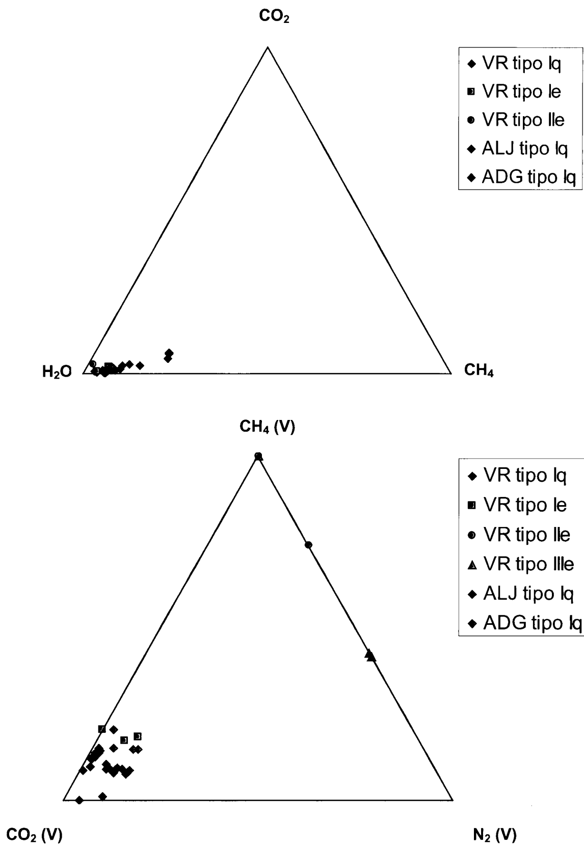
Figura V. 21 – Diagramas ternários a) composição global H 2 O-CO 2 -CH 4 das IF estudadas à microsonda Raman; b) composição da fase volátil CO 2 -CH 4 -N 2 das IF estudadas à microsonda Raman.
