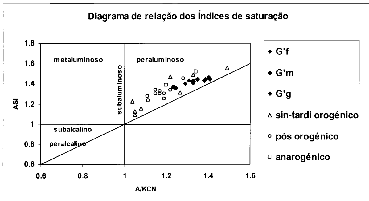
Figura VI.12 – Diagrama relacionando os dois índices de saturação em alumínio (ASI e A/CNK) enquadrando os granitos de Cabeceiras de Basto nos granitos férteis da família LCT (modificado de Černý, 1994b com dados de Almeida, 1994).
