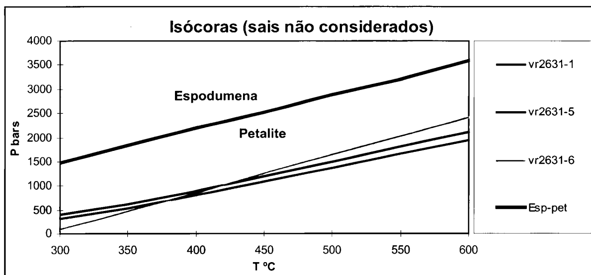
Figura V.23 – Diagrama P-T no qual estão representadas algumas isócoras das IF da espodumena, mas calculadas sem ter em consideração os sais presentes. A linha a negro representa a separação dos campos de estabilidade da espodumena e petalite definidos por London (1984).
