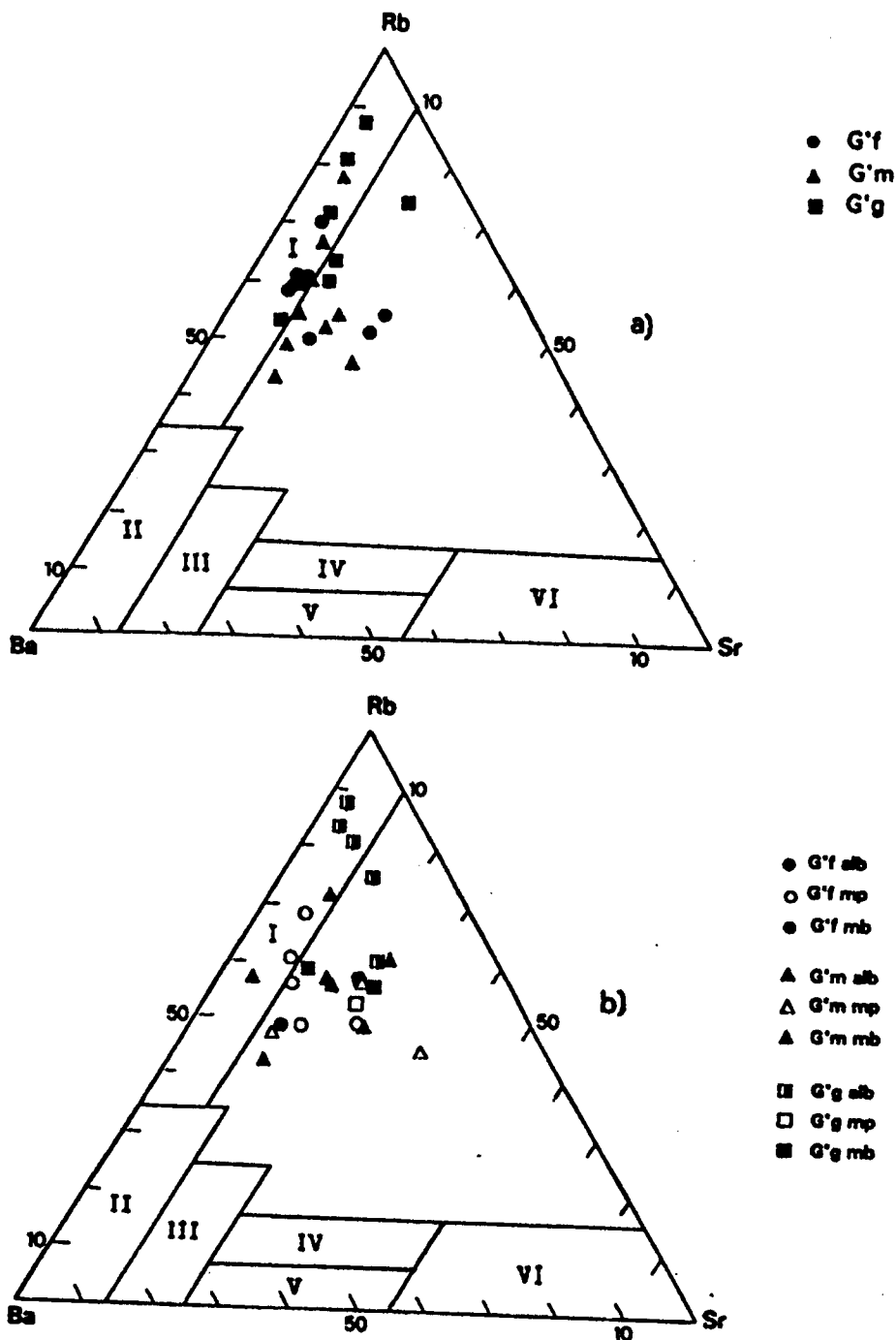
Figura VI.22 – Projecção de amostras sãs (a) e alteradas (b) do complexo granítico de Cabeceiras de Basto no diagrama Ba-Rb-Sr de El Bouseily & El Sokkary (1975). I – granitos fortemente diferenciados; II – granitos normais; III – granitos anómalos; VI – granodioritos; V – quartzodioritos; VI – dioritos.
