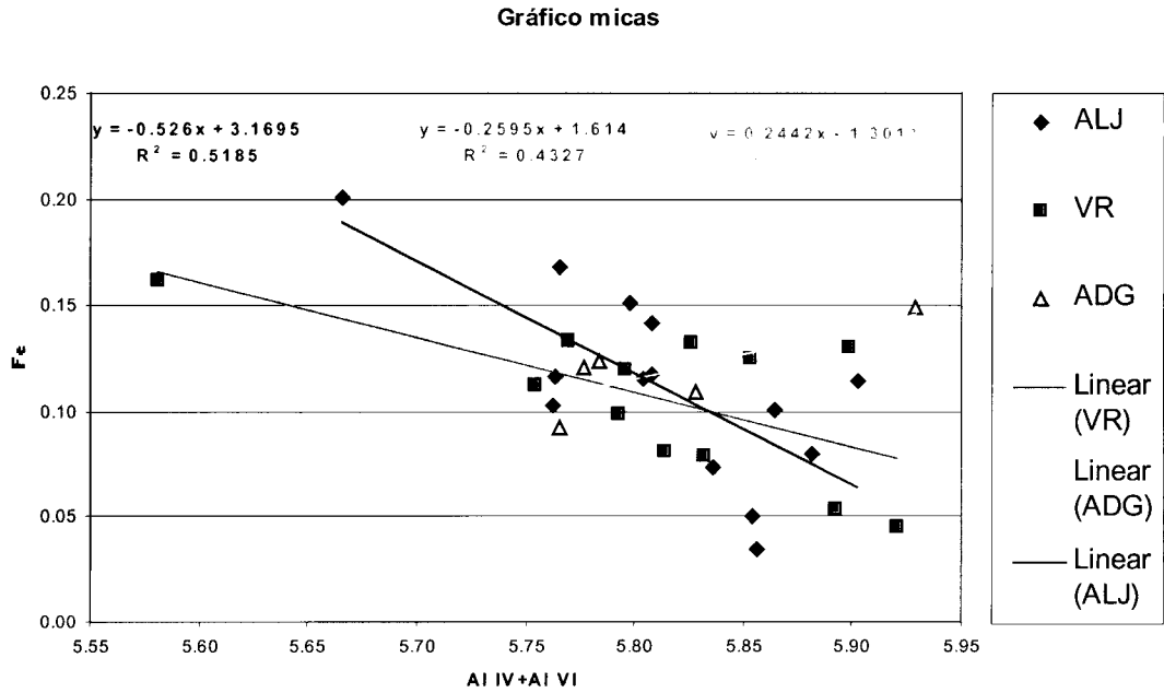
Figura VI.6 – Correlação entre o Al total e o Fe nas micas brancas dos três filões estudados.
