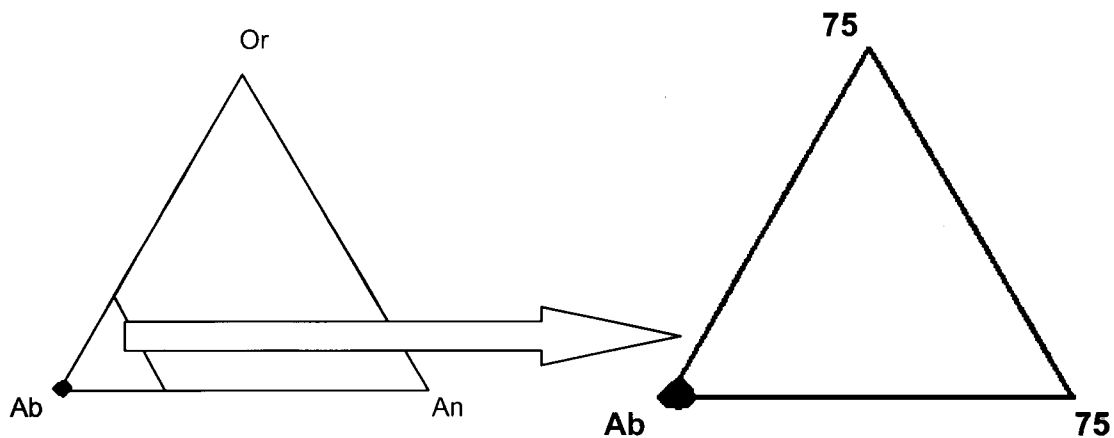
Figura VI.11 – Localização da composição da plagioclase dos filões aplitopegmatíticos em estudo no diagrama Or-Ab-An.
