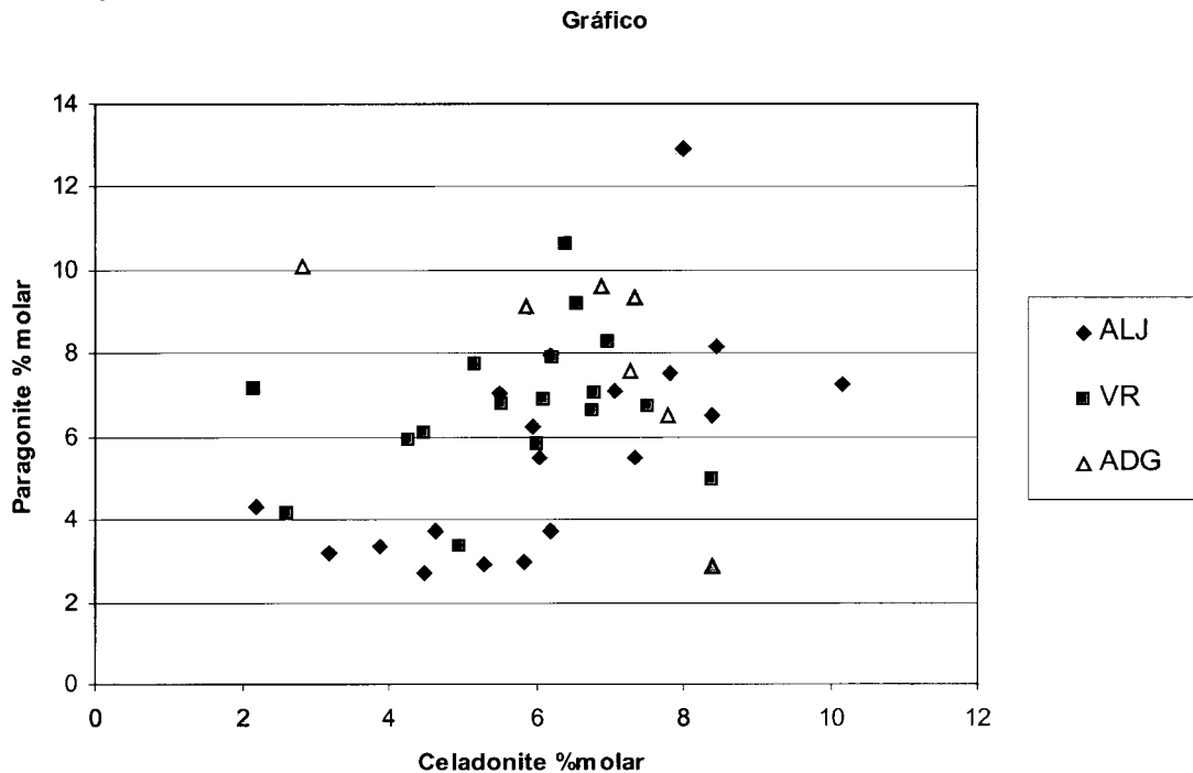
Figura VI.7 – Contribuição das moléculas de celadonite e paragonite na estrutura das moscovites primárias e secundárias dos três filões em estudo.
