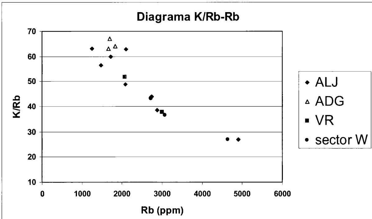
Figura VI.9 – Relação da composição em Rb relativamente à razão K/Rb em feldspatos de diferentes zonas do campo aplitopegmatítico estudado (Černý et al. (1985).
