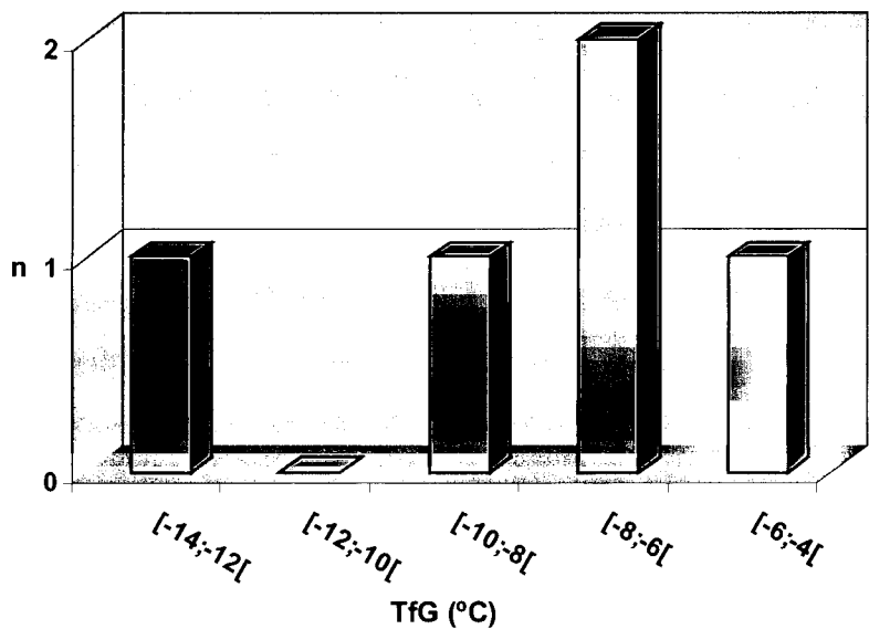
Histograma Tipo III Esp
