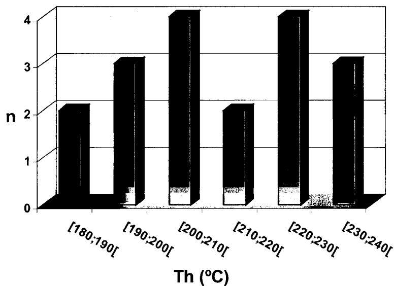
Fig. V.6b – Histograma do n.º de medidas em IF contido em cada classe de homogeneização global.
