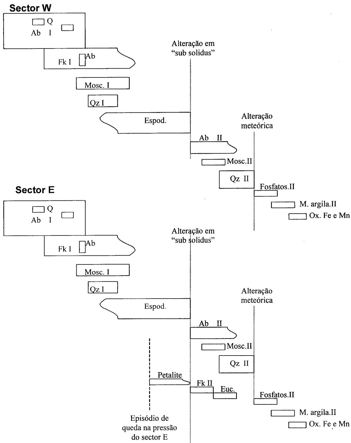
Figura IV.30 - Sequência interpretativa de cristalização. A altura de cristalização do crescimento da eucryptite não pode ser localizado no tempo com certeza, mas parece mais ou menos contemporâneo com o Fk túrbido e secundário. A montebrasite é demasiada rarefeita para ser posta na sequência mas supostamente é magmática tardia.
