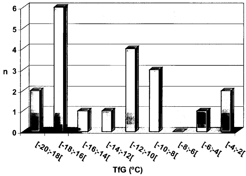
Fig. V.10a – Histograma do n.º de medidas em IF contido em cada classe de temperatura de fusão do gelo.
