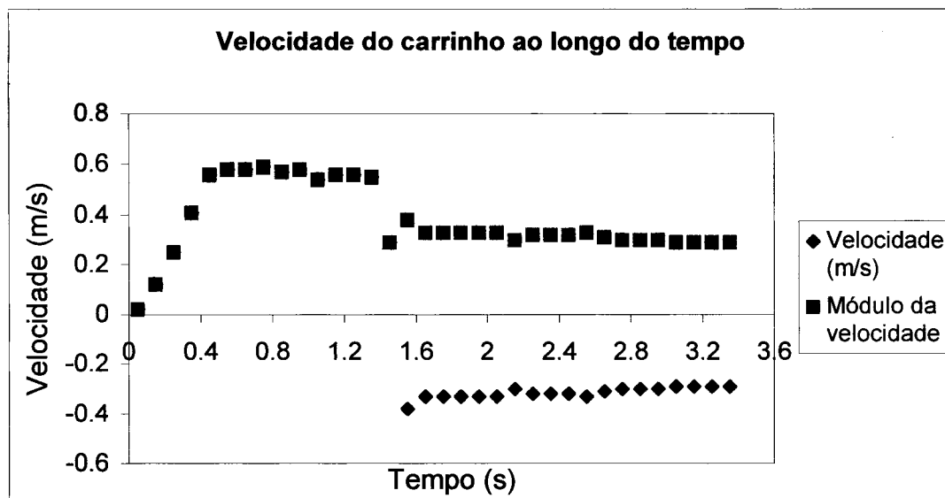
Gráfico 4.4 Velocidade e módulo da velocidade do sistema durante o seu movimento.
