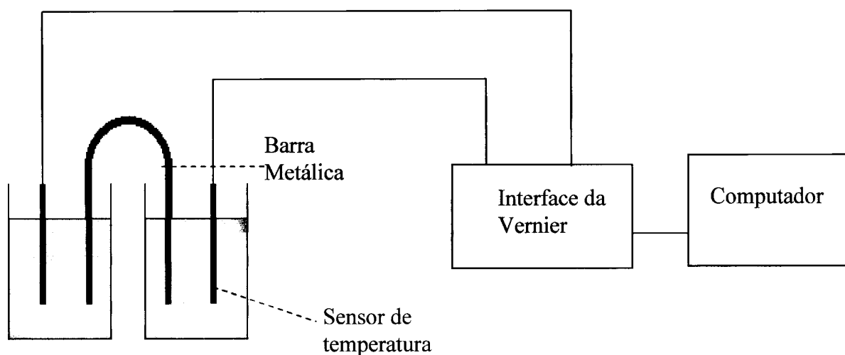
Figura 3.2 Esquema da montagem final usada.
