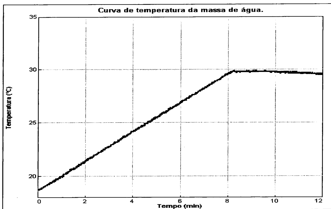
Gráfico 2.3 Aquecimento da água sem corante durante 8 minutos.
