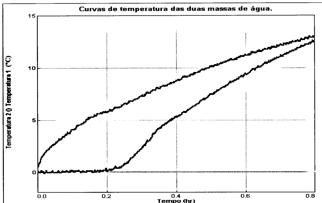
Gráfico 2.1 A curva azul corresponde à massa de água líquida e a curva vermelha corresponde à mistura de água e gelo.
