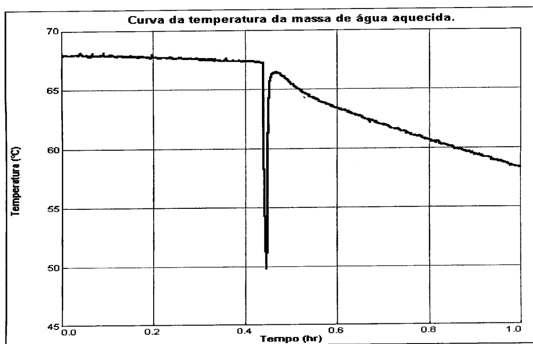
Gráfico 3.4 Variação da temperatura da massa aquecida devido à condução de calor pela barra de cobre antes e após a sua introdução.
