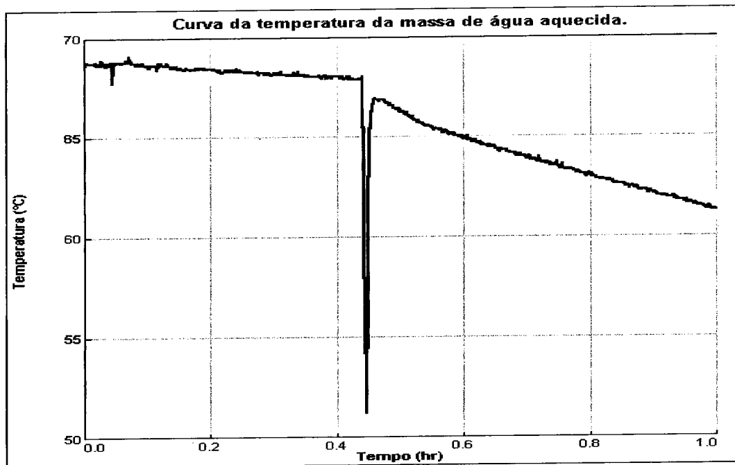
Gráfico 3.5 Variação da temperatura da massa aquecida devido à condução de calor pela barra de alumínio antes e após a sua introdução.
