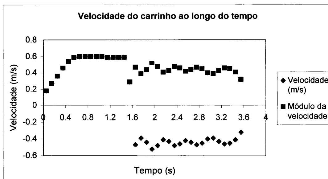
Gráfico 4.2 Velocidade e módulo da velocidade do sistema durante o seu movimento.
