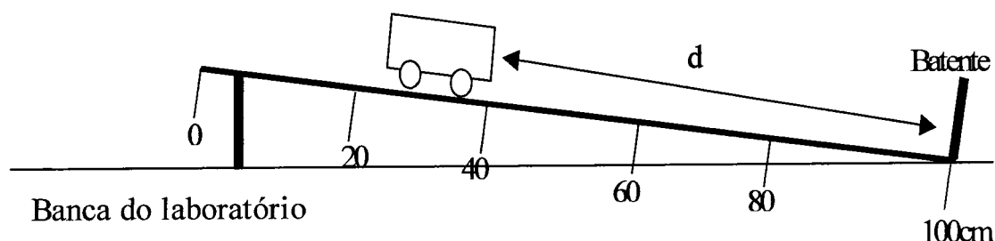
Figura 4.2 O carrinho encontra-se, sobre a calha, na posição onde foi abandonado em todos os ensaios apresentados, a uma distância, d , de 60 cm do batente.
