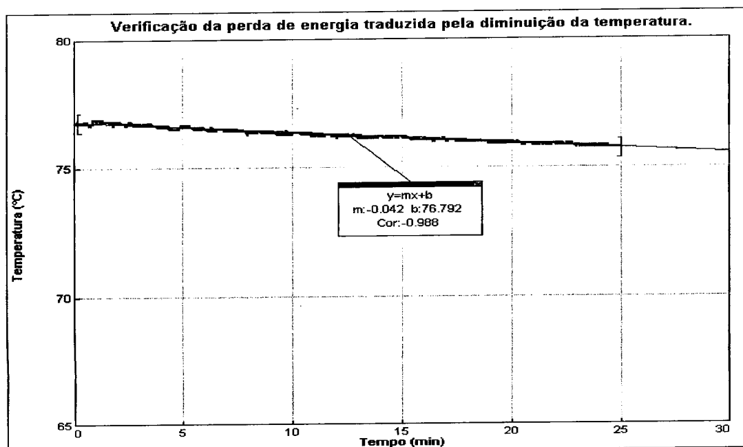
Gráfico 3.6 Declive da recta que traduz a diminuição da temperatura da massa de água.
