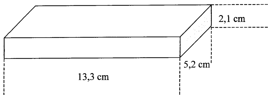
Figura I.1. Dimensões de uma caixa de alumínio para montagem em PASCAR
