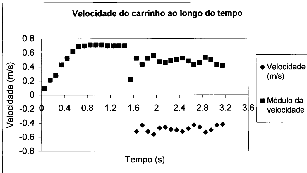
Gráfico 4.3 Velocidade e módulo da velocidade do sistema durante o seu movimento.
