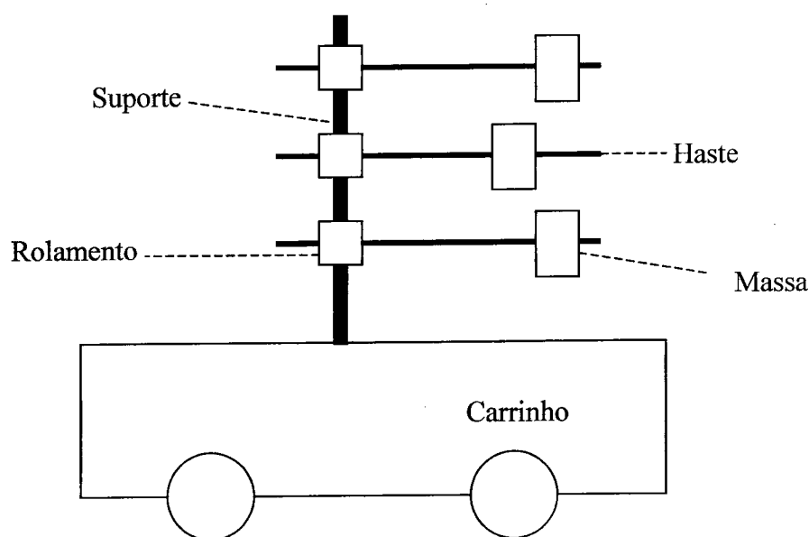
Figura 4.1 Esquema do dispositivo de massas com liberdade de rodarem em torno do suporte.
