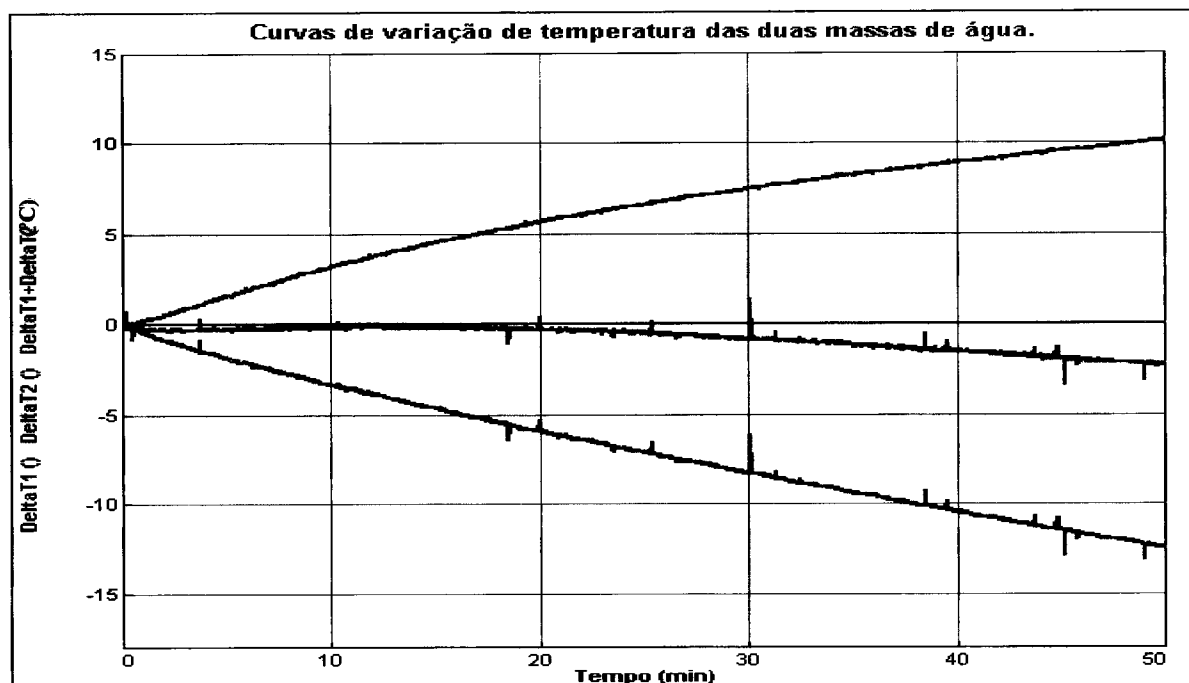
Gráfico 3.3 As curvas azul e vermelha representam as variações de temperatura da cada massa. A curva a verde representa a diferença entre estas variações.
