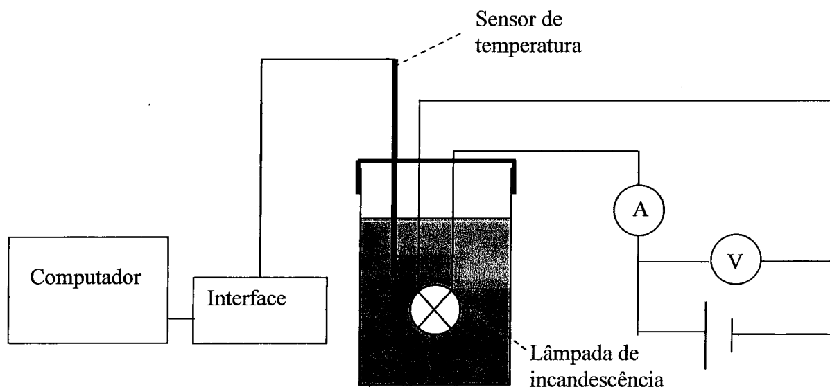
Figura 2.5 Esquema da montagem experimental usada.
