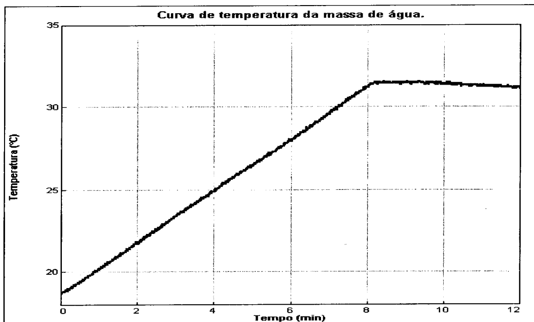
Gráfico 2.4 Aquecimento da água com corante durante 8 minutos.
