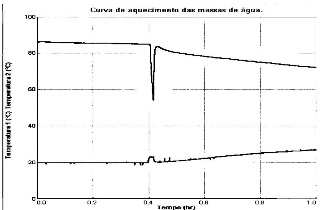
Gráfico 3.1 Variações da temperatura das duas massas antes e após a introdução da barra de cobre.
