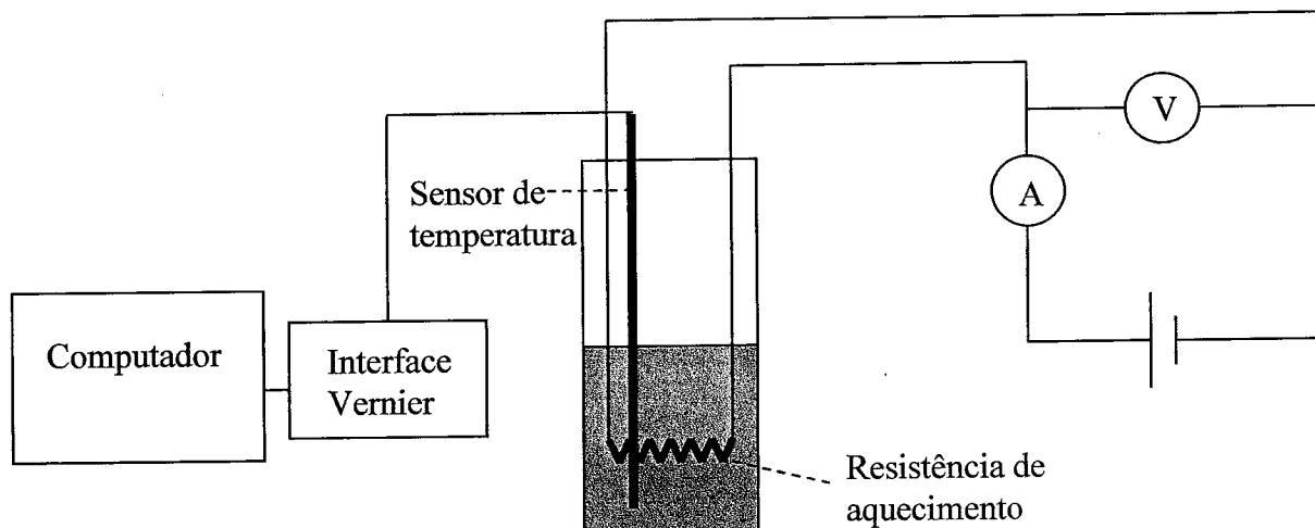
Figura 2.4 Esquema da montagem usada.
