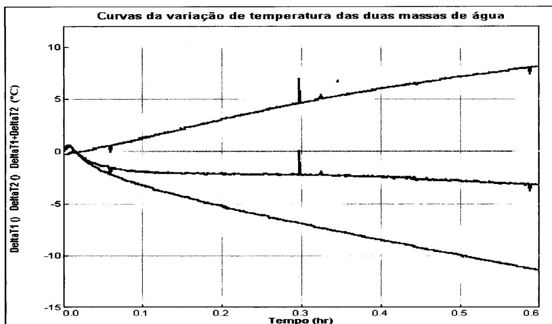
Gráfico 3.2 As curvas azul e vermelha representam as variações de temperatura da cada massa. A curva a verde representa a diferença entre estas variações.
