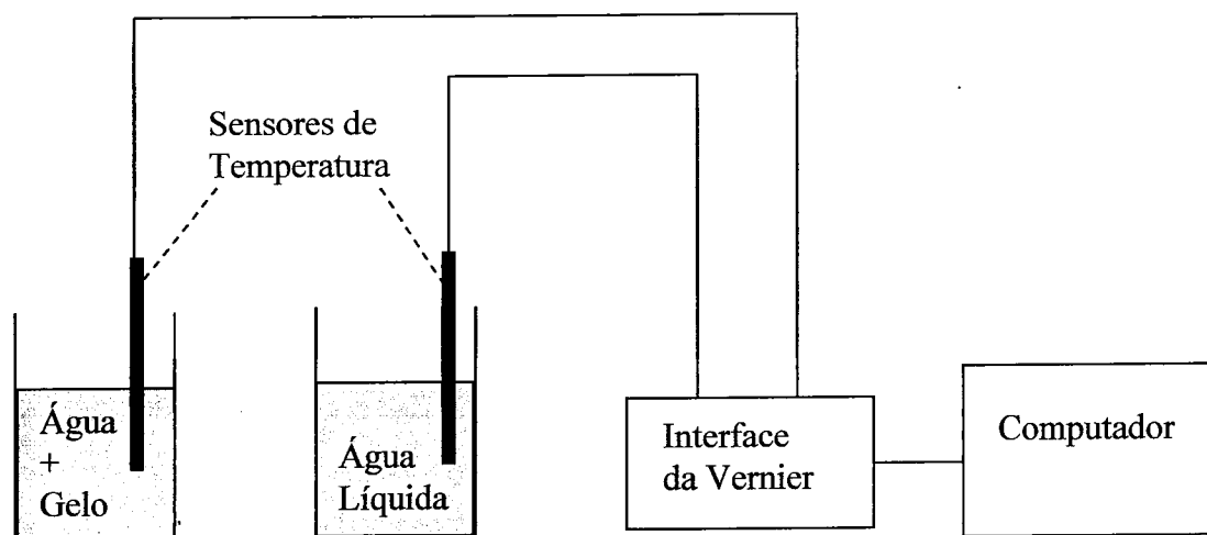
Figura 2.3 Esquema da montagem experimental usada para o aquecimento simultâneo de duas massas de água.
