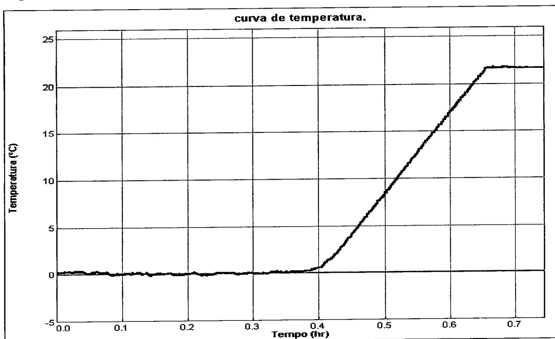
Gráfico 2.2 Variação da temperatura da massa de água ao longo do tempo.
