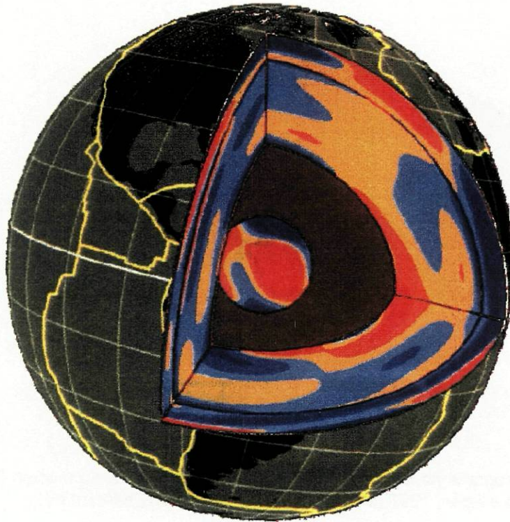
2.36. Modelo 3-D da estrutura interna da Terra, segundo Dziewonski et al. , 2000 (extraído de www.seismology.harvard.edu ).
