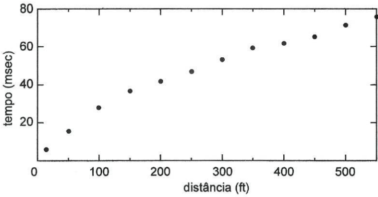
Representação gráfica (•) dos tempo de trajecto ( travel times ) dos 1ºs impulsos de cada sismograma.
