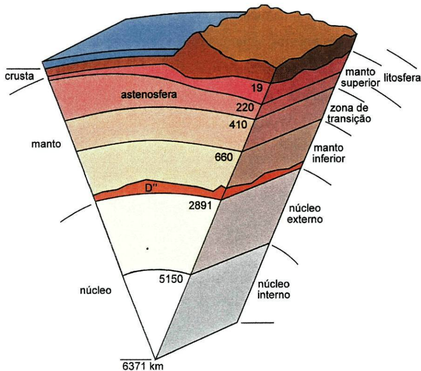
2.37. Esquema gráfico de um modelo teórico da estrutura interna da Terra.
