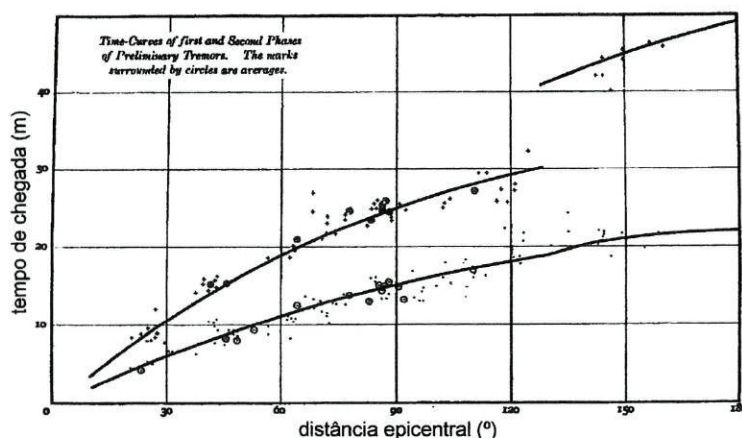
2.26. Curva t-x das ondas P e S elaborada por Oldham, 1906 (extraído de Olroyd, 1996:235).
