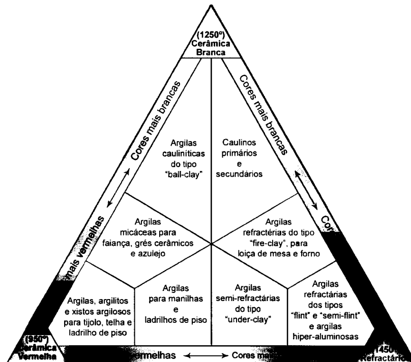
Figura 10.4 – Classificação de materiais cerâmicos com base na cor e na natureza das matérias primas (adaptado de Gomes, 1990).
