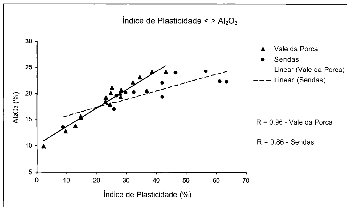
Figura 8.14 – Gráfico de correlação entre o índice de plasticidade e o teor de Al_2O_3 das amostras estudadas.
