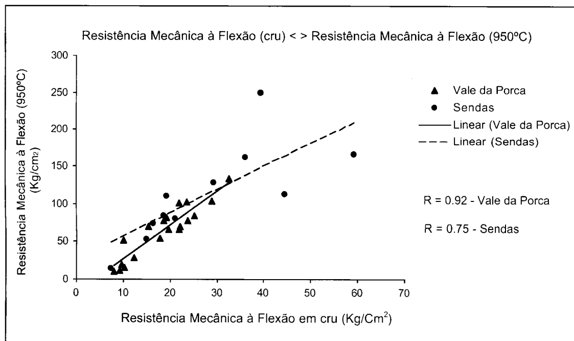
Figura 8.27 – Correlação entre a resistência mecânica à flexão em cru e a resistência mecânica à flexão após cozedura cerâmica a 950°C.
