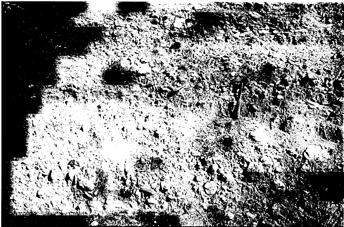
Figura 5.2 – Aspecto das camadas de conglomerado clasto-suportado de matriz areno-lutítica do Membro de Castro da Formação de Bragança, em Caçarelhos, Planalto Mirandês.
