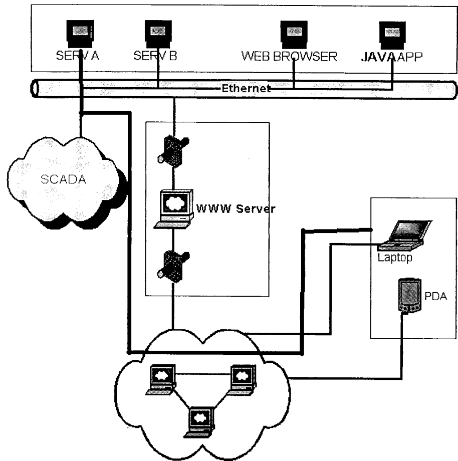
Figura 3.4: Solução Web para o canal — Diagrama de contexto
