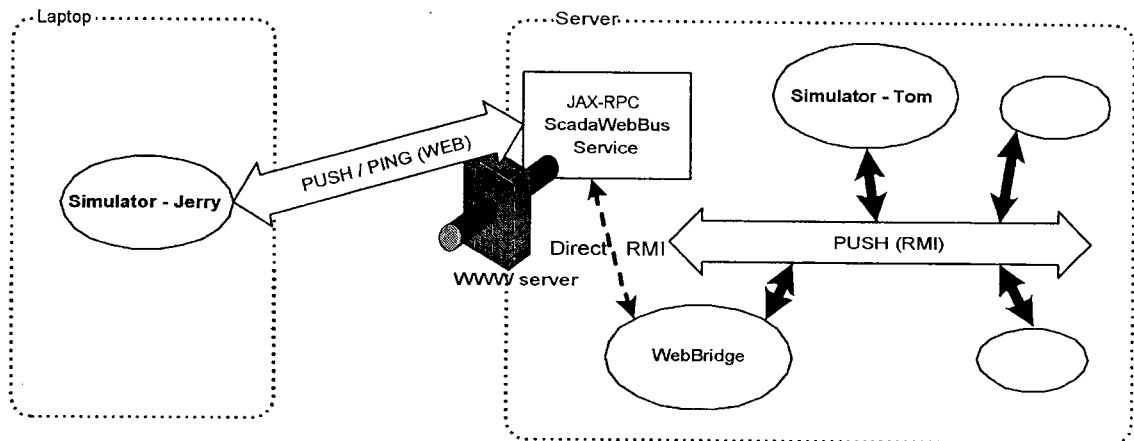
Figura 6.3: Tom & Jerry — Teste WEB
