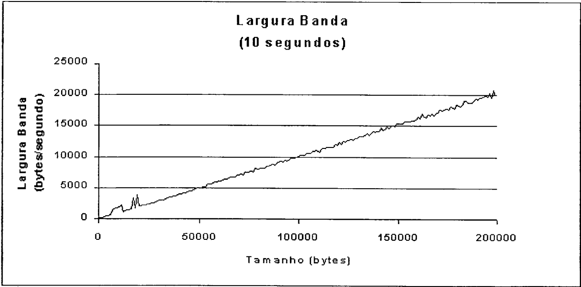
Figura 6.8: Largura de banda — Configuração WEB_10
