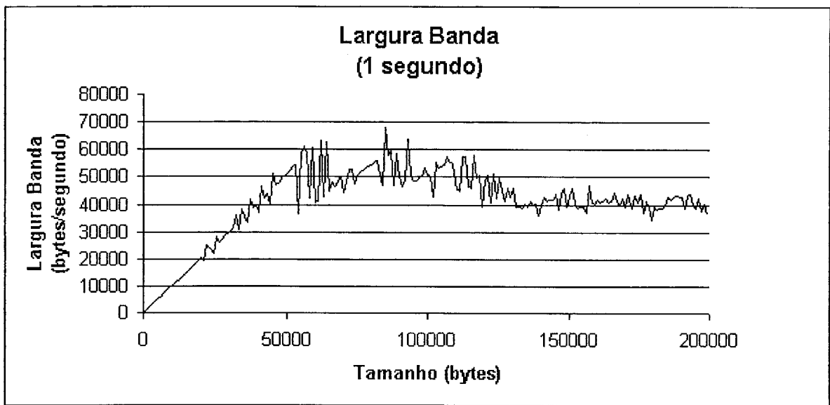
Figura 6.5: Largura de banda — Configuração WEB_1
