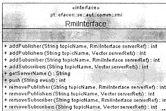
Figura 5.1: Interface RMI básica — PUSH
