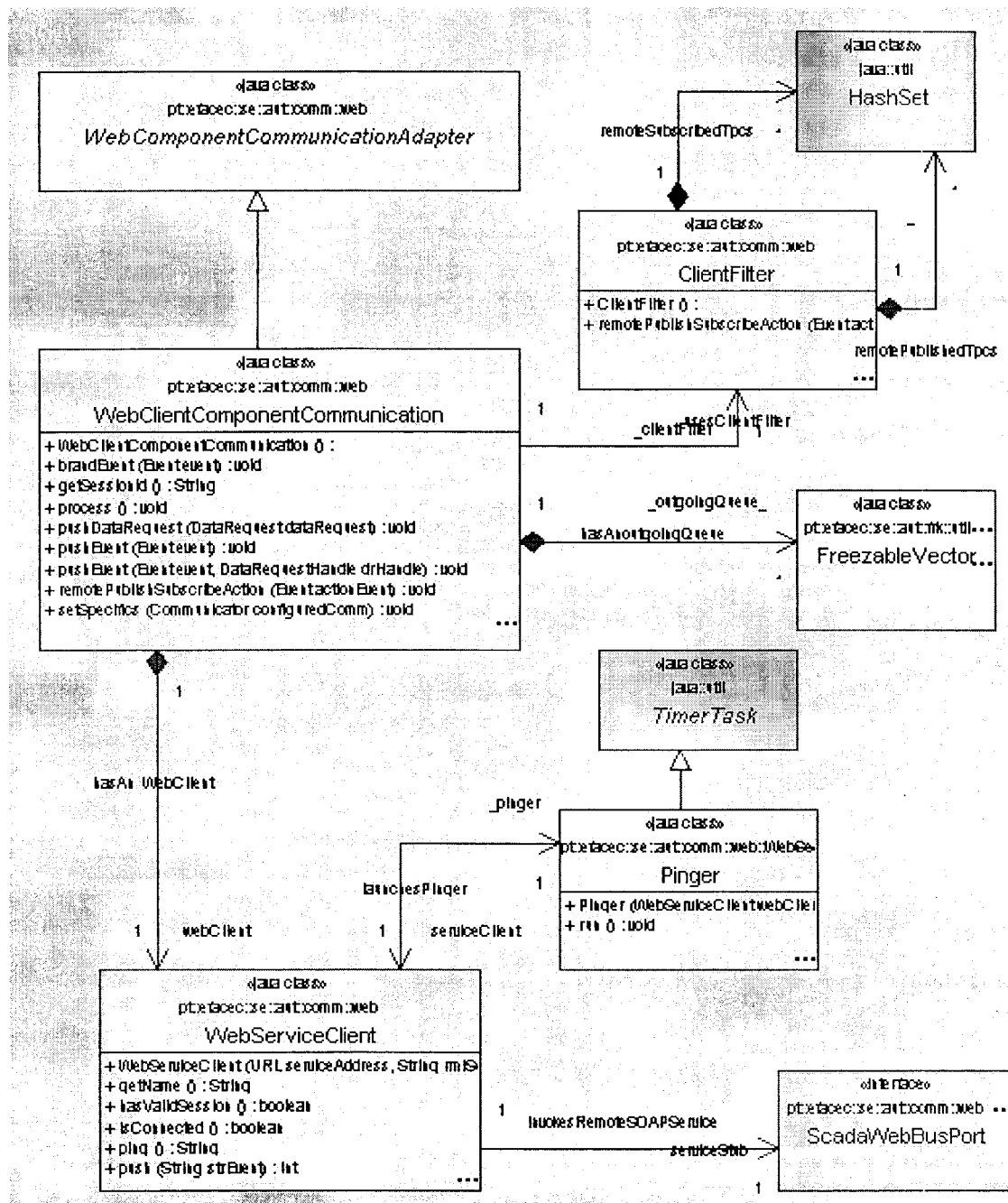
Figura 5.8: Pacote comm — Implementação WEB.client
