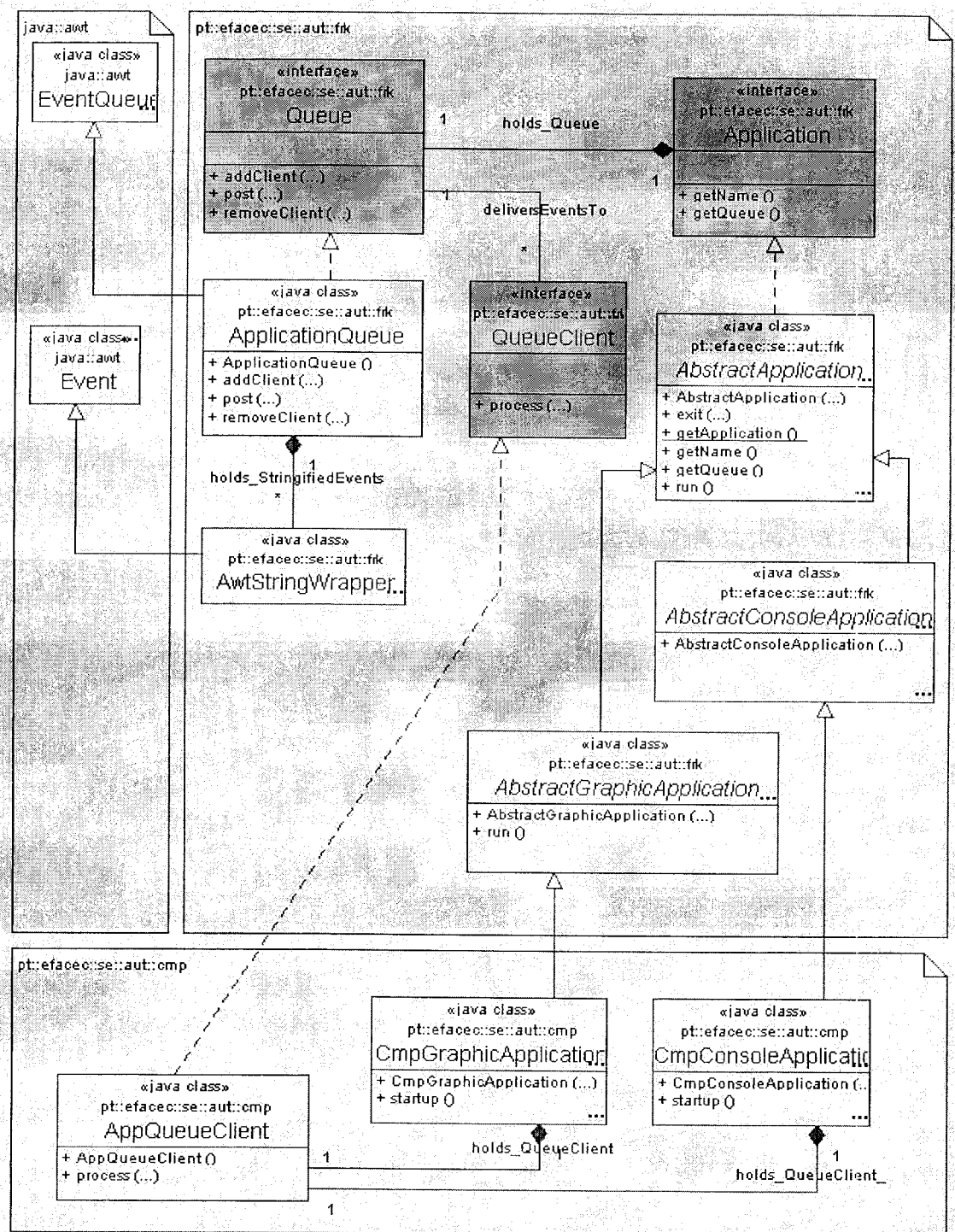
Figura 4.1: Pacote frk — Diagrama de Classes
