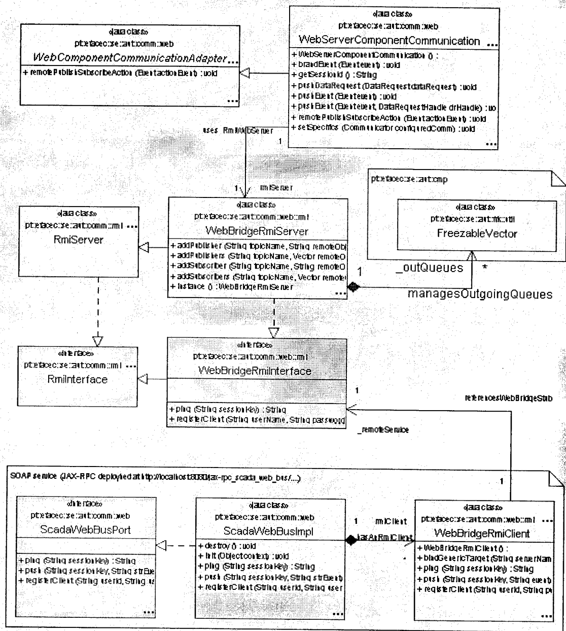
Figura 5.7: Pacote comm — Implementação WEB.server
