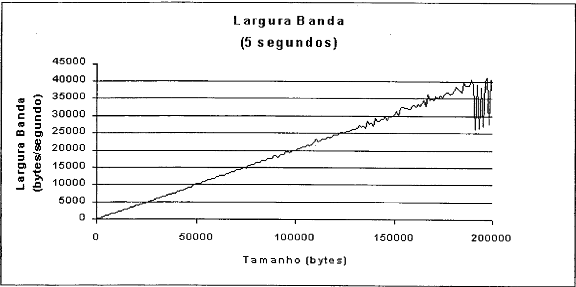
Figura 6.7: Largura de banda — Configuração WEB_5
