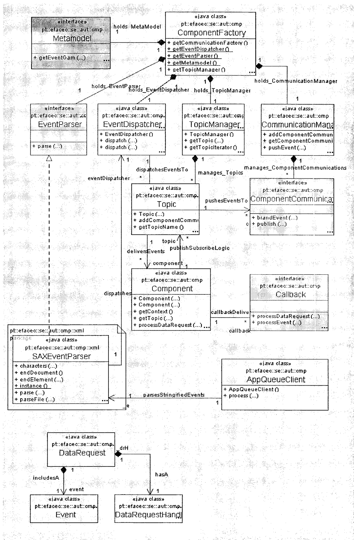
Figura 4.2: Pacote cmp — Diagrama de Classes
