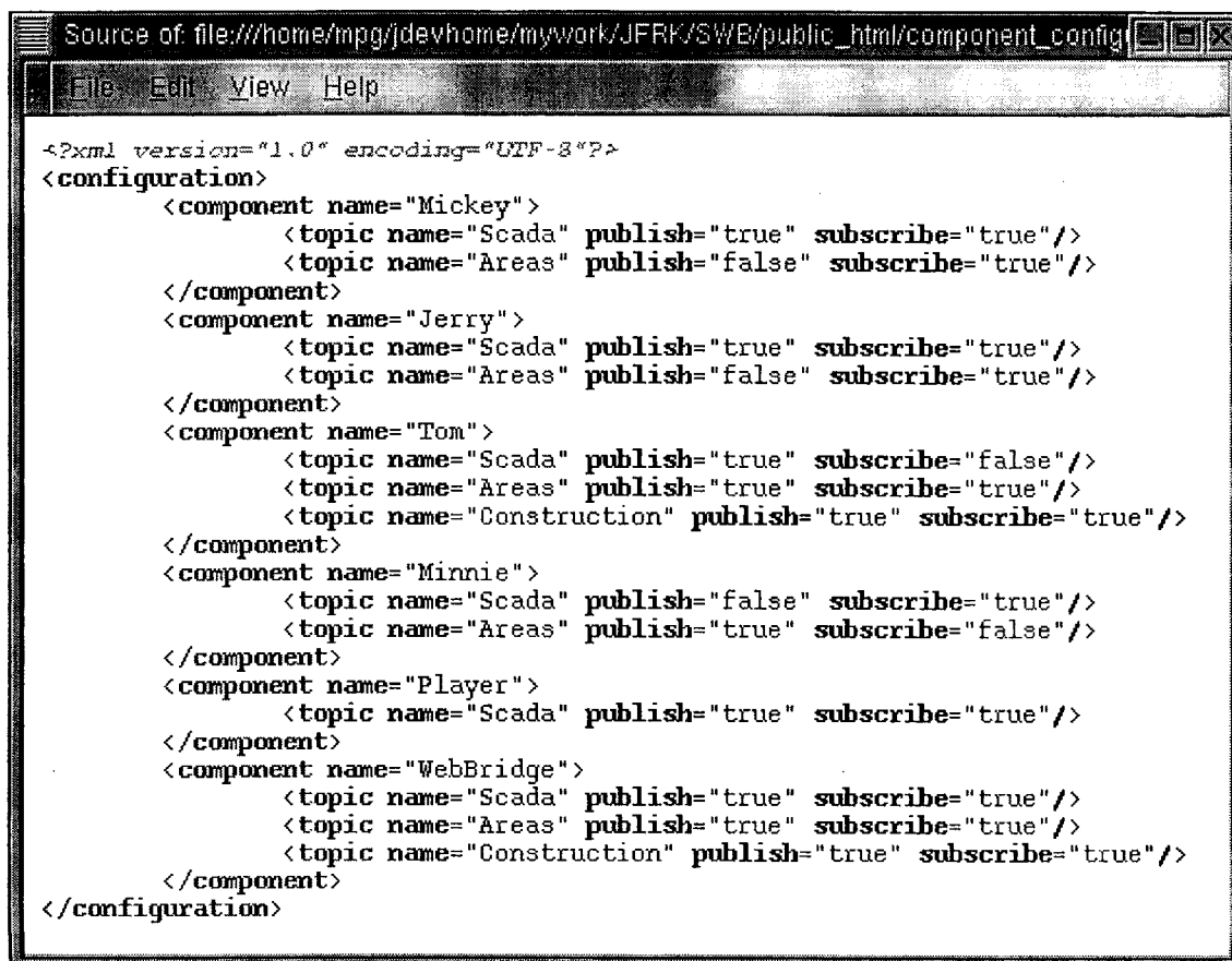
Figura 4.6: Configuração da lógica de publicação e subscrição em XML
