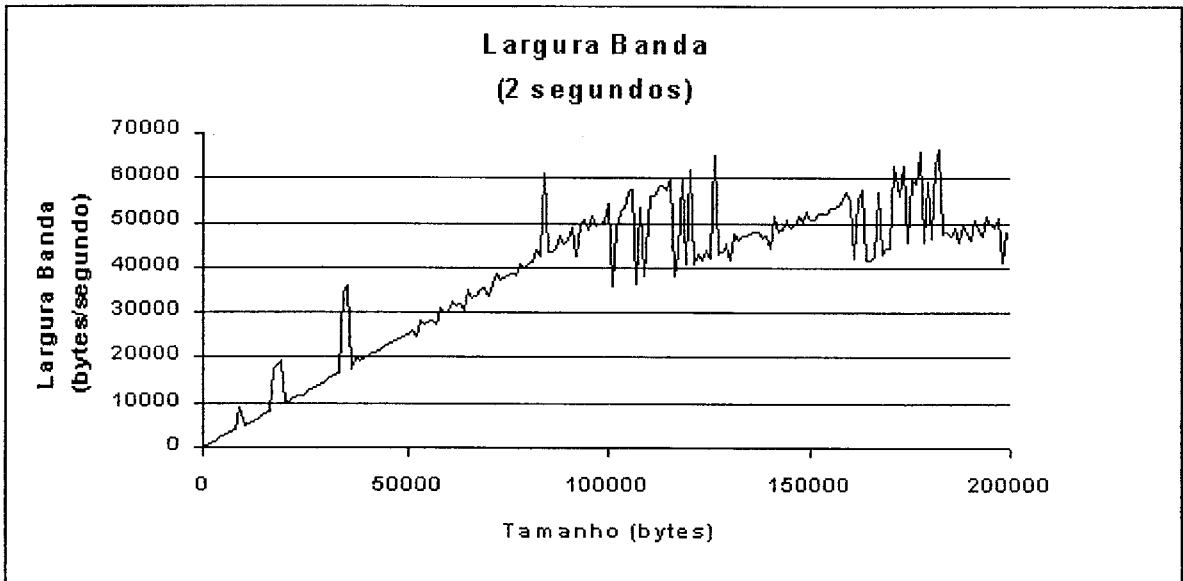
Figura 6.6: Largura de banda — Configuração WEB_2
