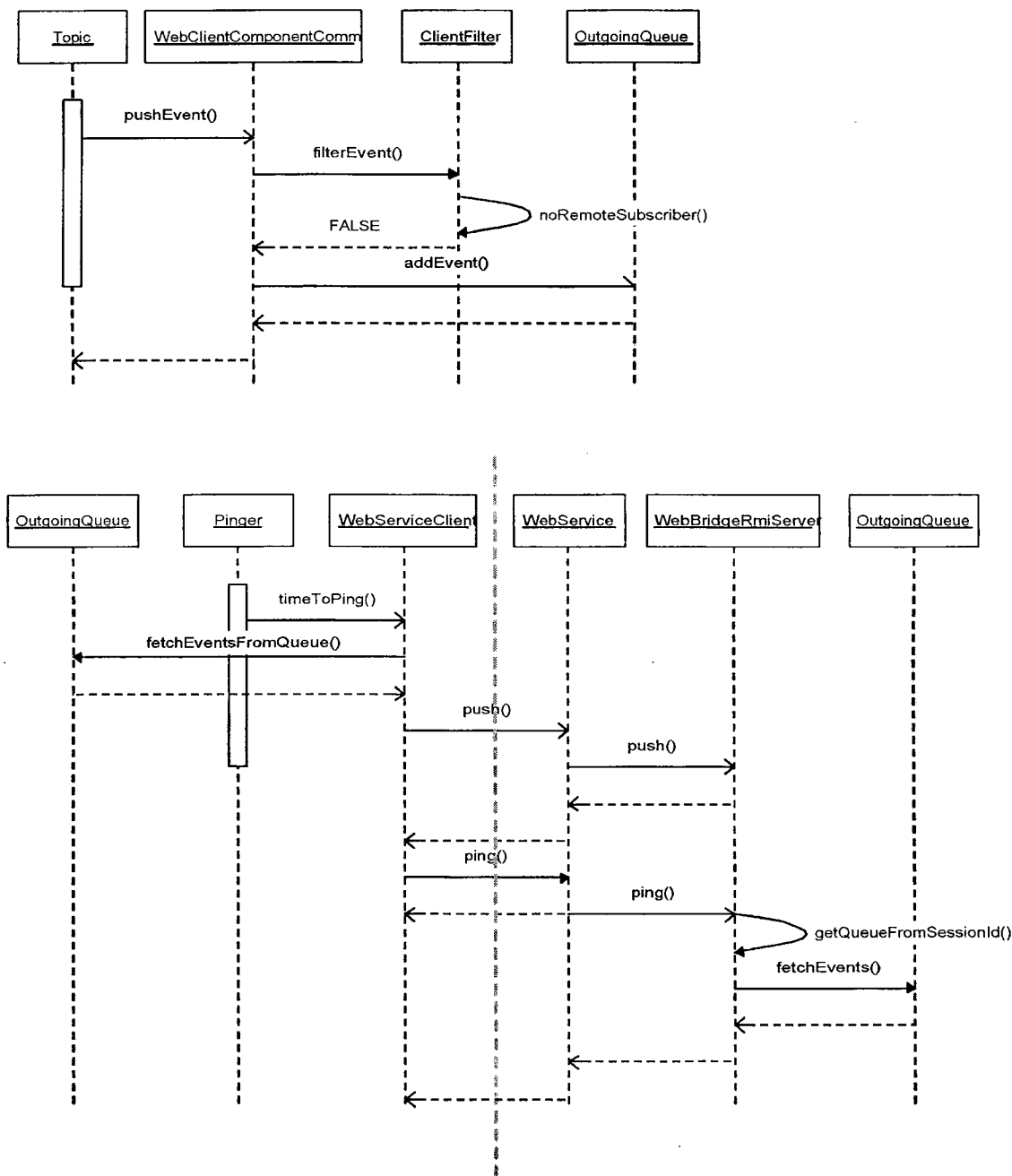
Figura 5.10: Publicação de evento por parte do WEB.client
