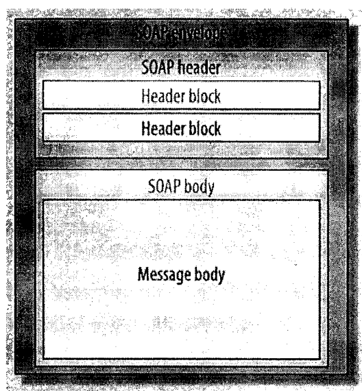
Figura 3.3: A estrutura da mensagem SOAP
