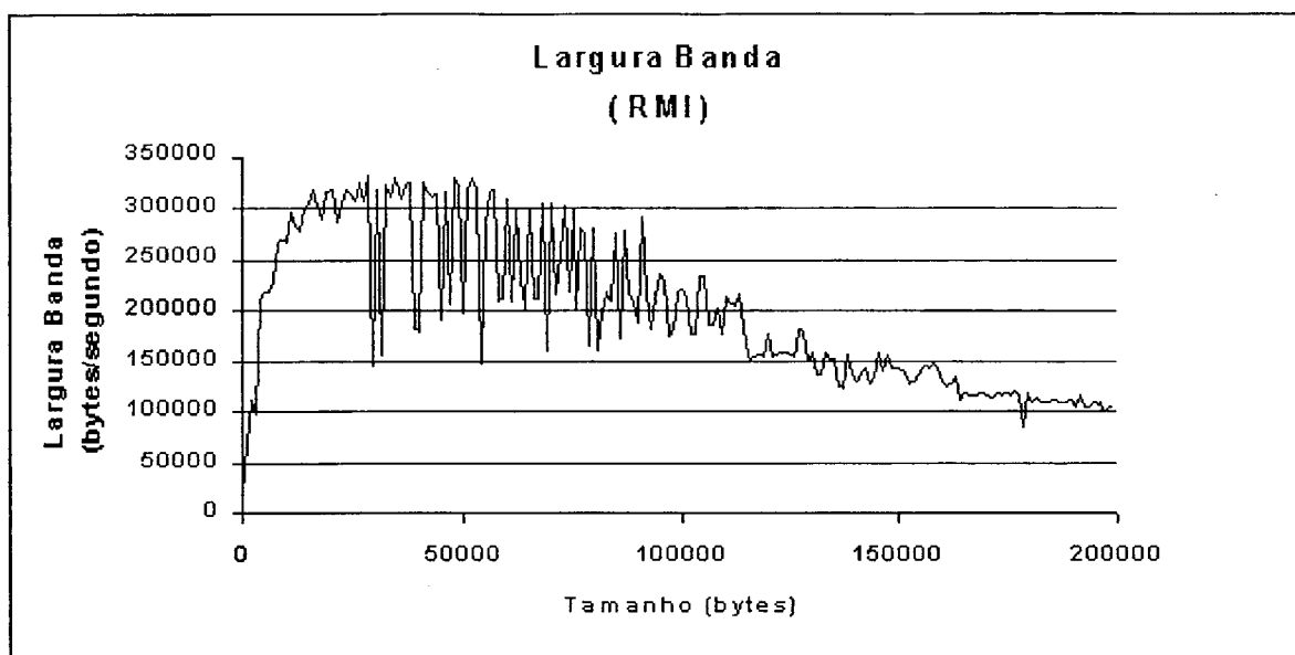
Figura 6.9: Largura de banda — Configuração RMI
