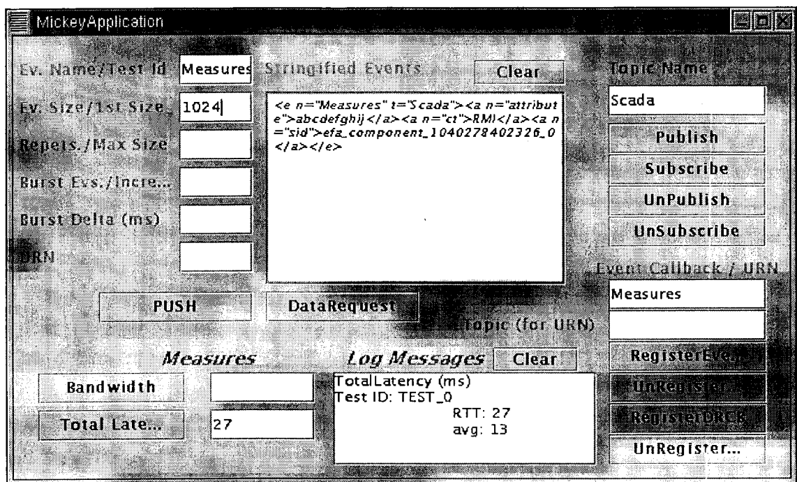
Figura 6.2: Interface gráfica do Simulator
