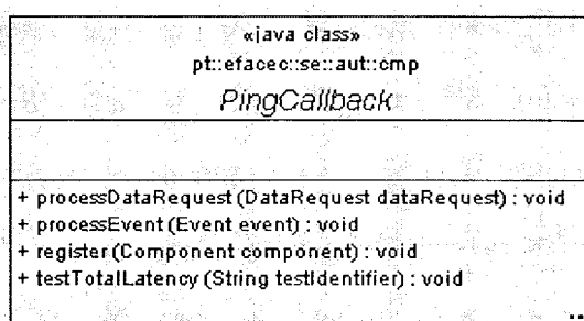
Figura 6.1: Classe PingCallback
