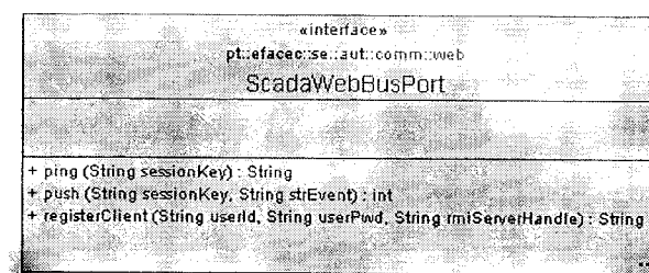
Figura 5.5: Interface do serviço Web
