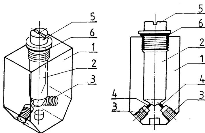
Figura 2.1.3.4 - Amortecedores de pulsos: (1)-bloco de perspex; (2)-cavidade; (3)-roscas; (4)-canais; (5)-tampa; (6)-rosca da tampa.
