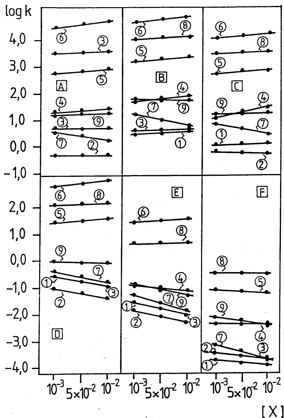
Figura 3.3.5.1- Variações nos coeficientes de selectividade ( \log K^{POT} ) dos eléctrodos construídos :[(A)-propionato; (B)-acetato; (C)-formiato; (D)-cloroacetato; (E)-dicloroacetato; (F)-tricloroacetato] de acordo com a concentração dos iões interferentes: (1)-propionato; (2)-acetato; (3)-formiato; (4)-cloroacetato; (5)-dicloroacetato; (6)-tricloroacetato; (7)-sulfato; (8)-nitrato; (9)-cloreto.
