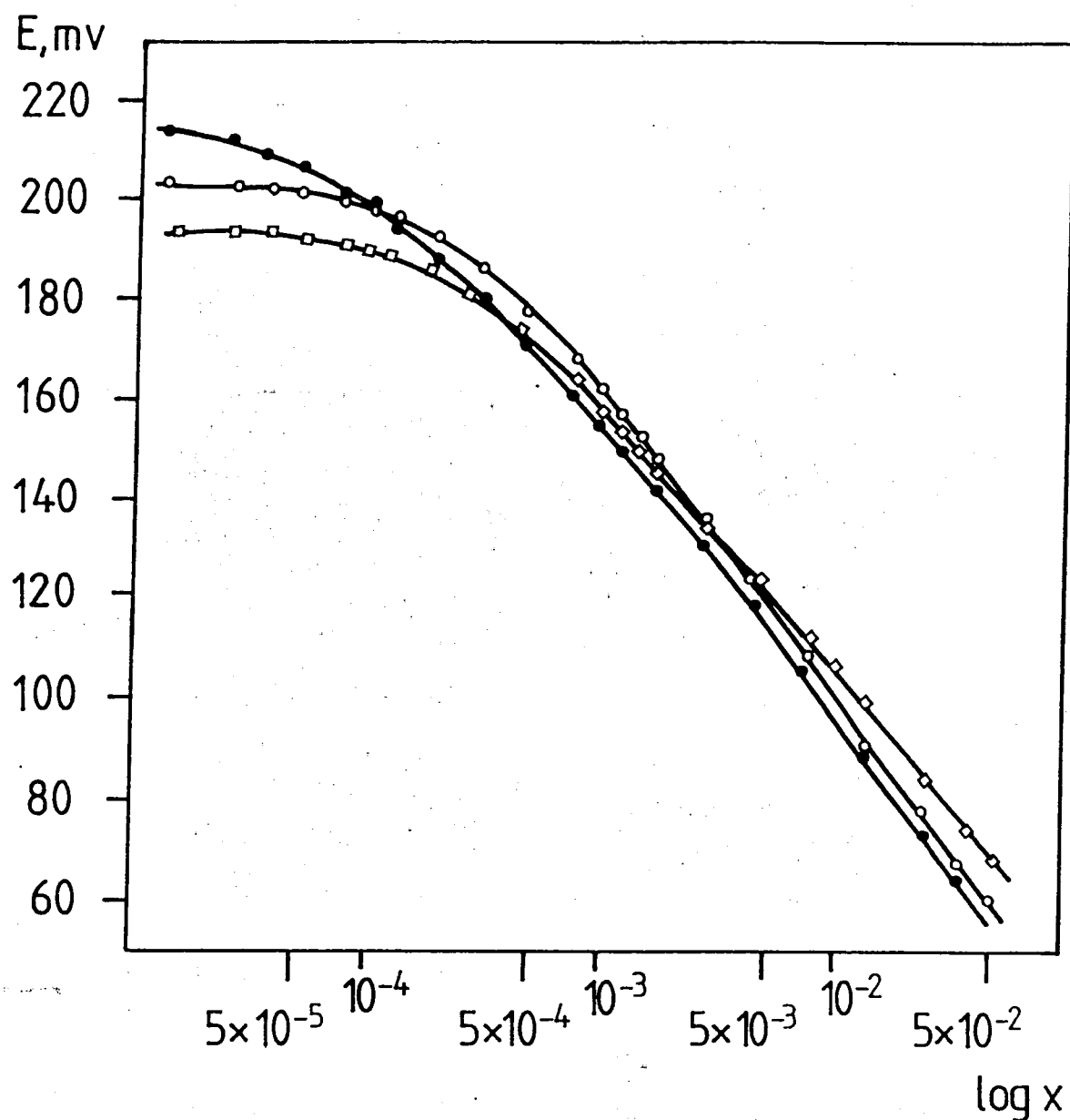
Figura 4.3.1.1 - Curvas de calibração típicas para eléctrodos de benzoato de tetraoctilamónio em dibutilftalato, efectuadas em soluções: (●) sem a força iónica ajustada; (○) com a força iónica ajustada a 0,1 M com sulfato de amónio 0,033 M e (◻) com a força iónica e pH ajustados.
