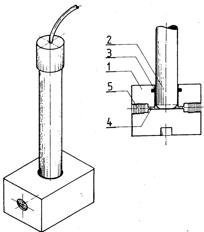
Figura 2.1.3.1 - Confluências: (1)-bloco de perspex; (2)-canais; (3)-roscas de ligação.
