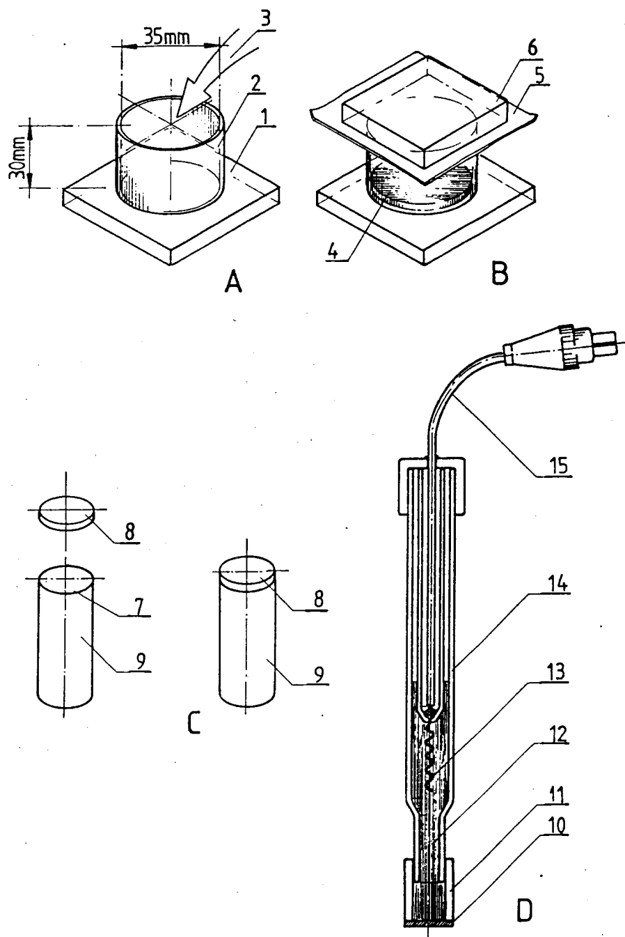
Figura 1.3.1 - Fases de preparação de um eléctrodo com solução de referência interna. (A) e (B)- preparação da membrana com o sensor imobilizado em PVC que após fixação a um tubo de PVC (C) e posterior adaptação ao corpo do eléctrodo (D) origina a unidade com solução de referência interna: (1)- placa de vidro; (2)-anel de vidro; (3)-solução constituída pelo permutador iónico, solvente mediador e PVC, em tetrahidrofurano; (4)-membrana plástica após evaporação do tetrahidrofurano; (5)-papel de filtro; (6)-peso, (7)-superfície lisa de um tubo de PVC; (8)-discos pequenos cortados da membrana "mãe"; (9)-extremidade inferior do tubo de PVC; (10)-membrana de PVC; (11)-tubo de PVC; (12)-solução de referência interna; (13)-eléctrodo de prata recoberto com cloreto de prata; (14)-corpo do eléctrodo em vidro; (15)-cabo condutor blindado.
