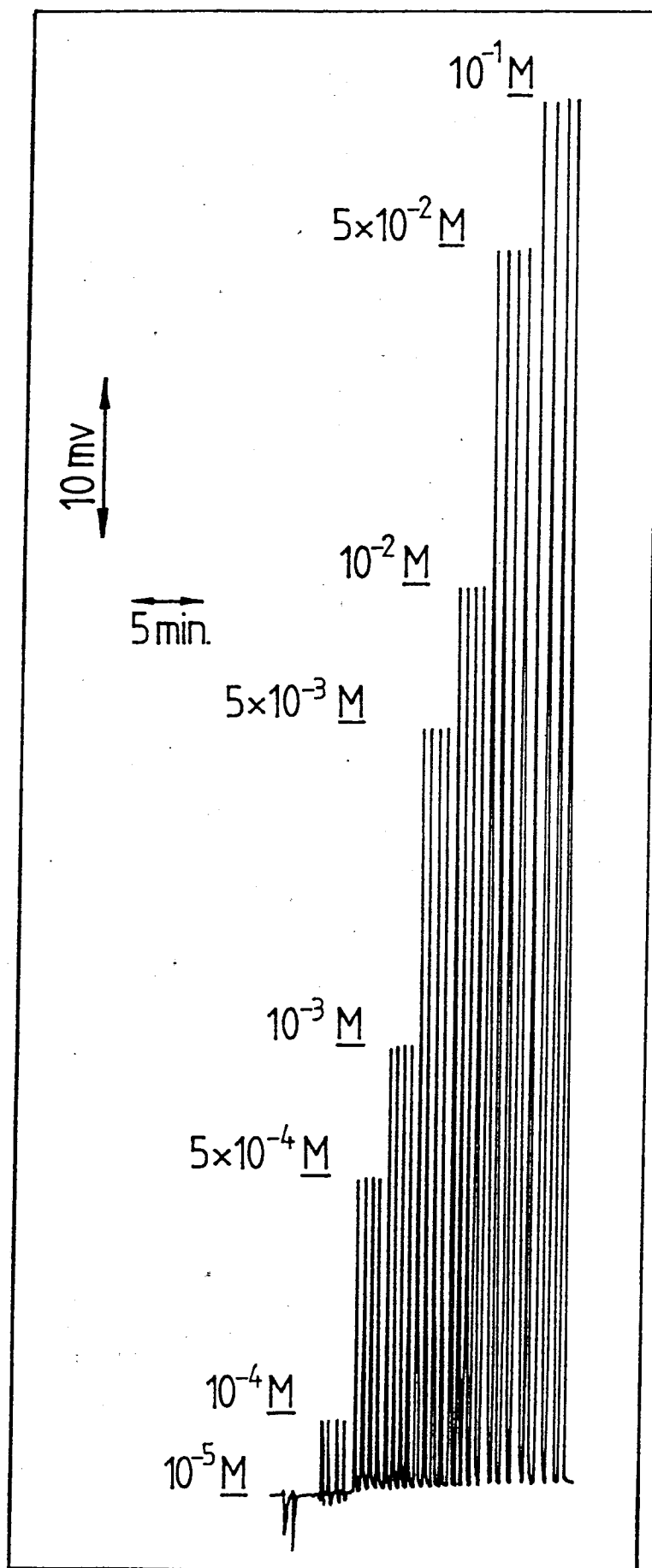
Figura 8.3.1.1- Registro de uma curva de calibração obtida em sistema de canal único com um detector potenciométrico sensível a salicilato.
