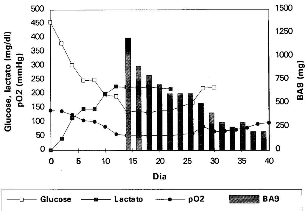
Figura VI-11 Ciclo de produção típico do biorreactor de fibras ocas. A produção decai marcadamente para lá dos 30 dias, provavelmente pela acumulação de detritos celulares.
