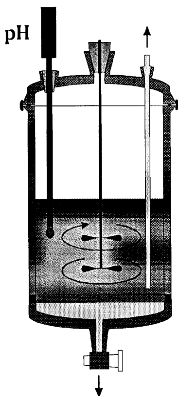
Figura VI-13 Reactor de activação pelo CNBr.
