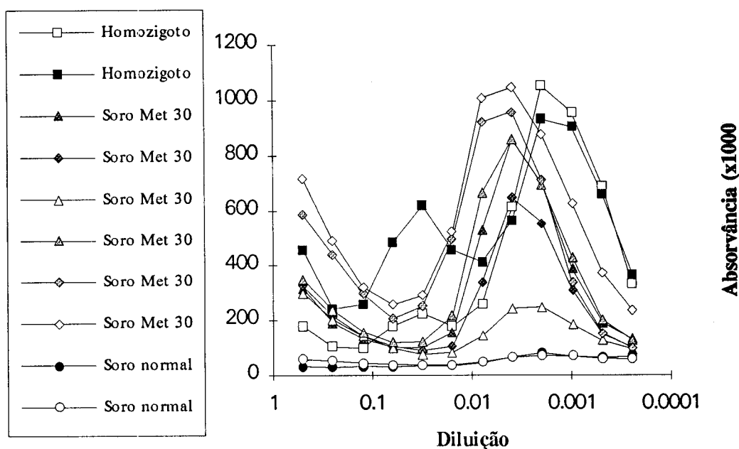
Figura IV-4 Efeito da diluição dos soros em H 2 O sobre o imunoensaio com FD6. Diluições seriadas a 1:2. Dois soros normais, seis de heterozigotos TTR Met 30, e dois de duas colheitas do mesmo homozigoto.
