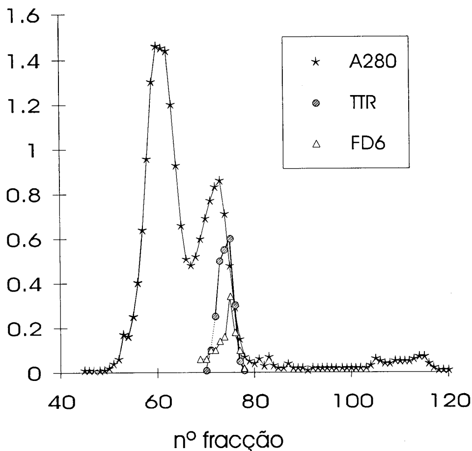
Figura IV-6 Imunoensaio com FD6 de um soro TTR Met 30 fraccionado por filtração em gel. Coluna Sephadex G-100 de 1,6 × 90 cm. Fluxo de 2 cm/hora. Amostra de 0,5 ml de soro. Colheram-se fracções de 1 ml, testadas por imunoensaio com FD6 após diluição em soro normal. Legenda: A280 - Absorvância a 280 nm. TTR - Concentração total de TTR (unidades arbitrárias). FD6 - Imunoensaio com FD6 (valores de absorvância a 280 nm não corrigidos).
