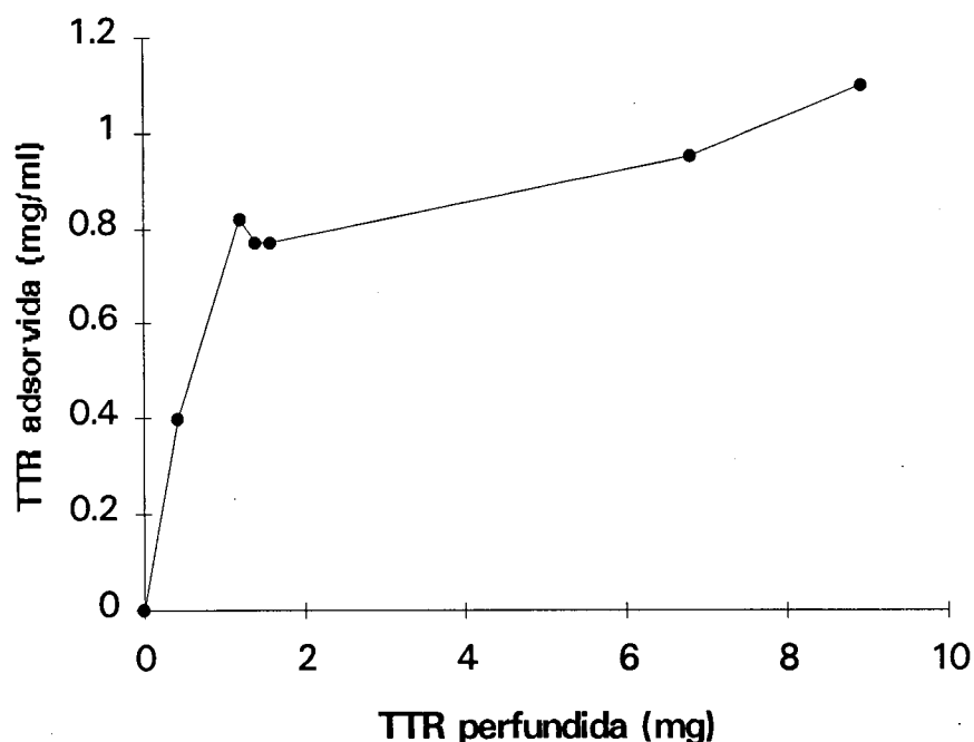
Figura VI-3 TTR adsorvida em função da TTR total perfundida. Imunoabsorvente BA9(4). Tempo de residência de 10 minutos. A adsorção é quantitativa até cerca de 80% da capacidade total.
