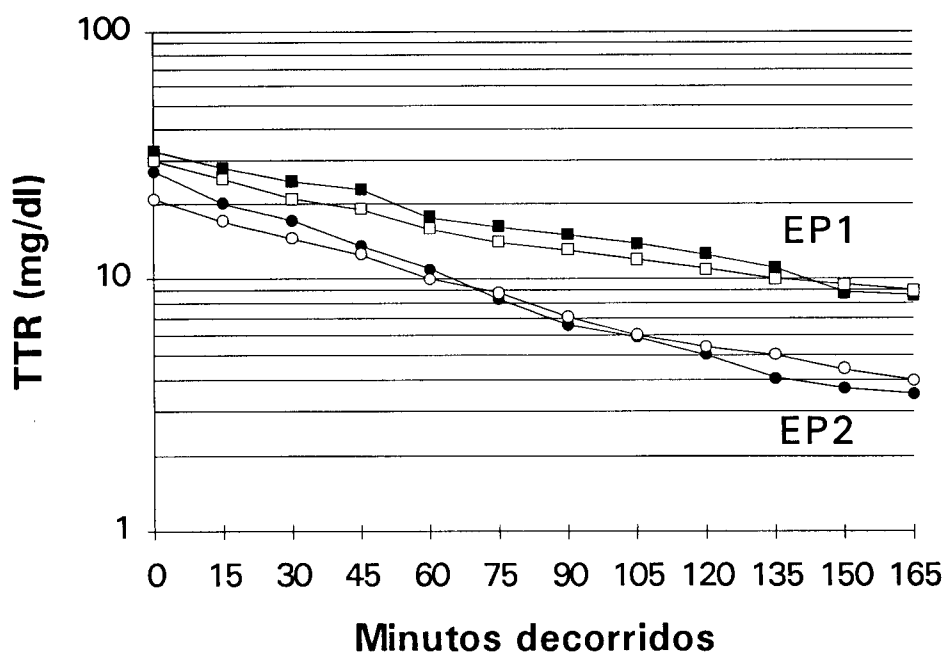
Figura VI-15 EP1 e EP2: perfil logarítmico da descida da concentração plasmática de TTR durante duas das primeiras sessões.
