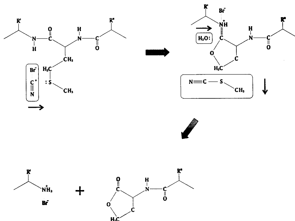
Figura III-2 Acção do CNBr sobre péptidos contendo resíduos de metionina.
