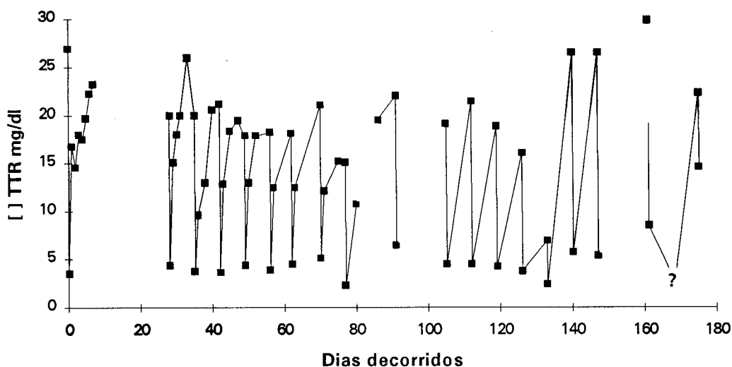
Figura VI-20 EP2: Evolução da concentração plasmática de TTR durante o ensaio.
