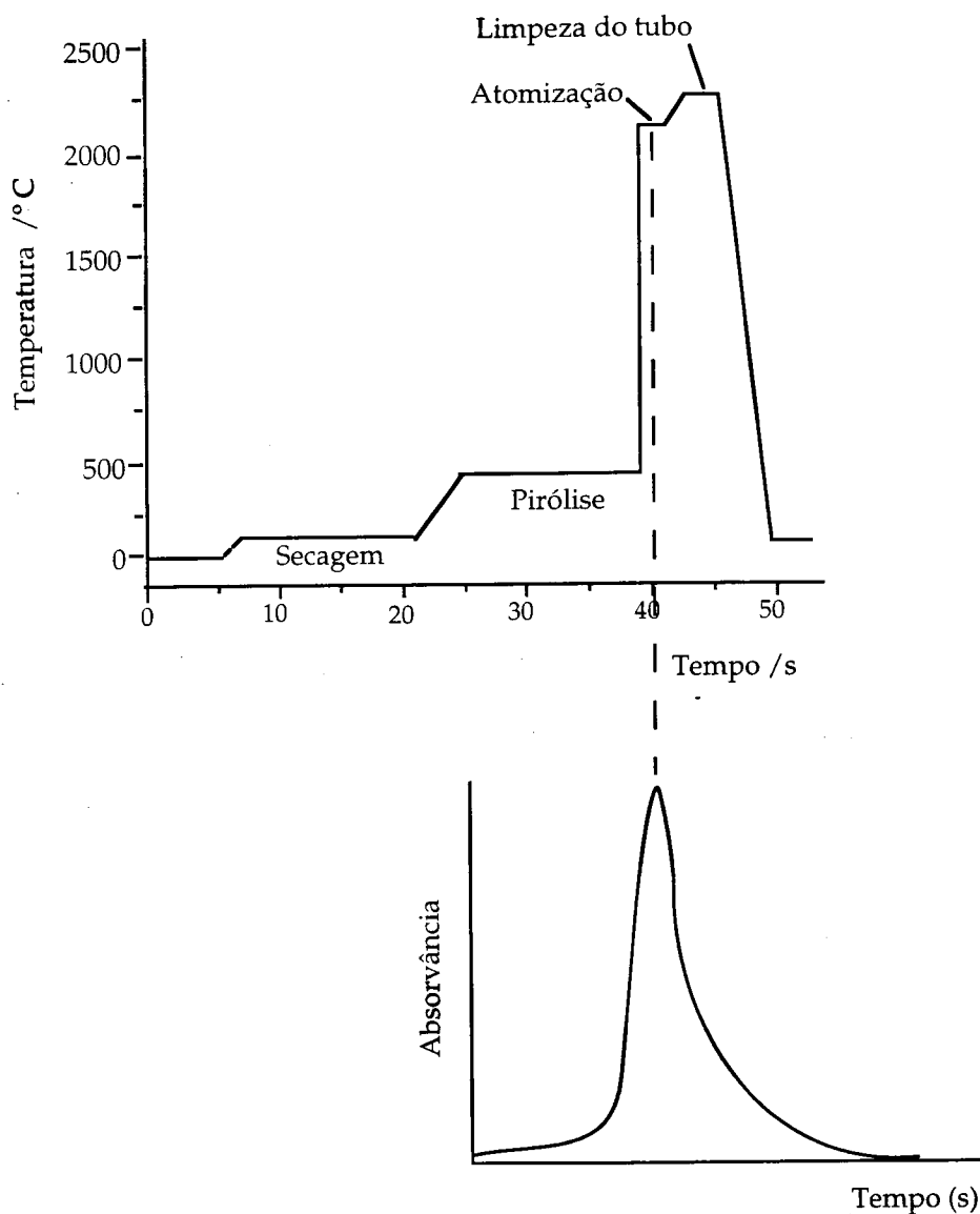
Figura 2.1.5. Exemplo de um programa de atomização electrotérmica e de um registo de sinal. Adaptado das referências 32,36 .
