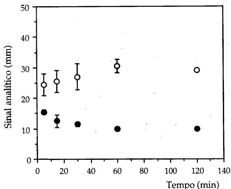
Figura 3.1.7. Variação do sinal analítico da PRA em função do tempo de pré-equilíbrio das soluções contendo 3,15 \mu\text{mol/L} de cobre e 10 (○) ou 50 (●) mg/L de AF. Os valores médios são acompanhados do desvio padrão ( n = 3 ).
