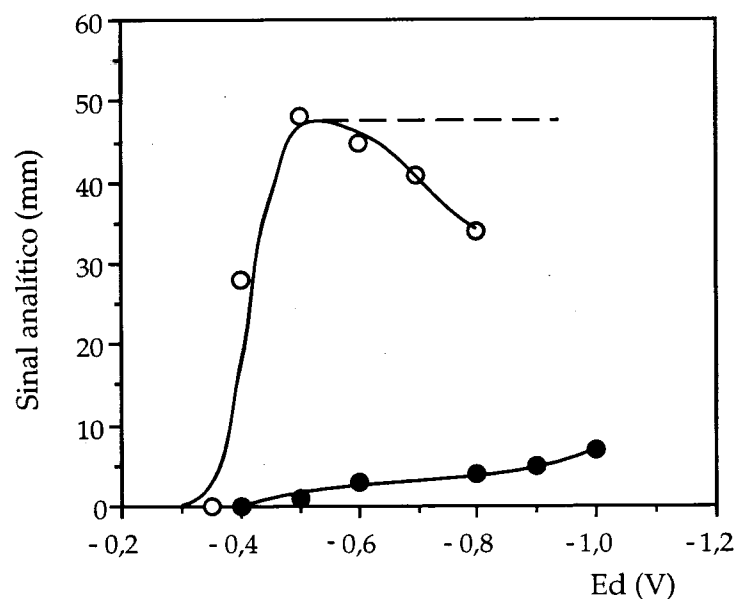
Figura 3.1.6. Variação do sinal analítico em função do potencial de deposição aplicado. Soluções de (○) 3,15 \mu\text{mol/L} de cobre(II) e de (●) 3,15 \mu\text{mol/L} de cobre(II) e 100 mg/L de AF em água do mar sintética para t_d = 1 min.
