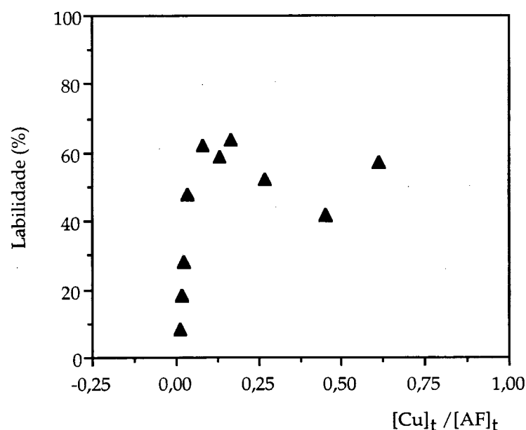
Figura 3.1.9. Variação da labilidade dos complexos de cobre com AF com a razão molar [\text{Cu}]_t / [\text{AF}]_t . As determinações foram efectuadas por PRA a um potencial de deposição de - 0,5 V vs. ESC em meio de perclorato de sódio 0,5 mol/L, a pH 6,5.
