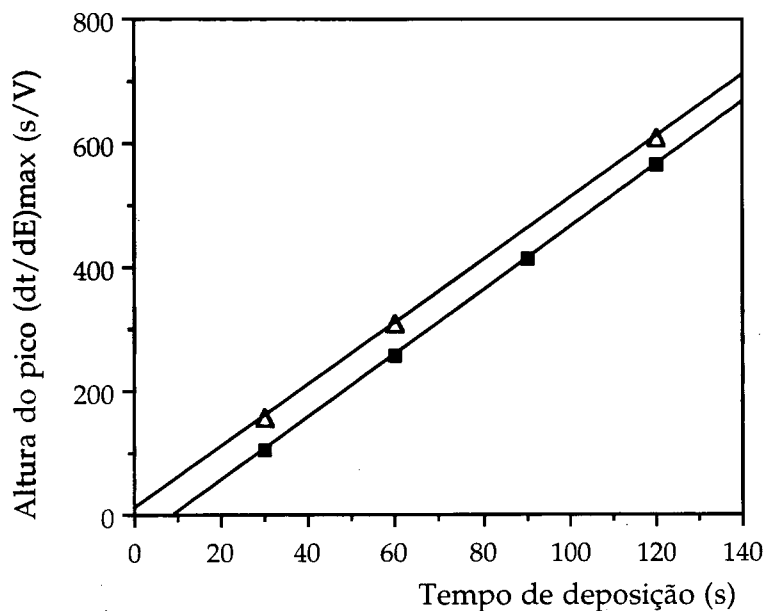
Figura 3.4.11. Influência do t_d na altura do pico [(dt/dE)_{\max}] observado por PRA, para concentração de cobre de 0,787 \mu\text{mol/L} , sem ( \Delta ) e com AH ( 18 \mu\text{mol/L} ) ( \blacksquare ), a um E_d = 0,4 \text{ V vs. Ag/AgCl (s)} , KCl 3 \text{ mol/L} . Parâmetros de regressão linear: ( \Delta ) [(dt/dE)_{\max}] = (5,0 \pm 0,2) t_d + (7 \pm 15) , R = 0,9999 , P = 0,05 , n = 3 ; ( \blacksquare ) [(dt/dE)_{\max}] = (5,1 \pm 0,0) t_d + (-48 \pm 1) , R = 1 , P = 0,05 , n = 4 . A figura representa os resultados experimentais de uma de duas experiências efectuadas.
