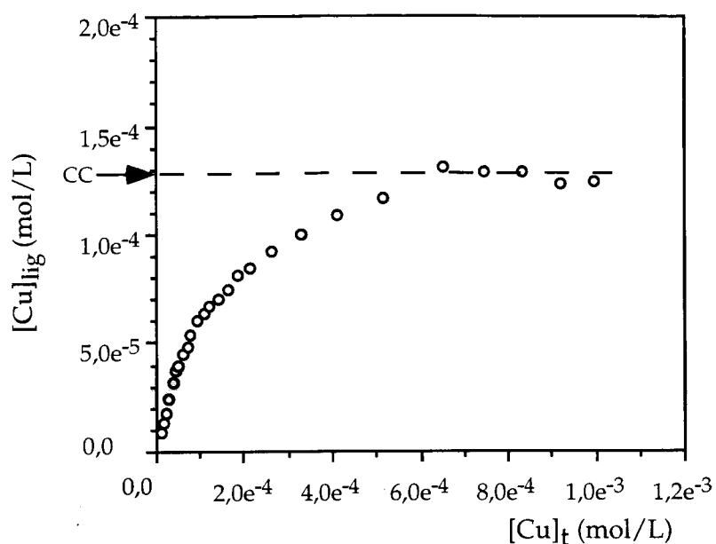
Figura 3.1.2. Variação de [Cu]_{lig} ao longo de uma titulação de AF 50 mg/L com cobre(II) ( I = 0,5 mol/L, perclorato de sódio pH 6,5, t = 20 °C). Valores calculados a partir dos dados apresentados na Figura 3.1.1.
