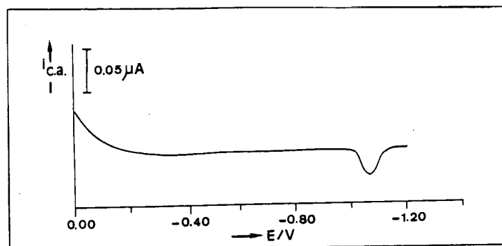
Figura 3.4.4. Polarograma obtido por PCA com uma solução de AH com 18 \mu\text{mol/L} . Amplitude do componente sinusoidal do potencial, 10 \text{ mV} ; frequência do potencial alternado, 75 \text{ Hz} ; velocidade de varrimento, 5 \text{ mV/s} e \phi = 0^\circ .
