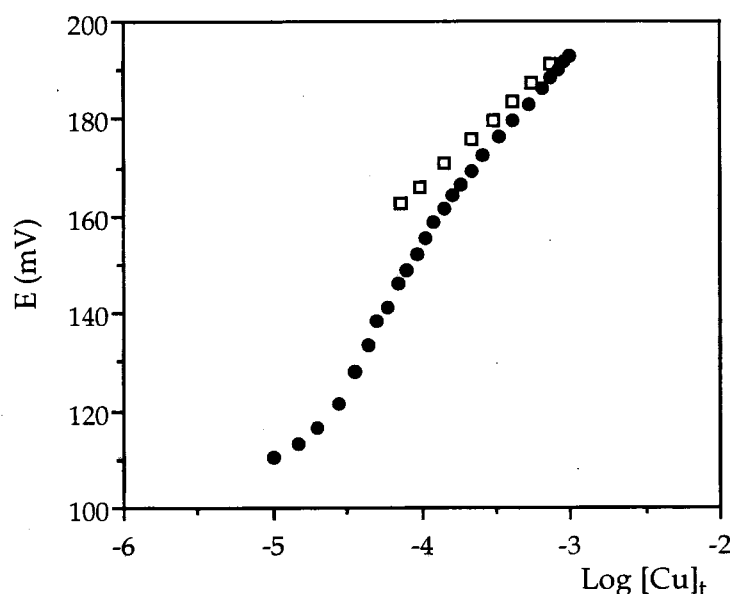
Figura 3.1.1. Curva de titulação, por PESC, (●) de AF 50 mg/L em perclorato de sódio 0,5 mol/L com cobre a pH 6,5 e à temperatura de 20 °C e respectiva curva de calibração (□): E \text{ (mV)} = (28,6 \pm 0,4) \log [Cu]_t + (280 \pm 1) ; R = 0,99992 , P = 0,05 , n = 8 . Os resultados apresentados são a média da resposta de dois eléctrodos colocados na mesma solução e constituem um exemplo típico de uma de cinco experiências efectuadas.
