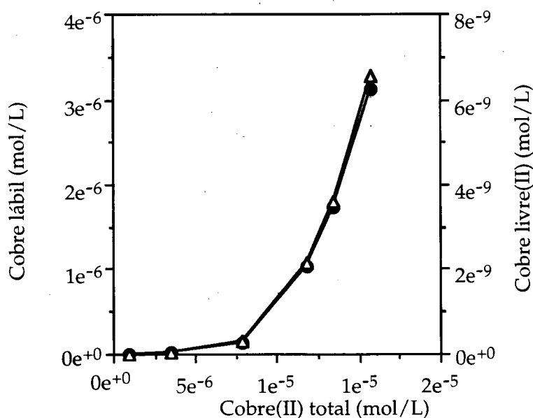
Figura 3.5.8. Variação das concentrações de cobre(II) livre (Δ) e lábil calculados (●), com a concentração total de cobre(II) em água do mar sintética.
