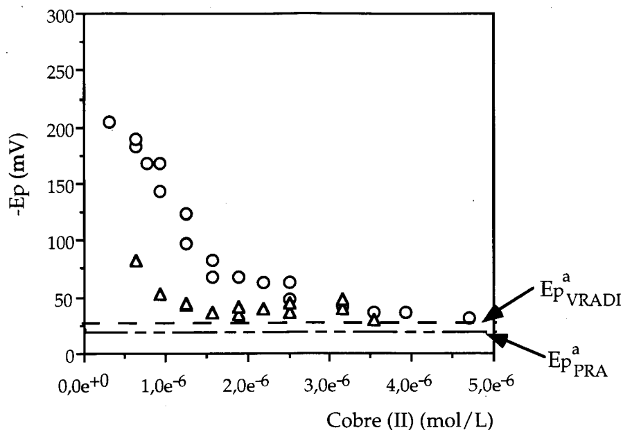
Figura 3.4.14. Variação de E_p obtida por PRA ( \Delta ) e VRADI ( \bigcirc ) ao longo da titulação de 8,28 \times 10^{-5} mol/L em AH com cobre(II). Os valores de E_p^a obtidos por cada uma das técnicas são também mostrados. A figura representa os resultados experimentais de uma de duas experiências efectuadas.
