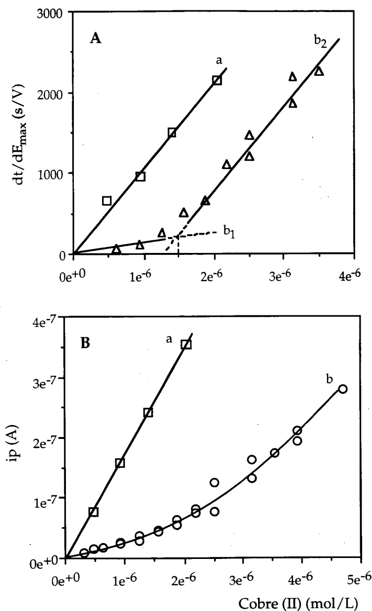
Figura 3.4.13. Variação de (dt/dE)_{\max} (A) e de i_p (B) obtidos por PRA e VRADI, respectivamente, durante a titulação de AH 8,28 \times 10^{-5} mol/L com cobre (II): curvas de calibração ( \square ), AH ( \Delta, \circ ). A figura representa os resultados experimentais de uma de duas experiências efectuadas.
