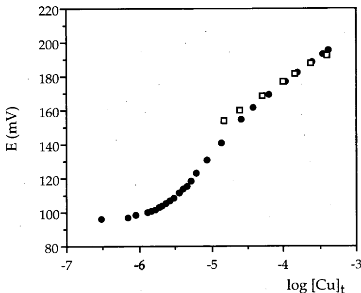
Figura 3.4.1. Curva de titulação (●) de uma solução de AH em nitrato de potássio 10 mmol/L com cobre a pH 6,5 e respectiva curva de calibração (□) ( E \text{ (mV)} = (28 \pm 1) \log [\text{Cu}]_t + (287 \pm 4) ; R = 0,9995 , P = 0,05 , n = 7 ). Valor de CC calculado: 22,8 \pm 0,9 \mu\text{mol/L} (média e desvio padrão, n = 3 ).
