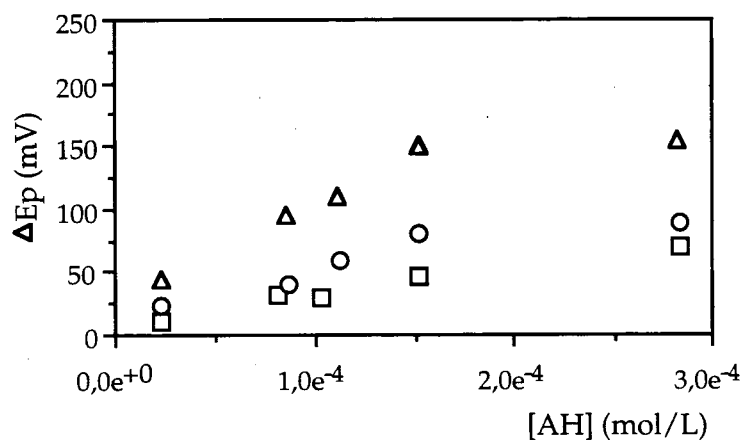
Figura 3.4.12. Variação de \Delta E_p ao longo da titulação de cobre(II) 2,20 \mu\text{mol/L} com AH. Resultados obtidos por VRADI ( \Delta ), PRA ( \circ ) e PESC/PDI ( \square ) (ver secção 3.4.4.3). A figura representa os resultados experimentais de uma de duas experiências efectuadas.
