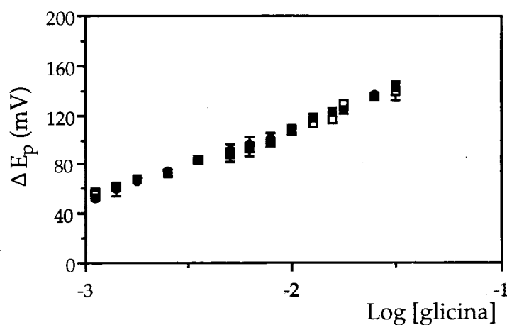
Figura 3.3.4. Valores médios e desvios padrão ( n = 3 ) de \Delta E_p vs. [glicina] para soluções 0,787 \mu\text{mol/L} em cobre (II) obtidos por PRA (□) e por VRADI (●), a pH 6,0.
