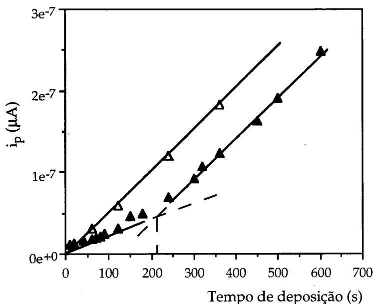
Figura 3.4.7. Variação de i_p com t_d (Δ sem AH, ▲ com AH 18 \mu\text{mol/L} ) por VRADI para uma solução de 0,787 \mu\text{mol/L} de cobre(II). A figura representa os resultados de uma de duas experiências efectuadas.
