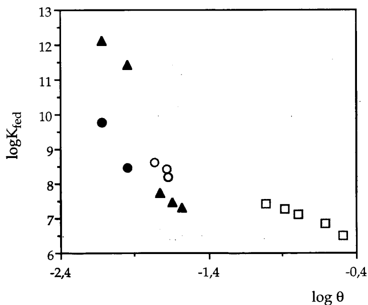
Figura 3.4.15. Comparação dos valores de \log K_{fed} obtidos para os complexos de cobre(II)-AH por PESC ( \square ), VRADI ( \blacktriangle ) e PRA ( \bullet, \circ ). Neste último caso, os valores de \log K_{fed} foram calculados a partir das equações [8] ( \bullet ) e [11], [15] e [16] ( \circ ), respectivamente.
