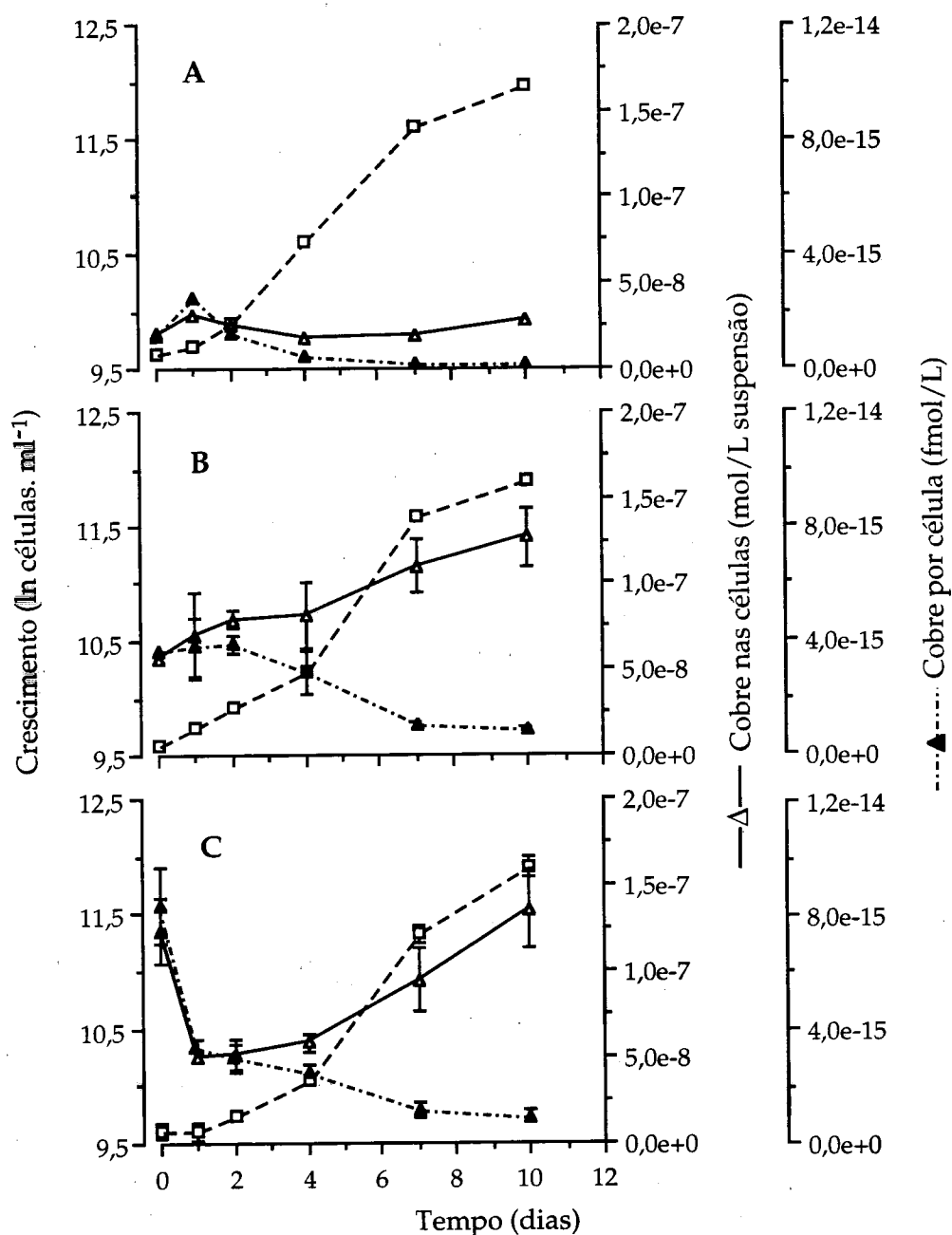
Figura 3.5.11. Comparação dos valores da concentração de cobre nas células ( \Delta , \blacktriangle ) e do crescimento celular ( \square ). (A) Controle, (B) 13,4 \mu\text{mol/L} de cobre(II) total inicial na solução com pré-equilíbrio e (C) a mesma concentração mas sem pré-equilíbrio. Os resultados apresentados correspondem à média e desvio padrão de três determinações, excepto para o controle em que apresenta-se apenas a média de dois ensaios.
