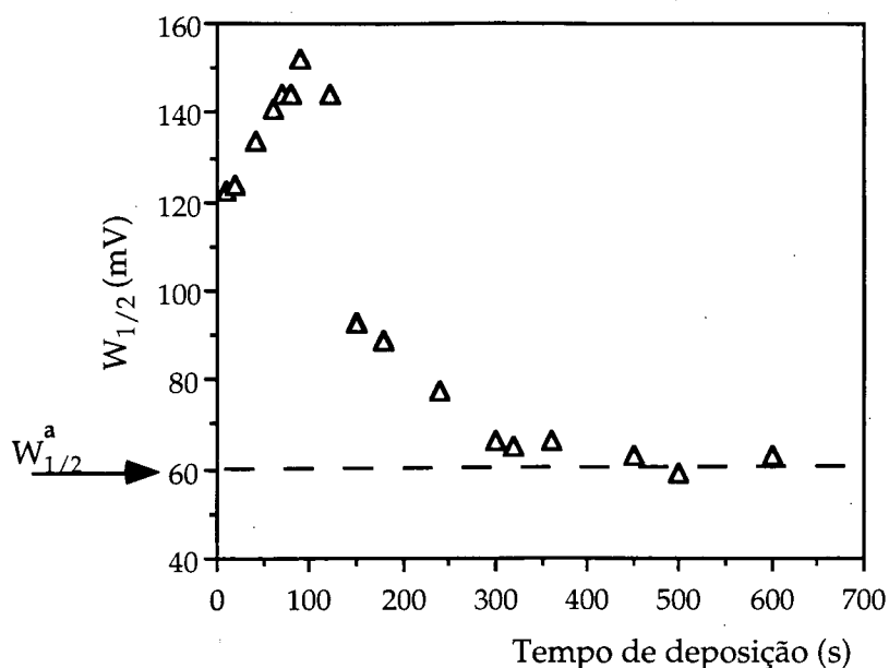
Figura 3.4.9. Variação de W_{1/2} com o t_d para uma solução 18 \mu\text{mol/L} em AH e 0,787 \mu\text{mol/L} em cobre. O valor de W_{1/2}^a , i.e. , o observado na ausência de ligando foi também incluído. A figura representa os resultados experimentais de uma de duas experiências efectuadas.
