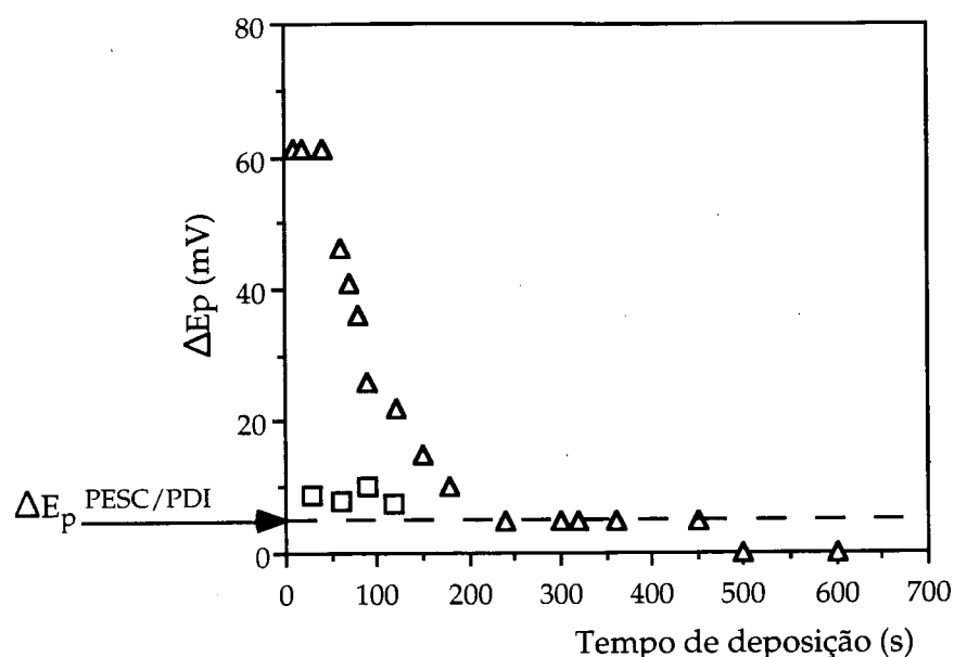
Figura 3.4.8. Variação de \Delta E_p com t_d por VRADI ( \Delta ) e por PRA ( \square ) para uma solução 18 \mu\text{mol/L} em AH e 0,787 \mu\text{mol/L} em cobre(II). O valor de \Delta E_p estimado por PESC/PDI (ver secção 3.4.4.3) foi também incluído. A figura representa os resultados experimentais de uma de duas experiências efectuadas.
