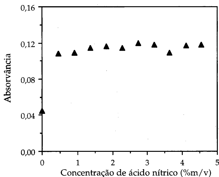
Figura 3.5.4. Estudo da influência da concentração de ácido nítrico no sinal analítico do cobre 0,315 \mu\text{mol/L} (ver programa de temperaturas na secção 2.2.4.4).
