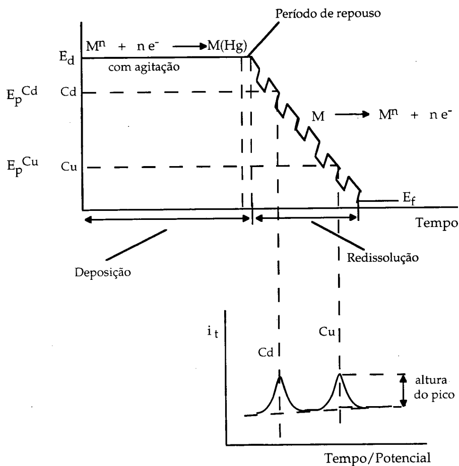
Figura 2.1.3. Procedimento da medição da corrente e do potencial do pico em VRADI. Adaptado das referências 8,18 .
