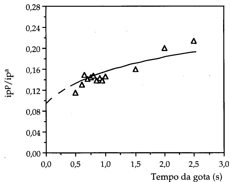
Figura 3.4.6. Variação de ipP/ip^a com o tempo da gota, obtido por PDI, para uma solução 152 \pm 29 \mu\text{mol/L} (média e desvio padrão, n = 3 ) em AH e 38 \mu\text{mol/L} em cobre(II).
