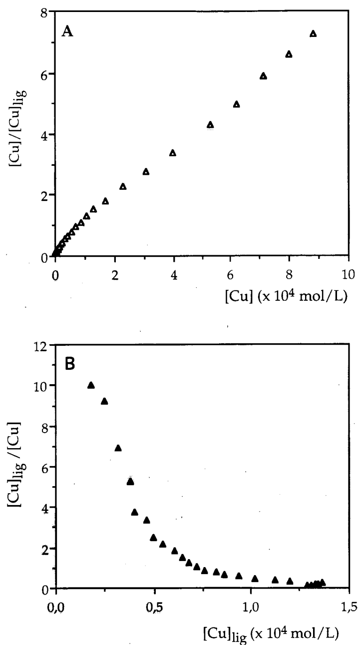
Figura 3.1.5. Resultados típicos obtidos com os modelos de Ruzic (A) e de Scatchard (B) para a titulação, por PES, de uma solução de AF 50 mg/L a 20 °C.
