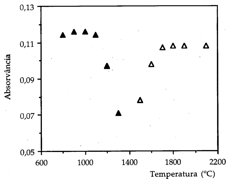
Figura 3.5.3. Estudo das rampas de temperatura de pirólise (▲) (temperatura de atomização 1900 °C durante 5 s) e de atomização (Δ) (temperatura de pirólise 1100 °C durante 20 s) para uma amostra de microalgas, cuja concentração de cobre foi, posteriormente, quantificada em 0,315 \mu\text{mol/L} .
