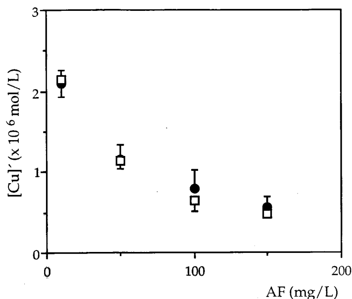
Figura 3.1.10. Influência do pH no valor da concentração de cobre lábil ( [Cu]' ) determinado em água do mar sintética a [Cu]_t = 3,15 \mu\text{mol/L} : (●) pH 6,5; (□) pH 7,5. São apresentados os valores médios de quatro determinações e os respectivos intervalos de confiança ( P = 0,05 ).
