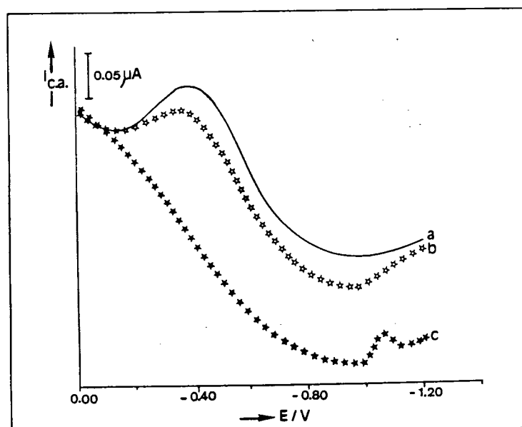
Figura 3.4.2. Polarogramas obtidos por PCA na ausência (a) e na presença de AH: (b) 8 ; (c) 18 \mu\text{mol/L} . Amplitude do componente sinusoidal do potencial, 10 mV; frequência do potencial alternado, 75 Hz; velocidade de varrimento, 5 mV/s e \phi = 90^\circ .
