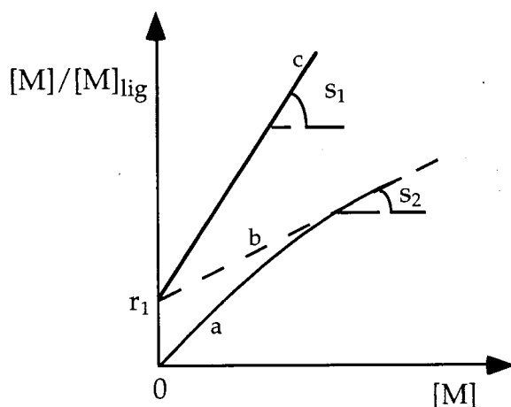
Figura 2.3.1. Representação gráfica de [M]/[M]_{\text{lig}} = f([M]) para a formação de complexos 1:1 entre um metal e dois tipos de locais de coordenação. (a) Representação gráfica original (ver equação [33]); (b) assíntota traçada na zona da curva em que os locais de fixação estão maioritariamente ocupados (ver equação [35]); (c) representação gráfica do inverso da diferença entre os valores das ordenadas da assíntota (curva b) e da curva de titulação com M (curva a) vs. [M] , na zona da curva onde a fixação do metal ao ligando está a ocorrer nos locais mais fortes (ver equação [36]). Adaptado da referência 9 .
