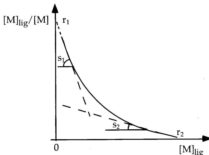
Figura 2.3.2. Representação gráfica de [M]_{\text{lig}}/[M] = f([M]_{\text{lig}}) para a formação de complexos 1:1 entre um metal e dois tipos de locais de coordenação. Adaptado da referência 10 .
