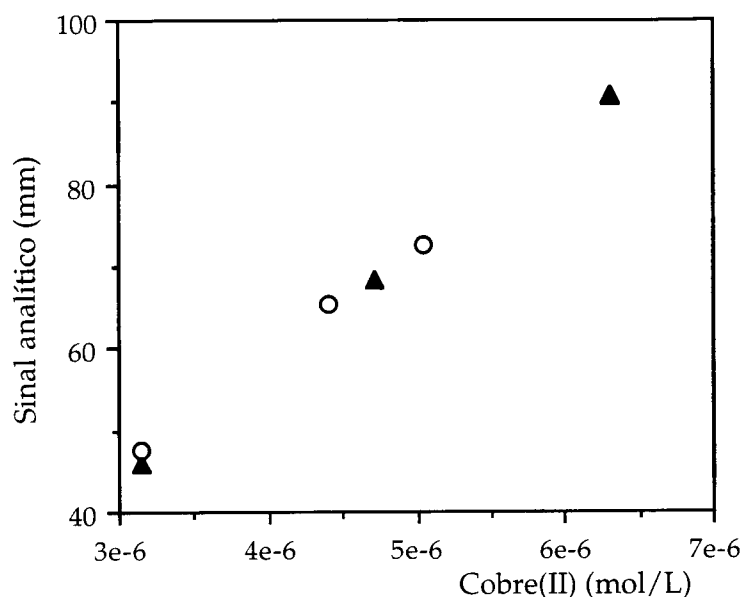
Figura 3.1.8. Variação do sinal analítico em soluções contendo cobre(II) (O) e 1 mg/L de AF (▲).
