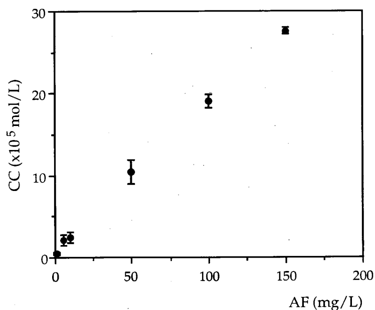
Figura 3.1.3. Valores médios da CC e limites de confiança respectivos ( P = 0,05 , n = 5 ) para diferentes concentrações de AF. Parâmetros de regressão linear: [CC] = (1,81 \pm 0,01) \times 10^{-6}[AF] + (0,8 \pm 0,8) \times 10^{-6} ; R = 0,998 , P = 0,05 , n = 6 .
