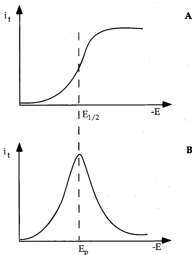
Figura 2.1.1. Polarogramas obtidos por polarografia clássica (A) e por polarografia diferencial com impulsos (B). Adaptado da referência 11 .
