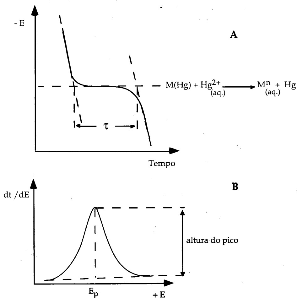
Figura 2.1.4. Potenciogramas típicos na forma directa (A) e na forma da primeira derivada (B). Adaptado da referência 26 .
