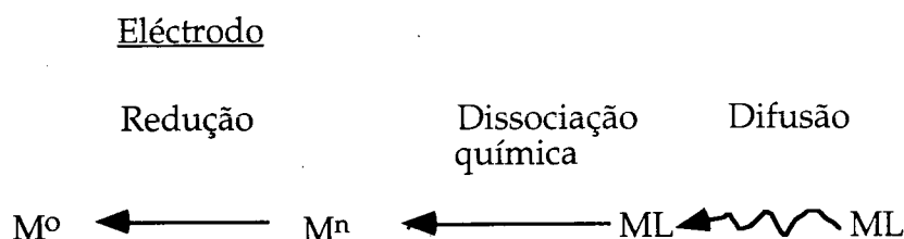
Figura 3.2 .1. Representação esquemática dos fenómenos que podem ocorrer à superfície do eléctrodo de trabalho para o complexo ML. Adaptado da referência 5 .
