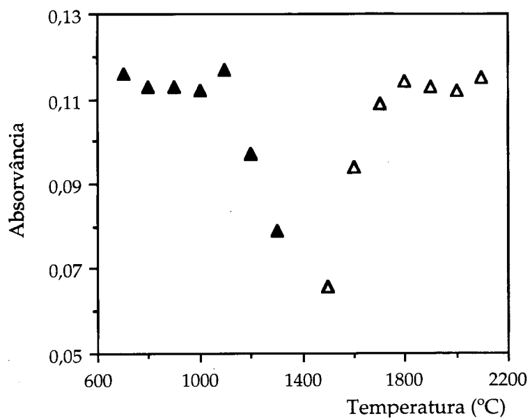
Figura 3.5.2. Estudo das rampas de temperatura de pirólise (▲) (temperatura de atomização 1900 °C durante 5 s) e de atomização (Δ) (temperatura de pirólise 1100 °C durante 20 s) para uma solução padrão de cobre 0,315 \mu\text{mol/L} .
