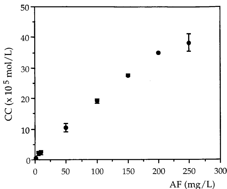
Figura 3.1.4. Variação dos valores médios da CC para diferentes concentrações de AF. Incluem-se os limites de confiança respectivos ( P = 0,05 , n \geq 3 ).
