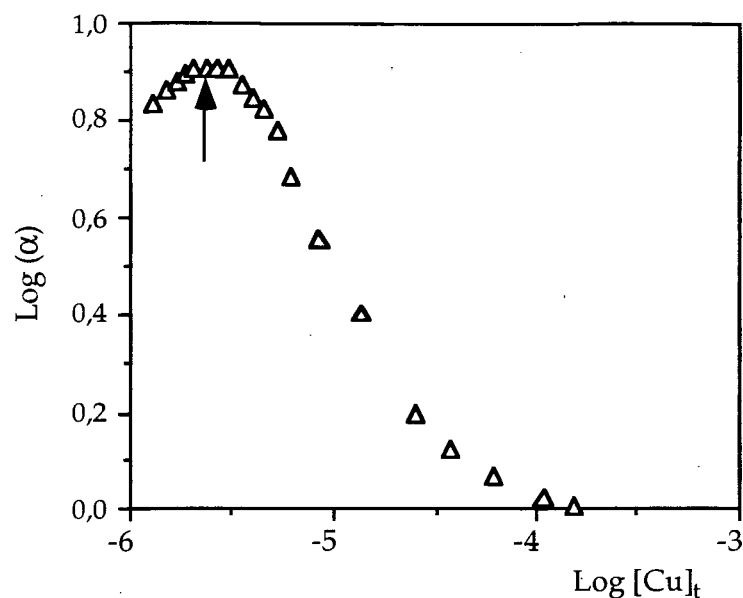
Figura 3.4.5. Exemplo típico do modo de determinação de \alpha ( = [\text{Cu}]_t/[\text{Cu}] ), obtido ao longo da titulação, por PESC, de uma solução 22,8 \mu\text{mol/L} em AH com cobre(II). Valores obtidos a partir dos resultados apresentados na Figura 3.4.1. A seta assinala o valor de \alpha utilizado no cálculo de \Delta E_p para a concentração de AH referida usada na Figura 3.4.12.
