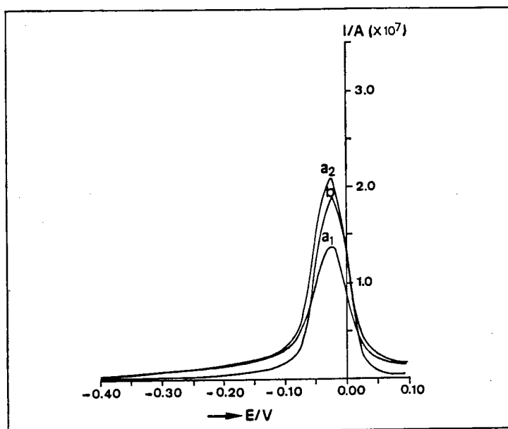
Figura 3.4.10. Voltamogramas obtidos com 0,787 \mu\text{mol/L} de cobre(II) na presença (a) e na ausência (b) de AH 18 \mu\text{mol/L} , a um E_d = -0,4 \text{ V vs. Ag/AgCl (s)} KCl 3 \text{ mol/L} , para vários t_d : (a 1 ) t_d = 360 \text{ s} , (a 2 ) t_d = 500 \text{ s} ; (b) t_d = 360 \text{ s} .
