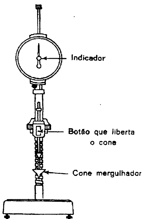
Fig. 31 - Penetrómetro da F.P.V
