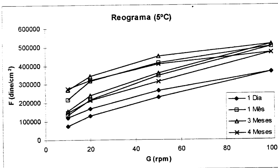
Fig. 35 - Reograma do creme F 3 armazenado a 5°C.
