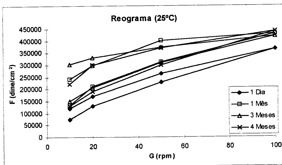
Fig. 36 - Reograma do creme F 3 armazenado a 25°C.
