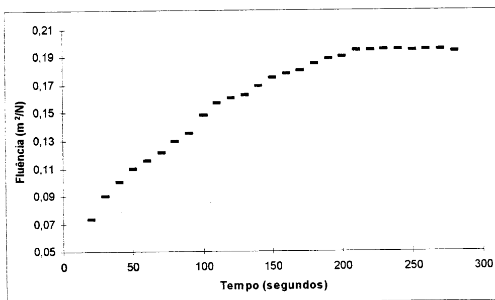
Fig. 41 - Curva de fluência em função do tempo, do creme F_3 armazenado a 25^\circ\text{C} , 4 meses após a preparação.
