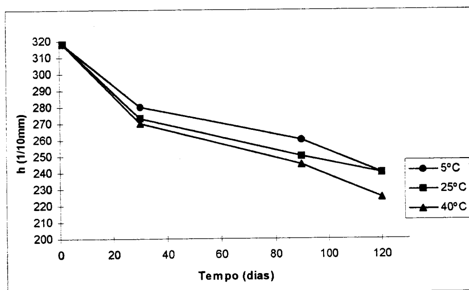
Fig.32 - Profundidade de penetração em função do tempo de armazenamento
