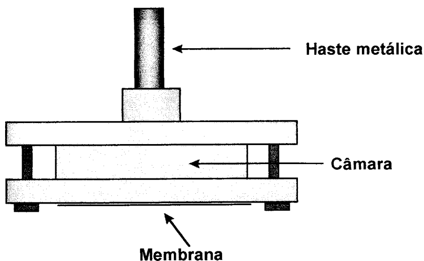
Fig. 18 - Célula de difusão de Jhawar-Lordi.
