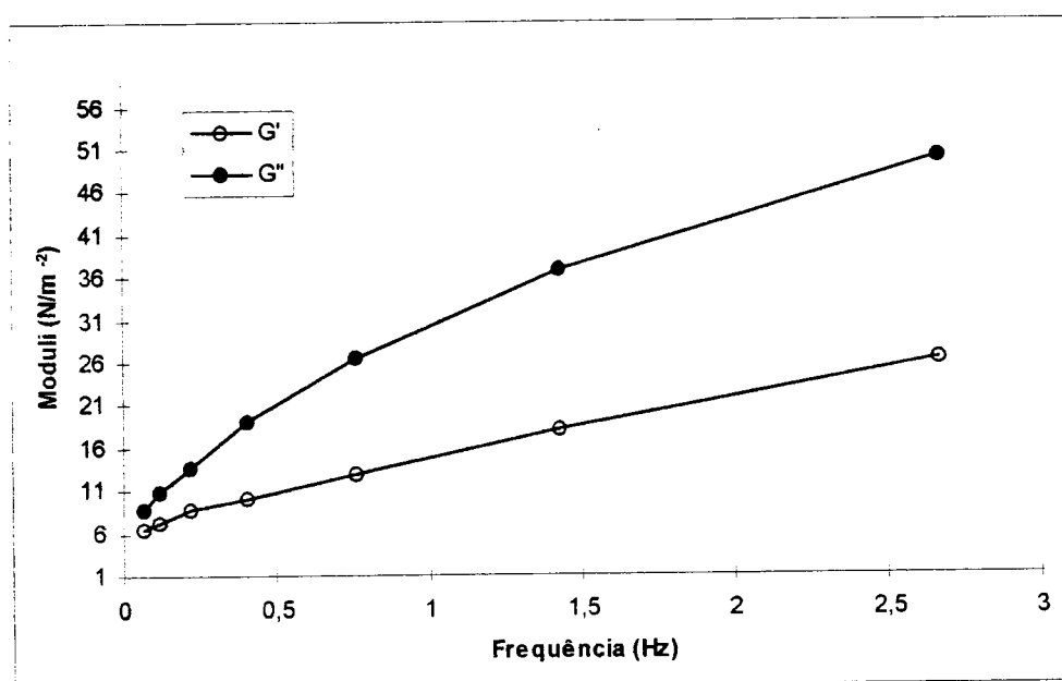
Fig. 40 - Espectro mecânico obtido com os moduli G' e G'' , 4 meses após a preparação do creme F_3 , armazenado a 25^\circ\text{C} .
