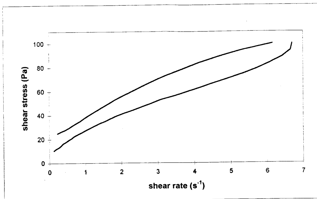
Fig,38 - Reograma do creme F 3 , 4 meses após o seu armazenamento a 25°C
