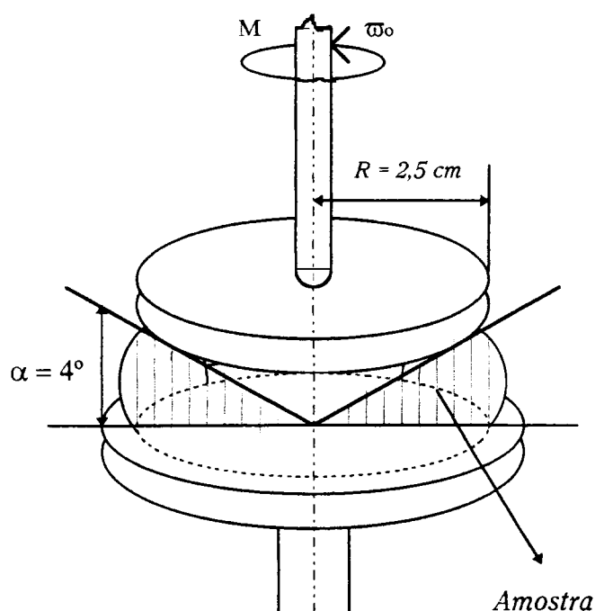
Fig.39 - Cone/prato do CARRIMED CSL 50.
