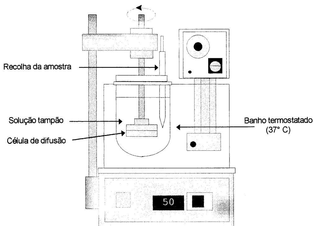
Fig. 19 - Adaptação da célula de difusão no aparelho de dissolução da F.P. V.
