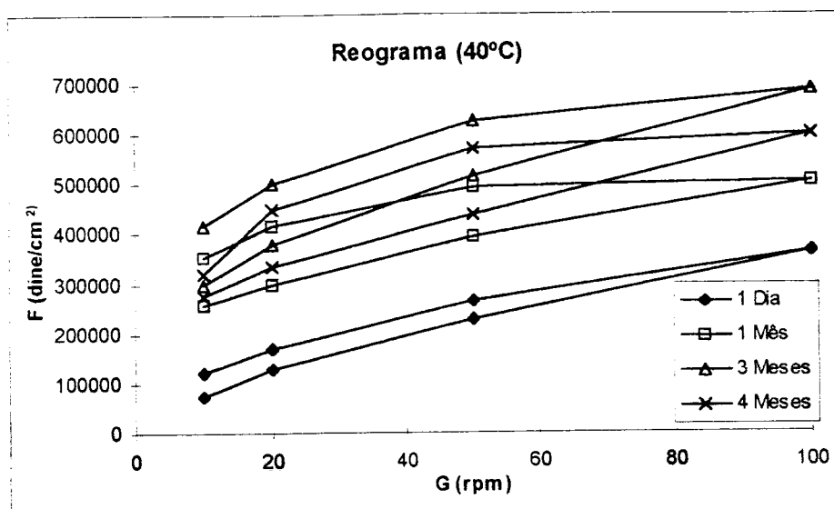
Fig. 37 - Reograma do creme F_3 armazenado a 40°C.
