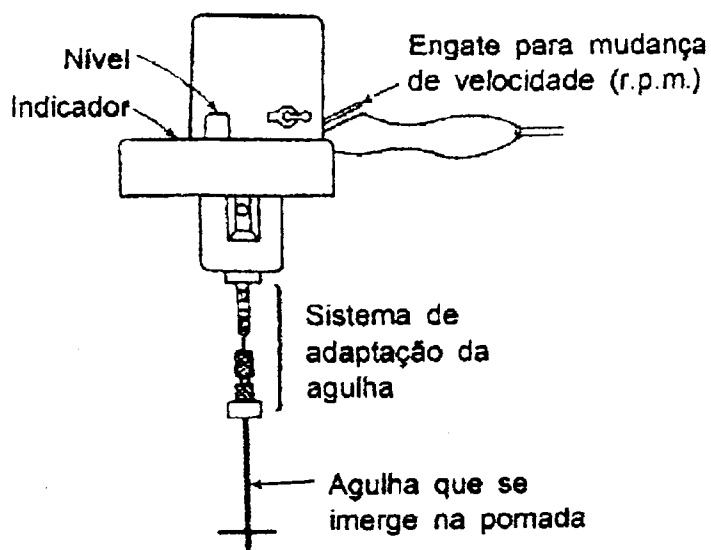
Fig. 34 - Viscosímetro rotativo Brookfield, RV.
