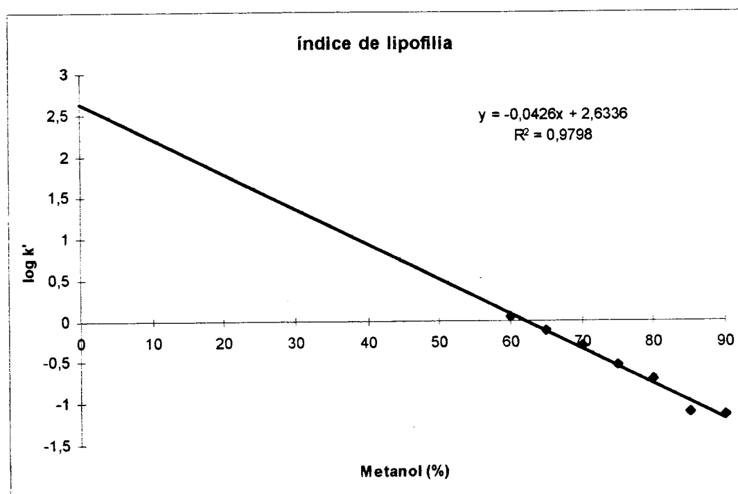
Fig.14 - Índice de lipofilia do naproxeno correspondente às determinações efectuadas utilizando uma coluna C 18 , 250x4,6mm, 10µm.
