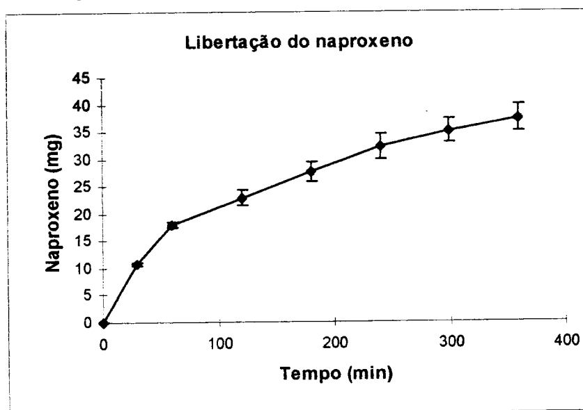
Fig. 16 - Quantidade acumulada de naproxeno libertado em função do tempo.
