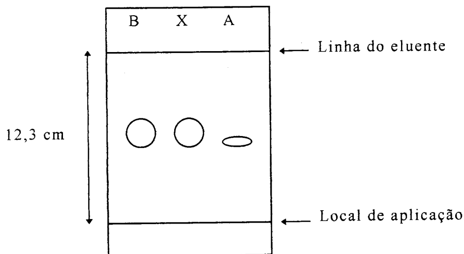
Fig. 7 - Cromatograma do naproxeno matéria-prima.
