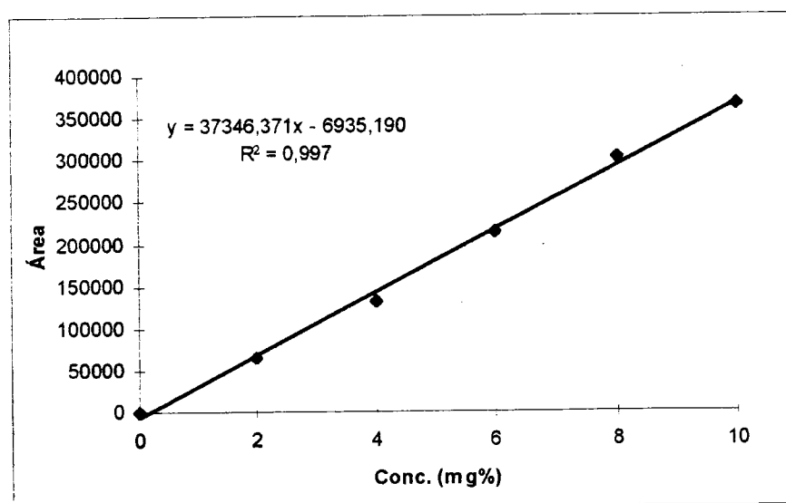
Fig.11 - Correlação entre as áreas de pico e a concentração de naproxeno.
