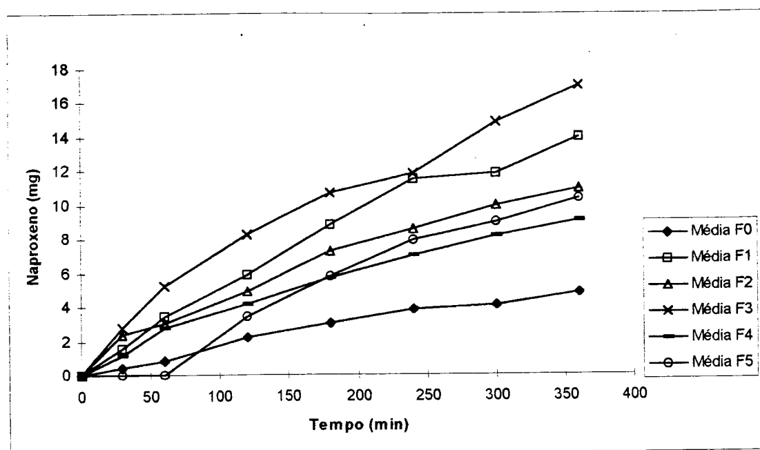
Fig. 29 - Quantidade acumulada de naproxeno que penetra em função do tempo.
