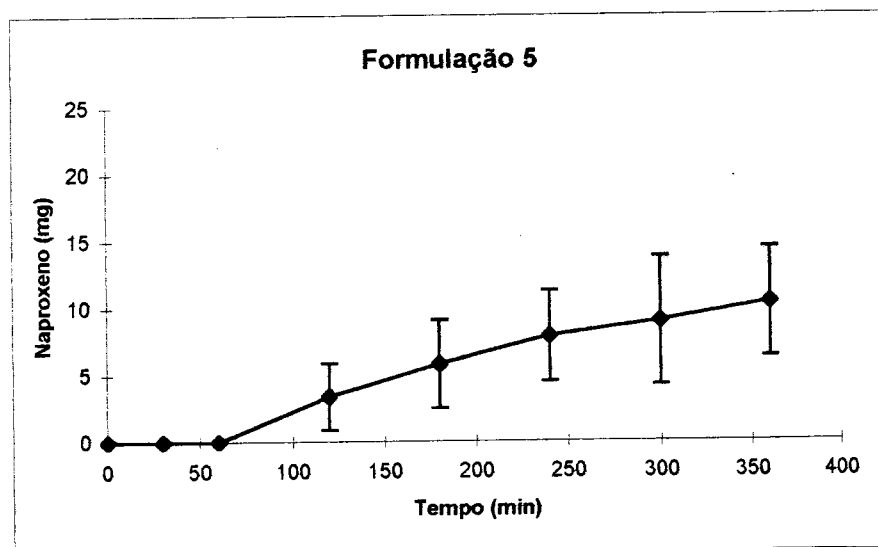
Fig. 28 - Quantidade acumulada de naproxeno da F_5 que difunde.
