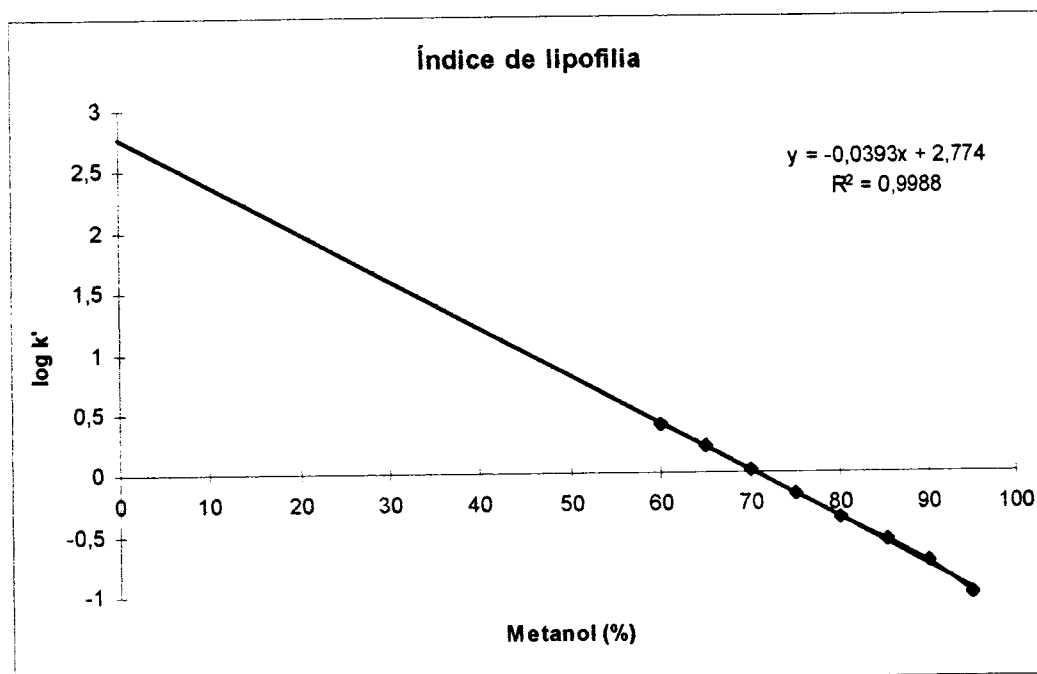
Fig.13 - Índice de lipofilia do naproxeno correspondente às determinações efectuadas com a coluna ODS2, 150x4,6mm, 5 \mu m.
