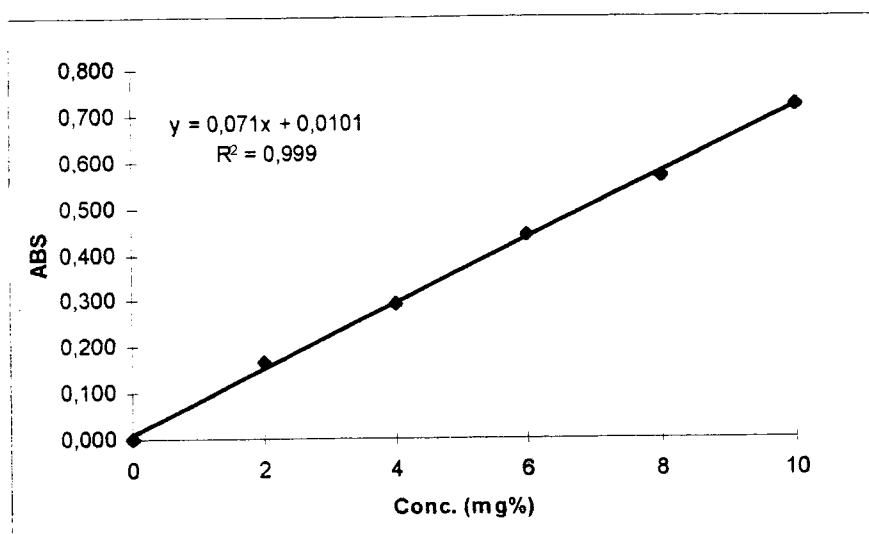
Fig.10 - Correlação entre os valores de absorvência e a concentração de naproxeno.
