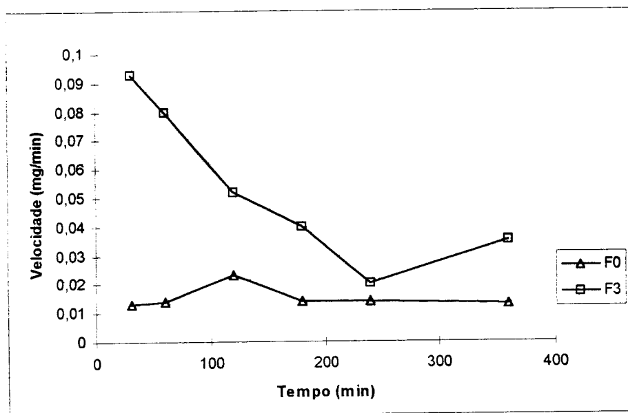
Fig.30 - Velocidade de penetração da F_0 em comparação com a da F_3 .
