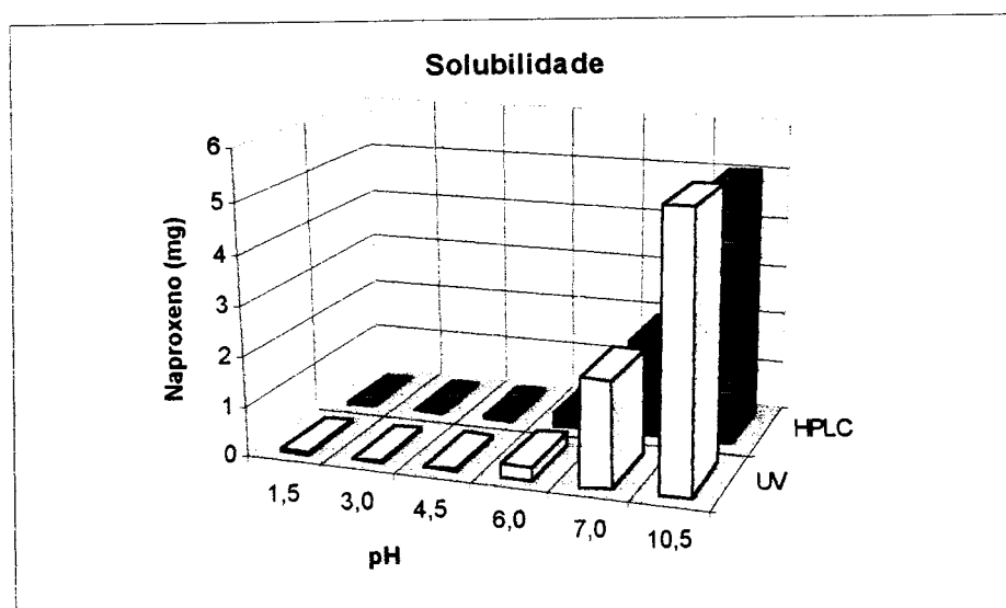
Fig. 12 - Solubilidade do naproxeno em função do pH.
