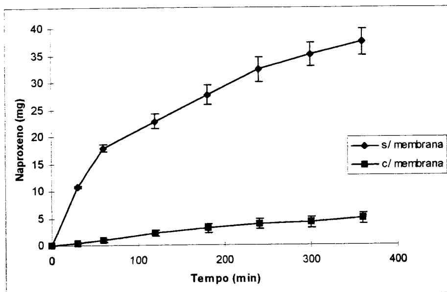
Fig. 21 - Quantidade acumulada de naproxeno detectada na fase receptora nos ensaios realizados com e sem membrana.
