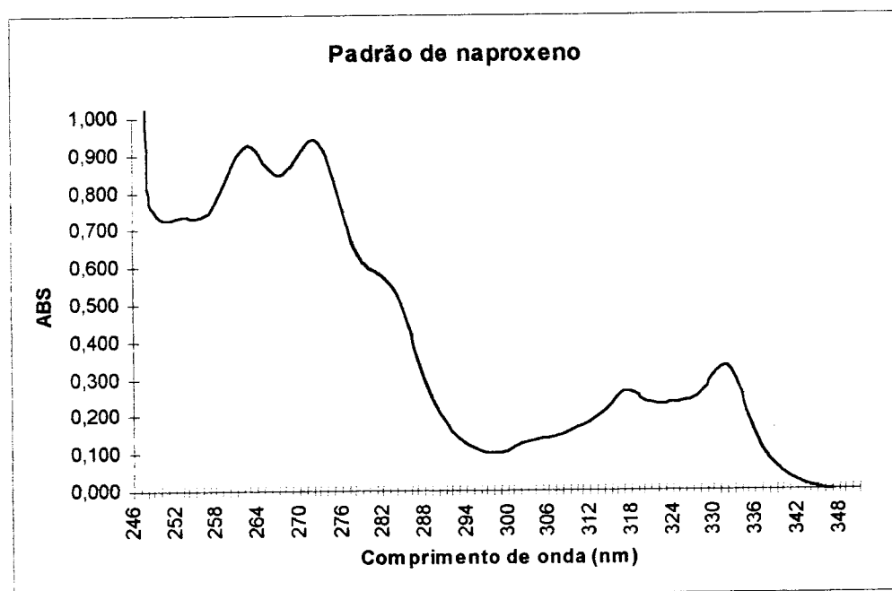
Fig. 6 - Espectro de UV do naproxeno (29).
