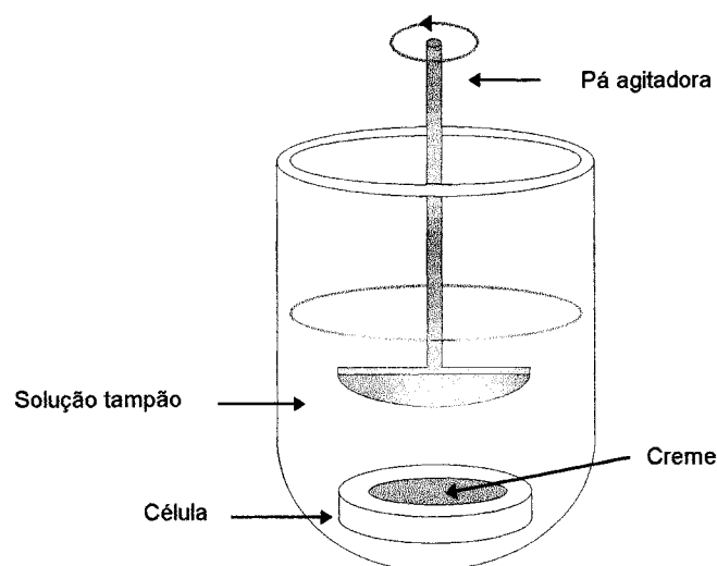
Fig. 15 - Vaso de dissolução adaptado para o ensaio de libertação de formas semi-sólidas.
