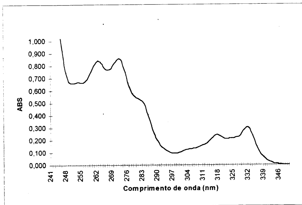
Fig. 5 - Espectro de UV da amostra.
