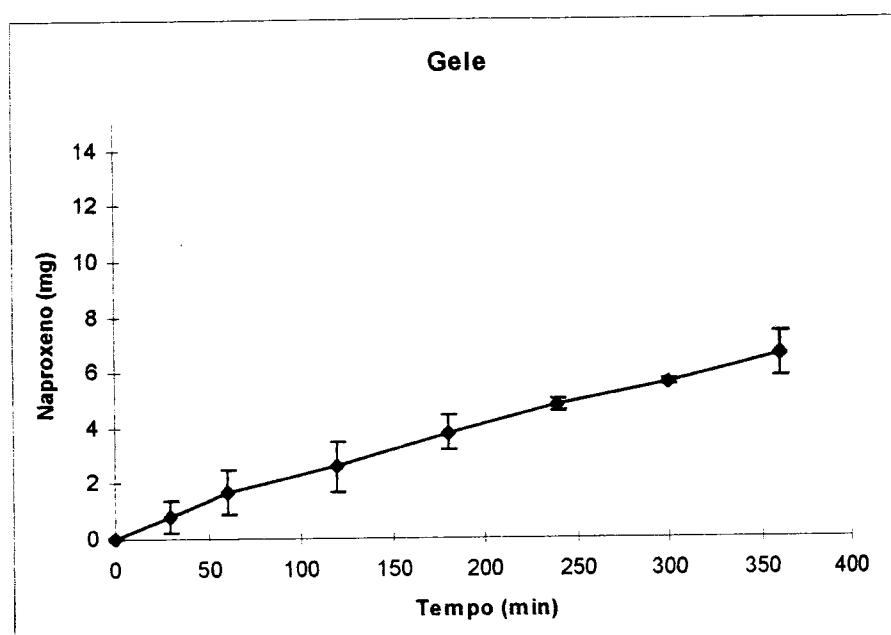
Fig. 31 - Quantidade acumulada de naproxeno contido no gele que difunde em função do tempo.
