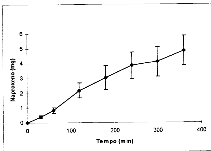
Fig.20 - Quantidade acumulada de naproxeno da F_0 que difunde, em função do tempo.
