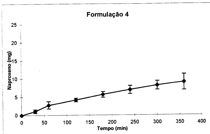
Fig. 27 - Quantidade acumulada de naproxeno da F_4 que difunde.
