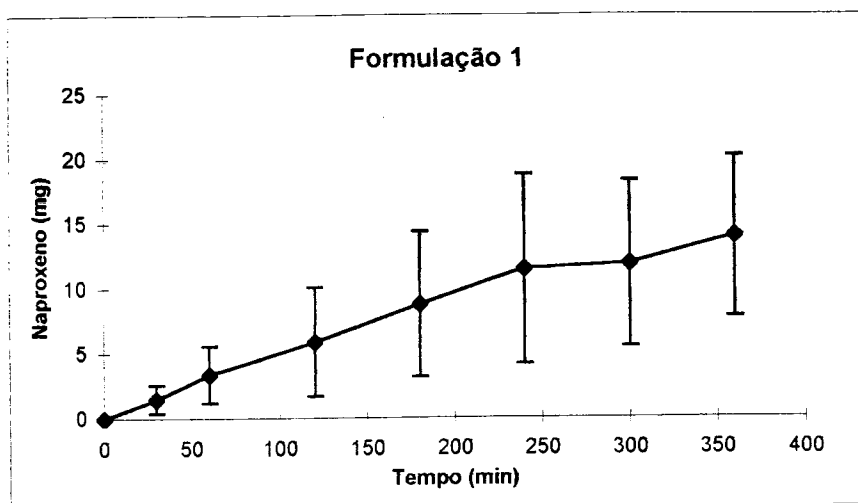
Fig. 24 - Quantidade acumulada de naproxeno da F_1 que difunde.
