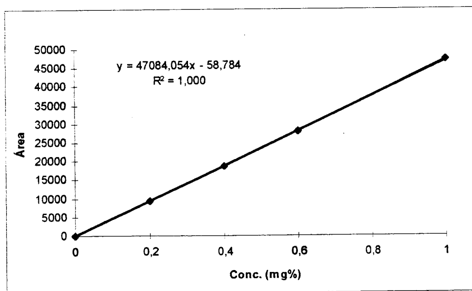
Fig. 9 - Correlação entre a concentração de naproxeno e a área integrada dos picos.
