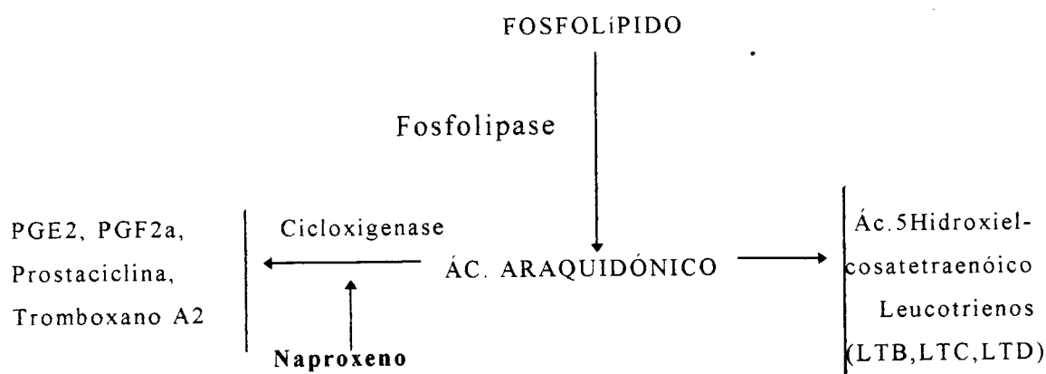
Fig.4-Metabolismo do ácido araquidônico e nível de actuação do naproxeno.
