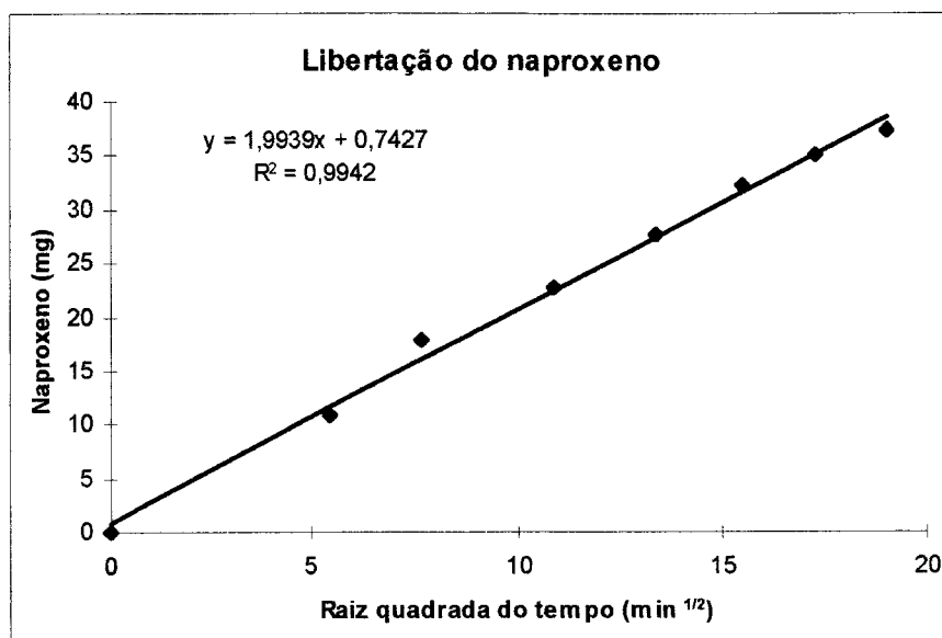
Fig. 17 - Quantidade acumulada de naproxeno libertado em função da raiz quadrada do tempo.
