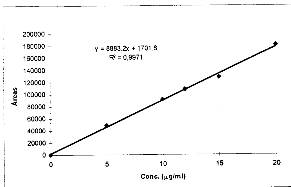
Fig.44 - Correlação entre as áreas correspondentes ao naproxeno recuperado e a concentração do naproxeno adicionado ao soro.
