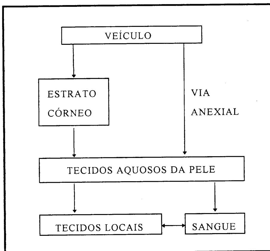
Fig. 2 - Principais vias de permeação cutânea (2).
