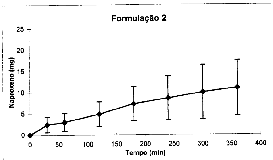
Fig. 25 - Quantidade acumulada de naproxeno da F_2 que difunde.
