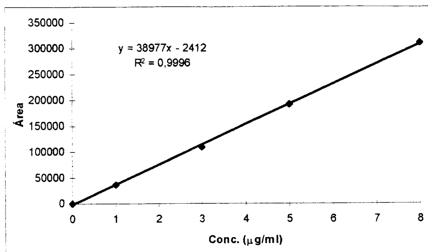
Fig.42 - Correlação entre a concentração de naproxeno e as áreas de pico ( R^2=0,9996 ).
