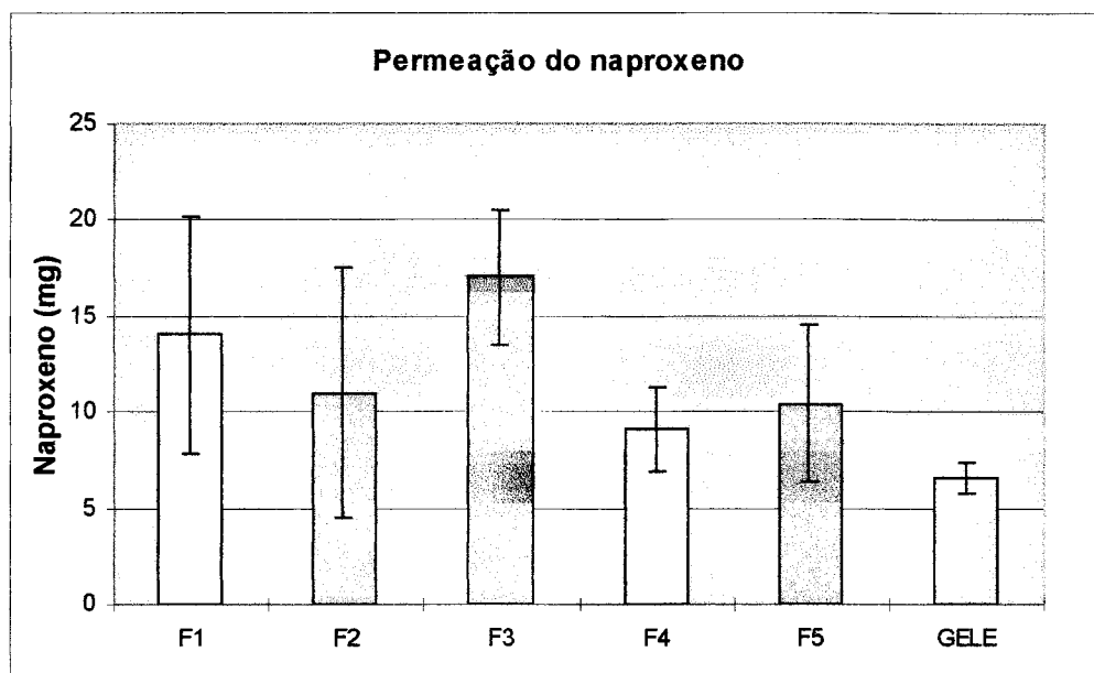
Fig. 32 - Difusão “in vitro” do naproxeno contido num gele comercial ao fim de 6 horas de ensaio, comparativamente com a das diversas fórmulas ensaiadas.
