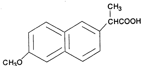
Fig. 3 - Estrutura química do naproxeno
