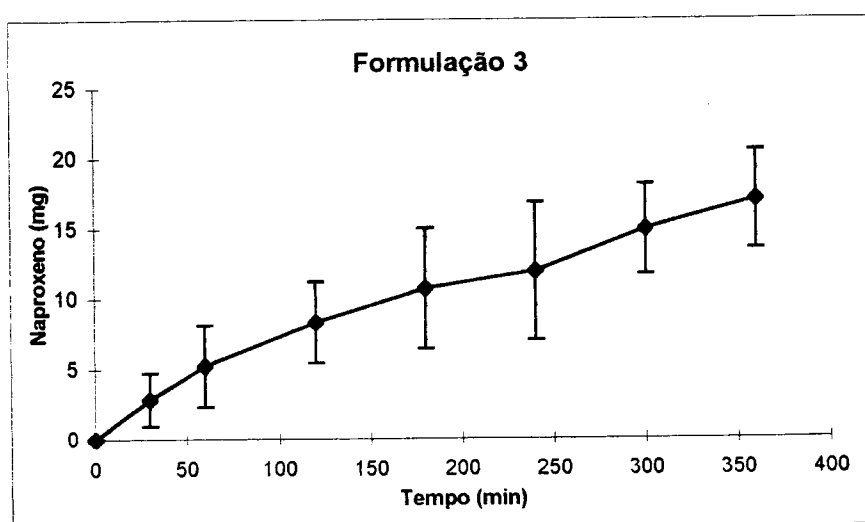
Fig. 26 - Quantidade acumulada de naproxeno da F_3 que difunde.
