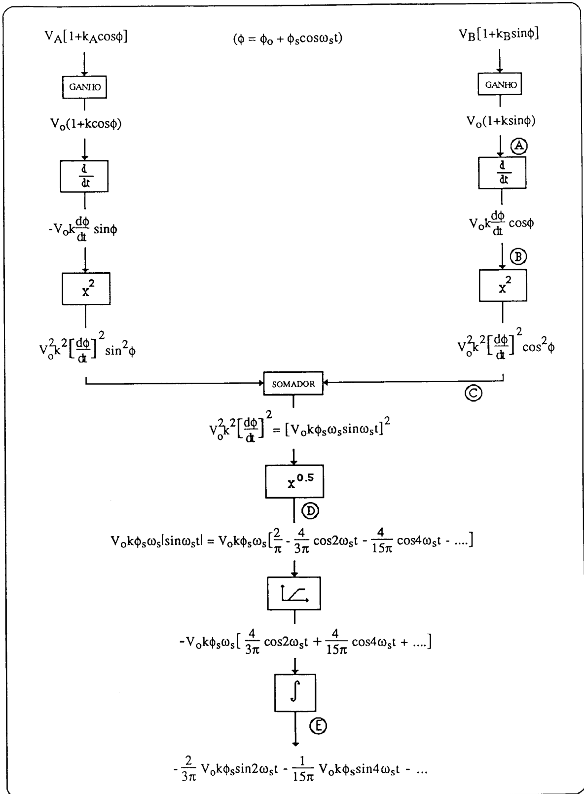
Figura 8.13. Técnica de processamento que permite a leitura de sinais de fase de espectro simples, sem qualquer restrição fundamental sobre o valor da sua amplitude.
