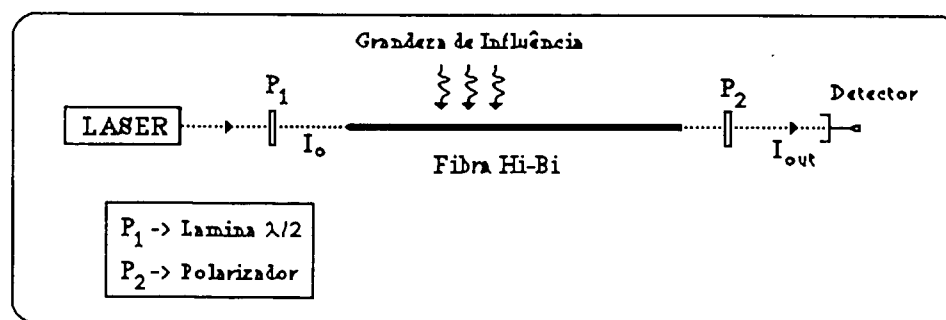
Figura 1.8. Exemplo de um sensor polarimétrico utilizando fibra linearmente birrefringente ("Hi-Bi").
