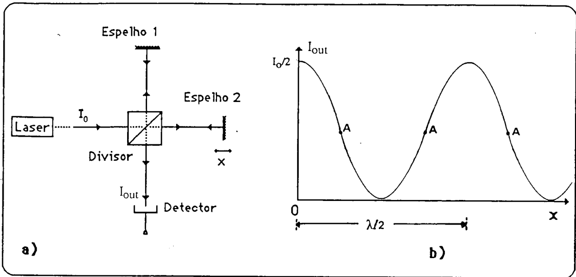
Figura 1.4. Configuração convencional do interferómetro de Michelson e função de transferência para visibilidade unitária (os pontos marcados "A" são designados "pontos de quadratura"; \phi = 4\pi x/\lambda )
