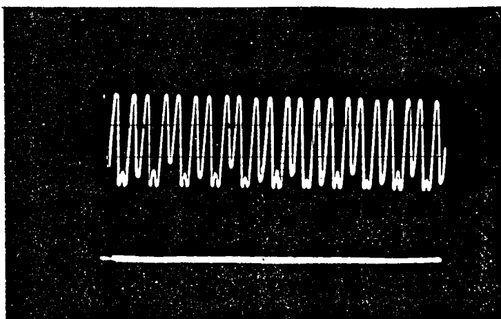
Figura 7.14. Sinal " V_{\text{out}} " com o sistema sintonizado para o sensor "1", ao qual se aplicou um um sinal sinusoidal de fase a 200 Hz com uma amplitude de \approx 3.1 rad (mostra-se igualmente o nível de referência, isto é, V_{\text{out}} = 0 ; escala: 0.2 V/div).
