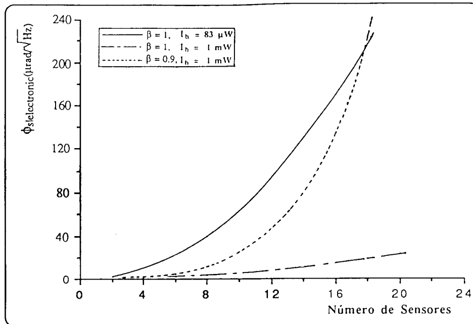
Figura 4.6. Sensibilidade de fase (valor eficaz) determinada pelo ruído electrónico (amplificador bipolar 741), em função do número de sensores ( = 2N ), para os três casos indicados.
