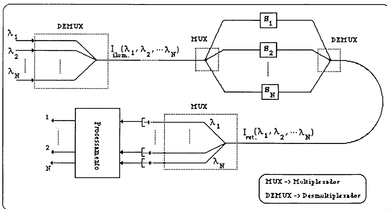
Figura 2.7. Endereçamento no comprimento de onda de sensores numa rede estrela transmissiva utilizando-se o conceito de fontes múltiplas.
