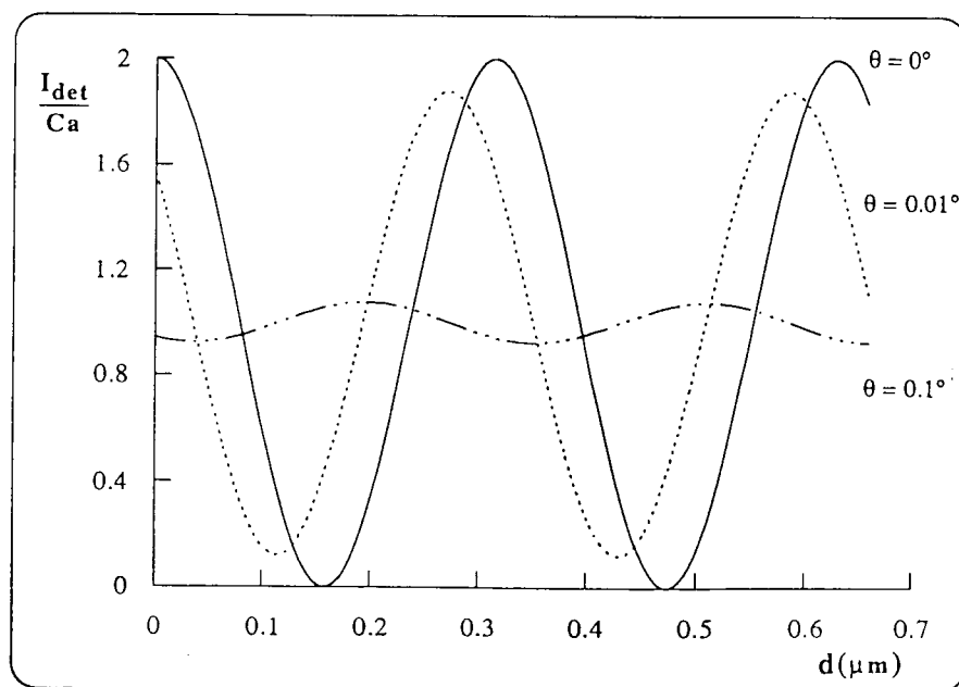
Figura F.3. Dependência da intensidade detectada com " d ".
