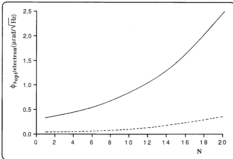
Figura 7.10. Sensibilidade de fase quando se considera somente o ruído electrónico (curva contínua: amplificador bipolar - 741; curva a tracejado: amplificador FET - 725).
