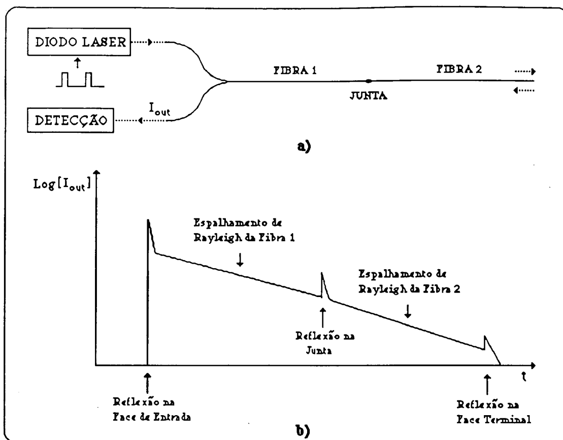
Figura 2.9. a) Implementação da técnica OTDR; b) Dependência temporal de \text{Log}[I_{out}] .
