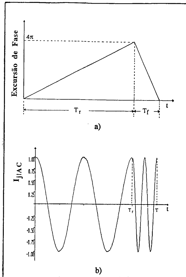
Figura 5.9. a) Forma de onda aplicada ao interferômetro para modulação da fase de 4\pi rad; b) sinal à saída do interferômetro (componente AC; I_{int}V = 1 ).
