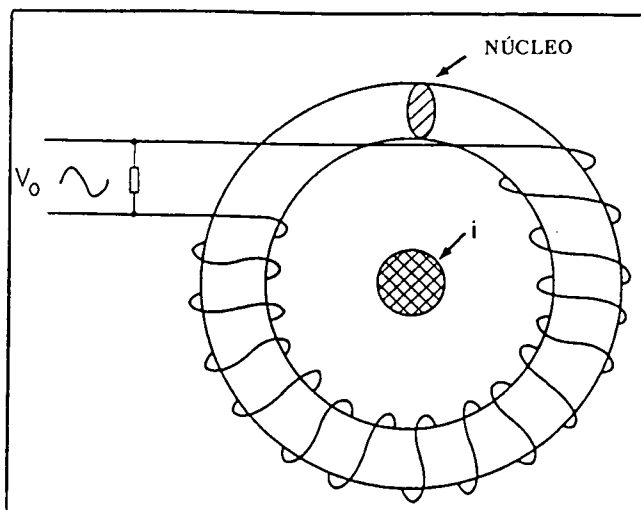
Figura 3.10. Esquema de um transformador de corrente convencional utilizado para a medição de correntes eléctricas elevadas, circulando através do centro do toróide.
