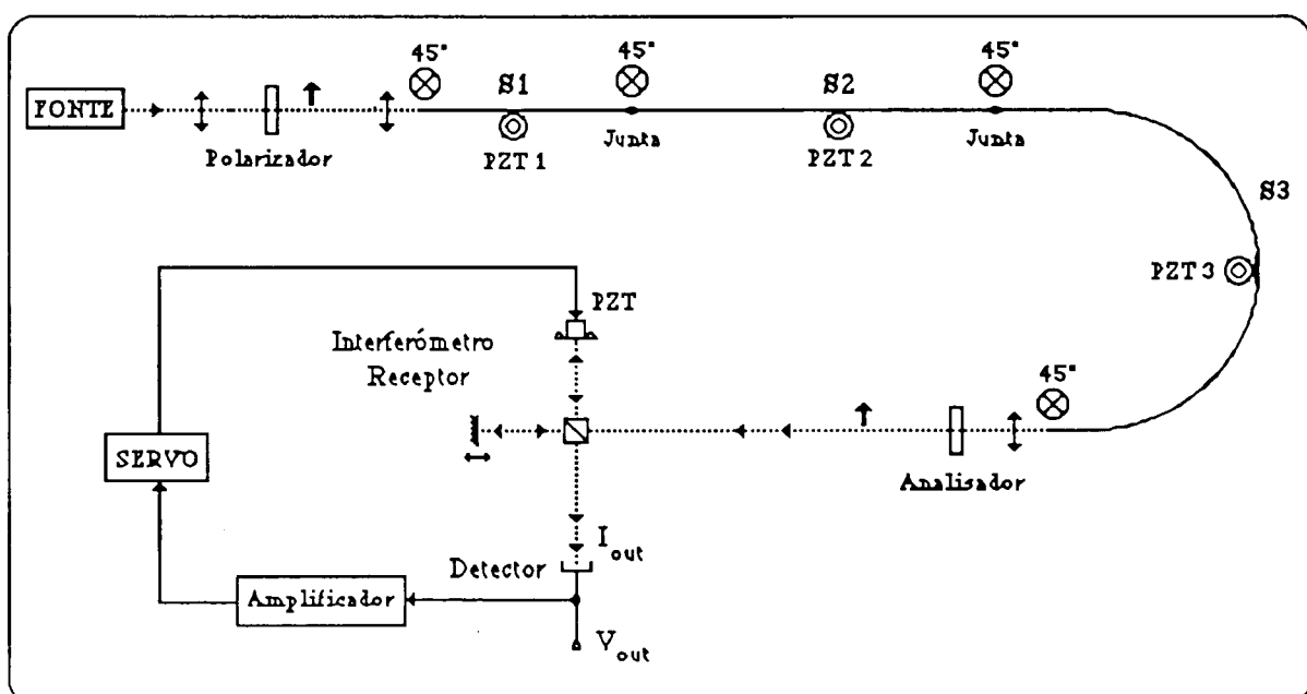
Figura 7.12. Esquema da experiência efectuada.
