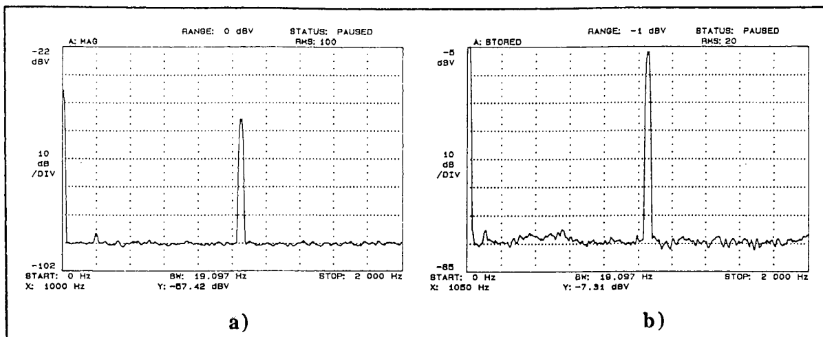
Figura 8.9. Saída do canal "A" ( V_{outA} ) quando um sinal de fase a 1000 Hz foi aplicado ao interferómetro "A", em quadratura: a) amplitude de 5 mrad; b) amplitude de 100 mrad.
