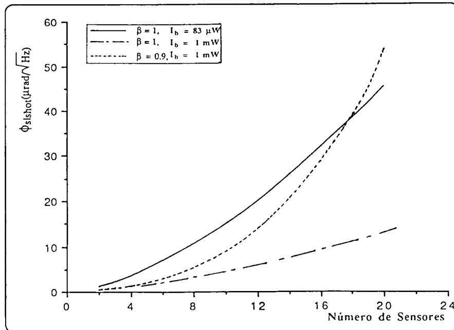
Figura 4.5. Sensibilidade de fase (valor eficaz) determinada pelo ruído quântico, em função do número de sensores da rede ( = 2N ), para os três casos indicados.
