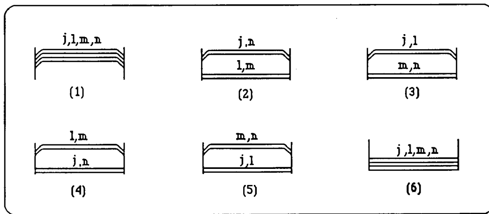
Figura 7.4. Ilustração das possibilidades que satisfazem a condição " T_j - T_\ell = T_n - T_m " em cada interferómetro.
