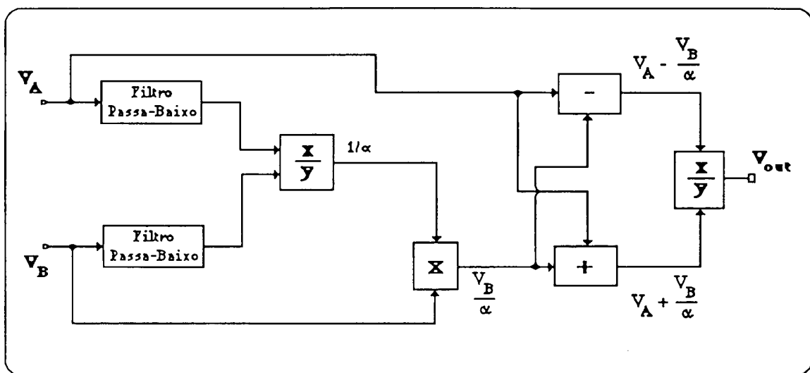
Figura E.1. Esquema do processamento necessário para se eliminar os efeitos da modulação de intensidade da radiação de um laser semiconductor, quando neste actua uma corrente de injeção variável.
