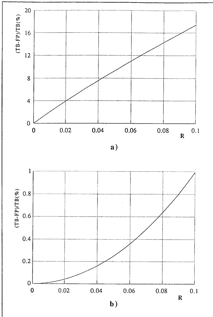
Figura 8.24. Desvio relativo entre a função de transferência de Fabry-Pérot e a função de transferência correspondente à interferência de duas ondas: a) \phi = 2(m+1/2)\pi ; b) \phi = (m+1/2)\pi .
