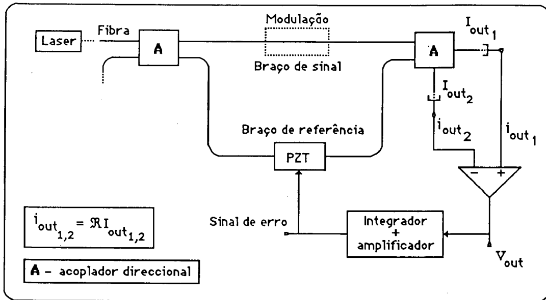
Figura 1.10. Interferómetro de Mach-Zehnder com processamento homodino activo.
