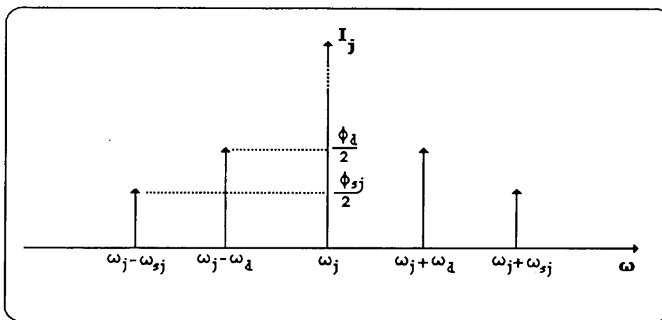
Figura 5.13. Espectro de " I_j " em torno da portadora de frequência " \omega_j " ( \phi_d, \phi_{sj} \ll 1 ).
