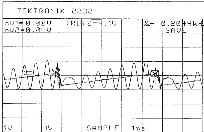
Figura E.2. Sinal de modulação em dente-de-serra da corrente de injeção do laser semiconductor, e a correspondente saída do interferómetro (os dois sinais foram obtidos com escalas verticais distintas).
