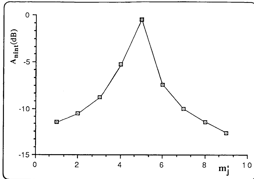
Figura 5.12. "Crosstalk" do sensor "j" ( m_j = 5 ) para outros harmônicos devido à modulação da fase do interferômetro "j" por um número não-inteiro de franjas ( \epsilon = 0.95 , p = m'_j ).
