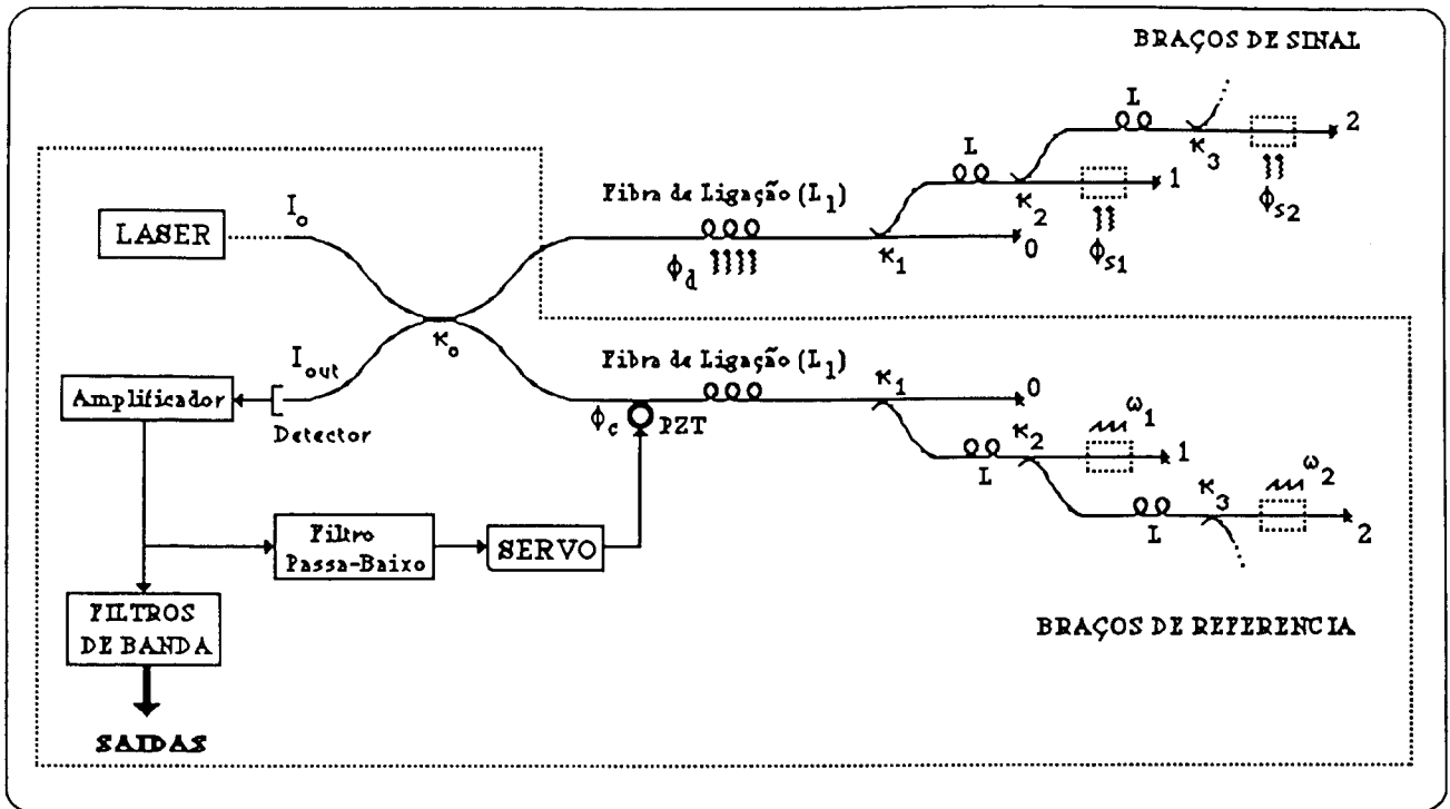
Figura 5.1. Representação do conceito de multiplexagem em frequência de sensores interferométricos (interferômetros de Michelson) com insensibilidade a perturbações induzidas nas fibras de ligação.
