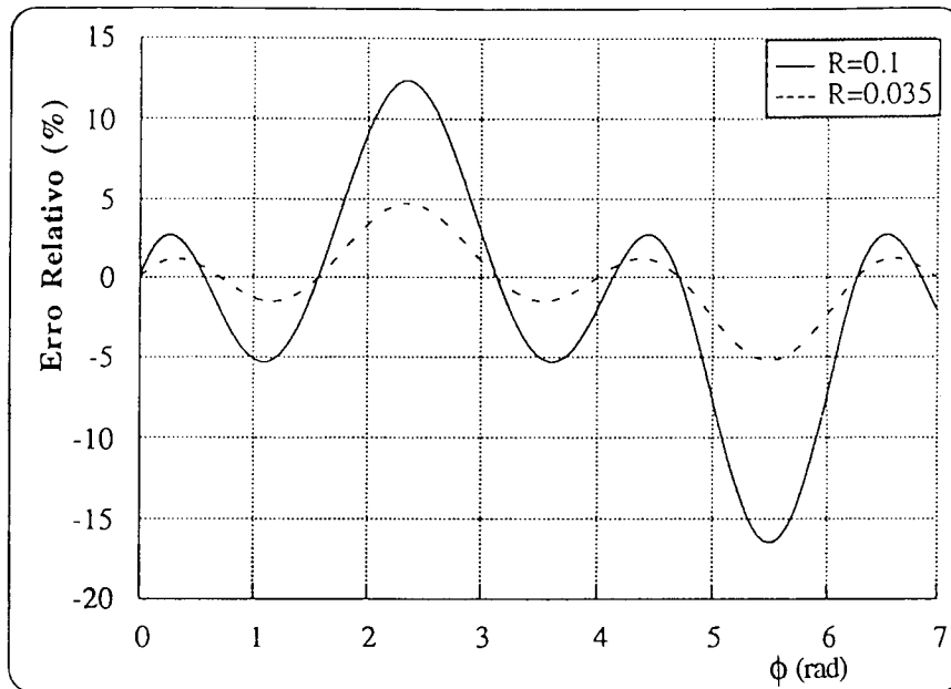
Figura 8.28. Erro de escala introduzido pela técnica de desmodulação "Soma dos Quadrados" ao processar a função de transferência de Fabry-Pérot.
