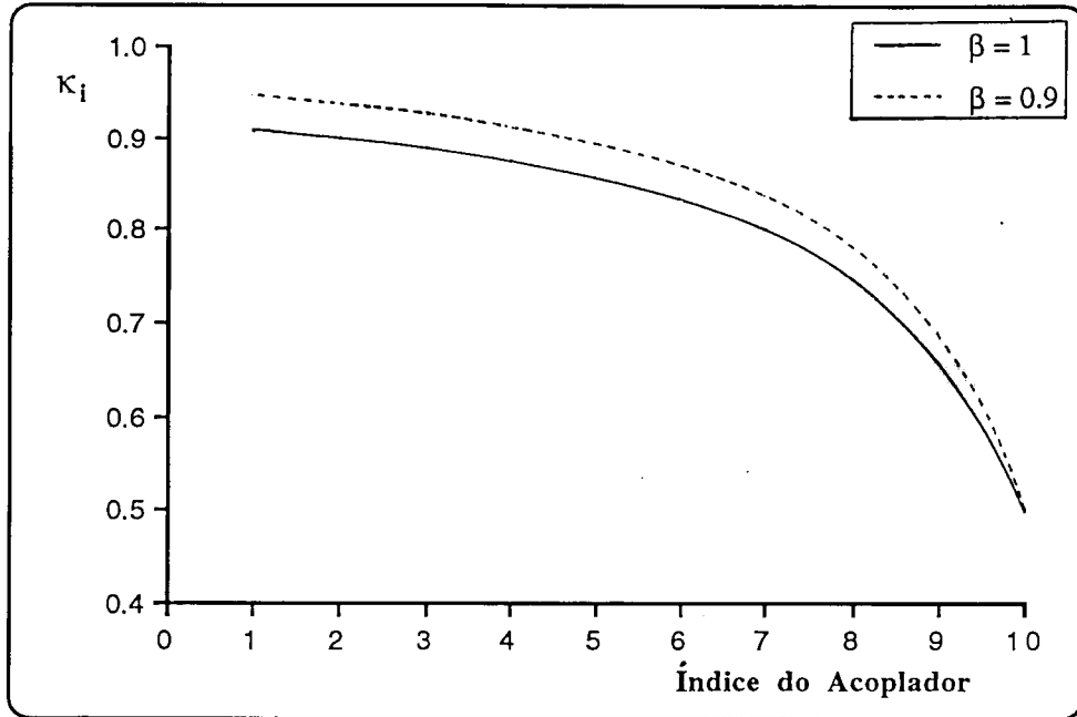
Figura 5.2. Factor de divisão de potência dos acopladores direccionais nos ramos de sinal e de referência, em função da sua posição ao longo destes. Considera-se N = 10 , e representa-se os casos de ausência de perdas ( \beta = 1 ) e de perda de 0.45 dB por acoplador ( \beta = 0.9 ).
