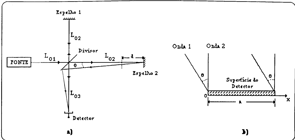
Figura F.1. Representação esquemática do desalinhamento das duas ondas que interferem num interferômetro de Michelson convencional (em b representa-se a orientação das duas ondas relativamente à superfície do detector).
