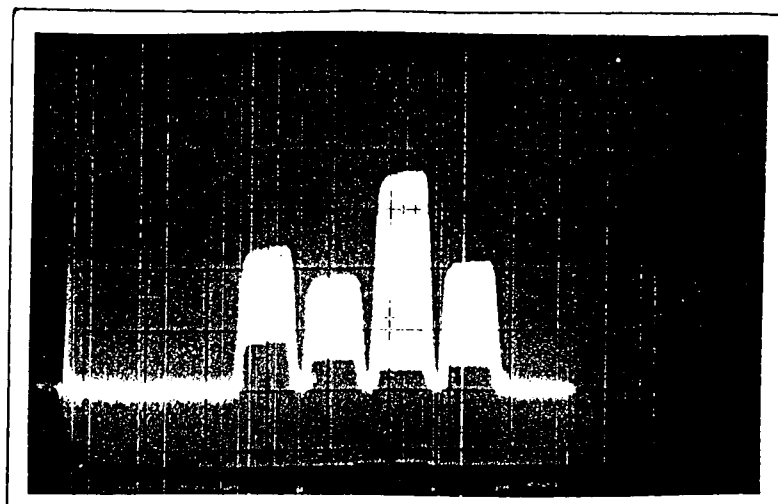
Figura 3.5. Trem de impulsos proveniente dos sensores da rede (1V/div; 1 \mu s/div).
