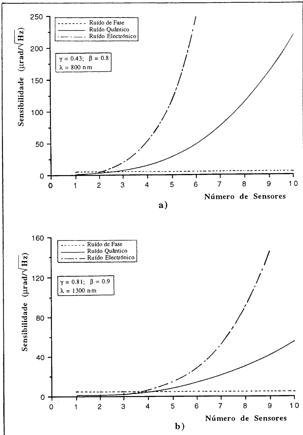
Figura 6.9. Sensibilidade dos sensores da rede, determinada por cada uma das fontes de ruído, quando se considera a utilização de um detector p-i-n: a) operação a 800 \text{ nm} ; b) operação a 1300 \text{ nm} (atendendo a que o ruído electrónico é dominante, a sensibilidade que se obtém quando se considera todas as fontes de ruído é virtualmente idêntica à conseguida quando se tem somente o ruído electrónico).
