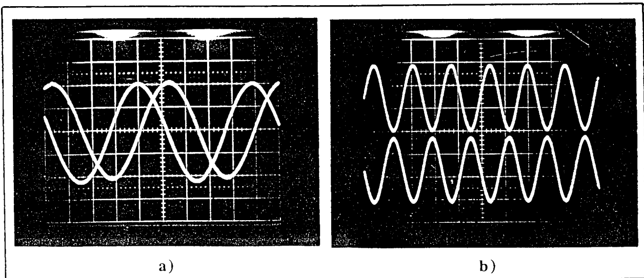
Figura 8.6. Portadoras dos interferómetros "A" e "B": a) \phi_A - \phi_B = \pi/2 (módulo 2\pi ); b) \phi_A - \phi_B = \pi (módulo 2\pi ).
