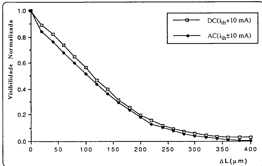
Figura 6.5. Visibilidade das franjas no padrão central de interferência para os casos representados na Fig 6.3.
