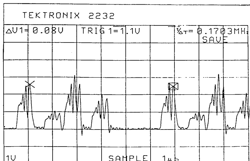
Figura 3.6. Sequência de impulsos à saída do sistema quando a modulação da radiação é efectuada através da modulação da corrente de injeção do laser semiconductor.
