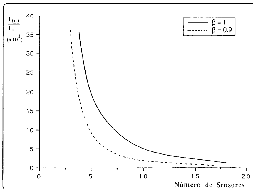
Figura 4.4. Potência óptica média de retorno de cada sensor da rede, normalizada pela potência óptica média injectada no sistema. Considera-se dois casos: ausência de perdas ( \beta = 1 ); perda de 0.45 dB por acoplador ( \beta = 0.9 ).
