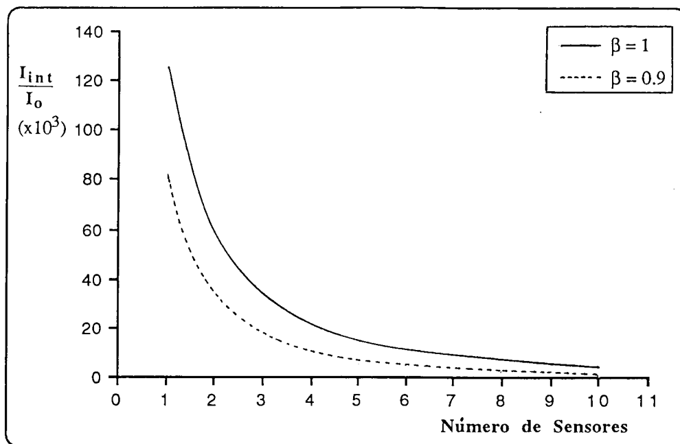
Figura 5.3. Potência óptica média de retorno de cada interferómetro, normalizada pela potência óptica média injectada no sistema. Considera-se os casos \beta = 1 e \beta = 0.9 .
