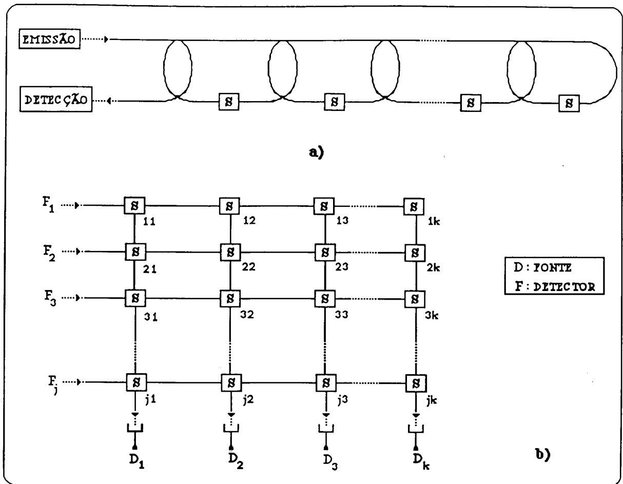
Figura 2.3. Exemplos de estruturas topológicas alternativas para redes de sensores:
