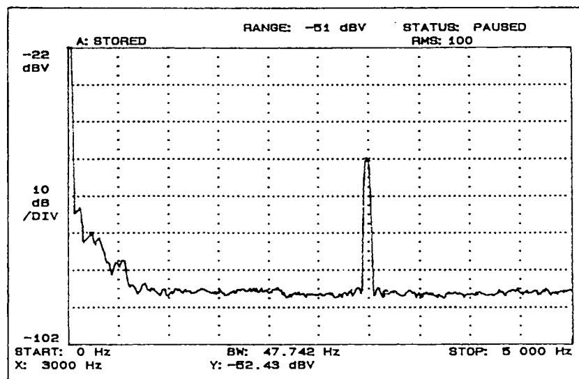
Figura 6.17. Sinal " V_{out} " sem o isolador óptico, estando o sistema sintonizado para o sensor "A", ao qual se aplicou um sinal de 10 mrad de amplitude a 3 kHz.
