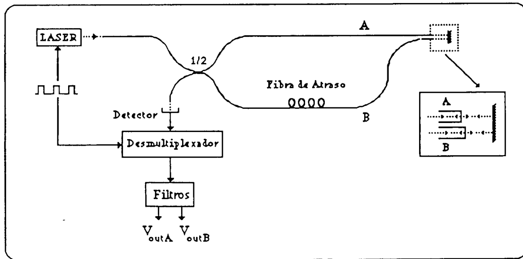
Figura 8.1. Esquema que ilustra a geração de dois sinais interferométricos, os quais variam em quadratura.
