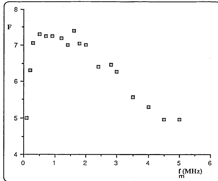
Figura 5.23. Factor de redução do nível de ruído do sistema, em função da frequência da corrente de modulação (mantida a amplitude constante: 2.3 mA).
