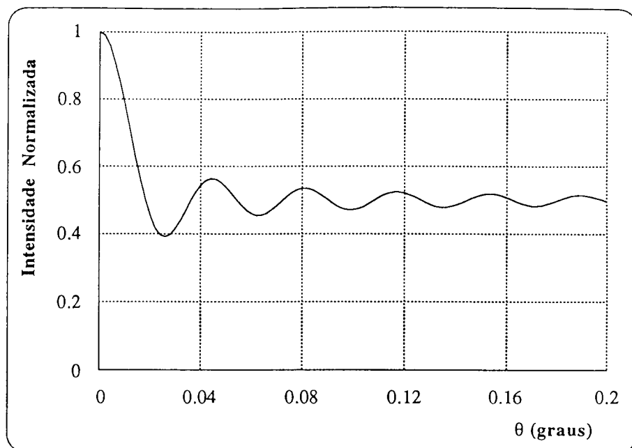
Figura F.2. Dependência da intensidade detectada com o desalinhamento " \theta " do espelho (" d " constante).
