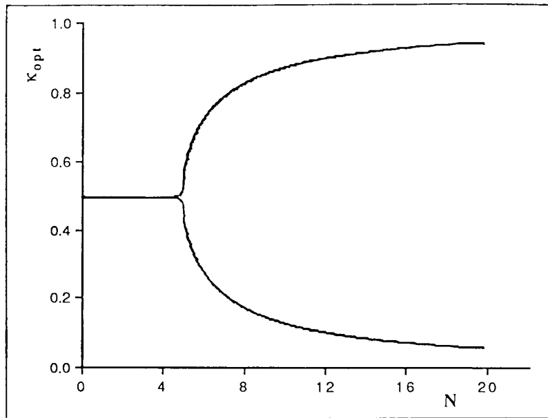
Figura 7.7. Valores de " \kappa " que minimizam " \phi_{\text{sfonte}} ".
