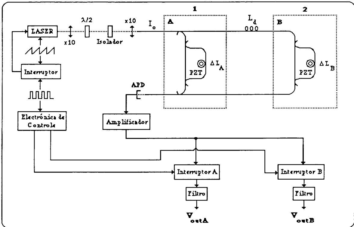
Figura 4.8. Esquema da experiência efectuada.
