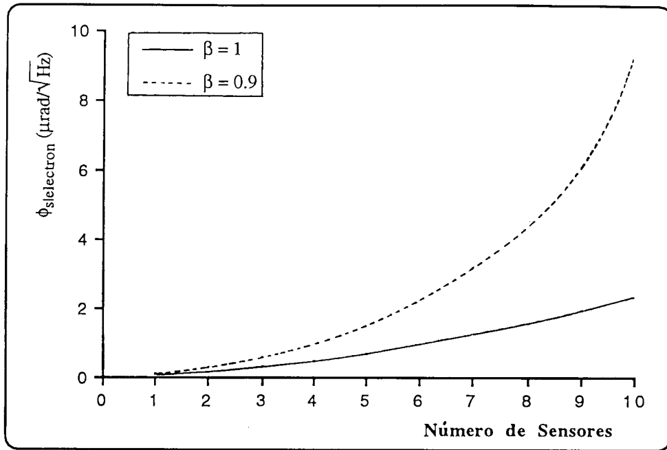
Figura 5.5. Sensibilidade de fase determinada pelo ruído electrónico, em função do número de sensores da rede. Considera-se os casos \beta = 1 e \beta = 0.9 .
