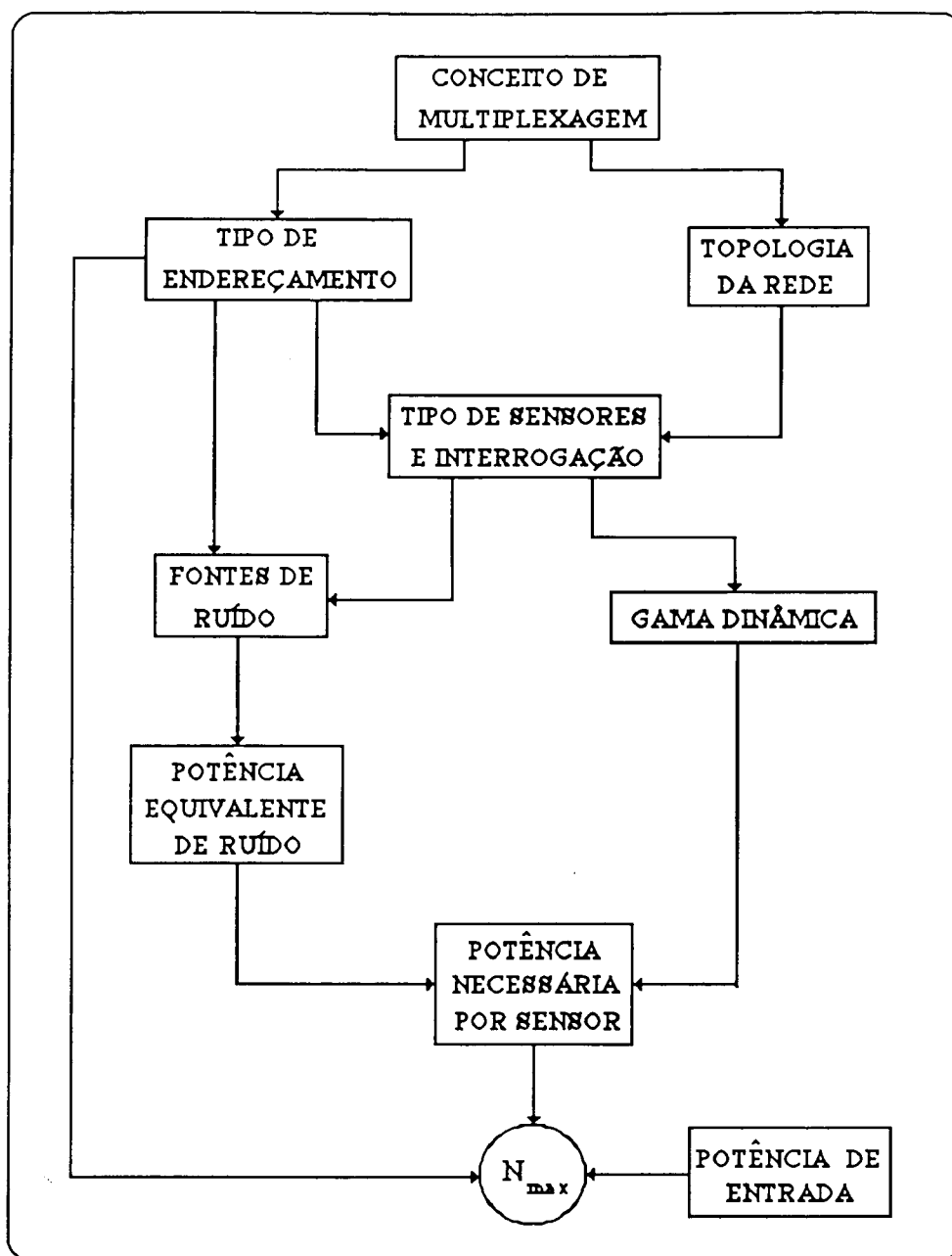
Figura 2.8. Interdependência entre as várias características da rede de sensores que determinam o número máximo de sensores, " N_{max} ", que podem ser multiplexados.
