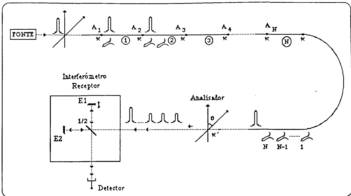
Figura 7.1. Diagrama da configuração de multiplexagem, em que sensores polarimétricos distribuídos em série são endereçados em coerência (somente uma fracção das ondas - representadas como impulsos - é mostrada na figura).
