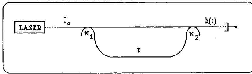
Figura D.1. Interferômetro de duas ondas (Mach-Zehnder em fibra).
