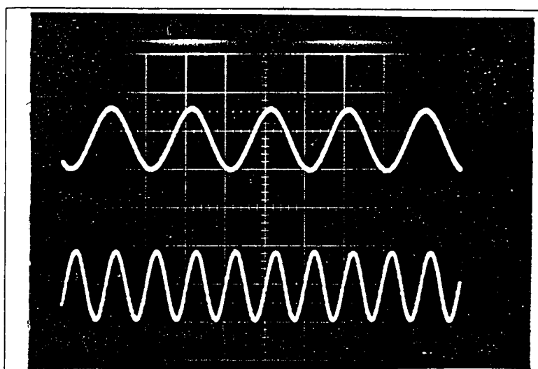
Figura 4.12. Portadoras geradas pela técnica pseudo-heterodina (0.1 ms/div; 0.2 V/div): cima: portadora do interferómetro "B" (5 kHz); baixo: portadora do interferómetro "A" (10 kHz); relativamente ao de cima este sinal tem um ganho adicional de \approx 20 dB.
