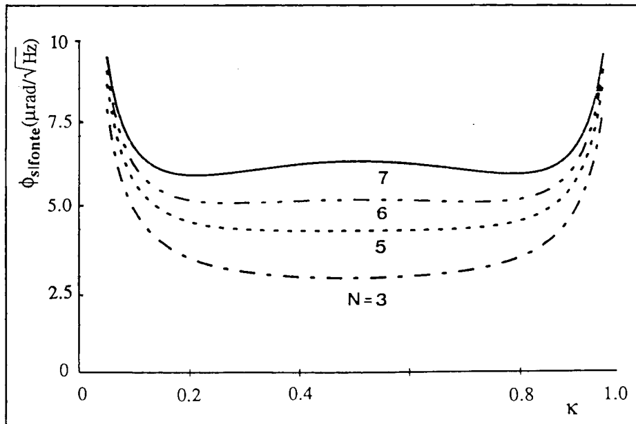
Figura 7.6. Fase mínima detectável, em função de " \kappa ", quando se considera somente o ruído da fonte, tendo como parâmetro o número de sensores.
