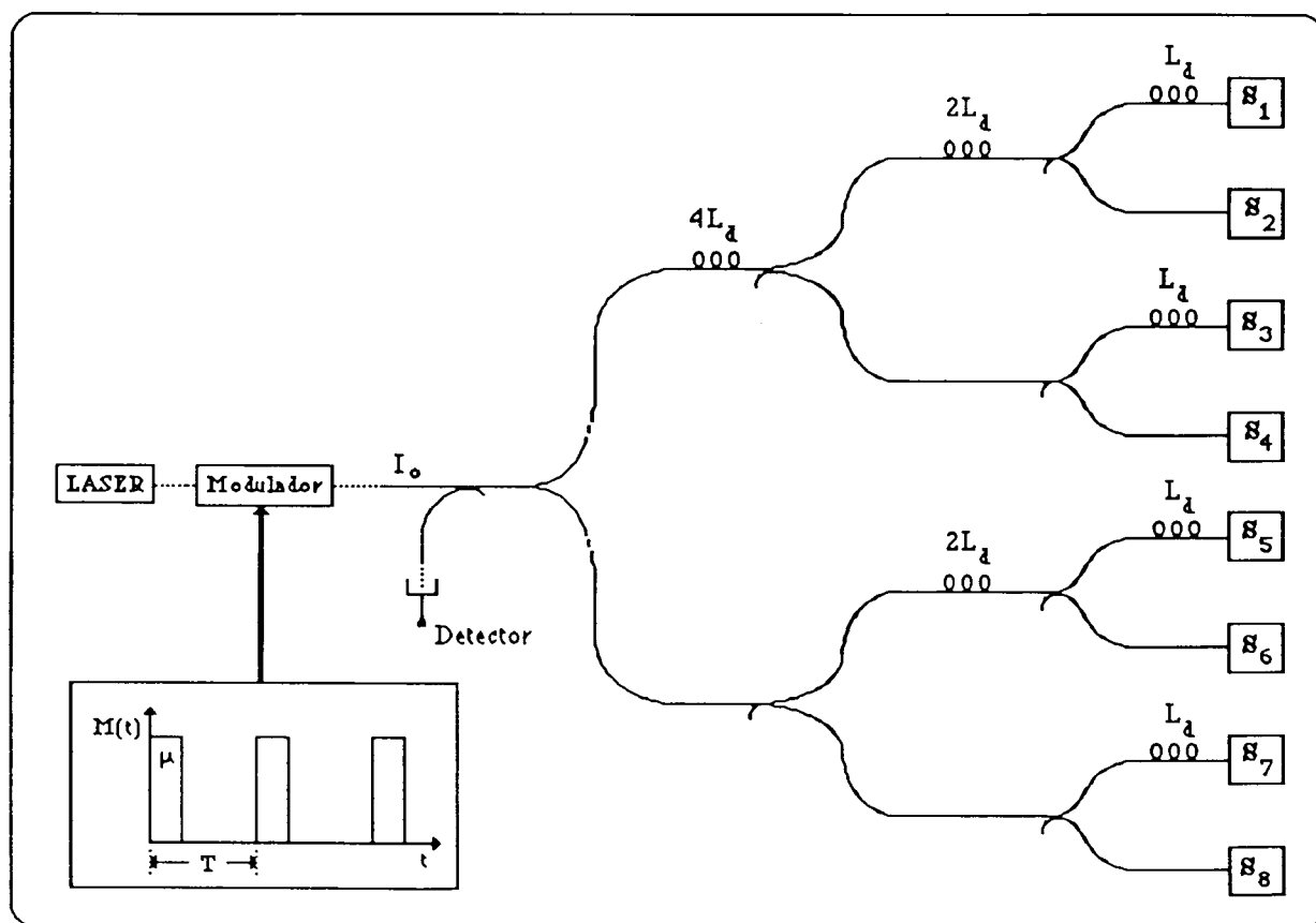
Figura 3.1. Endereçamento temporal de sensores distribuídos numa topologia em árvore (o coeficiente de divisão nominal dos acopladores é 1/2).
