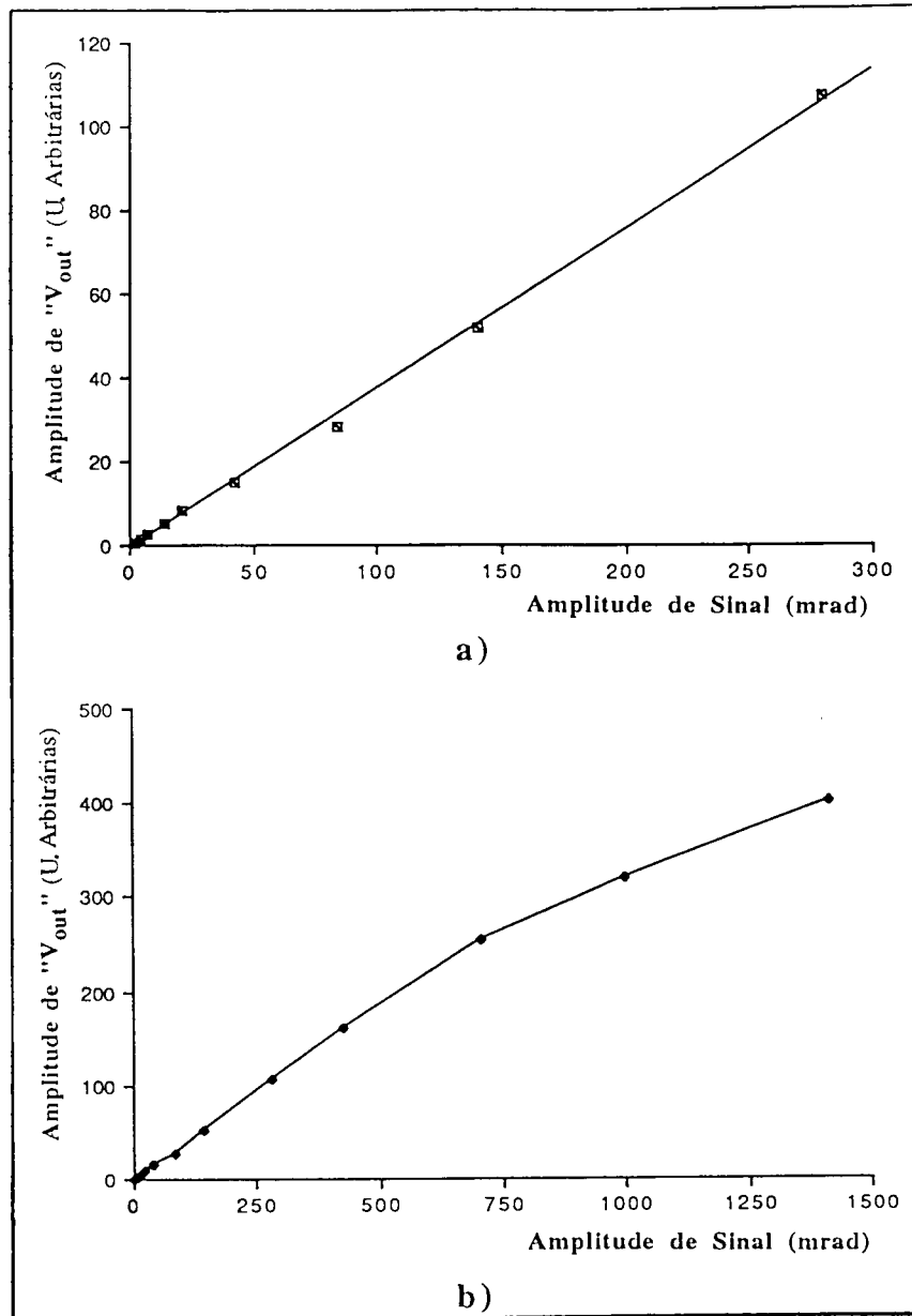
Figura 8.12. Amplitude de "V out " em função da amplitude do sinal de fase aplicado à cavidade. a) 0 \leq \phi_s < 0.3 rad; b) 0 \leq \phi_s < 1.5 rad.
