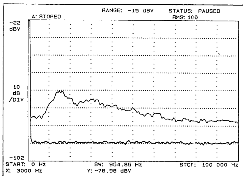
Figura 3.9. Saída do canal 1 com nenhum sinal aplicado ao sensor 1; a curva superior diz respeito ao ruído total do sistema (electrónico + óptico); a curva inferior corresponde à situação em que a radiação é impedida de atingir o detector (nível de ruído determinado pelo ruído electrónico).
