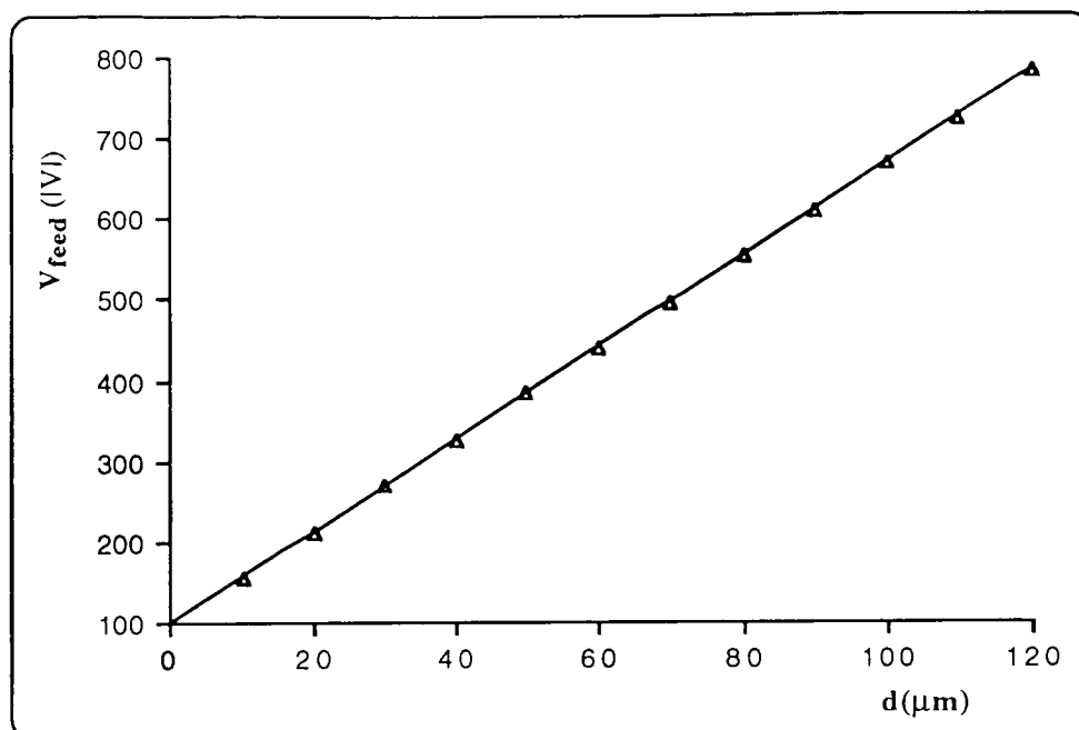
Figura 6.19. Variação da tensão " V_{feed} " em função do deslocamento " d " induzido num dos espelhos do interferómetro receptor, quando o sistema se encontra sintonizado para o sensor "A".
