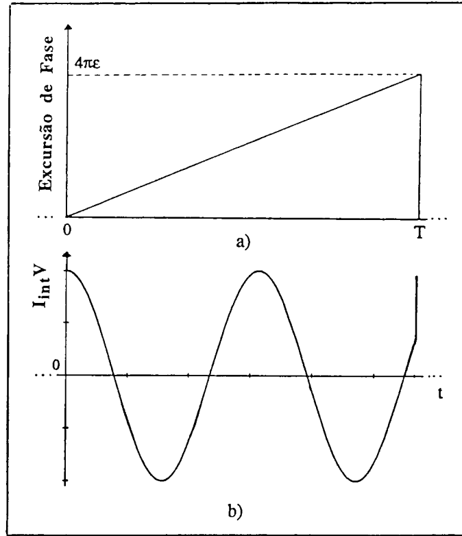
Figura 5.11. a) Forma de onda de fase aplicada ao interferómetro para uma modulação de "2ε" franjas (ε = 0.9); b) saída do interferómetro (componente AC).
