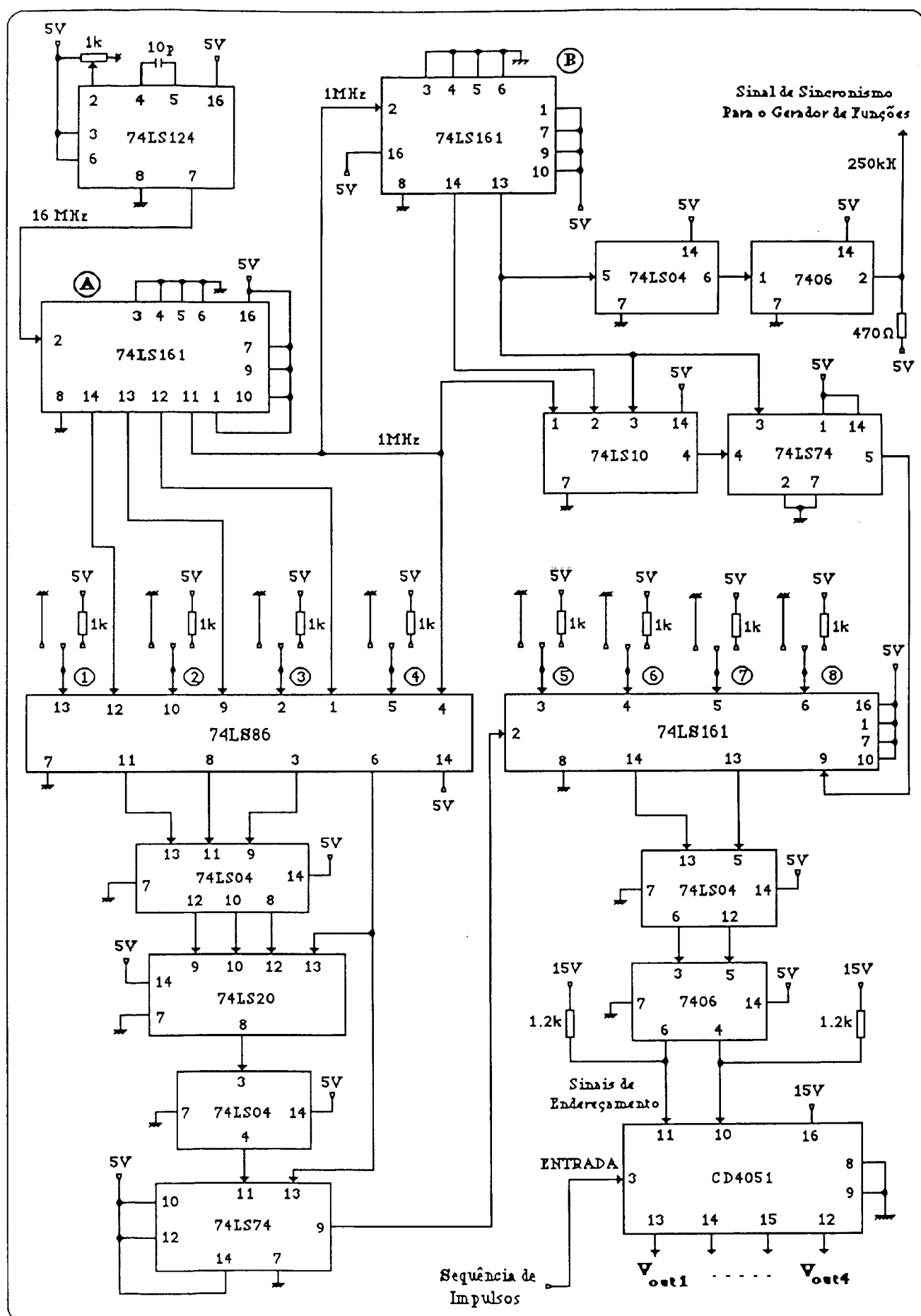
Figura C.2. Esquema do desmultiplexador de quatro canais.
