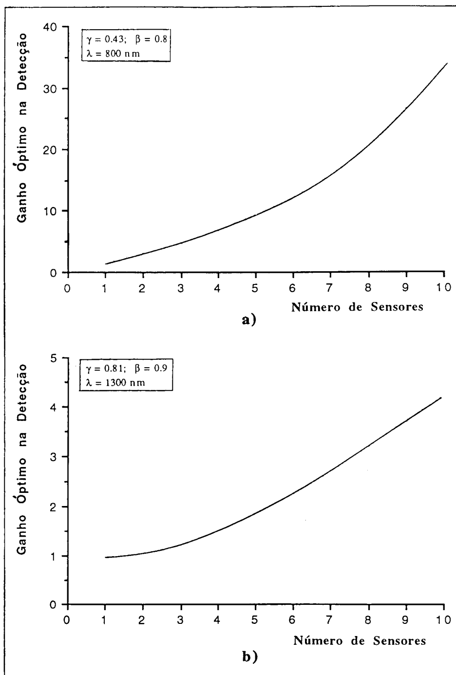
Figura 6.10. Ganho na detecção que otimiza a sensibilidade dos sensores da rede: a) operação a 800 nm; b) operação a 1300 nm.
