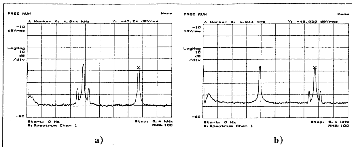
Figura 5.20. Portadoras dos interferómetros "1" e "2" geradas através da modulação da corrente de injeção do laser semiconductor, juntamente com sinais de teste ( f = 250 Hz, B = 64 Hz):
