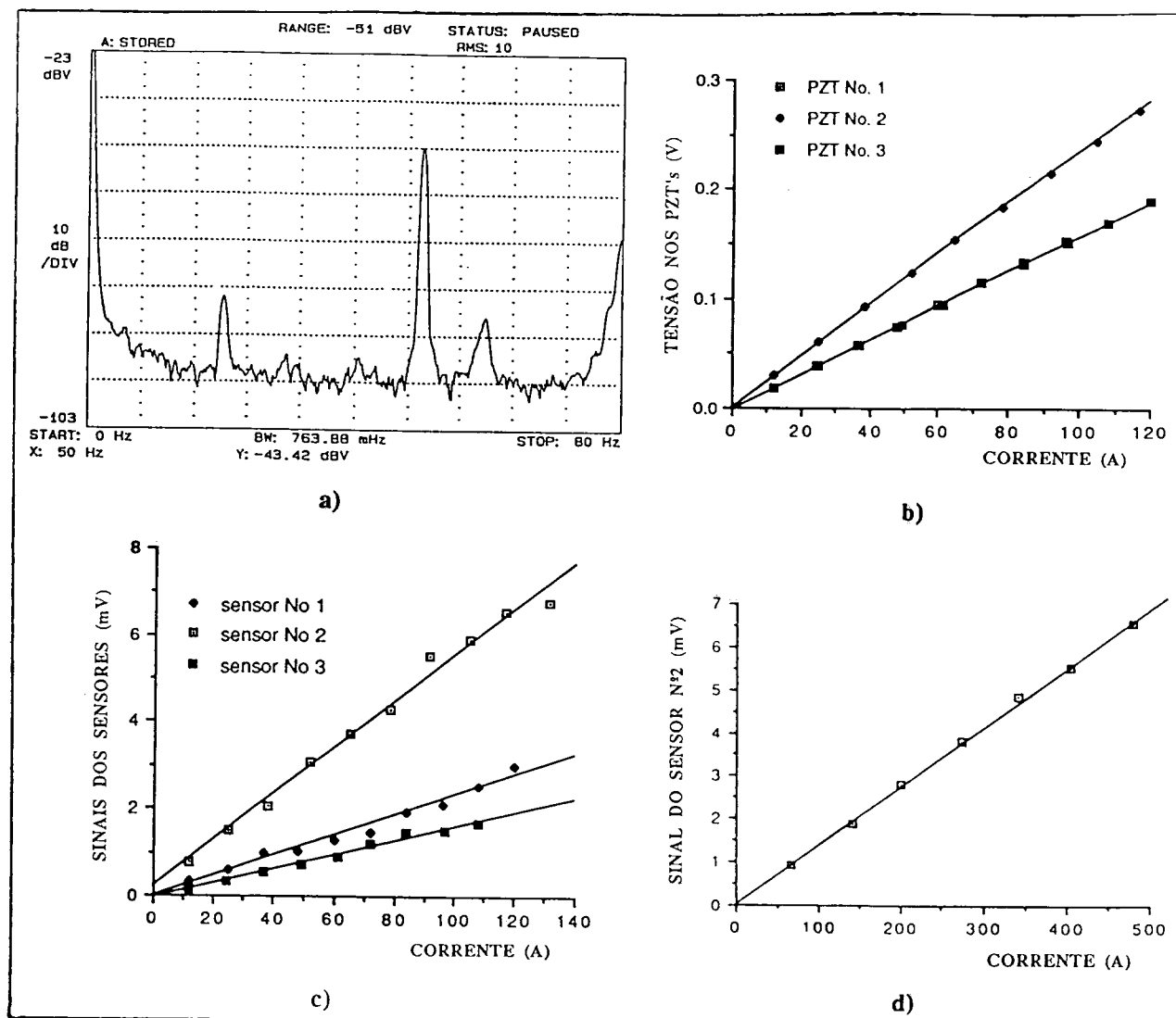
Figura 3.12. a) Saída do canal 2 quando é aplicado ao sensor 2 uma corrente eléctrica correspondente à indução de um sinal de fase com amplitude de 100 mrad a 50 Hz; b) tensão aplicada a cada um dos PZT's em função da corrente que atravessa o respectivo TC; c) amplitude dos sinais à saída de cada um dos canais do desmultiplexador, em função da corrente eléctrica aplicada a cada sensor; d) saída do canal 2 com o sensor 2 configurado para a detecção de correntes mais elevadas.
