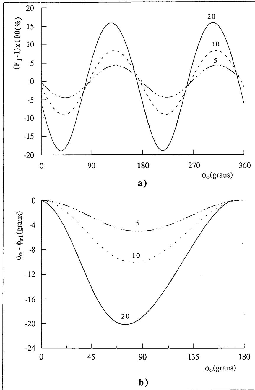
Figura 8.19. Erro de escala (a) e erro na leitura de fase (b) introduzidos pela técnica de processamento "Desvio de Fase" quando os dois sinais interferométricos não variam em quadratura. As curvas são apresentadas para \Delta\phi = 5^\circ, 10^\circ e 20^\circ .
