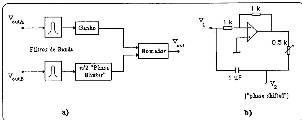
Figura 8.10. a) Esquema de processamento; b) Detalhe do "Phase Shifter".
