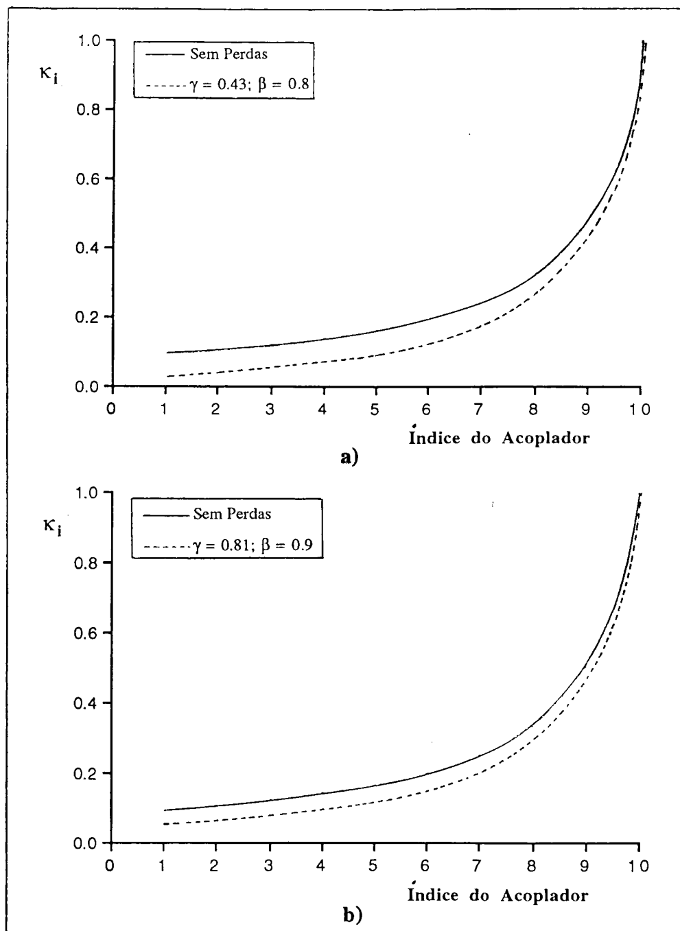
Figura 6.7. Factor de divisão de potência dos acopladores direccionais em função da sua posição ao longo da rede. Considera-se N = 10 e os casos sem e com perdas de potência. a) operação a 800 nm; b) operação a 1300 nm.
