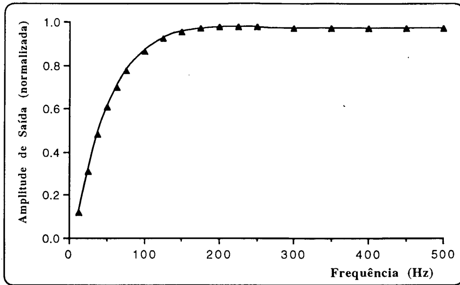
Figura 8.18. Resposta em frequência do sistema.
