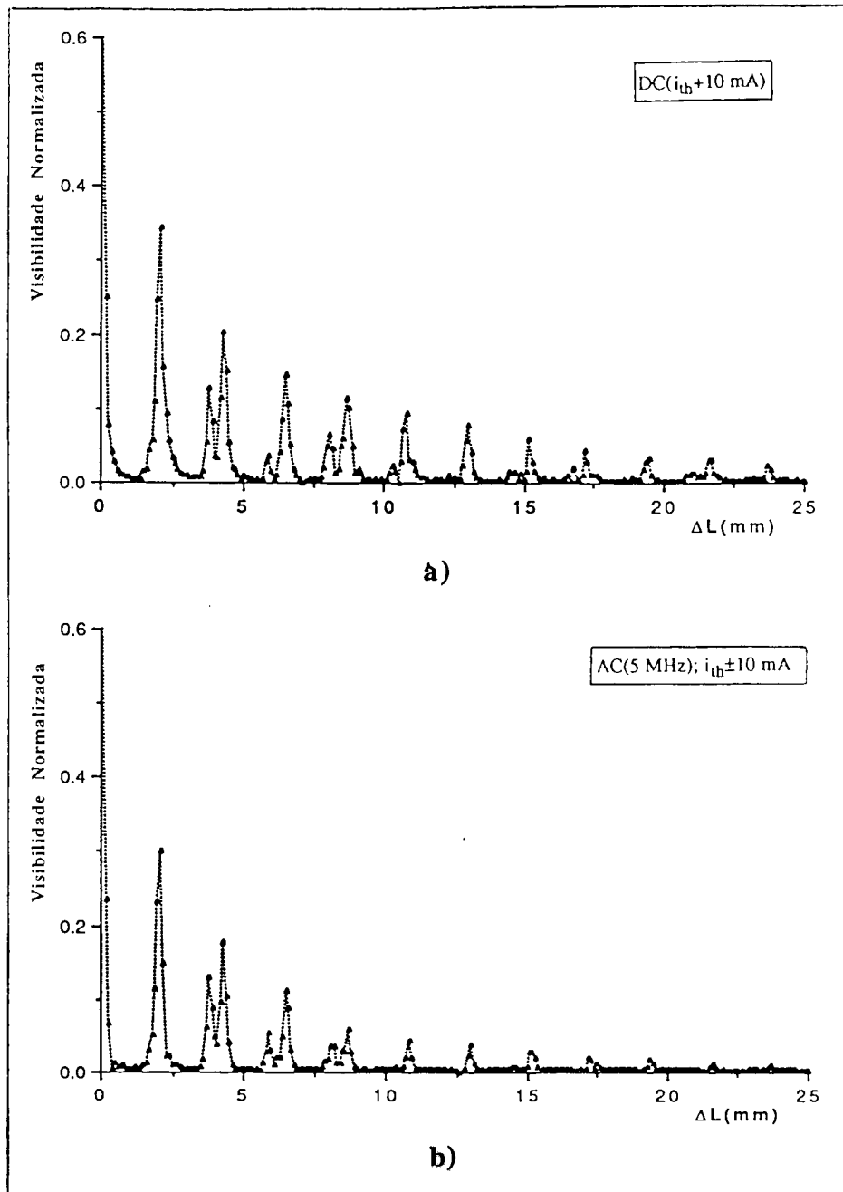
Figura 6.3. Visibilidade das franjas em função do não-balanceamento do interferômetro: a) laser operado em contínuo; b) laser modulado por intermédio de uma onda quadrada de frequência 5 MHz aplicada à sua corrente de injeção.
