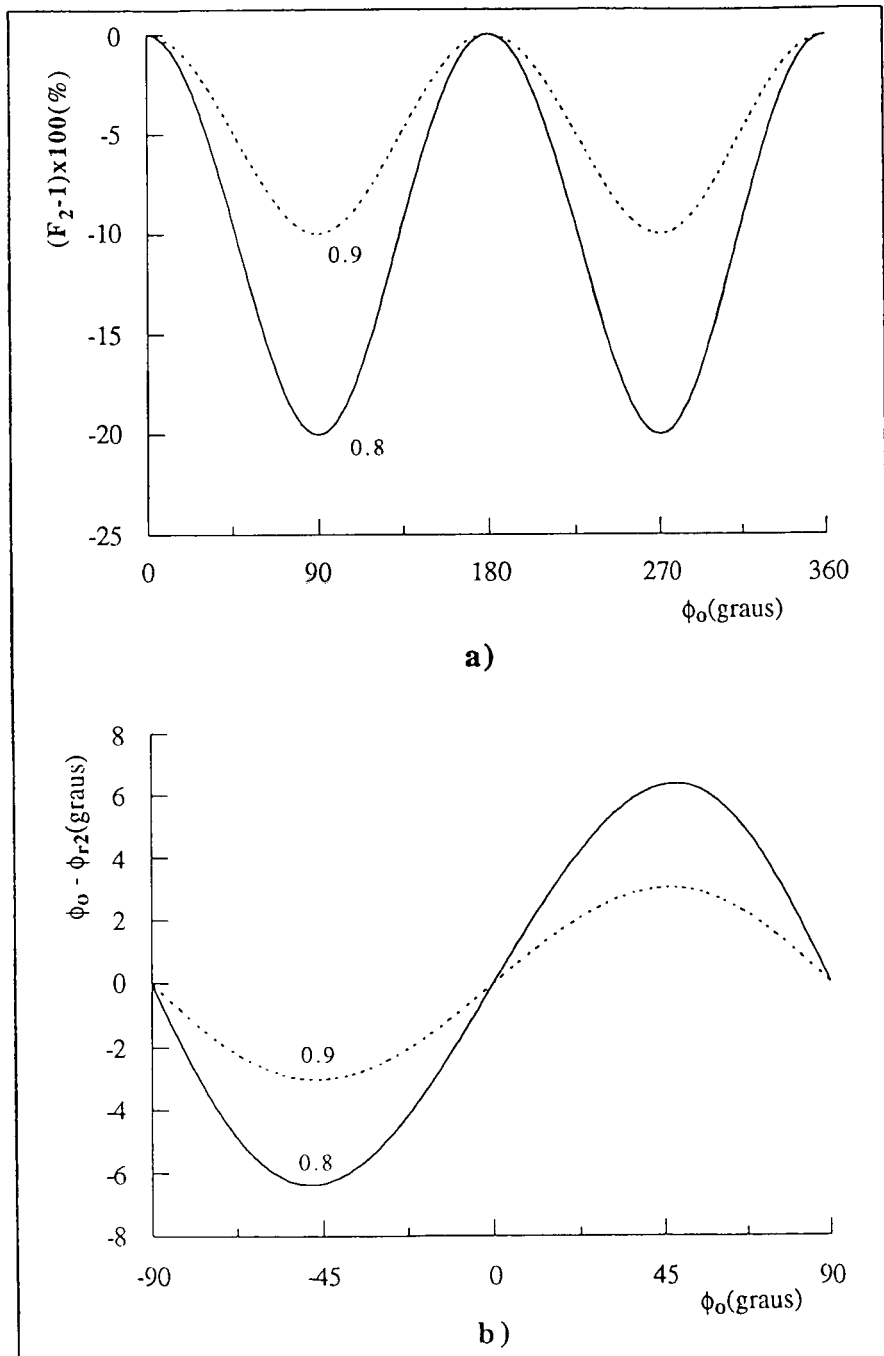
Figura 8.20. Erro de escala (a) e erro na leitura de fase (b) introduzidos pela técnica de processamento "Desvio de Fase" quando os dois sinais interferométricos não têm a mesma amplitude. As curvas são apresentadas para \beta = 0.8 e \beta = 0.9 .
