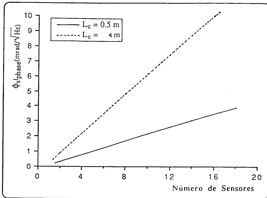
Figura 4.7. Sensibilidade de fase (valor eficaz) determinada pelo ruído de fase, em função do número de sensores ( =2N ), para os dois casos indicados.
