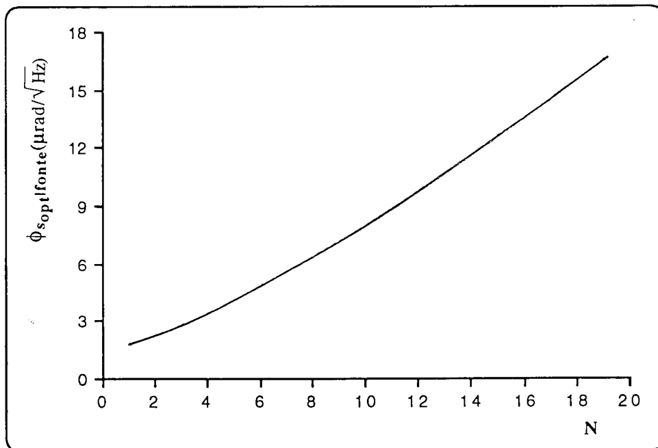
Figura 7.8. Sensibilidade de fase, em função de " N ", quando se considera somente o ruído da fonte e se utiliza para " \kappa " os valores óptimos ilustrados na Fig 7.7.
