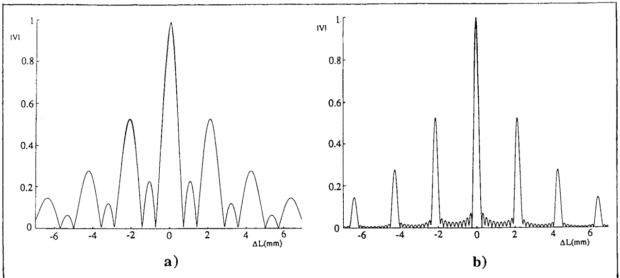
Figura 6.1. Visibilidade das franjas em função do não-balanceamento do interferómetro iluminado por radiação multimodo (visibilidade normalizada pelo seu valor em \Delta L = 0 ): a) m = 1 (3 modos longitudinais); b) m = 5 (11 modos).
