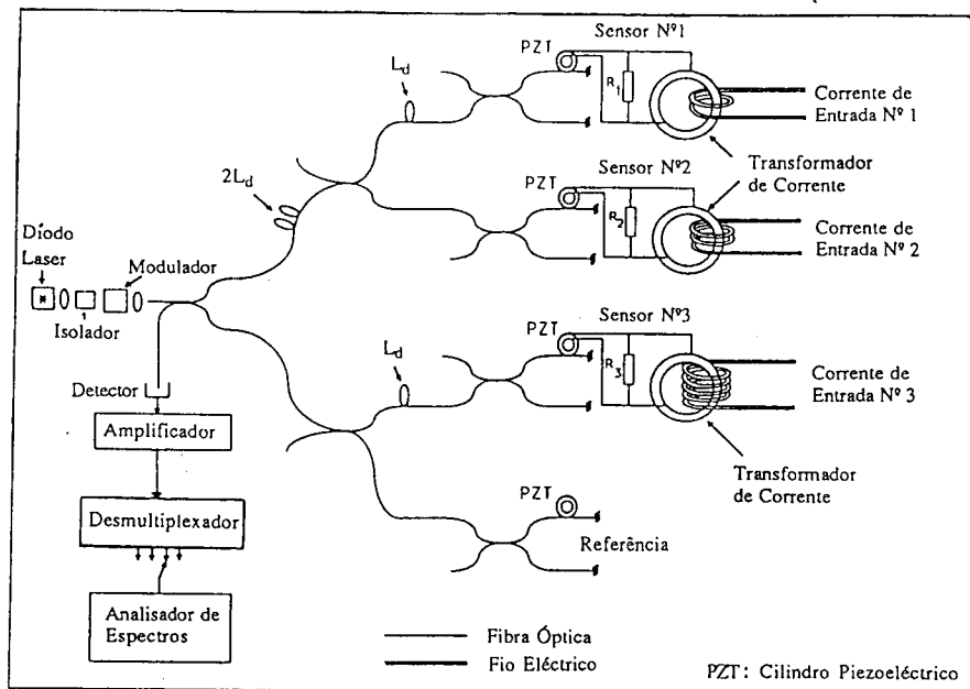
Figura 3.11. Esquema da experiência efectuada.
