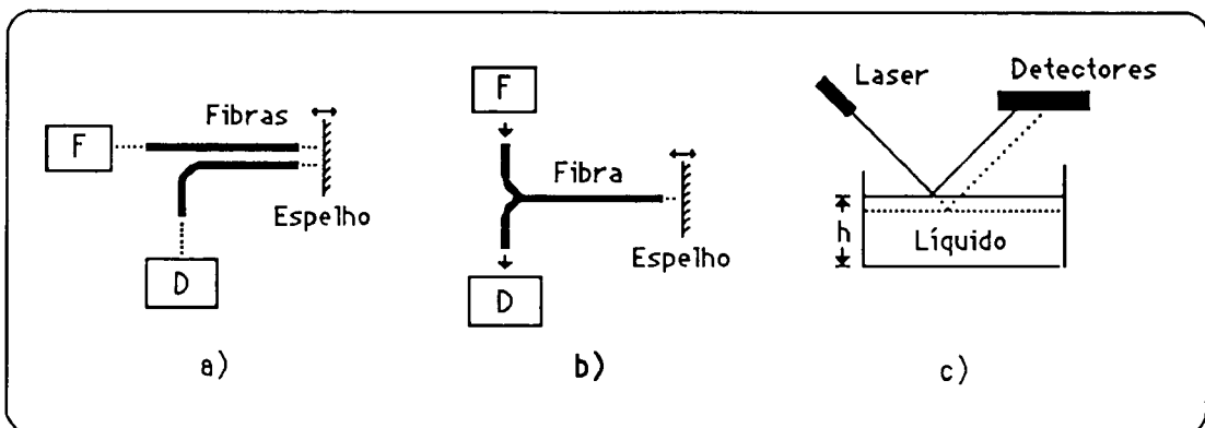
Figura 1.2. Modulação de intensidade por reflexão utilizando: a) duas fibras; b) uma fibra e divisor; c) esquema para determinar o nível dum líquido.
