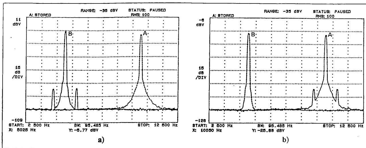
Figura 4.13. Saída dos dois canais (na situação da Fig 4.10-a) quando sinais de teste de 50 mrad de amplitude a 750 Hz foram aplicados alternadamente a cada um dos interferômetros: a) canais "A" e "B" - sinal aplicado ao interferômetro "B"; b) canais "A" e "B" - sinal aplicado ao interferômetro "A".
