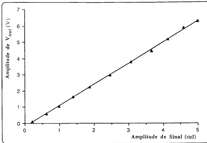
Figura 8.17. Amplitude de " V_{out} " na componente a 2 kHz em função da amplitude do sinal de fase (a 1 kHz) aplicado à cavidade.
