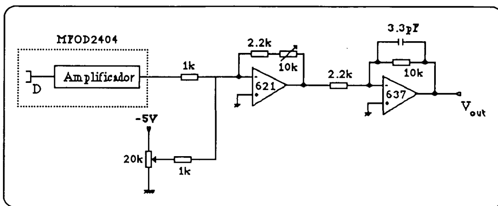
Figura 3.4. Esquema do bloco de detecção e amplificação.
