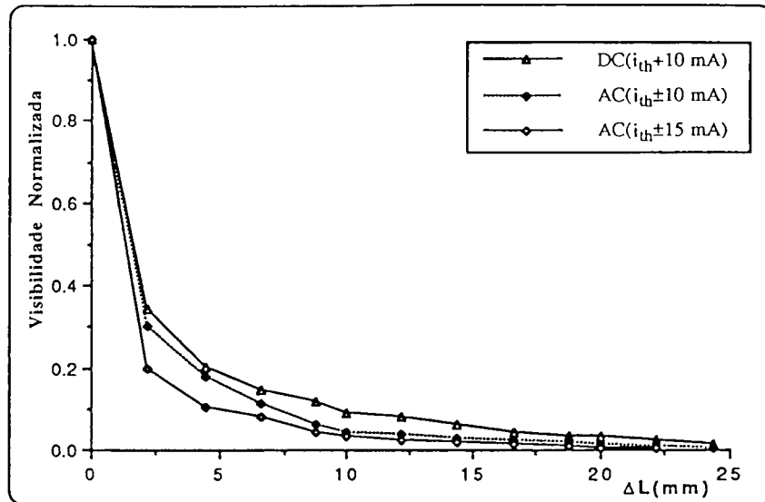
Figura 6.4. Envolvente das funções de visibilidade apresentadas na Fig 6.3 (e também para o caso da modulação com uma amplitude de corrente de 15 mA em torno do limiar).
