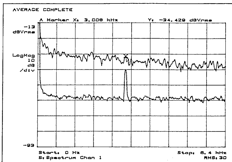
Figura 5.24. Efeito da modulação da corrente de injeção do laser semiconductor sobre o nível de ruído induzido por acoplamento da radiação para a cavidade laser (pontilhado: modulação activada; B = 64 Hz).
