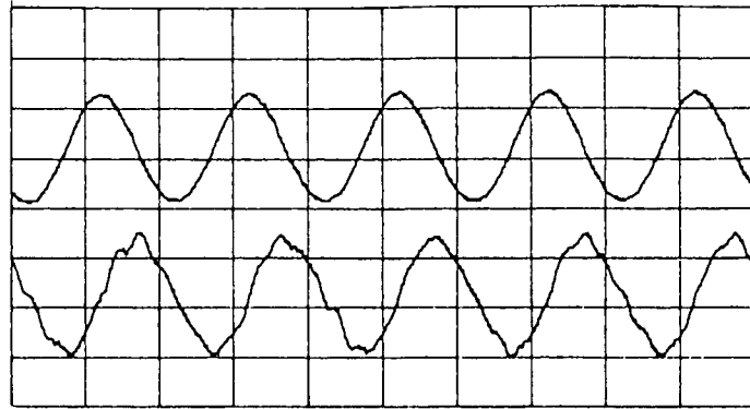
Figura 8.15. Sinais antes ( cima ) e depois ( baixo ) do diferenciador, quando um sinal sinusoidal de fase com 0.3 rad de amplitude é aplicado ao interferómetro "B" em quadratura.
