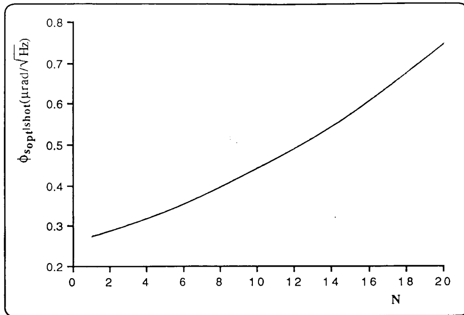
Figura 7.9. Sensibilidade de fase quando se considera somente o ruído quântico.
