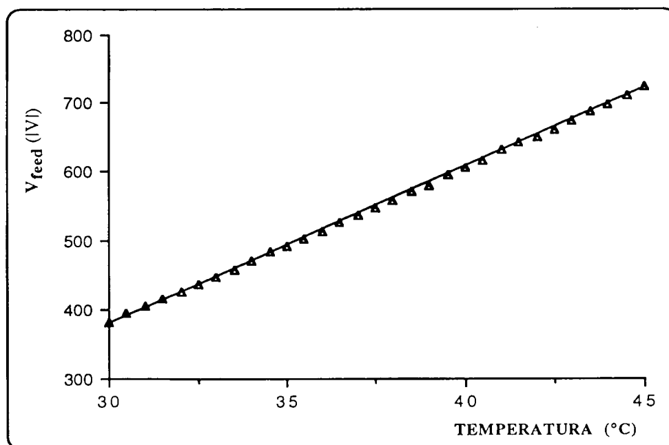
Figura 6.20. Variação da tensão " V_{feed} " em função da temperatura, com o sistema sintonizado para o sensor "B".
