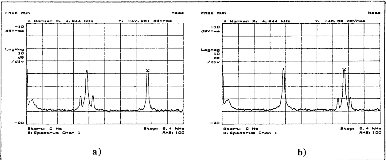
Figura 5.18. Portadoras dos interferómetros "1" e "2" juntamente com sinais de teste ( f = 250 Hz):
