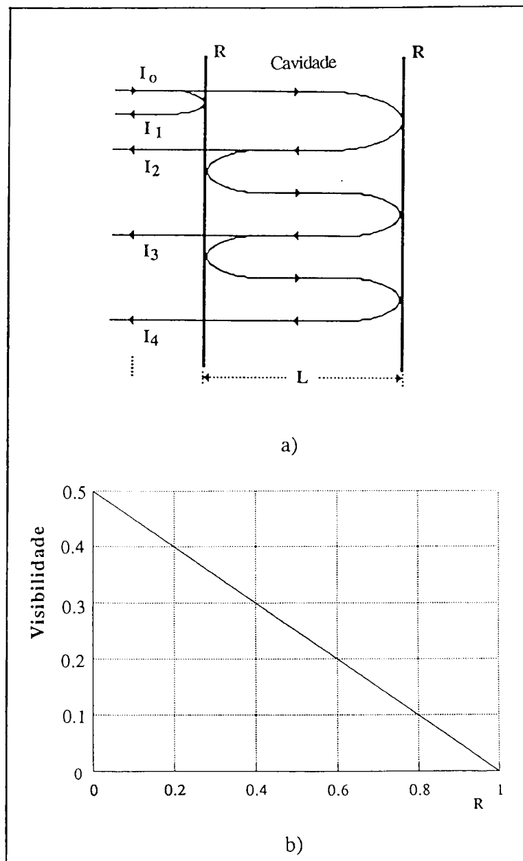
Figura 8.30. a) Ondas geradas na cavidade até à quarta ordem (representam-se as ondas separadas lateralmente apenas para tornar a figura mais clara); b) Visibilidade das franjas da função de transferência da cavidade.
