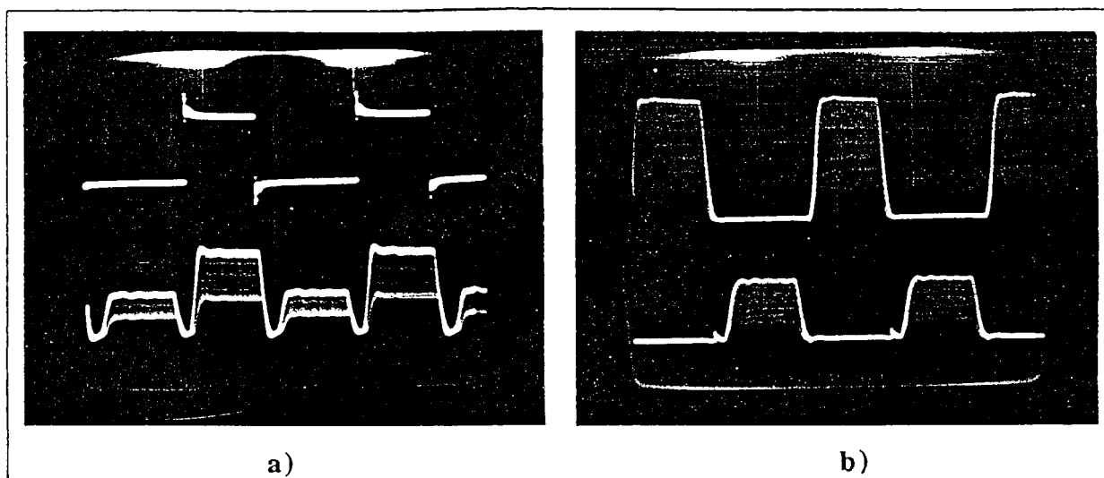
Figura 6.14. a) Cima: Forma de onda emitida pelo laser; baixo: sinal à entrada do desmultiplexador ( 2\mu\text{s/div} ; 1\text{ V/div} ). b) Formas de onda à saída dos canais "A" (cima) e "B" (baixo) - 2\mu\text{s/div} , 0.5\text{ V/div} . Em ambos os casos aplicou-se modulação de baixa frequência a um dos espelhos do interferómetro receptor ajustado para não-balanceamento nulo.
