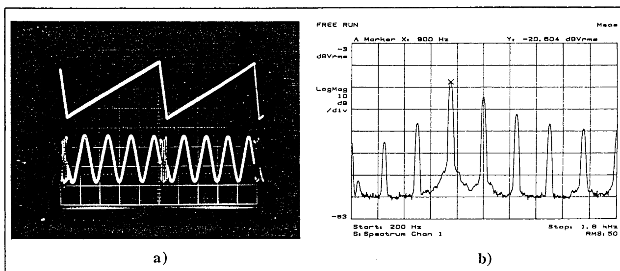
Figura 5.17. a) Cima: forma de onda aplicada ao interferómetro "0"; baixo: saída deste (1 ms/div); b) Espectro da saída do interferómetro.
