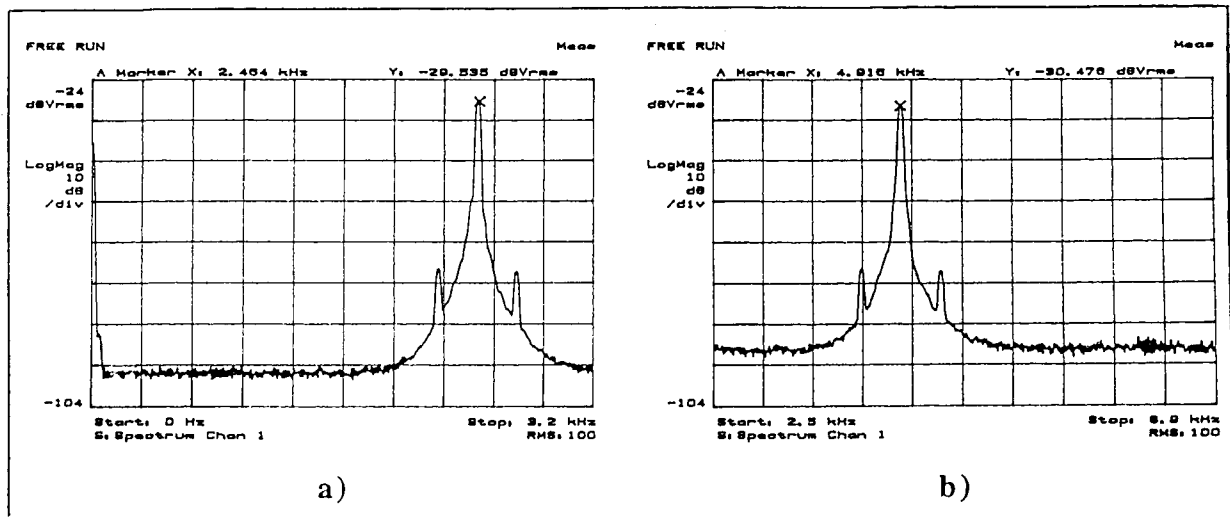
Figura 5.19. Sinais " V_{out1} " (a) e " V_{out2} " (b) à saída dos filtros de banda que proporcionam a saída dos canais associados aos interferómetros "1" e "2", respectivamente (sinal aplicado: amplitude - 123 mrad; frequência - 250 Hz). Para o caso a) B = 32 Hz; para o caso b), B = 64 Hz.
