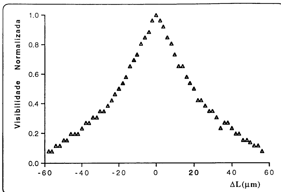
Figura 7.13. Visibilidade das franjas em função do não-balanceamento " \Delta L " de um interferómetro de Michelson iluminado pela fonte óptica utilizada na experiência (visibilidade normalizada pelo seu valor em \Delta L = 0 ).
