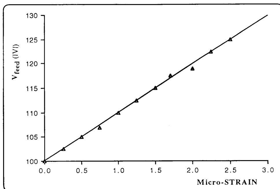
Figura 6.18. Variação da tensão " V_{\text{feed}} " em função da deformação aplicada ao sensor "A".
