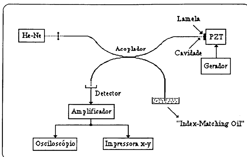
Figura 8.26. Esquema da experiência efectuada para determinar a função de transferência da cavidade de Fabry-Pérot.
