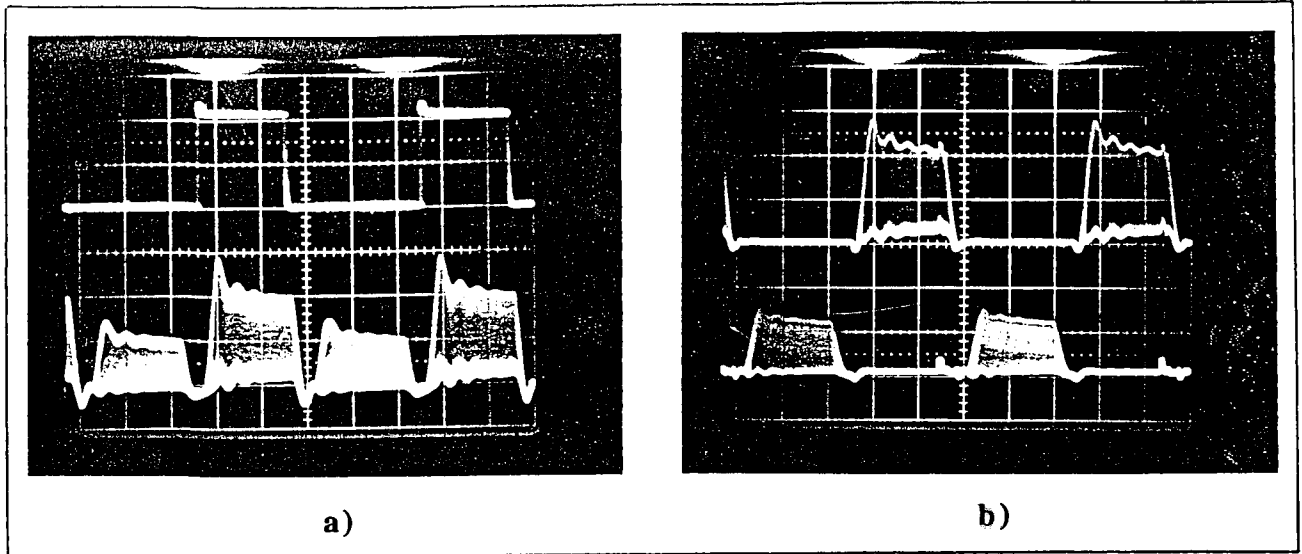
Figura 8.4. a) Cima: forma de onda injectada na fibra de iluminação do sistema; baixo: sinal à saída do amplificador ( 2 \mu\text{s}/\text{div} ). b) cima: sinal à saída do canal "A"; baixo: sinal à saída do canal "B" ( 1 \text{ V}/\text{div} ; 2 \mu\text{s}/\text{div} ).
