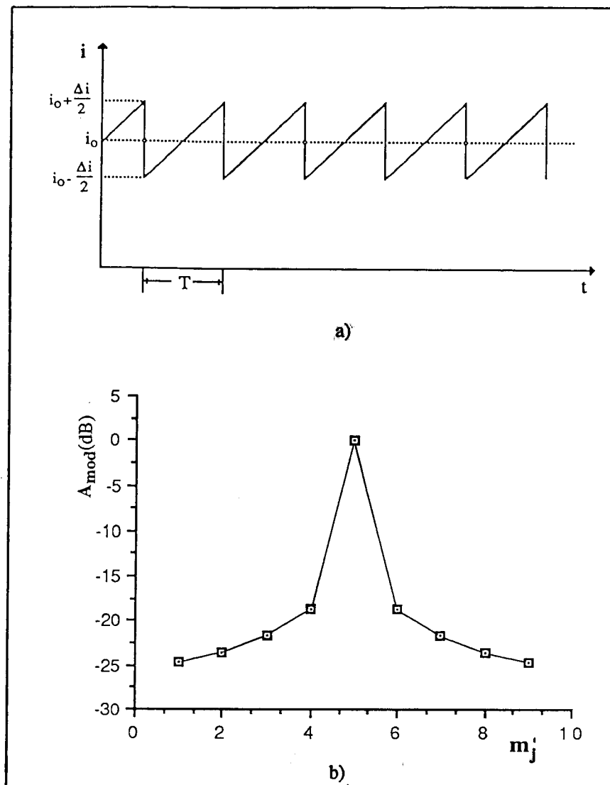
Figura 5.8. a) Forma de onda de corrente aplicada ao laser semiconductor; b) "crosstalk" do sensor "j" (com \omega_j = 5\omega_r ) para outros harmônicos devido à modulação da radiação emitida ( p = |m_j - m_j'| ).
