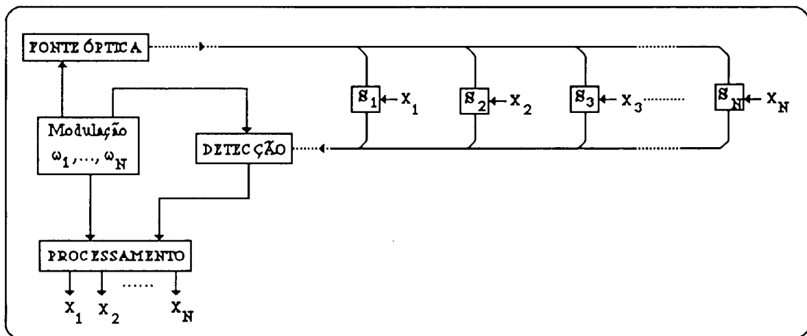
Figura 2.5. Endereçamento de sensores em frequência por sub-portadora numa rede escada transmissiva.
