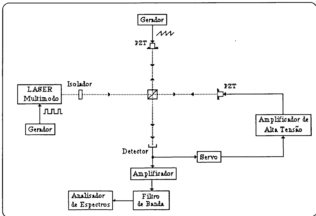
Figura 6.2. Esquema da experiência efectuada para se determinar o efeito da modulação da corrente de injeção do laser semiconductor multimodo na sua estrutura espectral.
