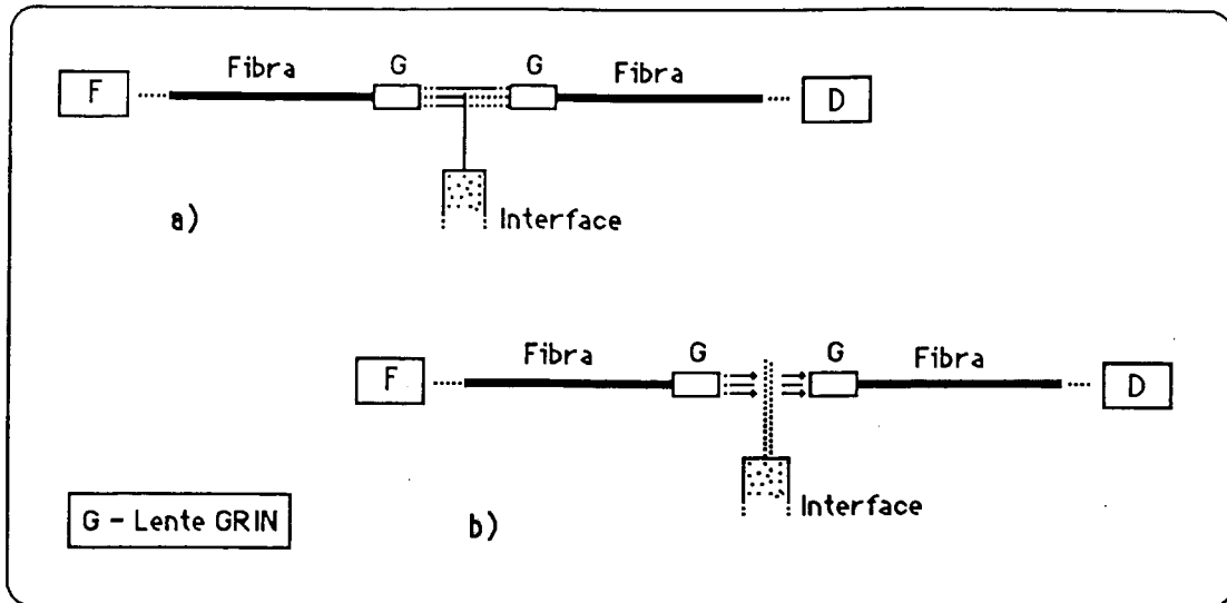
Figura 1.1. Modulação de intensidade por ocultação: a) por lâmina; b) por rede ("F"- Fonte; "D" - Detector).
