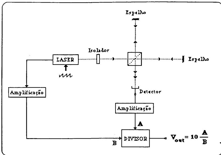
Figura E.3. Esquema da experiência efectuada.
