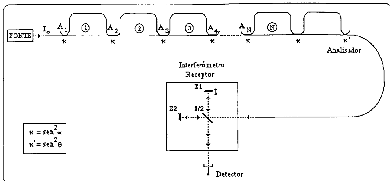
Figura 7.2. Esquema equivalente ao da Fig 7.1, com os dois modos da fibra Hi-Bi separados espacialmente.
