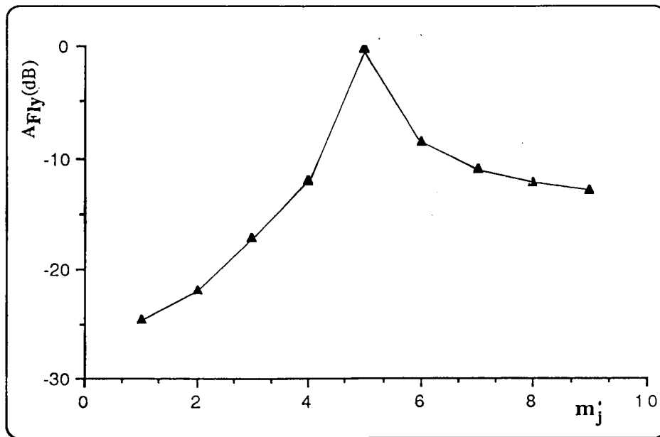
Figura 5.10. "Crosstalk" do sensor "j" (com m_j = 5 ) para outros harmónicos devido ao tempo de descida da onda em dente-de-serra ( \mu = 0.98 ; p = m_{j'} ).
