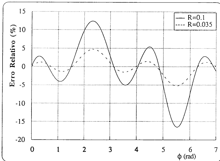
Figura 8.29. Erro de escala introduzido pela técnica de desmodulação "Desvio de Fase" ao processar a função de transferência de Fabry-Pérot.
