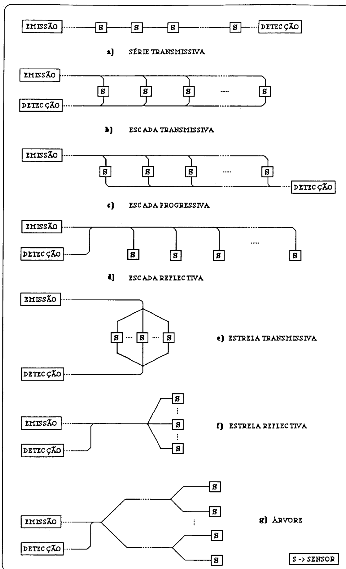
Figura 2.2. Topologias básicas de redes de sensores de fibra óptica.
