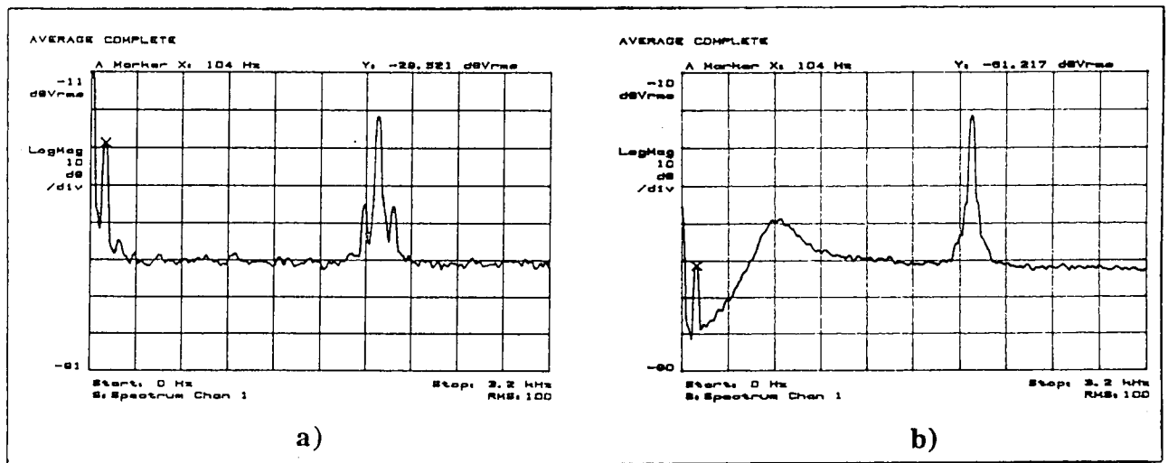
Figura 5.16. Demonstração do efeito do sistema de compensação: a) portadora gerada para o interferómetro "1"; sinal de perturbação aplicado ao interferómetro "0"; servo desligado; b) o mesmo que a), mas agora com o servo operacional.
