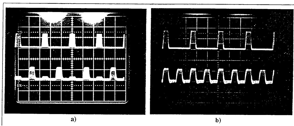
Figura 4.10. a) cima: sinal de modulação do díodo laser; baixo: sequência de impulsos à saída do amplificador ( 2 \mu\text{s/div} ); b) cima: sinal de modulação do díodo laser; baixo: sequência de impulsos à saída do amplificador quando a potência óptica de retorno do canal "B" é atenuada \approx 10 dB ( 2 \mu\text{s/div} ).
