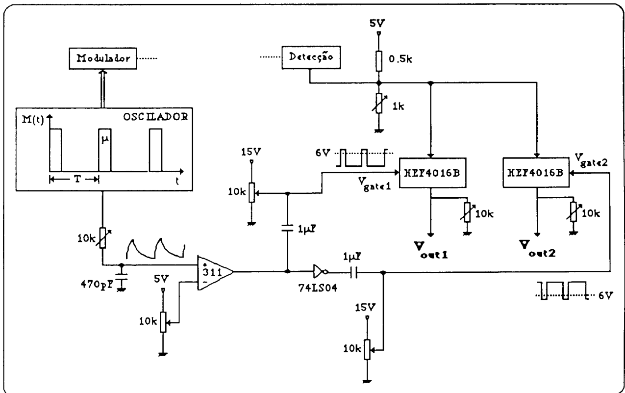
Figura C.1. Esquema de um desmultiplexador de dois canais.
