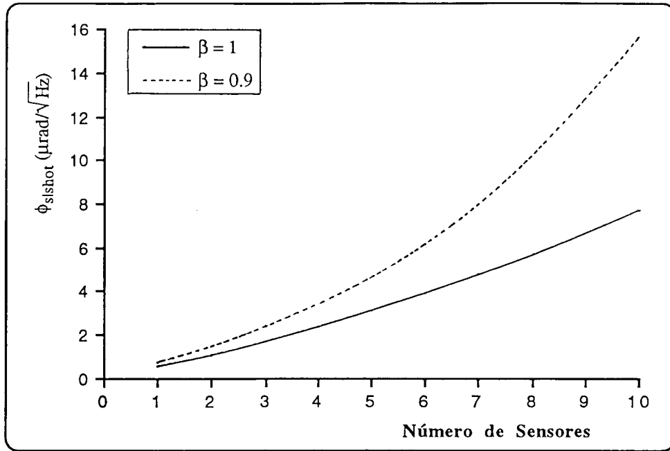
Figura 5.4. Sensibilidade de fase determinada pelo ruído quântico, em função do número de sensores da rede. Considera-se os casos \beta = 1 e \beta = 0.9 .
