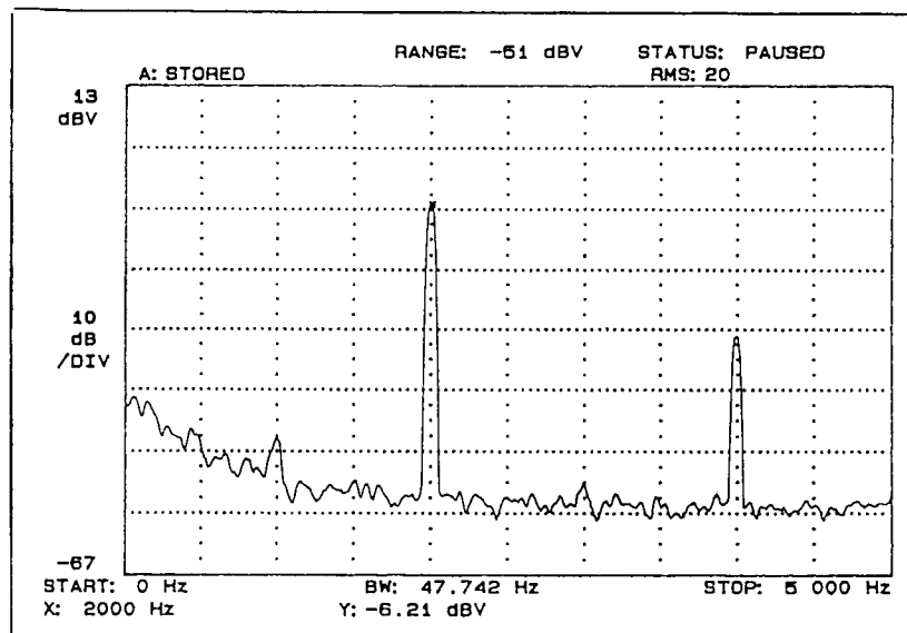
Figura 8.16. Sinal " V_{out} " na situação em que um sinal de fase com amplitude de 85 mrad (valor eficaz) a 1 kHz é aplicado à cavidade.
