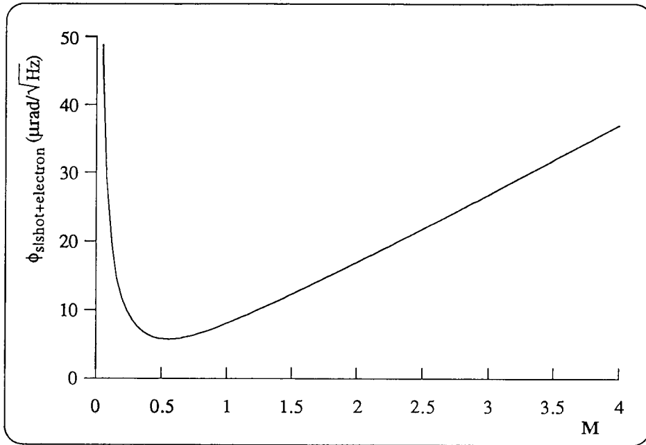
Figura 5.7. Sensibilidade de fase, em função de " M ", quando se considera somente o ruído quântico e o ruído electrónico ( \beta = 1 , N = 10 ).
