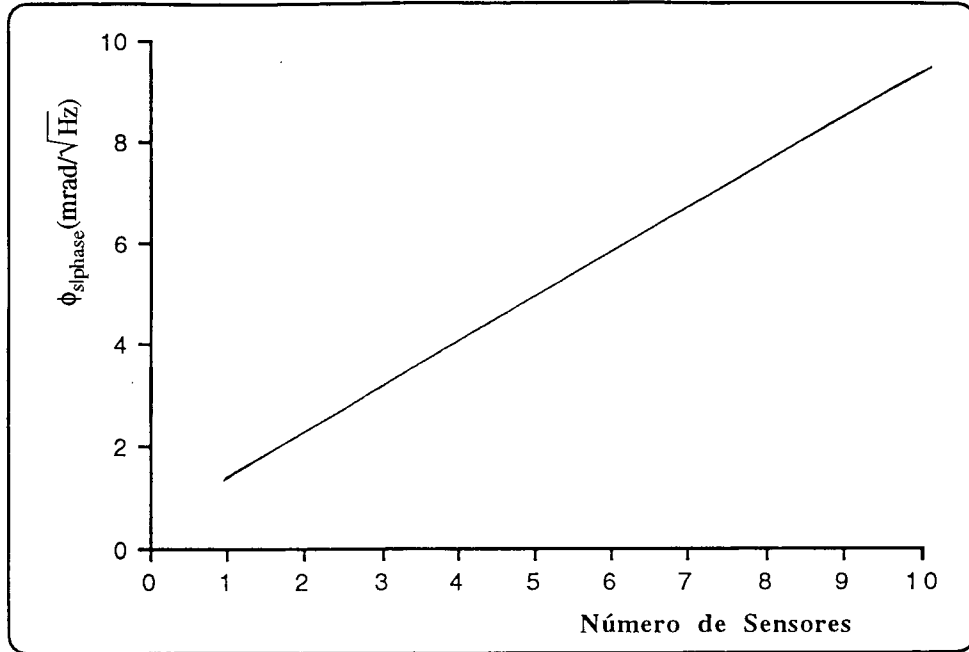
Figura 5.6. Sensibilidade determinada pelo ruído de fase, em função do número de sensores da rede.
