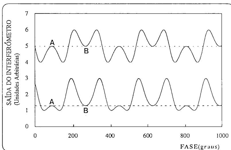
Figura B.1. Sinais à saída do interferómetro quando a amplitude da modulação de fase é igual a " \pi " [as duas formas de onda - que foram separadas verticalmente para melhor visualização - correspondem a: \phi_0 = \pi/4 (onda inferior); \phi_0 = \pi/2 (onda superior)].
