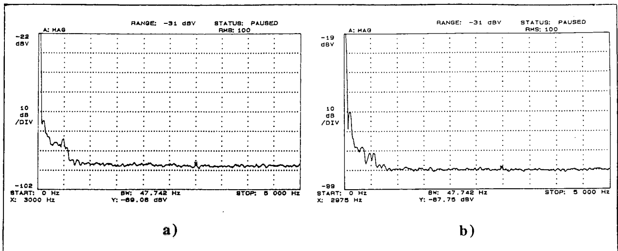
Figura 6.16. Resultados relativos à interferência entre sensores: a) sinal " V_{out} " com o sistema sintonizado para o sensor "A" e com um sinal aplicado ao sensor "B"; b) sinal " V_{out} " com o sistema sintonizado para o sensor "B" e com um sinal aplicado ao sensor "A".
