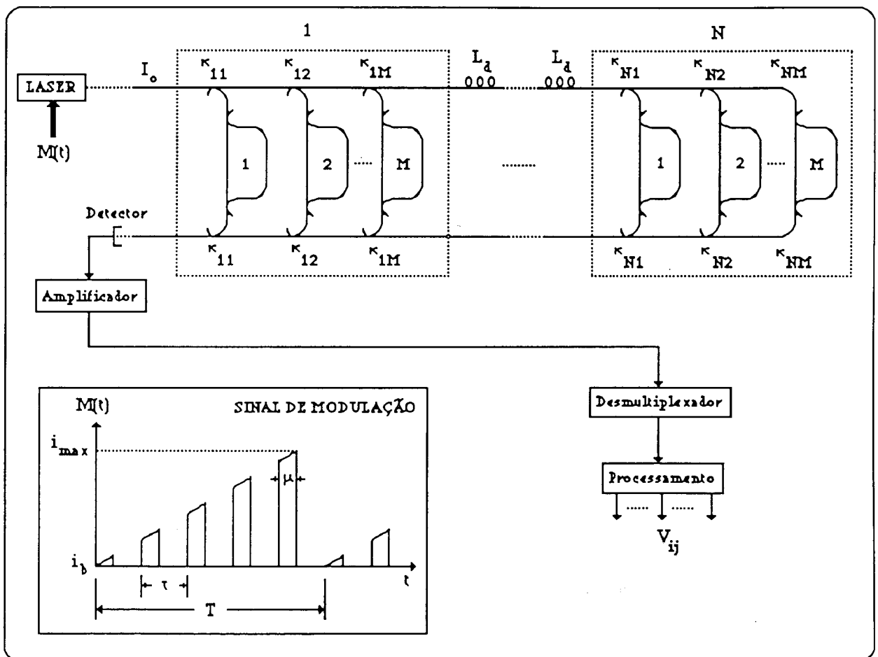
Figura 4.1. Multiplexagem mista de sensores interferométricos (Mach-Zehnder) distribuídos numa topologia escada transmissiva (" i_b ", " i_{max} " designam níveis para a corrente de injeção do laser semiconductor, a que correspondem as potências ópticas injectadas no sistema " I_b " e " I_{max} ", respectivamente).
