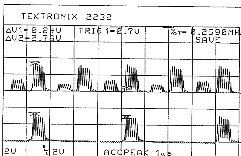
Figura 3.7. Exemplo do funcionamento do desmultiplexador (todos os sensores modulados): em cima - sequência de impulsos à entrada; em baixo - saída associada ao sensor 1.
