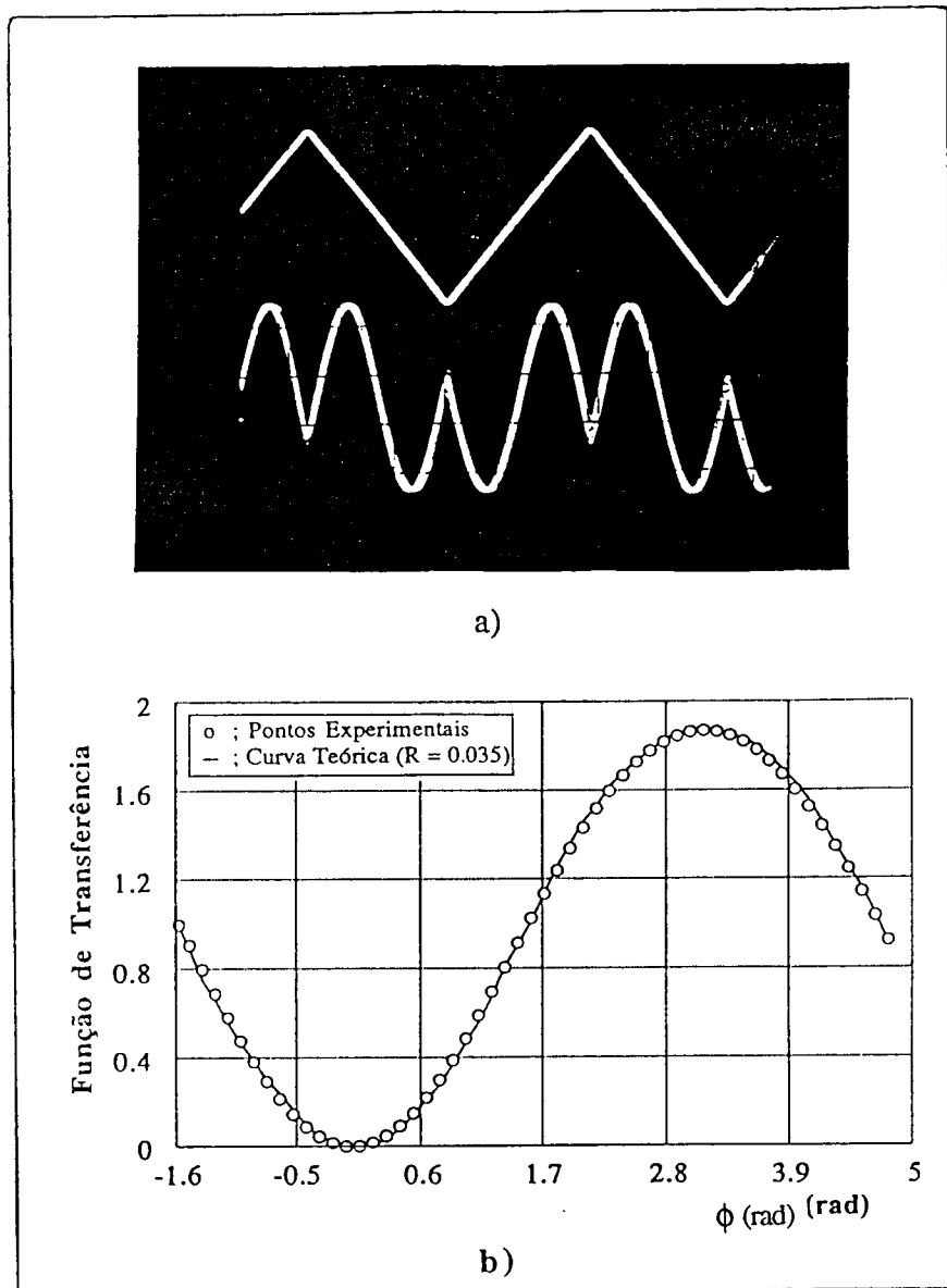
Figura 8.27. a)Cima: sinal aplicado ao PZT; baixo: saída do interferómetro; b) pontos experimentais e curva teórica obtida a partir de (8-27).
