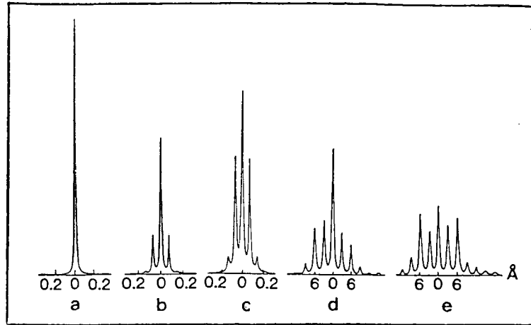
Figura 2.10. Modificação do espectro da radiação emitida por um laser semiconductor a 830 nm, em função da fracção "F" de potência óptica reinjectada na cavidade: a) F = 0 ; b) F = 0.041\% ; c) F = 0.06\% ; d) F = 0.3\% ; e) F = 1.5\% [141].
