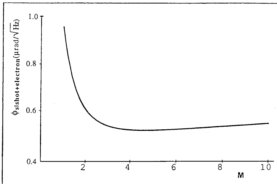
Figura 7.11. Sensibilidade determinada pelo conjunto "ruído quântico + ruído electrónico", em função de "M", para N = 10 , \kappa = 0.5 e amplificador 741.
