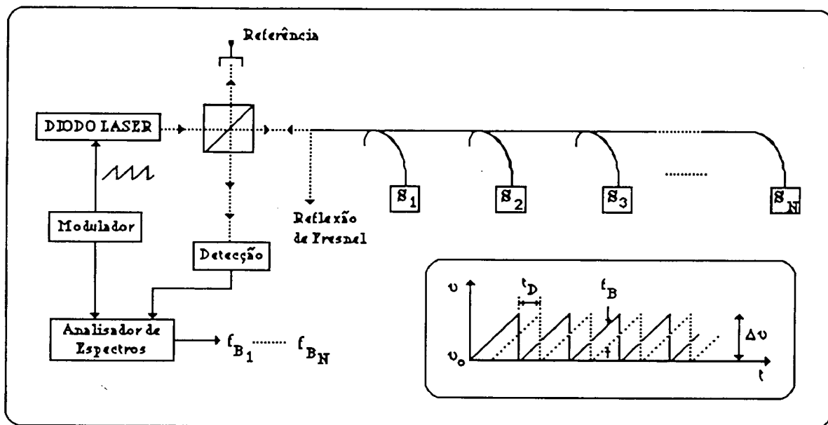
Figura 2.4. Endereçamento de sensores em frequência, por batimento de ondas numa rede escada reflectiva.
