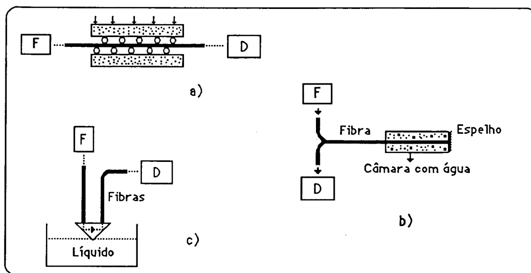
Figura 1.3. Modulação de intensidade por variação das perdas na fibra: a) sensor de microcurvatura; b) sensor de temperatura; c) sensor de nível de líquido.
