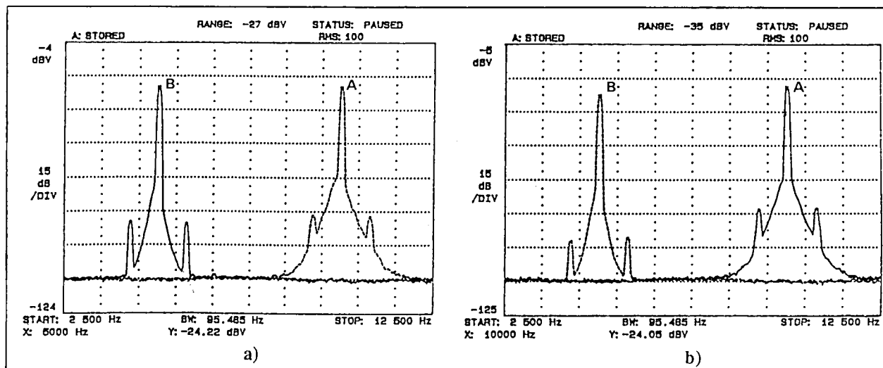
Figura 4.14. Saída dos dois canais (na situação da Fig 4.10-b) quando sinais de teste de 50 mrad de amplitude a 750 Hz foram aplicados alternadamente a cada um dos interferômetros: a) canais "A" e "B" - sinal aplicado ao interferômetro "B"; b) canais "A" e "B" - sinal aplicado ao interferômetro "A".
