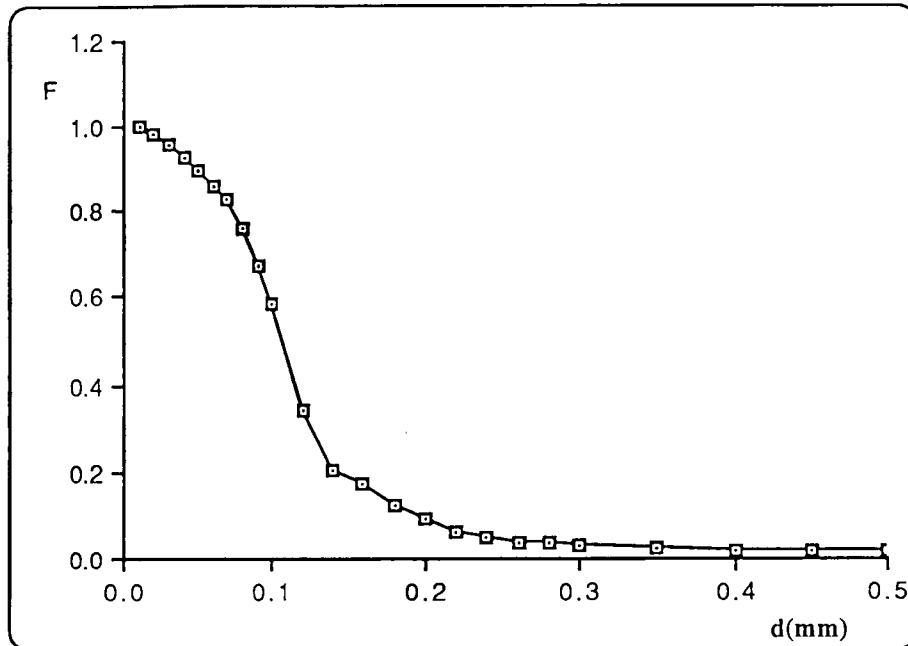
Figura 8.3. Dependência (normalizada) da potência reinjectada na fibra após reflexão no espelho à distância "d".
