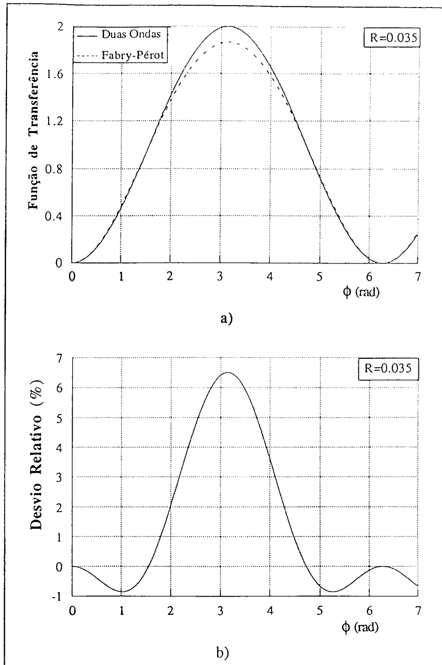
Figura 8.25. a) Função de transferência de Fabry-Pérot para R = 0.035 , e função correspondente à interferência de duas ondas; b) Desvio relativo entre estas duas funções.
