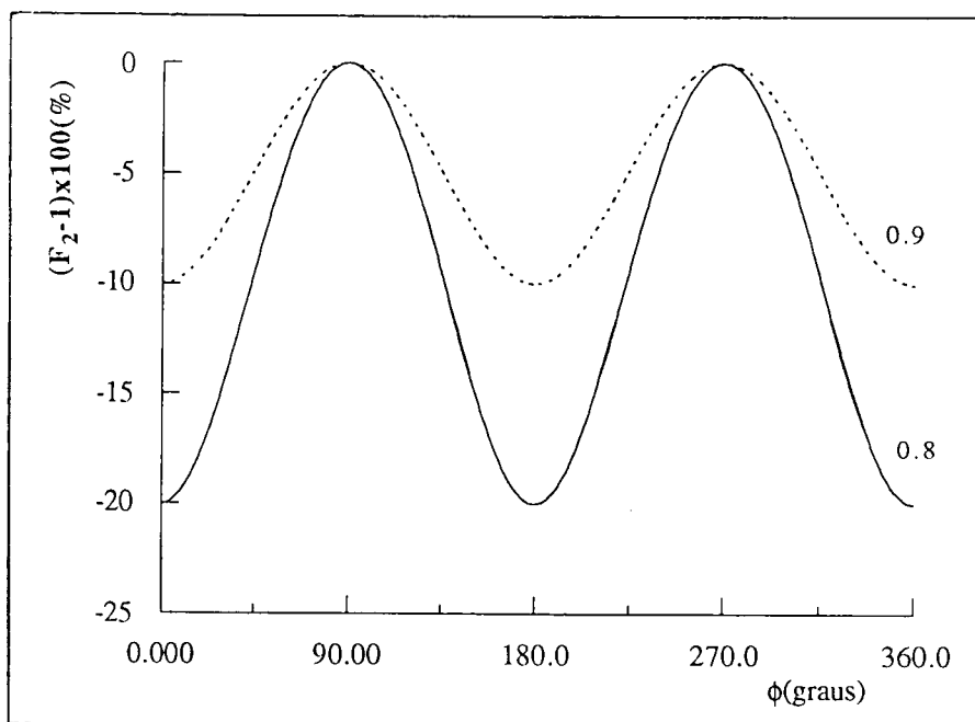
Figura 8.22. Erro de escala introduzido pela técnica de processamento "Diferenciação, Soma e Integração", quando os dois sinais interferométricos não têm a mesma amplitude. São considerados os casos \beta = 0.8 e \beta = 0.9 .
