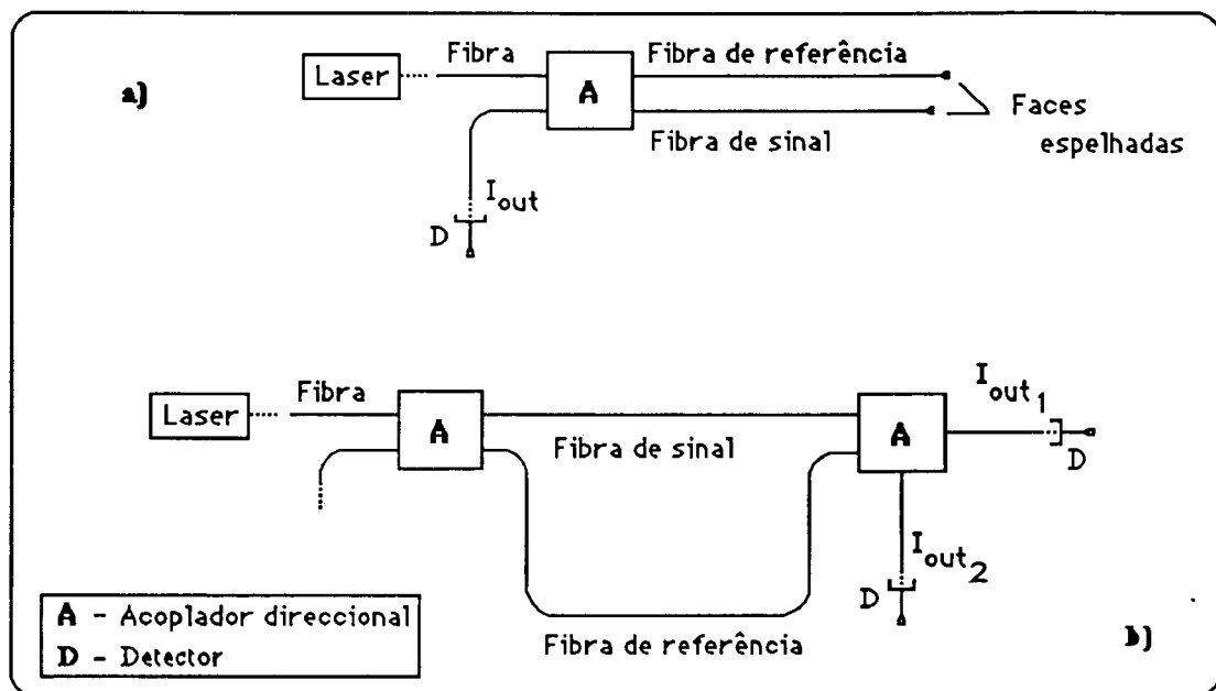
Figura 1.6. Implementação em fibra monomodo dos interferómetros de Michelson (a) e de Mach-Zehnder (b).
