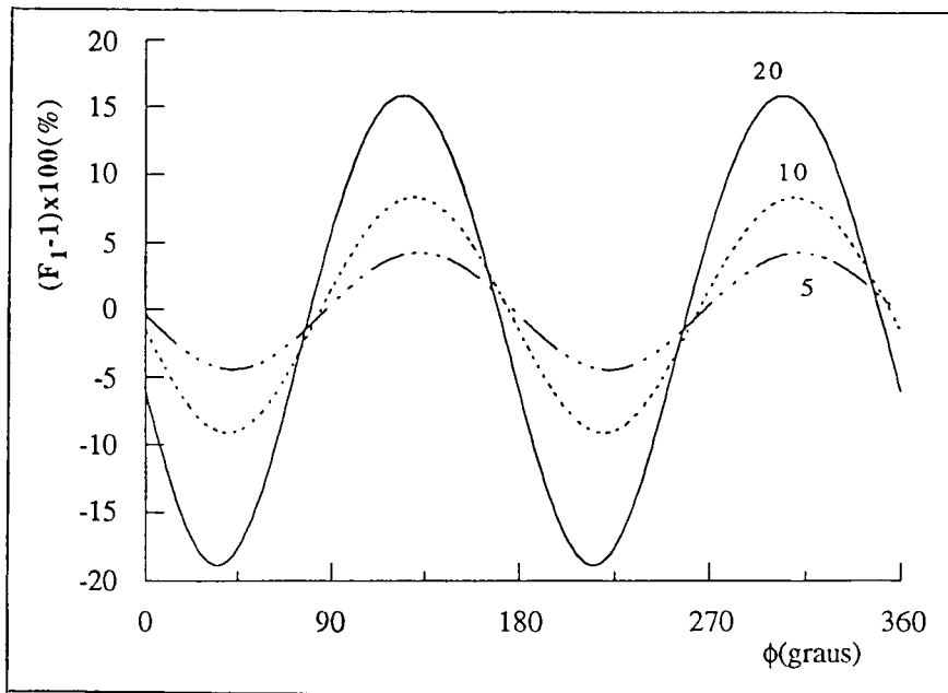
Figura 8.21. Erro de escala introduzido pela técnica de processamento "Diferenciação, Soma e Integração", quando os dois sinais interferométricos não variam em quadratura. São considerados os casos \Delta\phi = 5^\circ, 10^\circ e 20^\circ .
