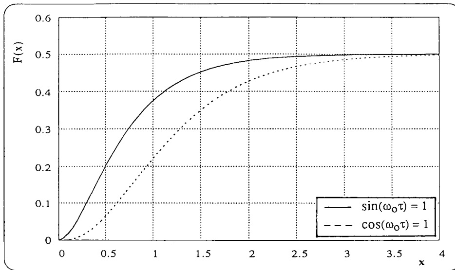
Figura D.2. Representação da função F(x) para os casos \sin(\omega_0 \tau) = 1 e \cos(\omega_0 \tau) = 1 .
