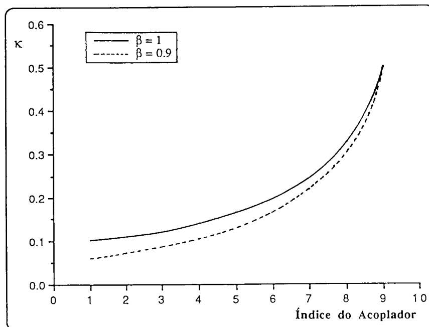
Figura 4.3. Factor de divisão de potência dos acopladores direccionais nas fibras de iluminação e de retorno, em função da sua posição ao longo da rede (considera-se NM = 10 ); representa-se os casos de ausência de perdas ( \beta = 1 ), e perda de 0.45 dB por acoplador ( \beta = 0.9 ).
