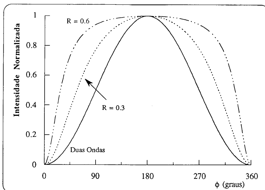
Figura 8.23. Funções de transferência em reflexão (normalizadas pelo seu valor máximo) de uma cavidade de Fabry-Pérot. Representa-se os casos correspondentes a R = 0.3 e R = 0.6 , assim como a situação limite relativa à interferência de duas ondas.
