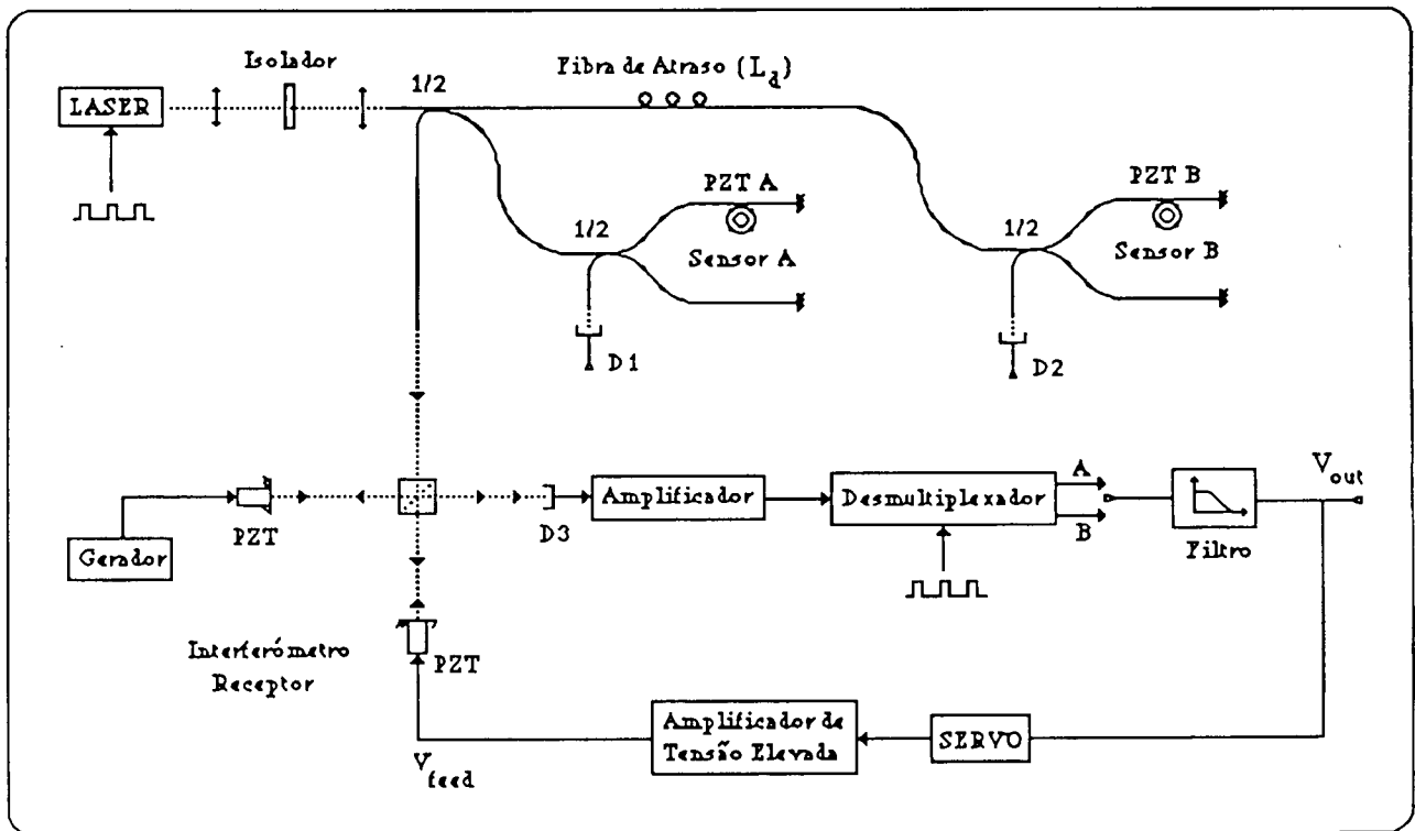
Figura 6.12. Esquema da implementação experimental.
