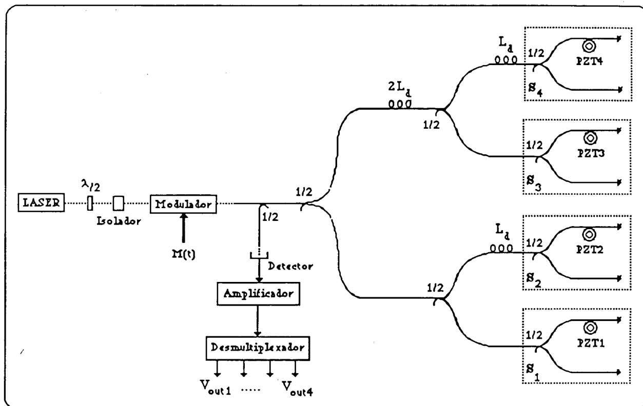
Figura 3.3. Esquema da experiência efectuada para testar a rede de sensores.
