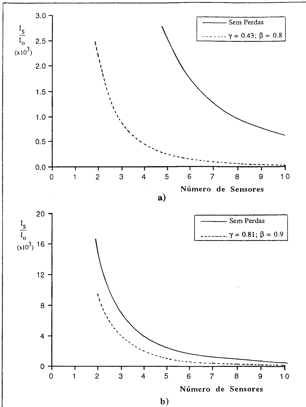
Figura 6.8. Potência óptica média de retorno de cada sensor, normalizada pela potência óptica média injectada no sistema. Considera-se os casos sem e com perdas de potência. a) operação a 800 nm; b) operação a 1300 nm.
