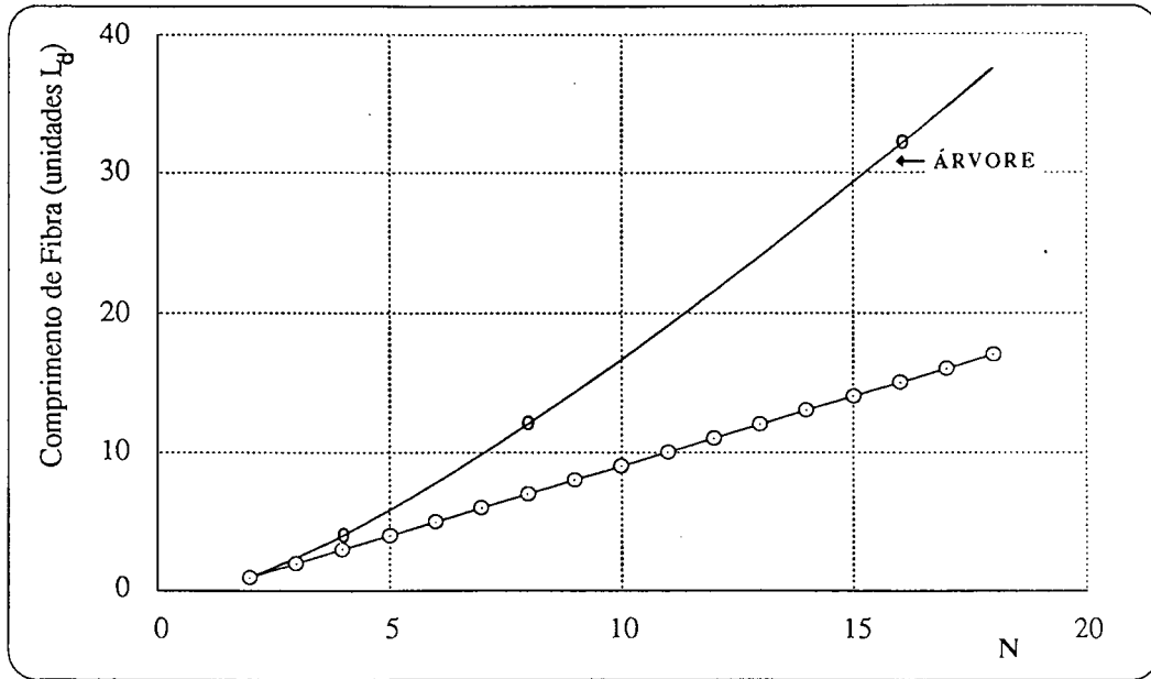
Figura 3.2. Extensão total de fibra (em unidades " L_d ") necessária para a implementação do endereçamento temporal de " N " sensores nas topologias árvore e série reflectiva.
