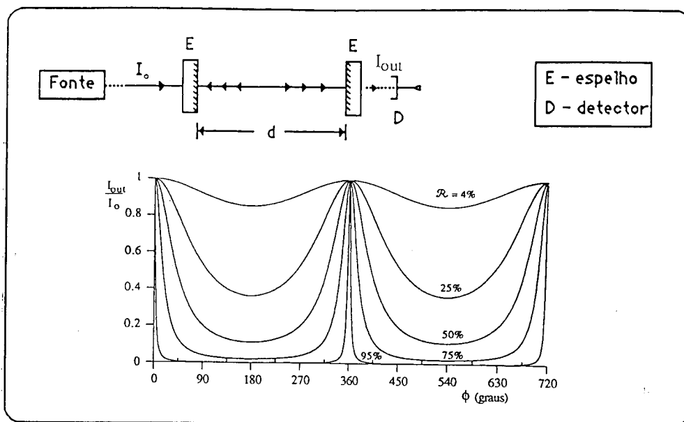
Figura 1.7. Configuração convencional do interferômetro de Fabry-Pérot em transmissão Os espelhos são parcialmente transparentes, de reflectividade "R".
