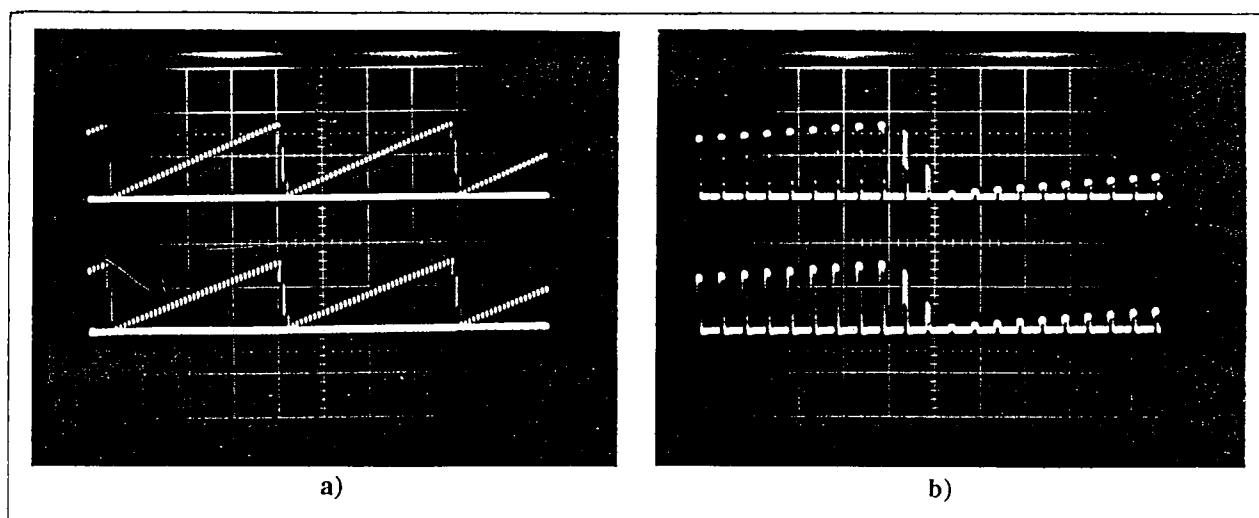
Figura 4.9. a) cima: sinal de modulação da corrente de injeção do laser semiconductor; baixo: sinal óptico emitido pelo laser (50 \mu s/div). b) versão expandida de a) (10 \mu s/div).
