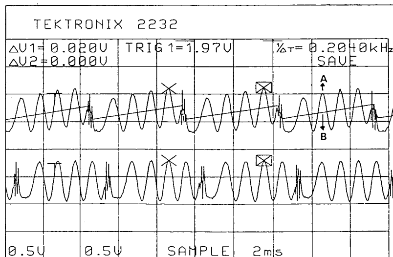
Figura E.4. Cima: A - sinal à saída do interferómetro; B - sinal de referência; Baixo: forma de onda à saída do divisor.
