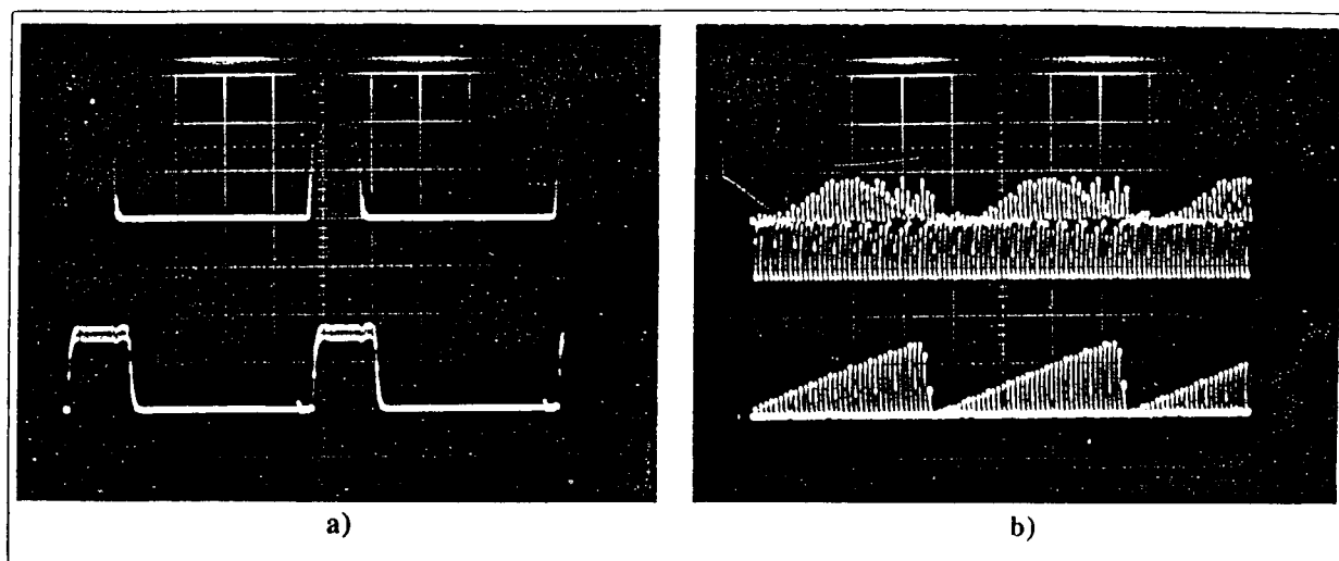
Figura 4.11. a) cima: sinal de modulação do díodo laser; baixo: saída do canal "A" do desmultiplexador (1 \mu s/div); b) cima: saída do canal "B" do desmultiplexador; baixo: sinal de modulação do díodo laser (0.2 ms/div).
