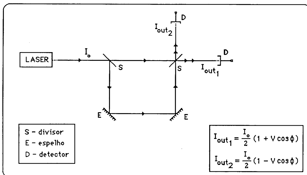
Figura 1.5. Configuração convencional do interferómetro de Mach-Zehnder (a função de transferência é idêntica à do interferómetro de Michelson).
