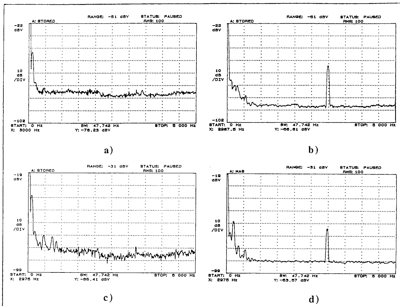
Figura 6.15. a) Sinal à saída do detector D1 com um sinal de fase de 10 mrad de amplitude aplicado ao sensor "A"; b) Sinal " V_{out} " com o sistema sintonizado para o sensor "A"; c) Sinal à saída do detector D2 com o mesmo sinal de fase aplicado ao sensor "B"; d) Sinal " V_{out} " correspondente.
