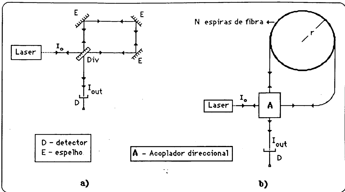
Figura 1.9. Configuração convencional do interferômetro de Sagnac (a) e correspondente implementação em fibra (b).
