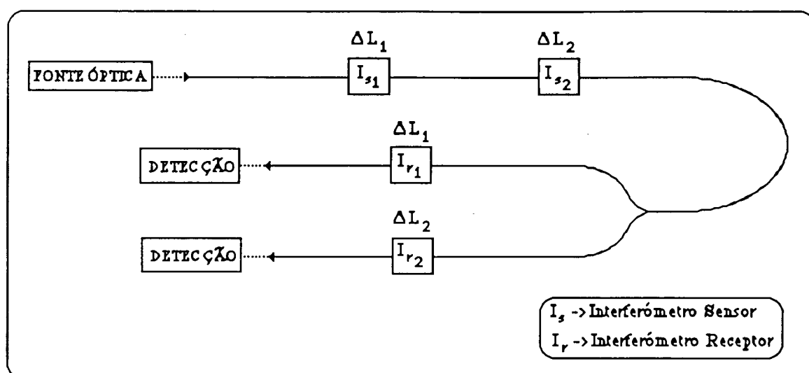
Figura 2.6. Endereçamento em coerência de dois interferómetros dispostos numa topologia série transmissiva.
