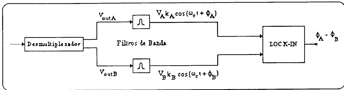
Figura 8.5. Esquema utilizado para determinar a estabilidade relativa da fase dos dois interferómetros.
