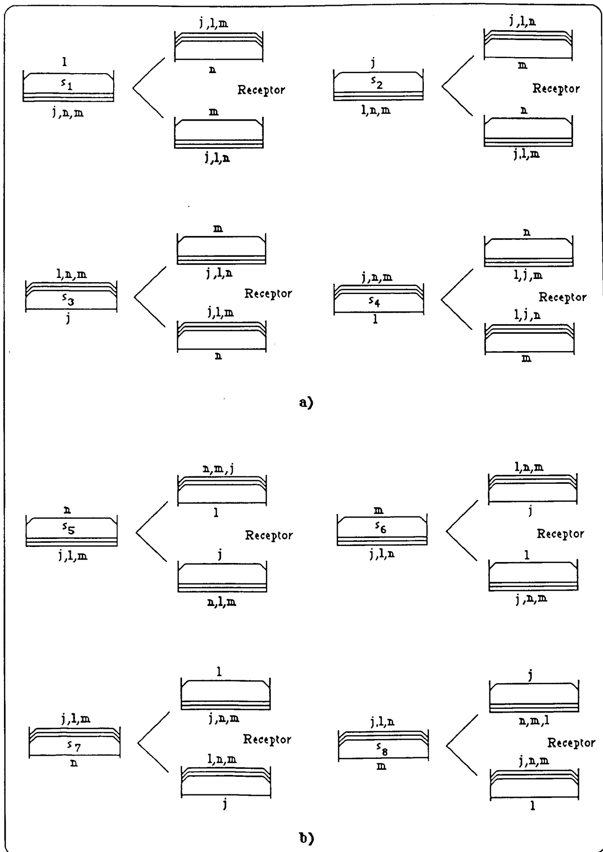
Figura 7.5. a) Configurações para os interferômetros sensor e receptor que satisfazem a condição T_j - T_\ell = T_n - T_m com os percursos "j" e "l" distintos no sensor ; b) casos para os quais os percursos "j" e "l" são comuns no sensor.
