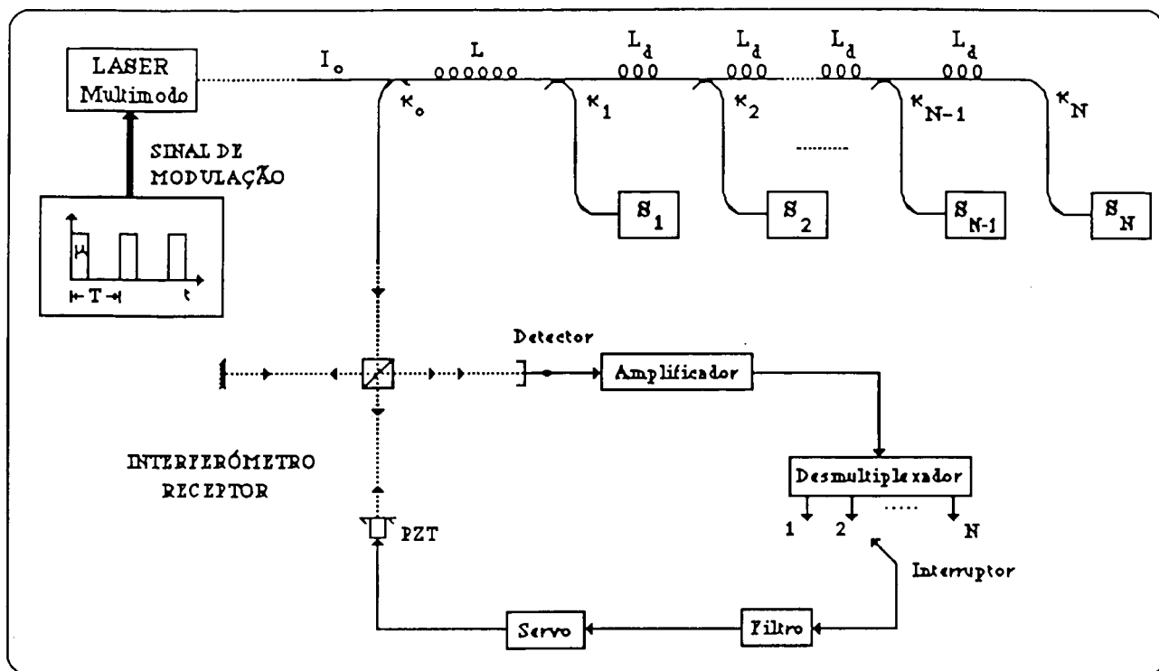
Figura 6.6. Esquema de multiplexagem com topologia "escada reflectiva", endereçamento temporal, desmodulação em coerência e iluminação multimodo.
