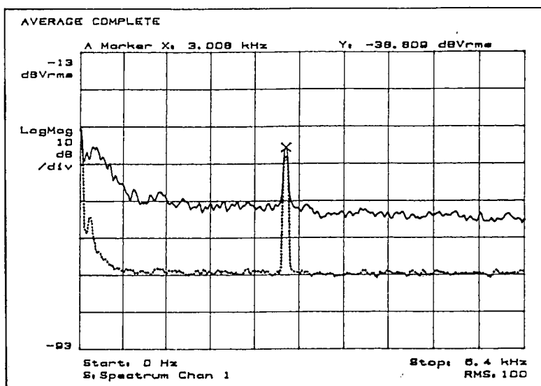
Figura 5.21. Saída do interferómetro "0" ilustrando o efeito da modulação (curva a pontilhado) da corrente de injeção do laser semiconductor ( B = 64 Hz).
