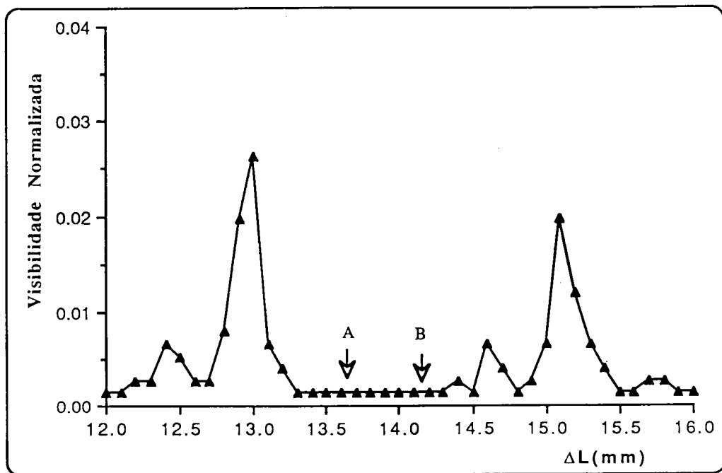
Figura 6.13. Não-balanceamento dos interferómetros sensores, ilustrando-se a sua localização numa das regiões de baixa visibilidade (visibilidade normalizada pelo seu valor em \Delta L = 0 ).
