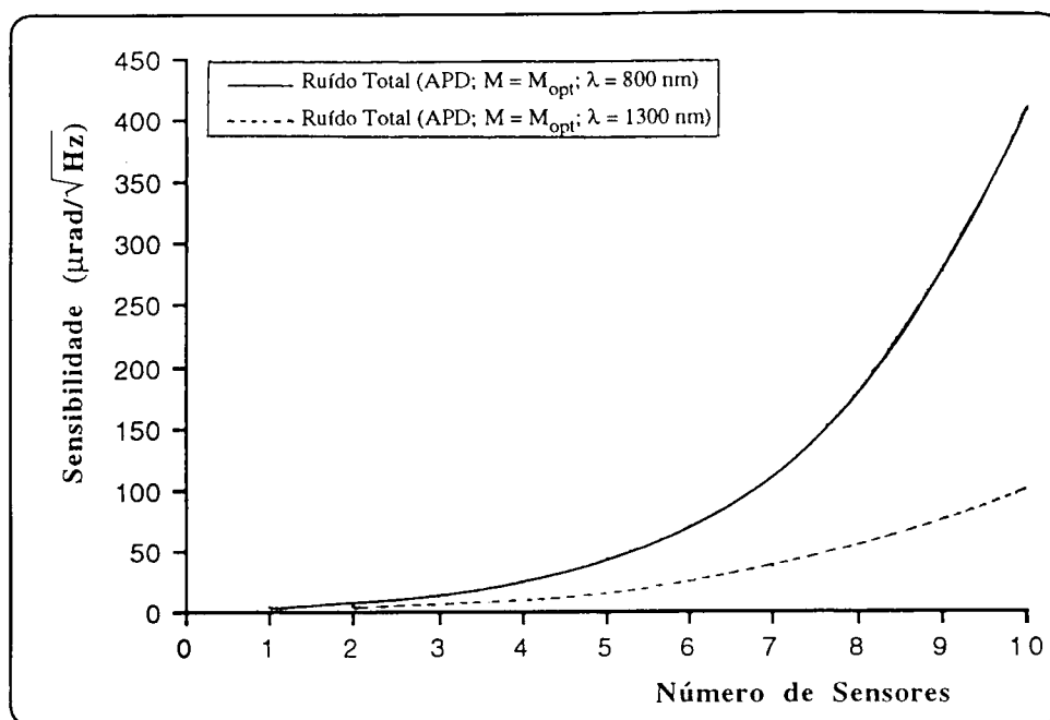
Figura 6.11. Sensibilidade dos sensores da rede para ganho ótimo na detecção.
