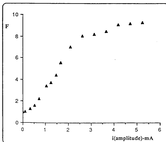
Figura 5.22. Factor de redução do nível de ruído do sistema em função da amplitude da modulação de corrente ( f_m = 2 MHz).
