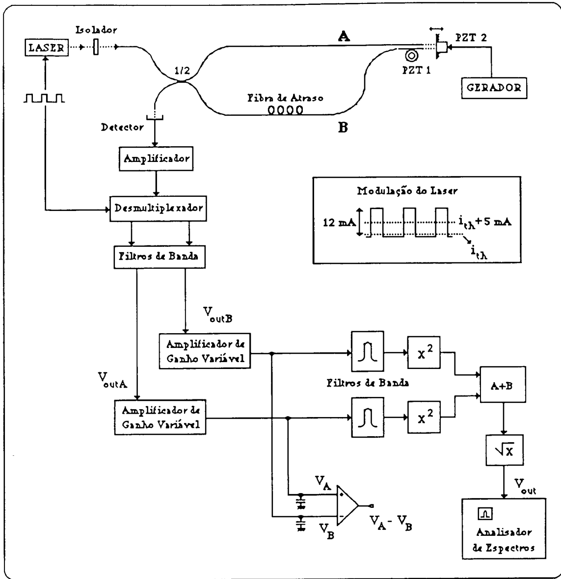
Figura 8.2. Esquema da experiência realizada.
