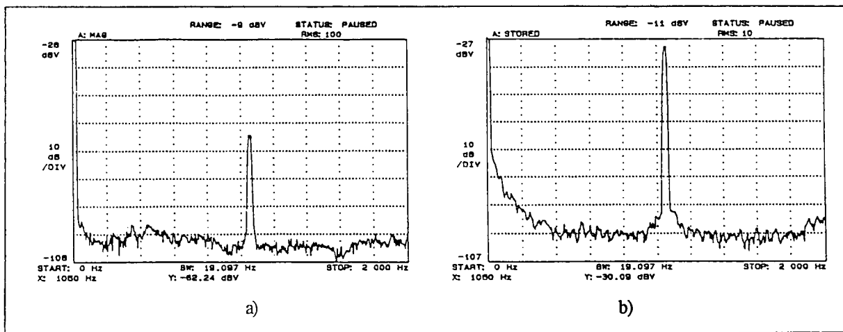
Figura 8.8. Sinal " V_{out} " quando um sinal de teste a 500 Hz foi aplicado ao PZT 2, originando sinais de fase com amplitudes de 5 mrad (a) e de 100 mrad (b).
