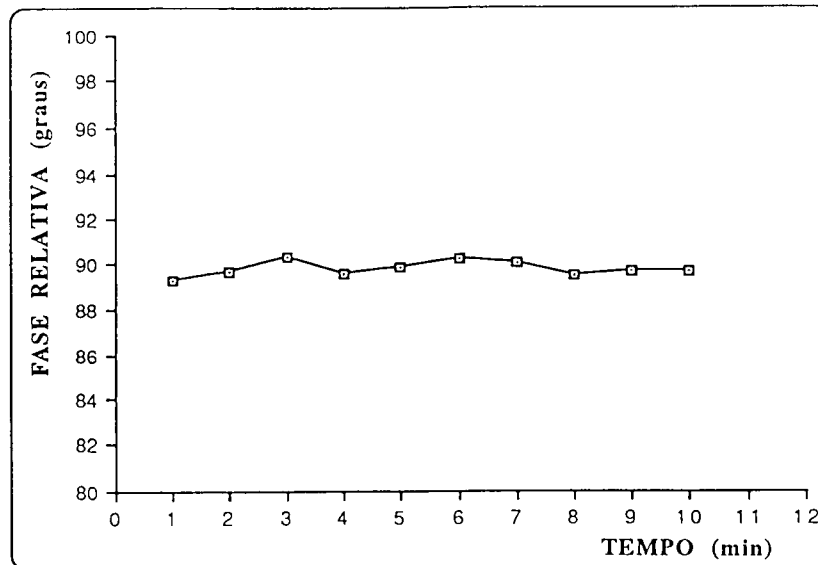
Figura 8.7. Variação temporal da fase relativa " \phi_A - \phi_B " dos dois interferômetros.
