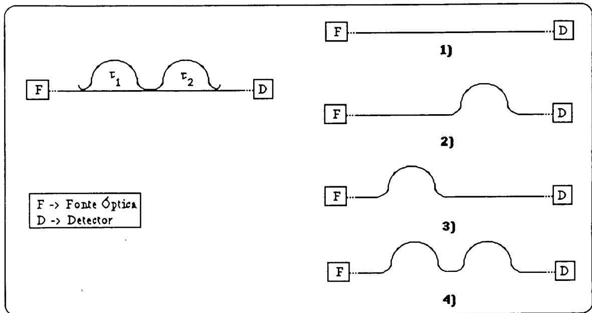
Figura 7.3. Percursos possíveis entre a fonte óptica e o detector, para a radiação que se propaga através de dois interferômetros com atrasos diferenciais " \tau_1 " e " \tau_2 ".
