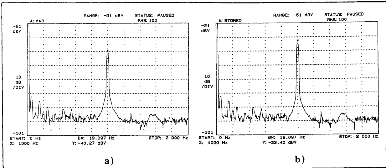
Figura 8.11. Sinal " V_{out} " quando é aplicado à cavidade um sinal de fase de 5 mrad (valor eficaz) a 1 kHz. Para o caso b, a potência óptica injectada no sistema é, relativamente ao caso a, o dobro.
