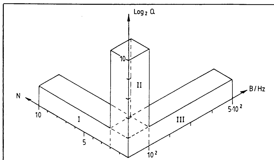
Figura 2.1. Cubo de informação representando "K" para três tipos diferentes de redes de sensores.
