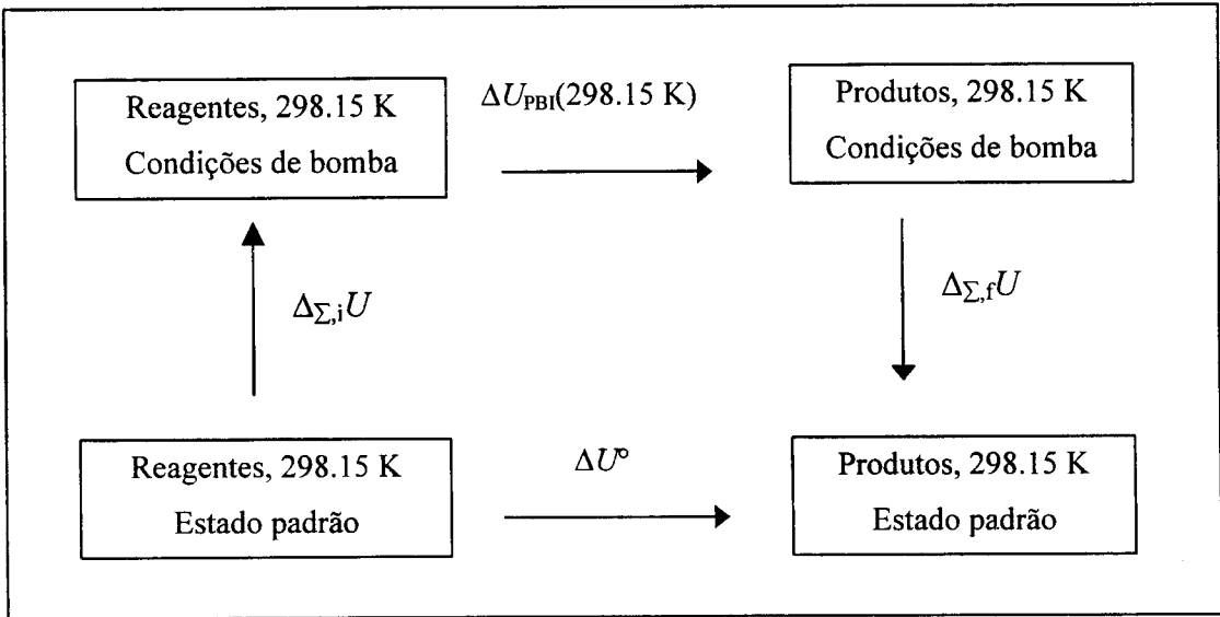
Figura 3.8- Esquema para a conversão do valor de \Delta U_{\text{PBI}}(298.15 \text{ K}) às condições padrão.
