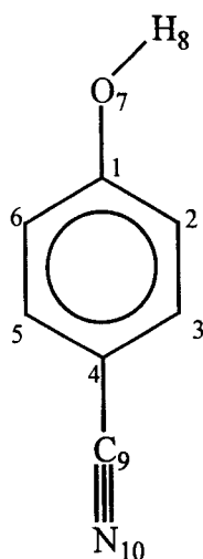
Figura 7.3- Esquema de numeração dos átomos nos isómeros cianofenol.
