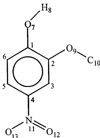
Figura 7.7- Esquema de numeração dos átomos nos metoxinitrofenóis.
