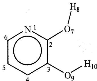
Figura 7.9- Esquema de numeração dos átomos nas mono- e dihidroxipiridinas.
