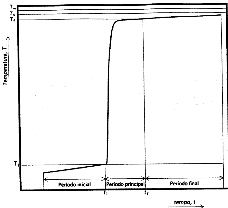
Figura 3.6- Curva T = f(t) para uma experiência de combustão.
