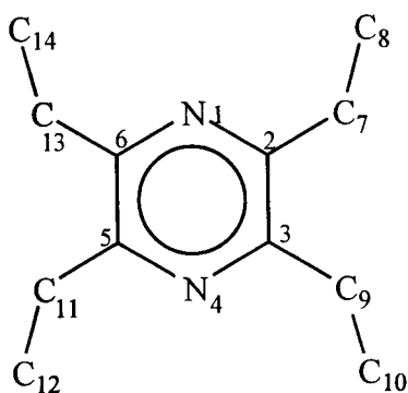
Figura 7.10- Esquema de numeração dos átomos nas etilpirazinas.
