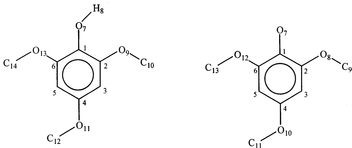
Figura 7.2- Esquema de numeração dos átomos nos metoxifenóis e respectivos radicais e aniões.
