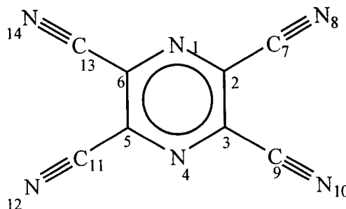
Figura 7.12- Esquema de numeração dos átomos nas cianopirazinas.
