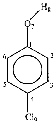
Figura 7.4- Esquema de numeração dos átomos nos isómeros clorofenol.
