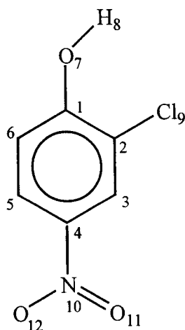
Figura 7.6- Esquema de numeração dos átomos nos cloronitrofenóis.
