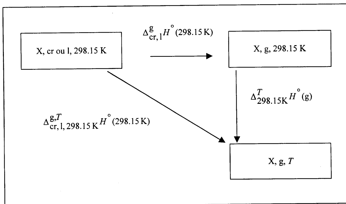
Figura 4.4- Ciclo termoquímico para o cálculo de entalpias de sublimação ou de vaporização padrão, a T = 298.15 \text{ K} .
