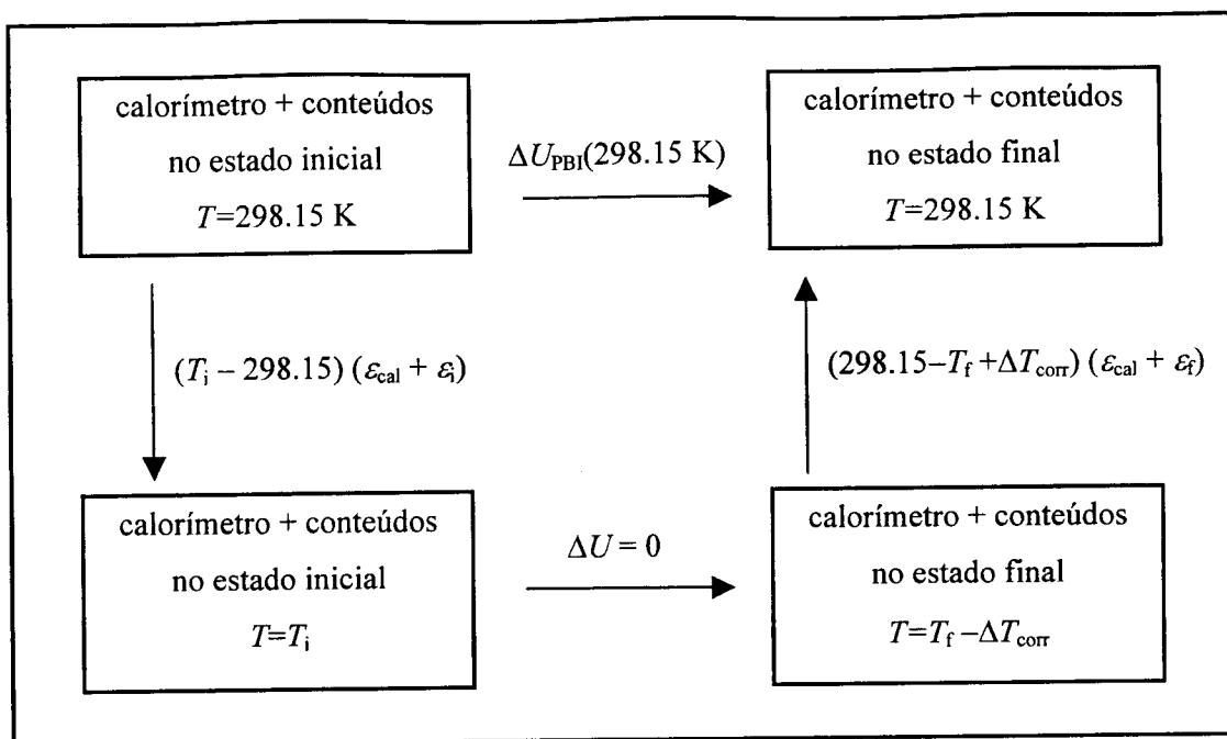
Figura 3.7- Ciclo termoquímico para o cálculo da variação de energia interna associada ao processo de bomba, a 298.15 K, \Delta U_{\text{PBI}}(298.15 \text{ K}) .
