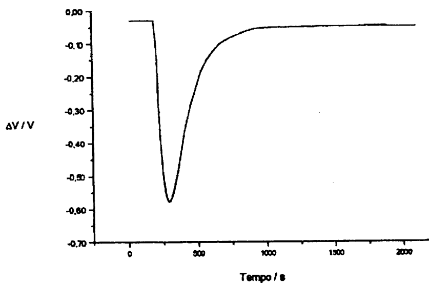
Figura 4.3- Termograma típico obtido para um processo endotérmico.
