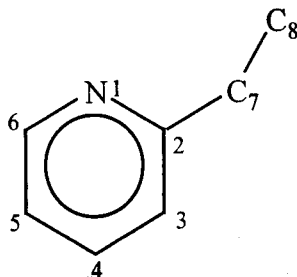
Figura 7.8- Esquema de numeração dos átomos nas etilpiridinas.
