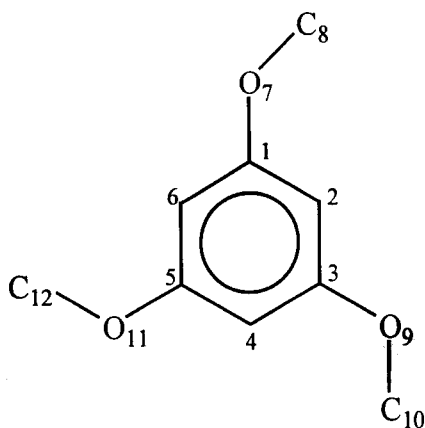
Figura 7.1- Esquema de numeração dos átomos nos metoxibenzenos.
